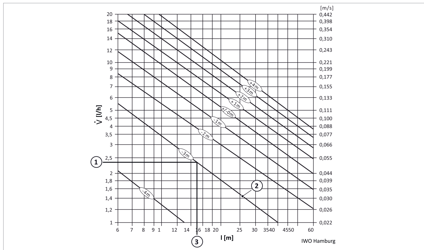
Fig. 72: Lunghezza massima della tubazione nel sistema a linea unica in funzione della prevalenza
