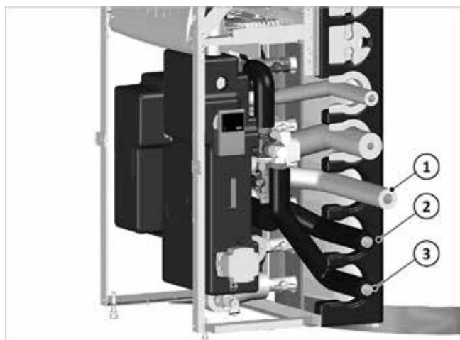
Fig. 75: Collegamento idraulico SolvisLea
