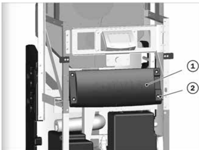
Fig. 95: fissaggio del coperchio del gruppo di rete
