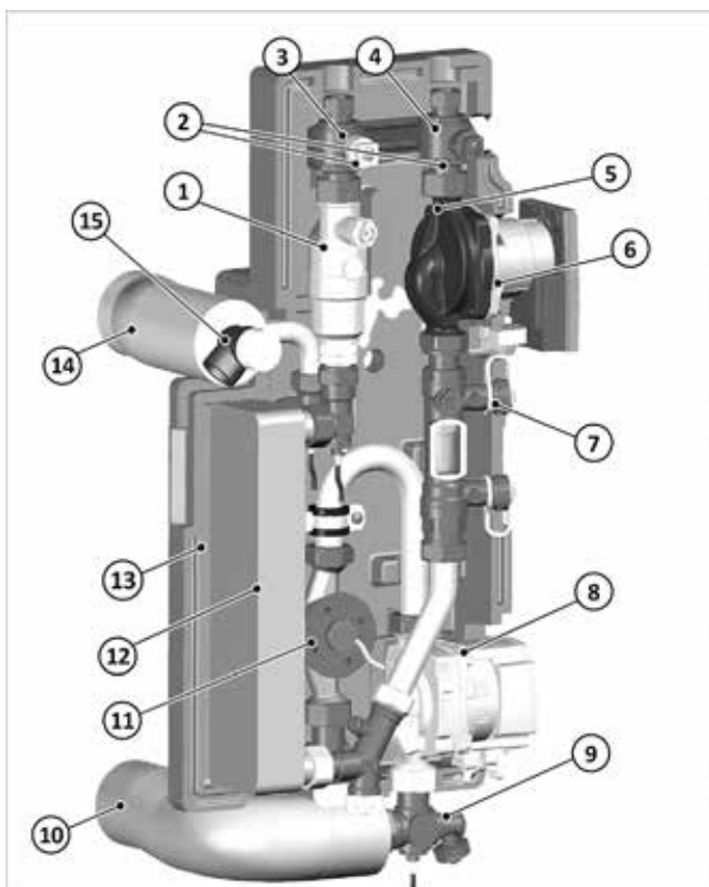
Fig. 81: panoramica dei componenti della stazione di trasmissione del calore solare
