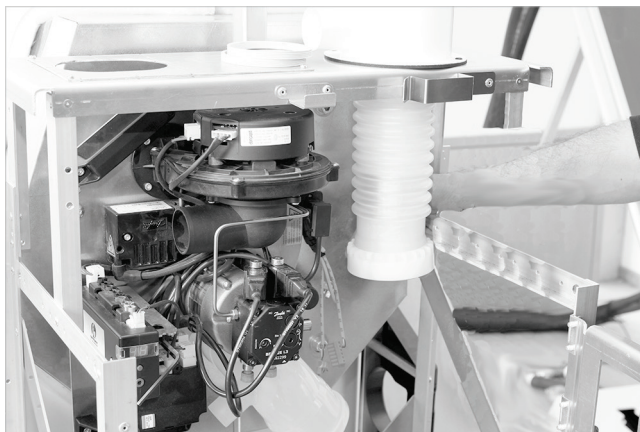
Fig. 61 : positionnement droit du raccord d'évacuation des gaz
