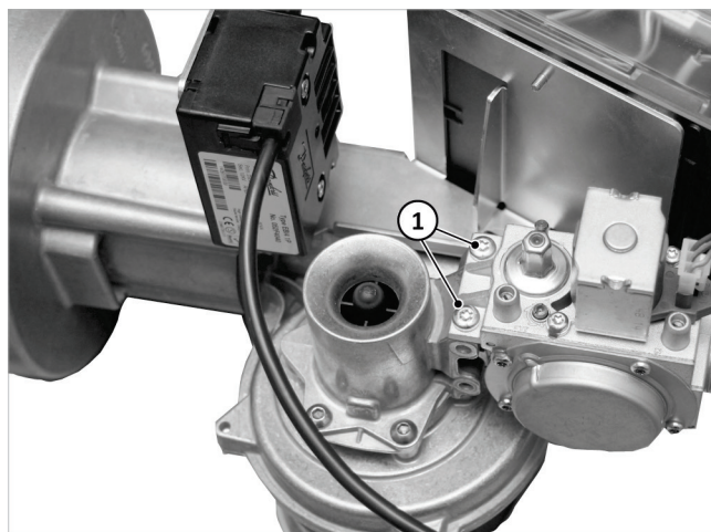
Fig.21 : Démontez la vanne mixte à gaz
