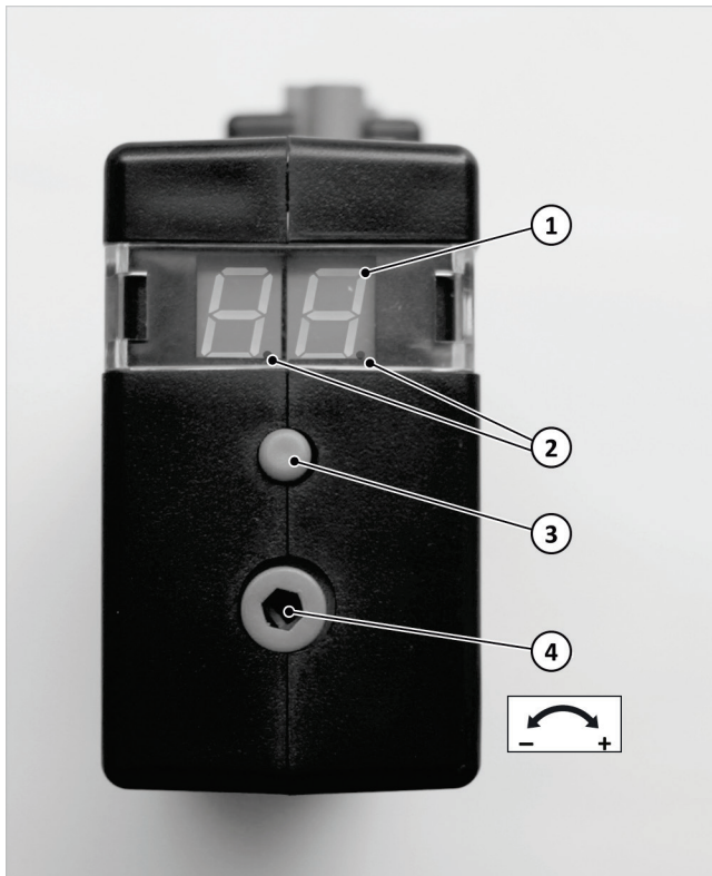
Fig. 121 : interface du dispositif d'allumage automatique CM 168
