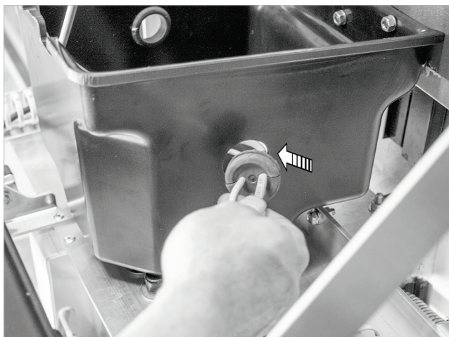
Fig. 32 : passage étanche du câble du brûleur
