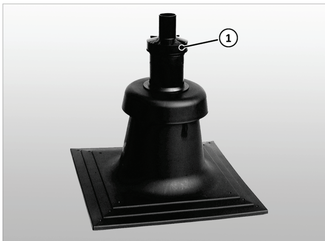
Fig. 73 : Silencieux à réflexion installé
