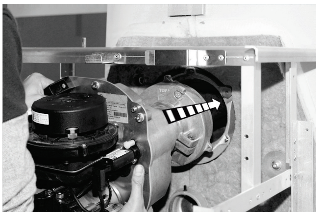
Fig. 55 : montage du brûleur
