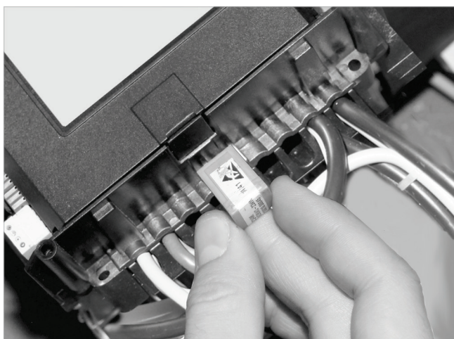
Fig. 24 : Installation de la carte à puce du brûleur
