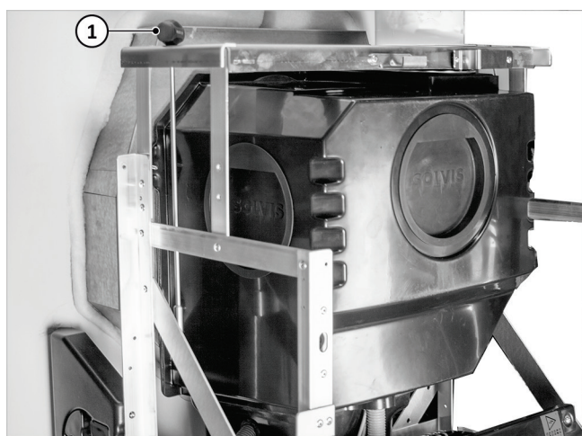
Fig. 46 : clé à douille en position rangée
