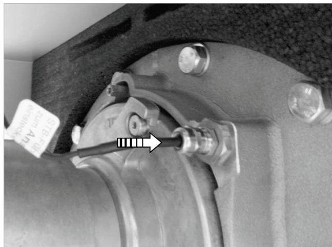
Fig. 68 : montage du dispositif mSTB
