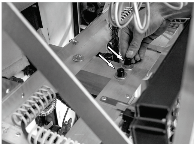
Fig. 30 : couvrir les têtes de vis de la console
