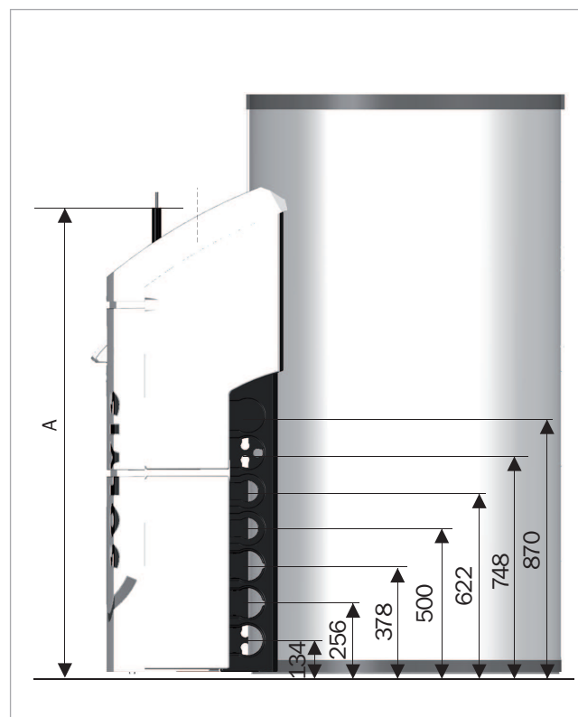
Fig. 124 : Vue latérale
