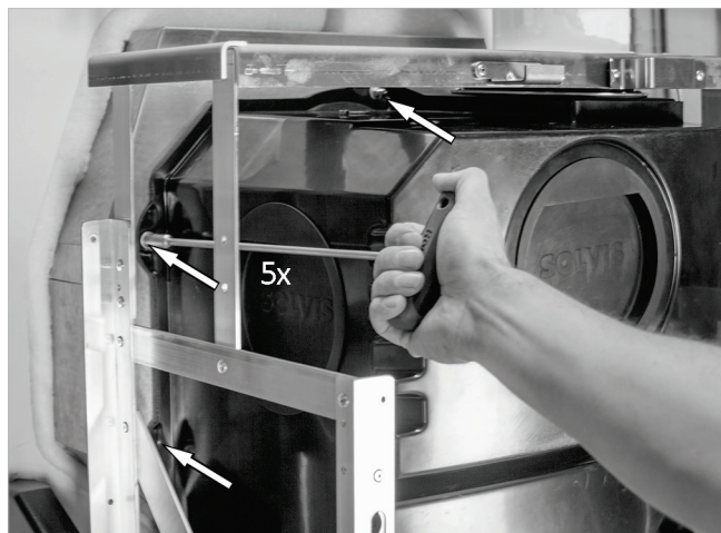
Fig. 45 : visser le couvercle de la chambre d'aspiration
