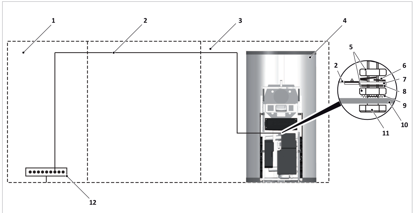
Fig. 89 : liaison équipotentielle du SolvisMax
