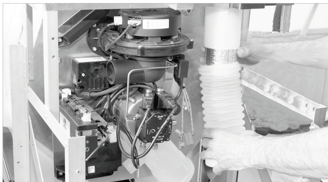
Fig. 60 : mise en place du raccord d'évacuation des gaz
