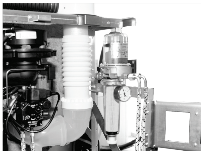
Fig. 66 : Raccordement des conduites de fioul
