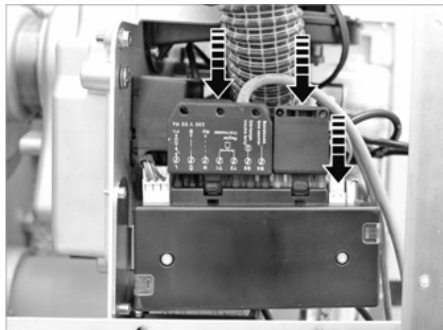
Fig. 71 : branchement des connecteurs
