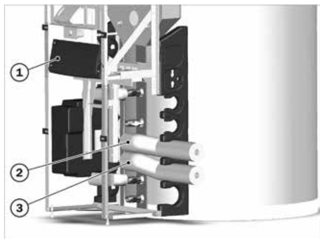
Fig. 76 : raccordement hydraulique des circuits de chauffage
