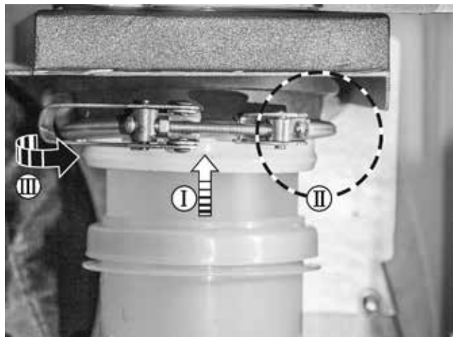
Fig. 36 : montage du collier de serrage
