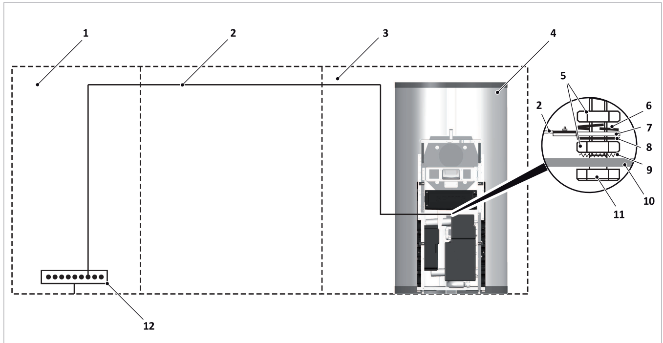
Fig. 89 : liaison équipotentielle du SolvisMax
