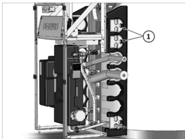
Fig. 67 : amener la conduite de fioul par la réduction de trois
