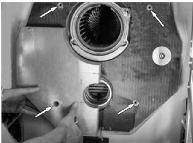
Fig. 25 : Montage de l'isolation avant de la bride
