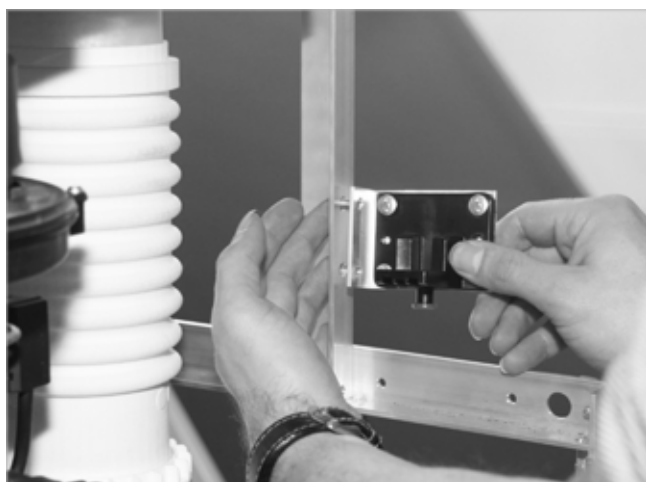
Fig. 64 : Fixation du support du filtre à fioul
