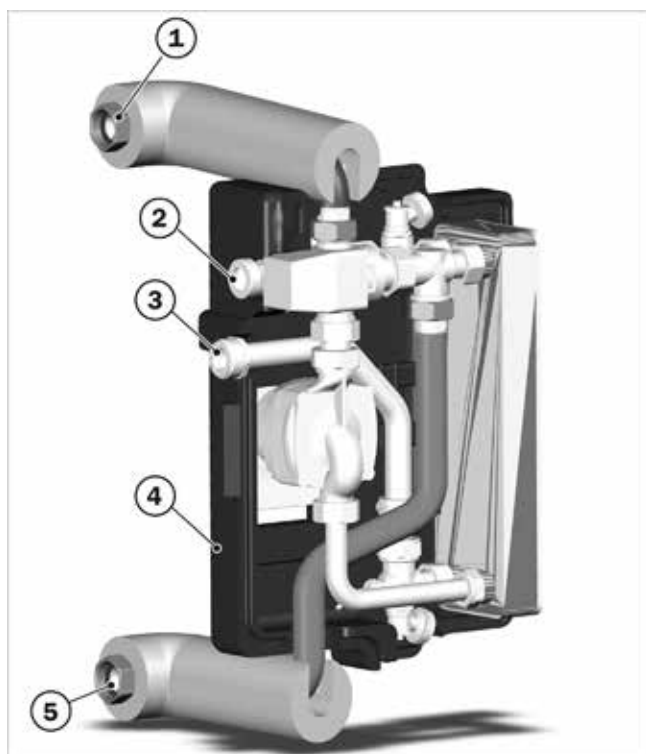
Fig. 77 : raccordement de WWS-24
