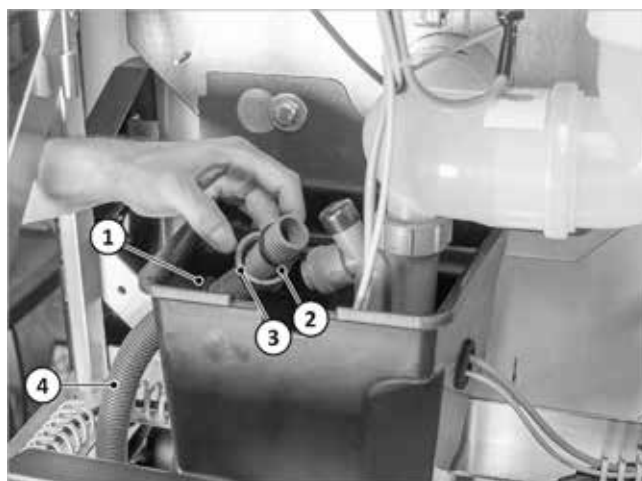
Fig. 40 : Passage et raccord du tuyau de condensat dans l'orifice
