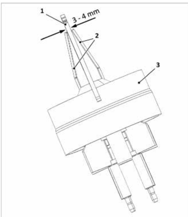
Fig. 52 : contrôle de l'écartement des électrodes d'allumage
