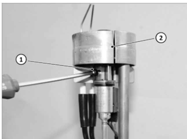
Fig. 115 : Tête mélangeuse du porte-vent
