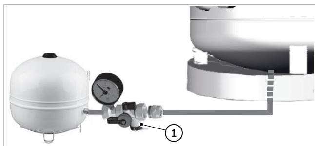
Fig. 96 : groupe de raccordement robinet RRV sur VEM
