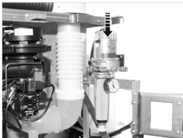
Fig. 65 : filtre à fioul en place
