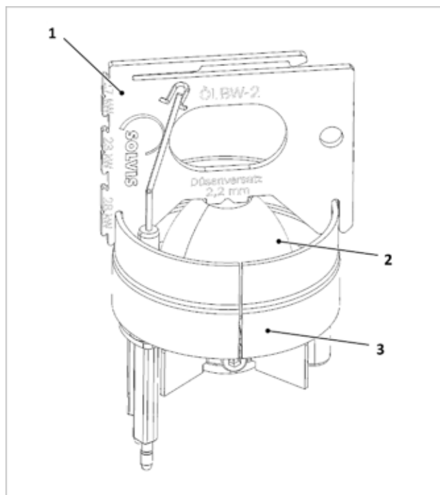
Fig. 117 : Tête mélangeuse avec gabarit de réglage
