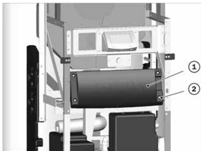
Fig. 95 : Fixez le couvercle de l'élément de réseau
