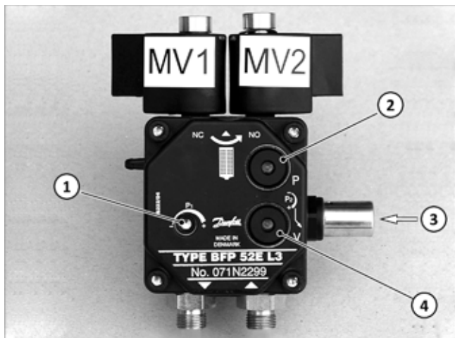
Fig. 98 : Réglage de la pression de la pompe à fioul
