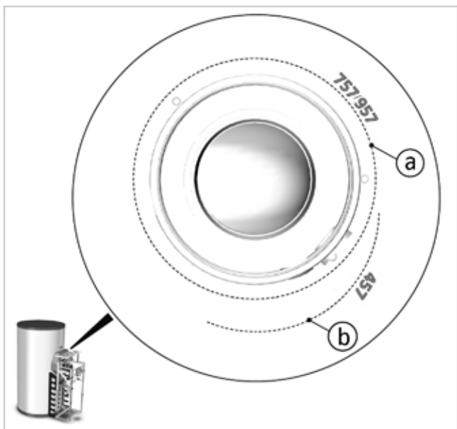
Fig. 35 : position du raccord d'évacuation des gaz
