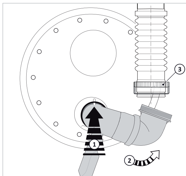
Fig. 62 : montage du coude d'évacuation des gaz
