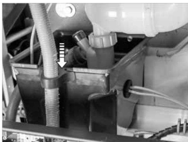
Fig. 44 : fixer la conduite de gaz au bac avec le clip de fixation
