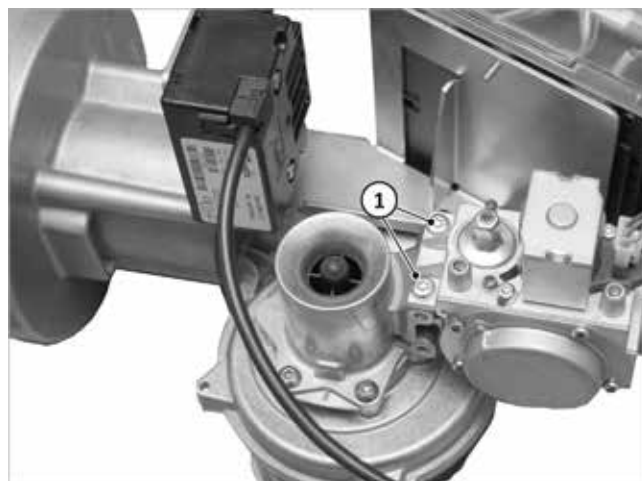
Fig.21 : Démonter la vanne mixte à gaz
