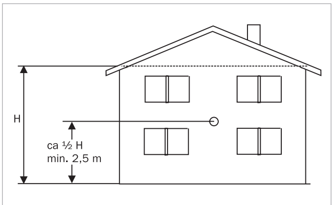
Fig. 90 : position du capteur extérieur
