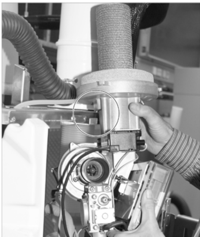
Fig. 109 : brûleur en position de maintenance sur la console
