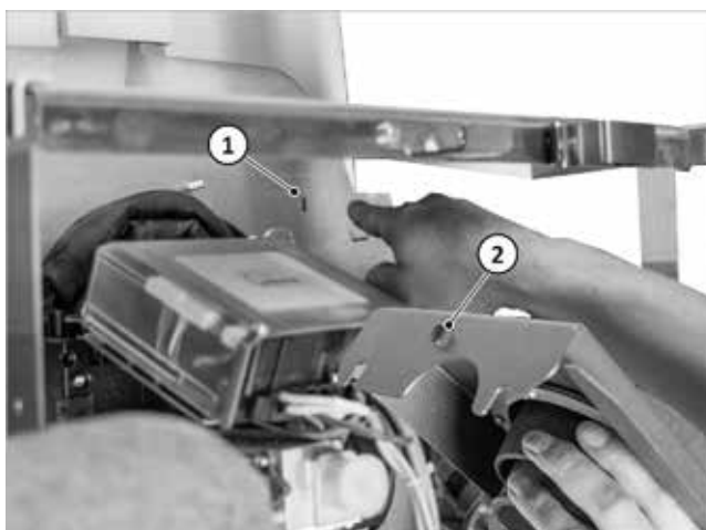
Fig. 33 : insérer le support du soufflet d'étanchéité
