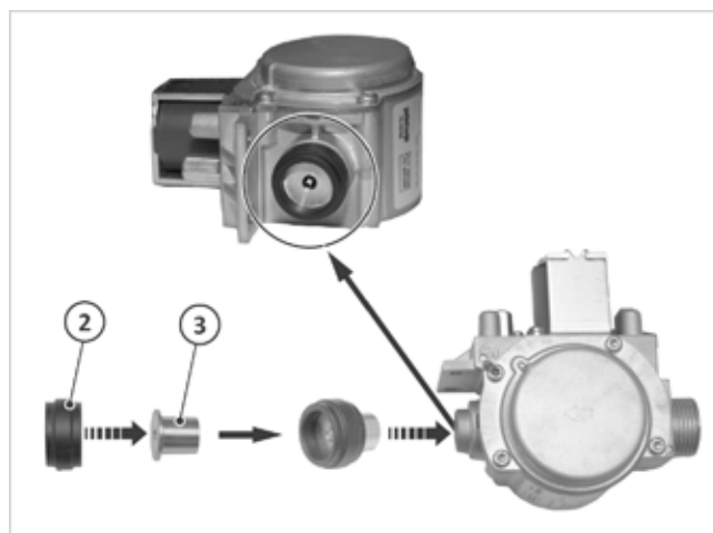
Fig.22 : Monter la buse à gaz liquide
