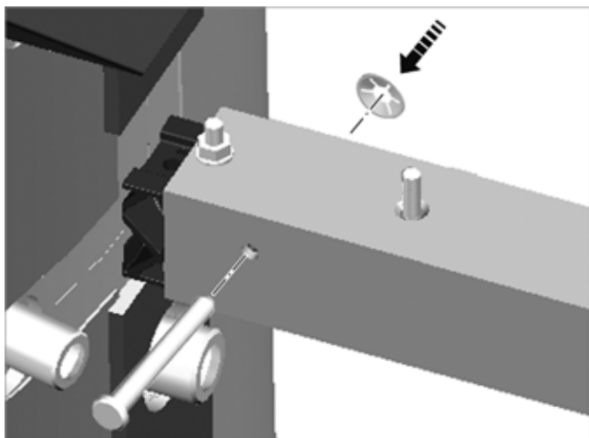
Fig.10 : goujon et rondelle d'arrêt
