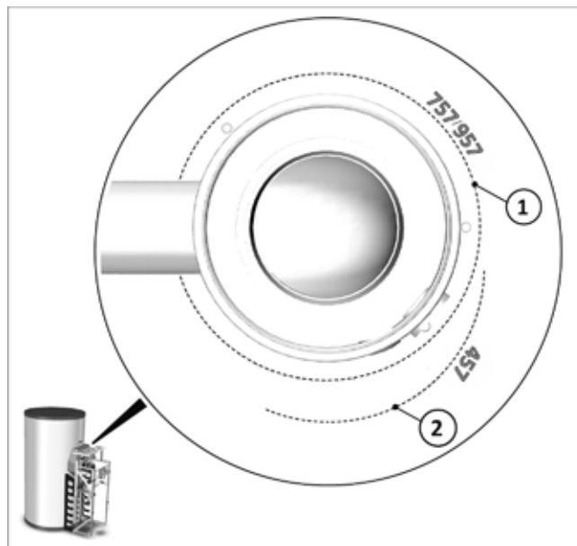
Fig. 57 : position du raccord d'évacuation des gaz
