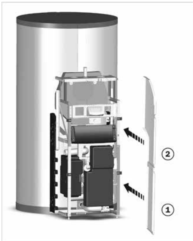
Fig. 107 : faire glisser d'abord l'élément latéral inférieur (1)
