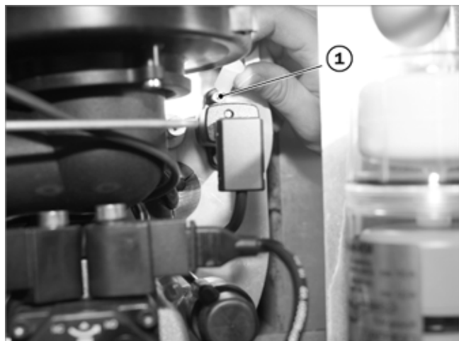
Fig. 101 : mesure de la pression de la soufflante
