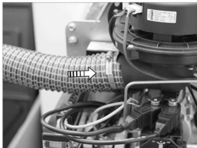
Fig. 56 : Fixation du tuyau d'amenée d'air sur la soufflante
