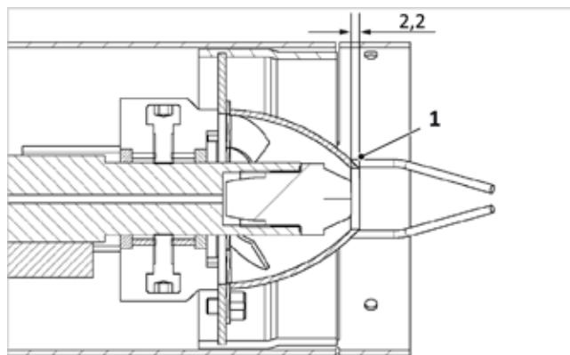
Fig. 116 : section de la tête mélangeuse
