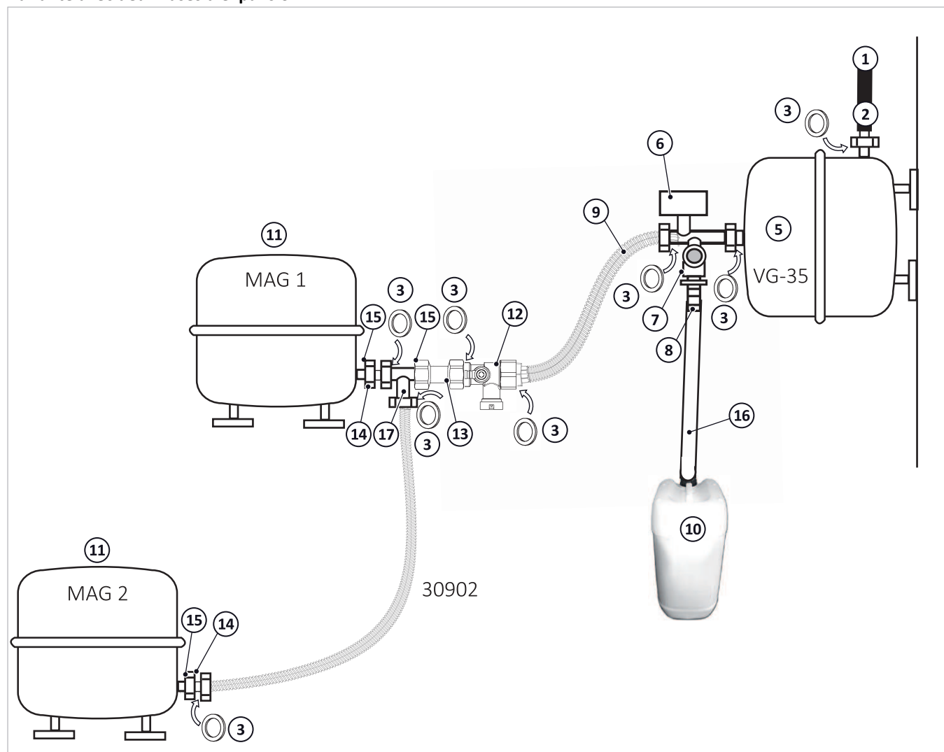
Fig. 88: raccordement du deux vases d'expansion à membrane solaire
