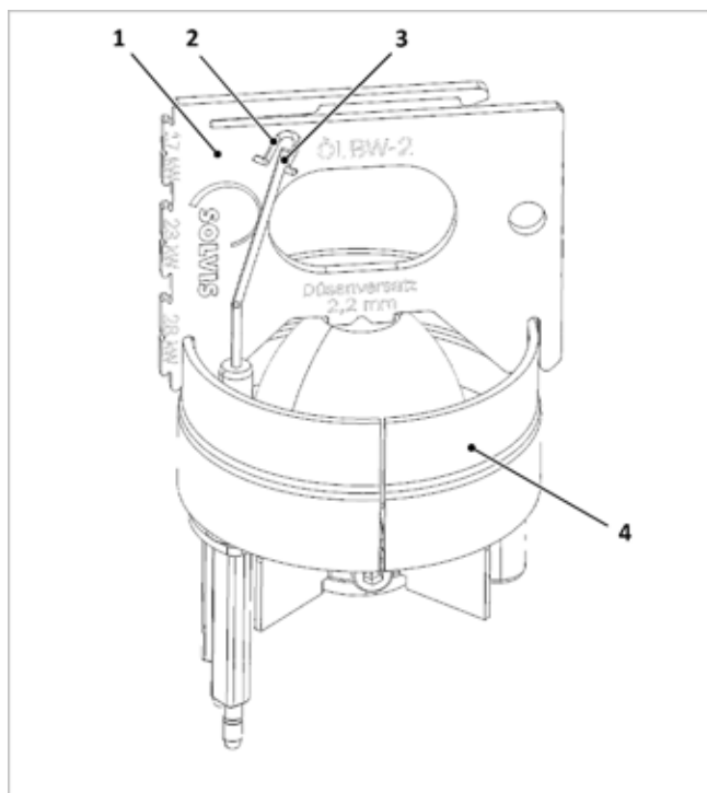
Fig. 51 : Contrôle de la position des électrodes d'allumage
