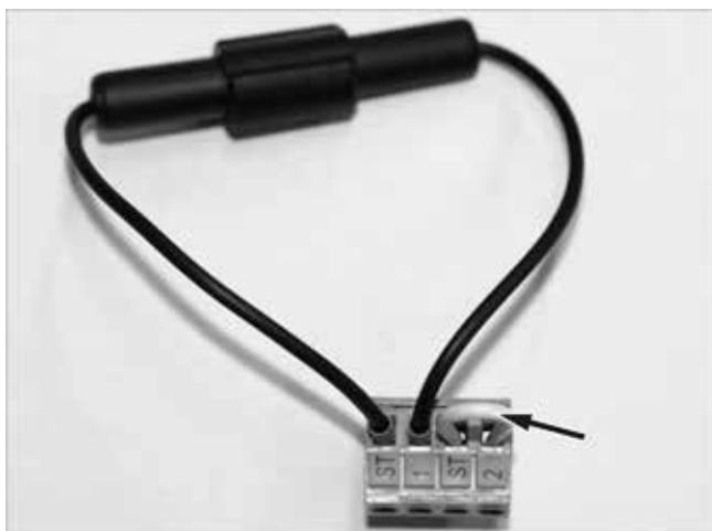
Fig. 42 : connecteur femelle avec sécurité (noir) pour brûleur SX-LN-3 (raccordement ASTB voir flèche)
