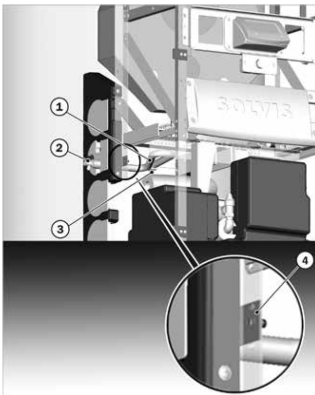
Fig.20 : le raccord de purge doté d'un tube ondulé
