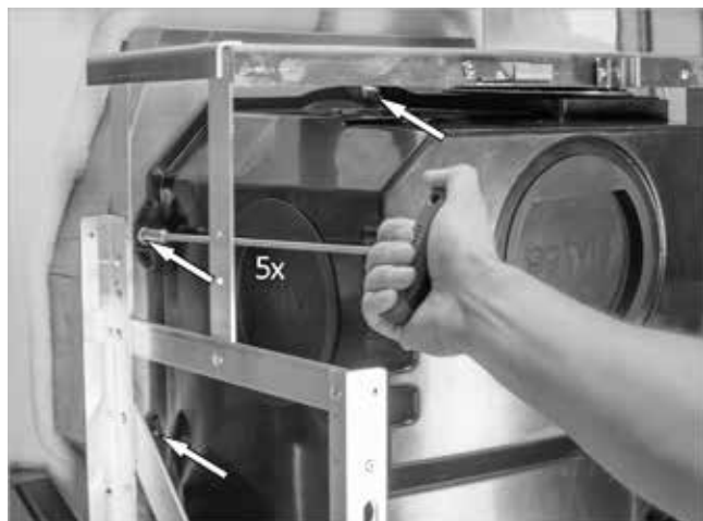
Fig. 45 : visser le couvercle de la chambre d'aspiration
