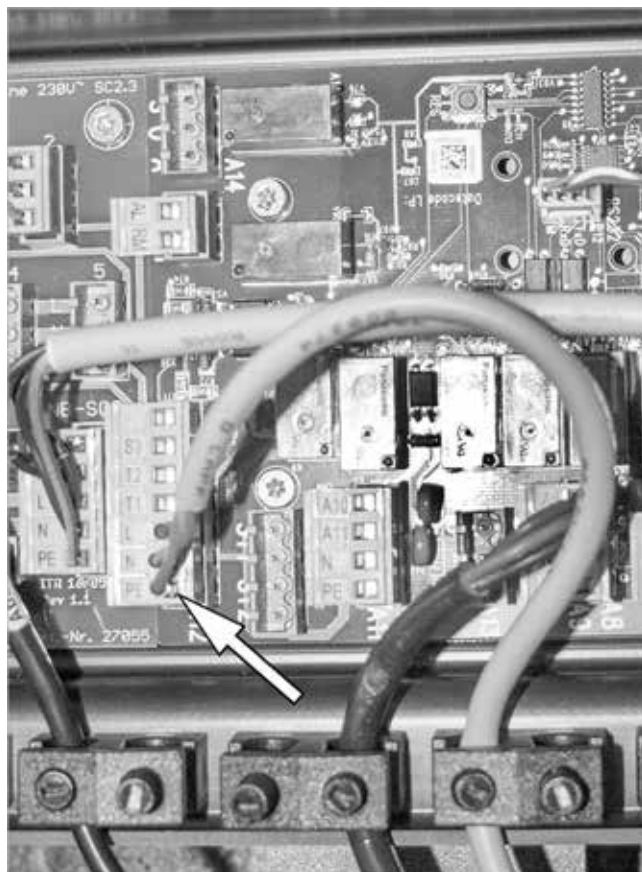
Fig. 47 : raccordement du connecteur du brûleur à gaz sur A12
