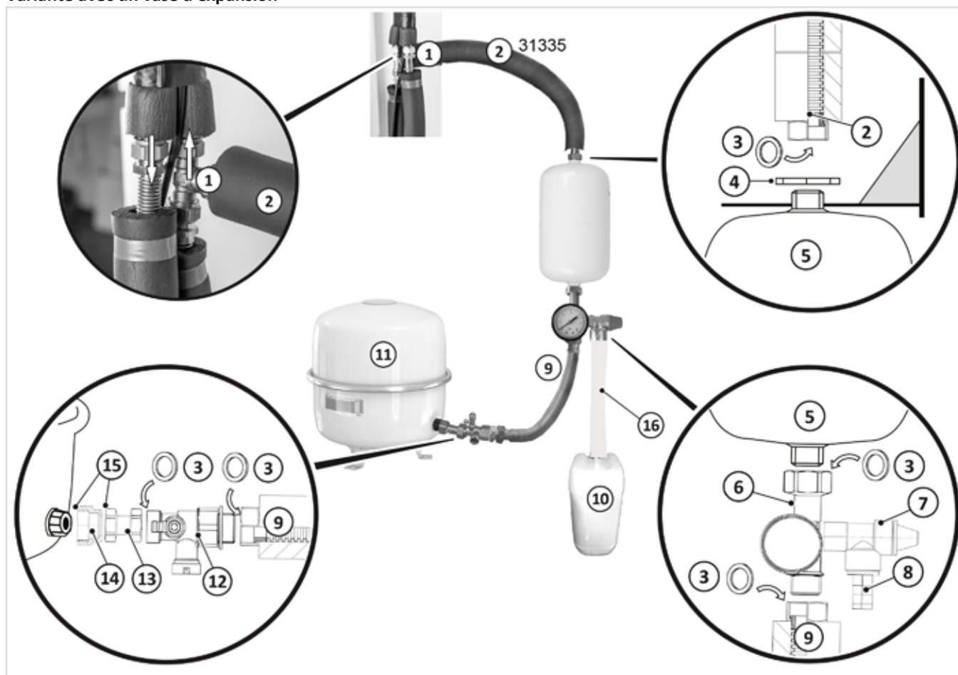
Fig. 87 : raccordement du vase d'expansion à membrane solaire
