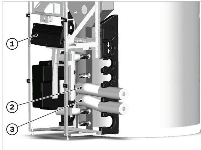
Afb.76: Hydraulische koppeling van de verwarmingsgroepen
