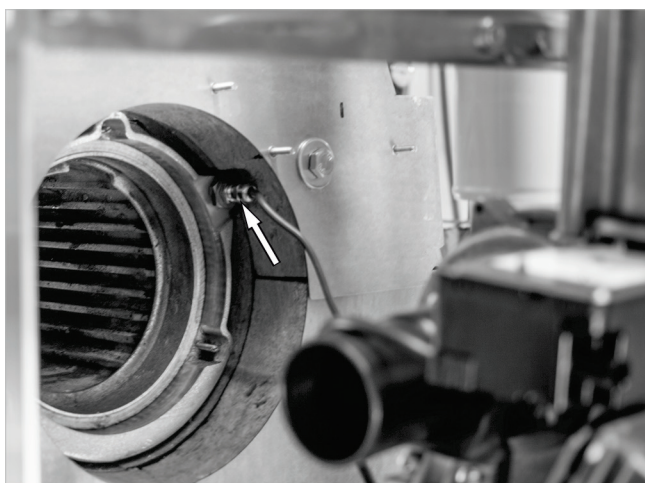
Afb. 27: eSTB insteken
