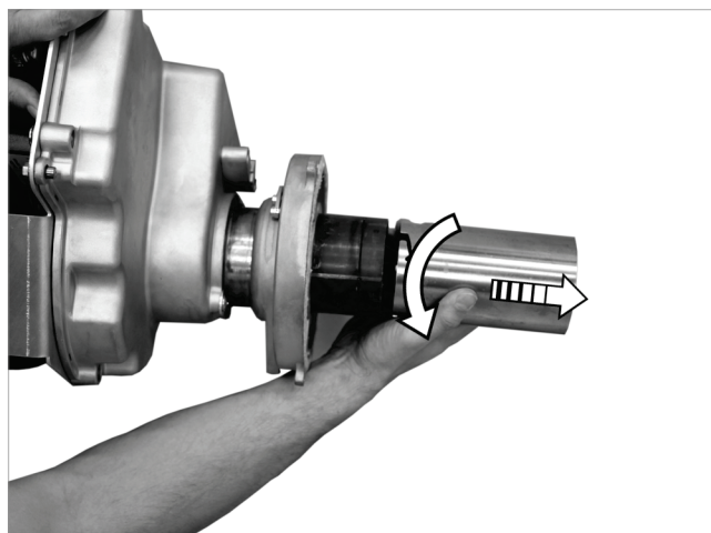
Afb. 50: Vlamhuis van de branderkop verwijderen
