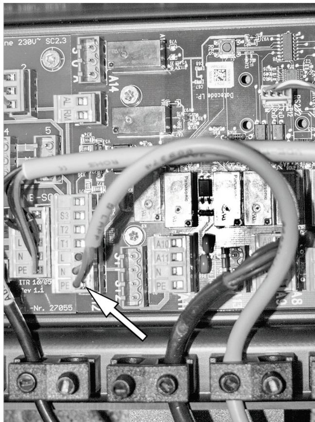
Afb. 47: Aansluiting branderstekker gasbrander op A12
