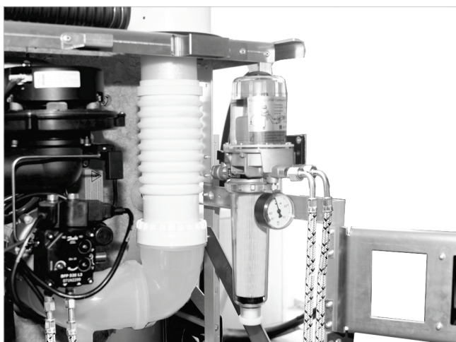
Afb. 66: Olieleidingen aansluiten
