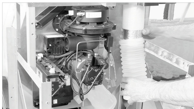
Afb.60: Rookgasaansluitstuk opsteken
