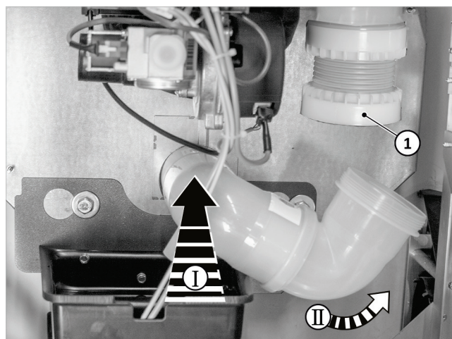
Afb. 38: De rookgasbocht monteren
