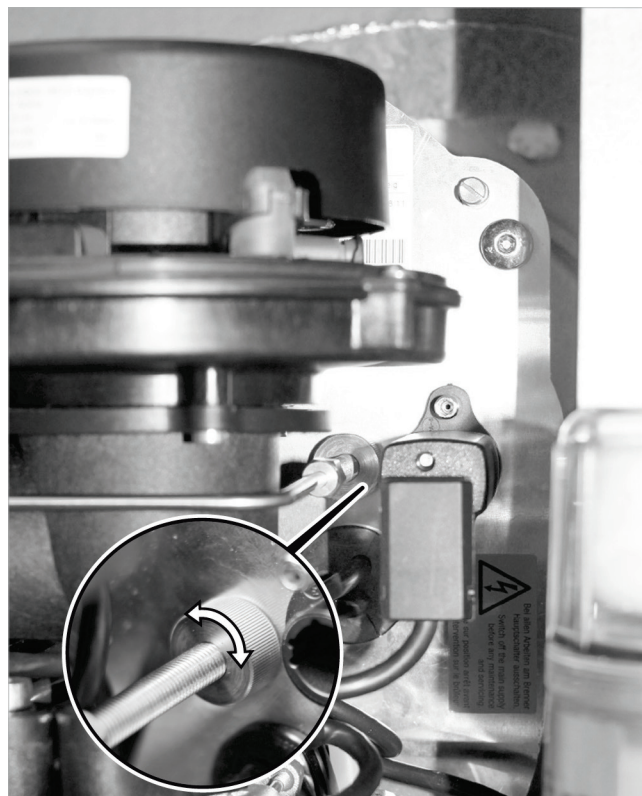
Afb. 120: Kartelmoer (aansluiting olieleiding/sproeierblok)
