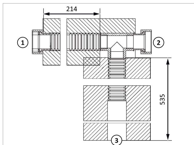
Afb.83: Aansluitleiding ketel voor vaste brandstof (RO-FBK-RL)
