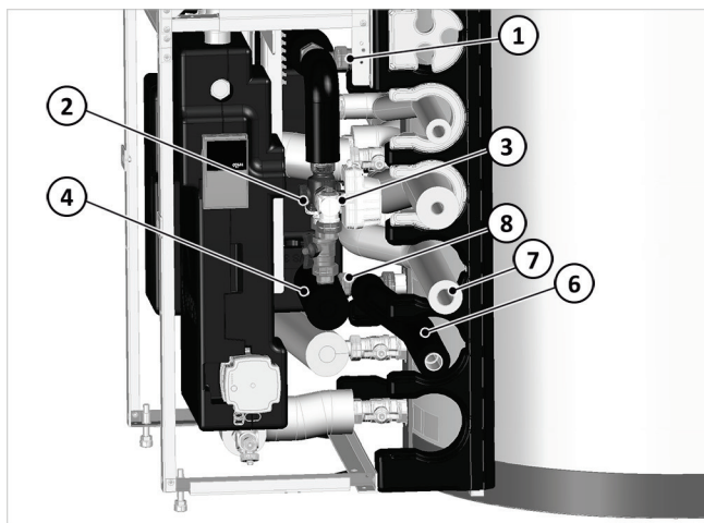
Afb.15: omschakelventiel monteren WP-aanvoer naar rechts
