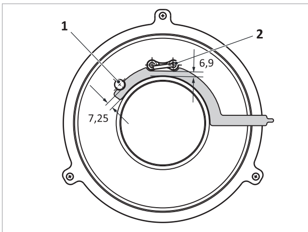
Afb. 110: Afstanden ionisatie- en ontstekingselektrode naar brandervezellaag
