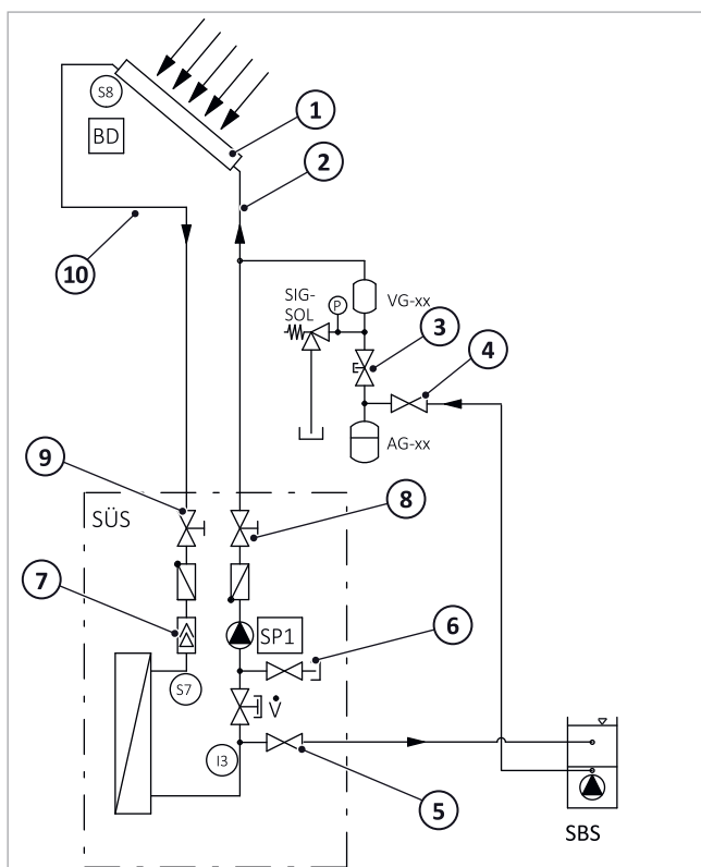
Afb. 103: Zonnewarmte-overdrachtsgroep: Spoelen van de warmtewisselaar
