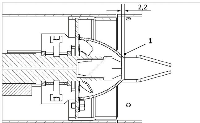
Afb. 116: Dwarsdoorsnede van mengkop
