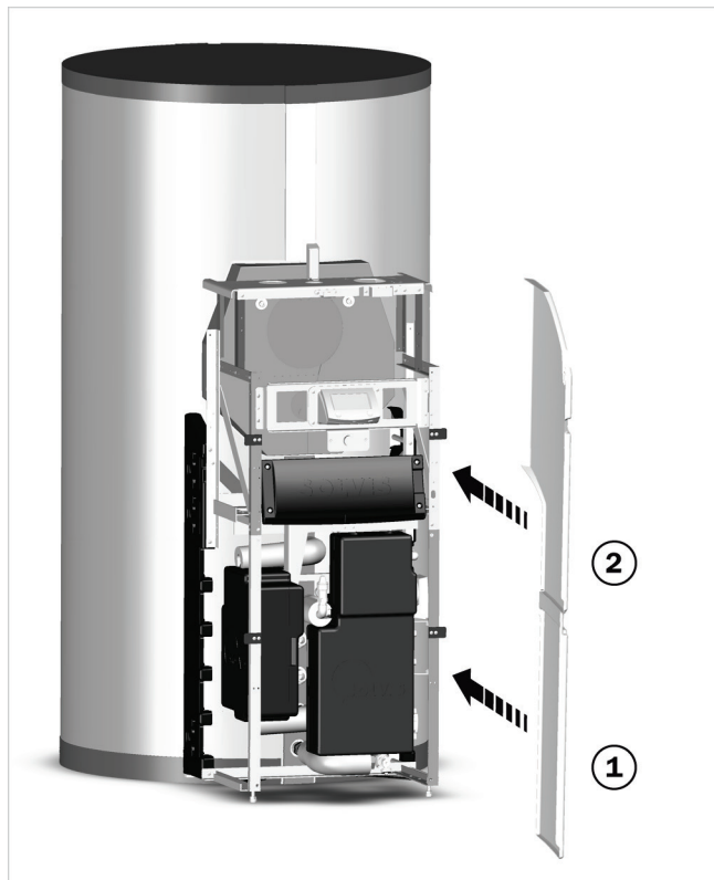
Afb. 107: Onderste zijdeel (1) er eerst inschuiven
