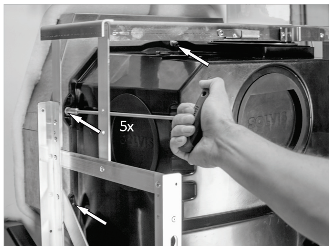
Afb. 45: Afdekking aanzuigkamer vastschroeven
