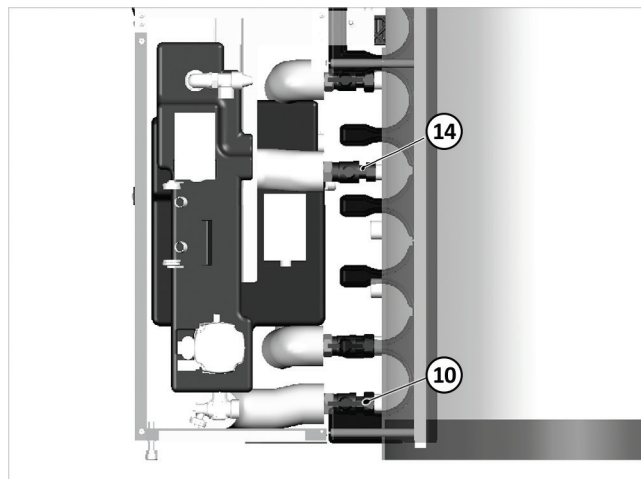
Afb.82: Zonnewarmte-overdrachtsgroep aansluiten
