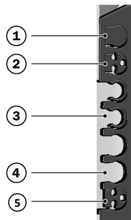
Afb.41: Inzetstukken van de leidingdoorvoeren
