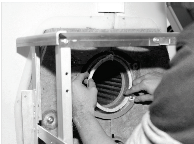
Afb. 49: Branderpakkingsnoer plaatsen, kopse kanten boven
