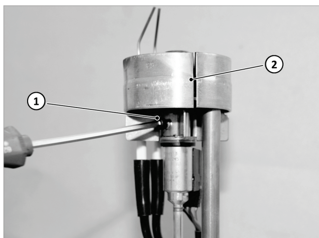
Afb. 115: Mengkop op het sproeierblok
