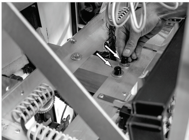
Afb. 30: Boutkoppen op console bedekken
