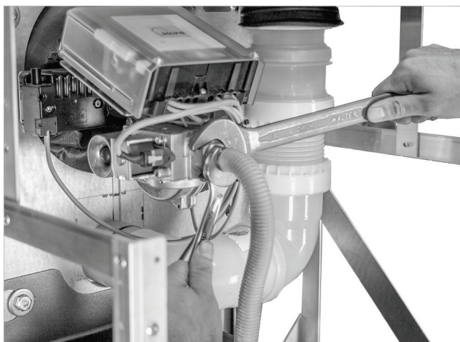
Afb. 43: Gasleiding aansluiten
