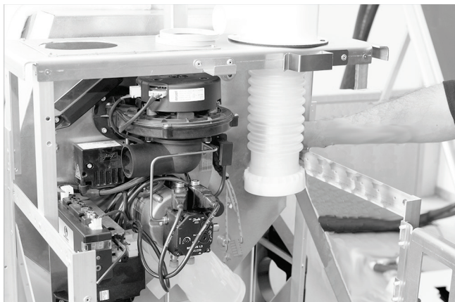
Afb. 61: Rookgasaansluitstuk recht uitlijnen.
