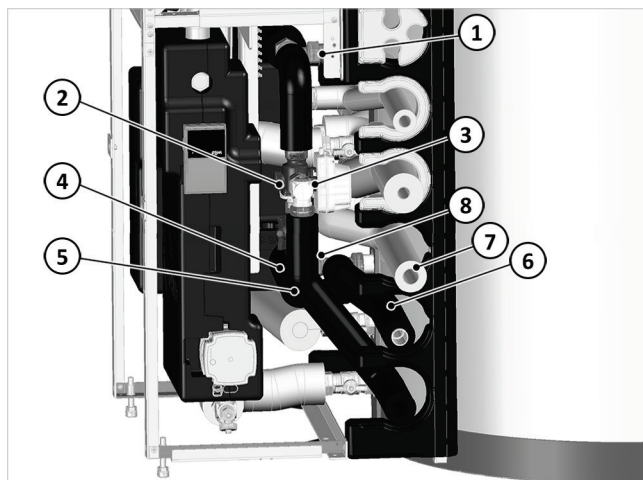
Afb.16: omschakelventiel monteren WP-aanvoer naar rechts
