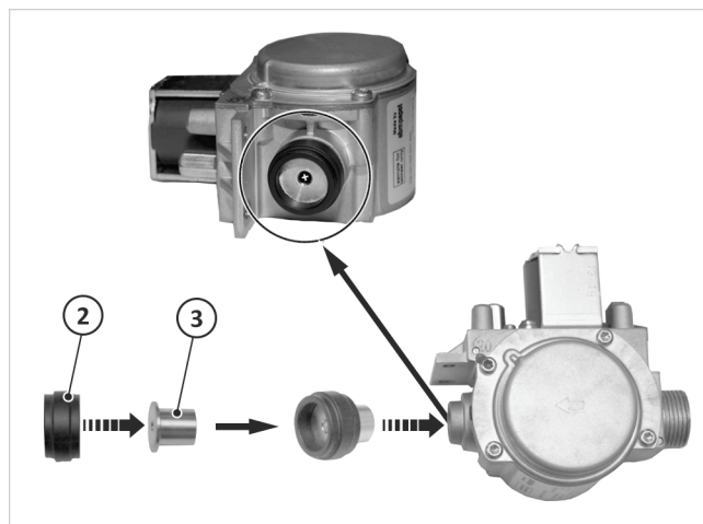
Afb. 22: Sproeier vloeibaar gas monteren
