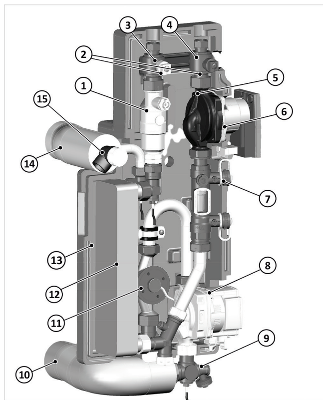
Afb.81: Overzicht component zonnewarmte-overdrachtsgroep
