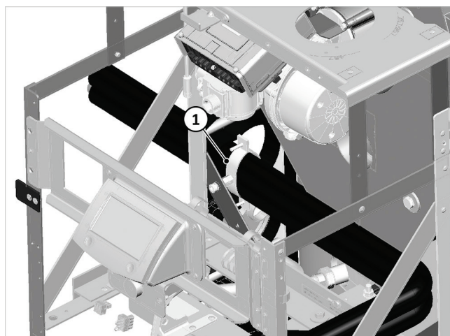
Afb. 86: Buizen bevestigen
