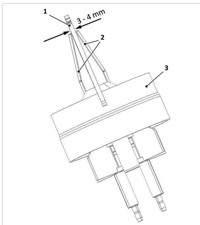
Afb. 52: De afstand van de ontstekingselektroden controleren
