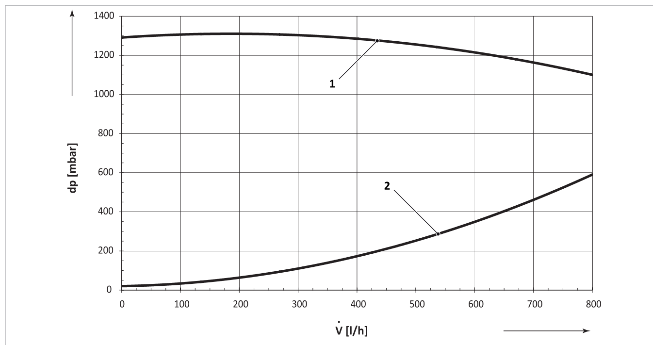
Afb. 127: drukverlieskromme van het primair circuit
