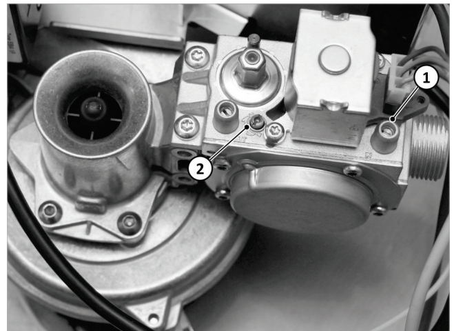
Afb. 97: Brander instellen
