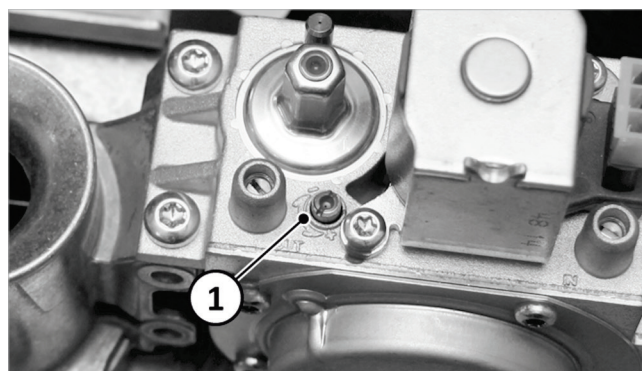
Afb. 23: Brander instellen
