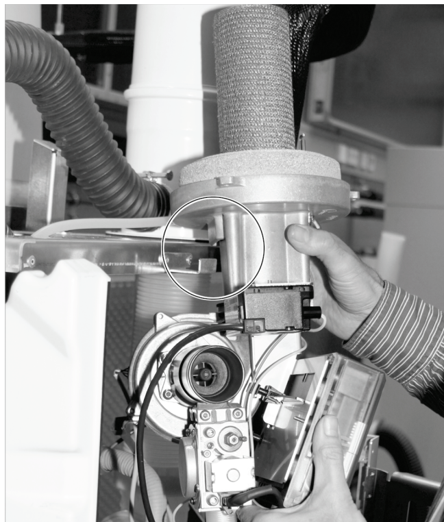
Afb. 109: Brander in onderhoudspositie aan de console
