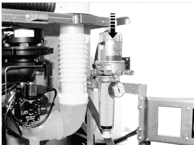
Afb. 65: Oliefilter opgestoken
