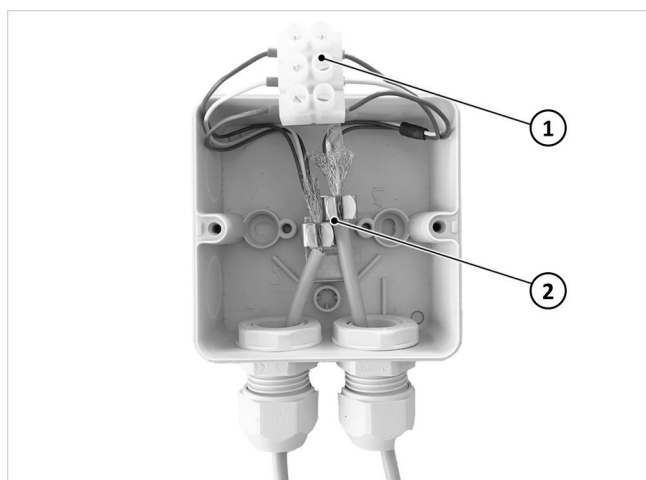
Afb. 94: Modbus-verbindingsdoos bevestigen
