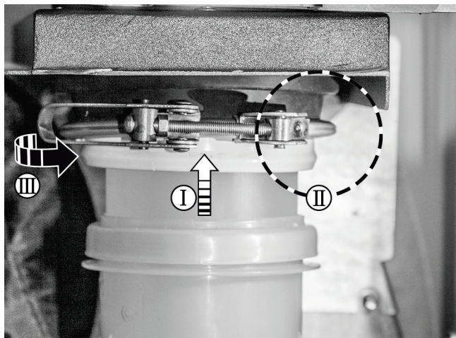
Afb. 36: Klem monteren
