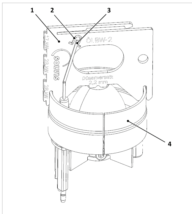
Afb. 51: Stand van de ontstekingselektroden controleren
