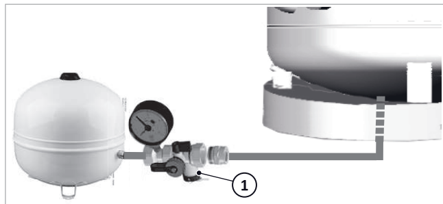
Afb. 96: KFE-kraan op MAG-aansluitgroep
