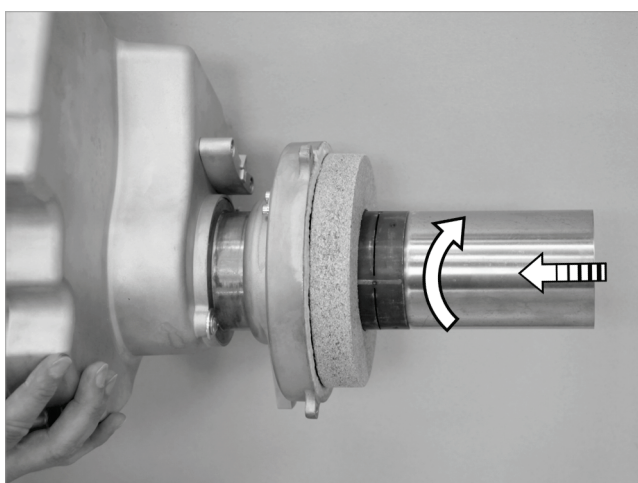
Afb. 54: Vlambuis plaatsen en vergrendelen
