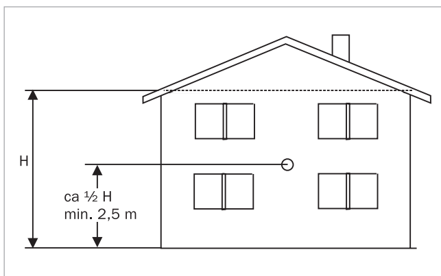
Afb. 90: Positie van de buitensensor
