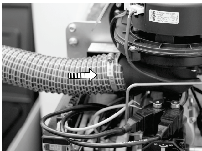
Afb. 56: Aanzuigluchtslang op de ventilator aansluiten
