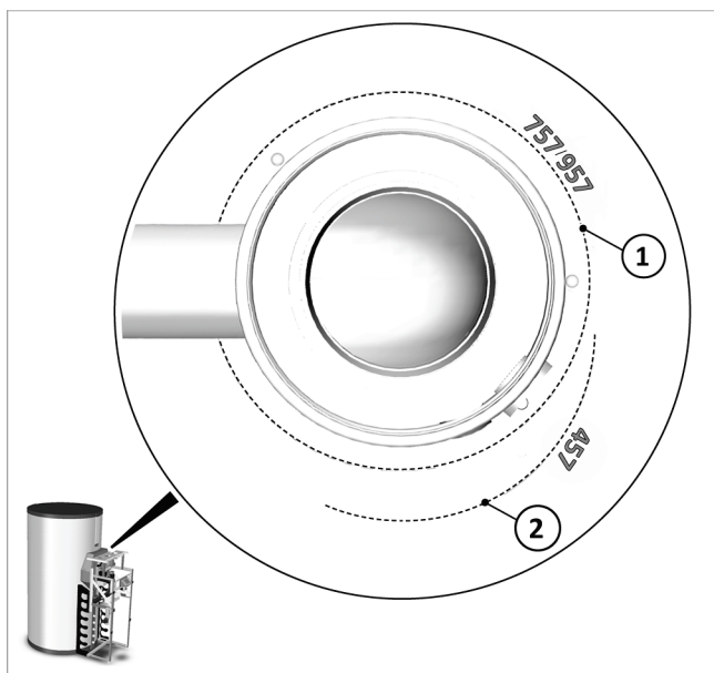
Afb.57: Positie Rookgasafvoeraansluitstuk
