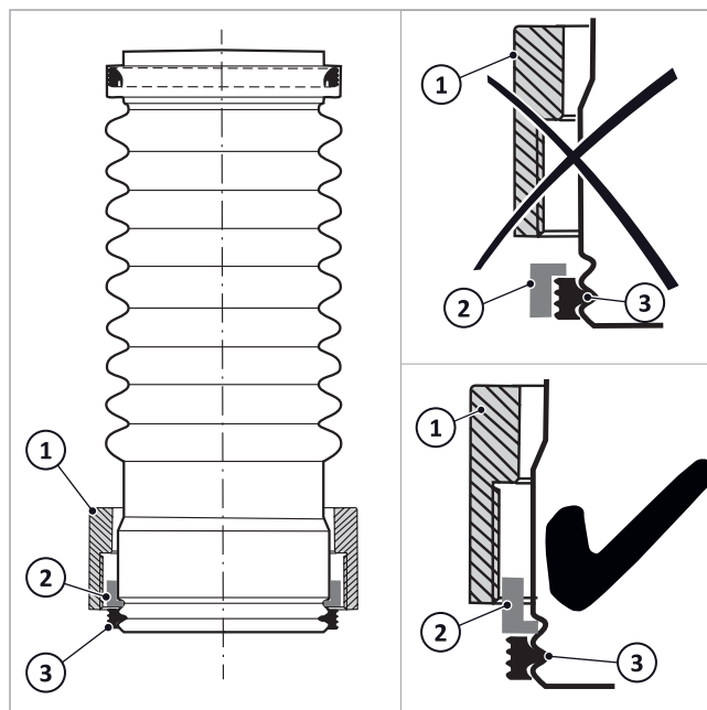
Afb. 37: Schroefkoppeling opgestoken
