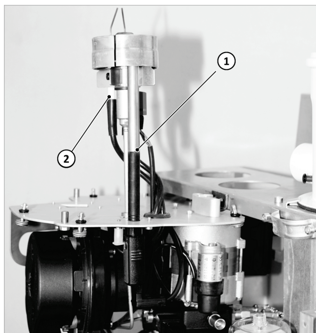
Afb. 114: Brander op console inhaken
