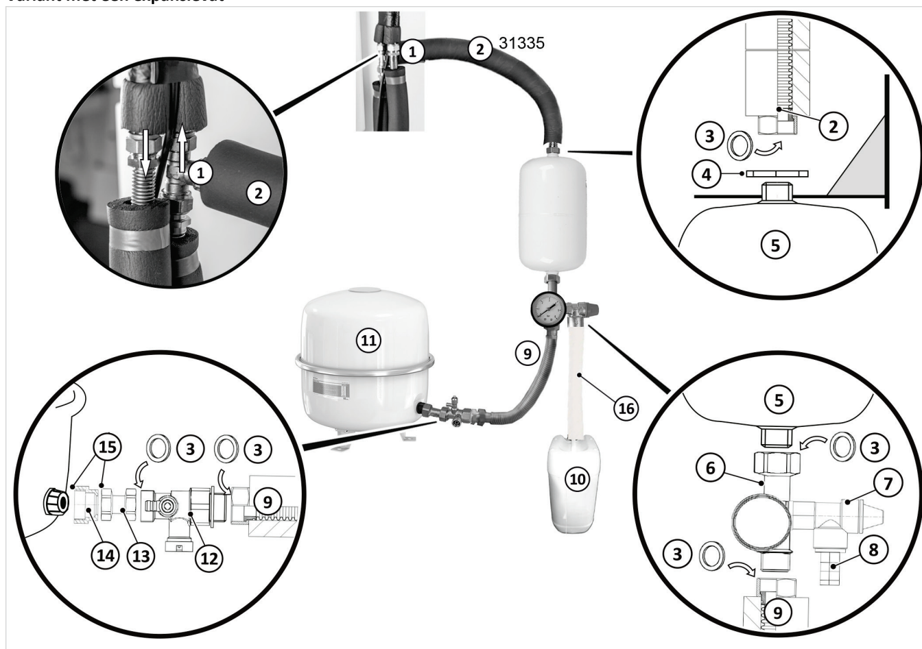
Afb. 87: Koppeling Solar-MAG
