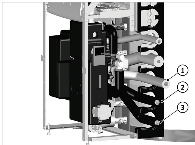
Afb. 75: Hydraulische aansluiting SolvisLea
