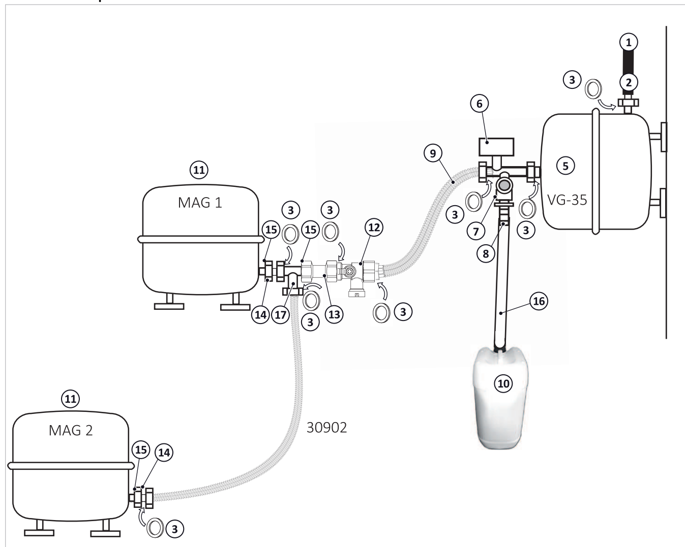
Afb. 88: Koppeling van twee Solar-MAG
