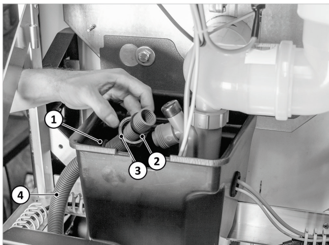
Afb. 40: Condensslang door de opening geleiden en aansluiten
