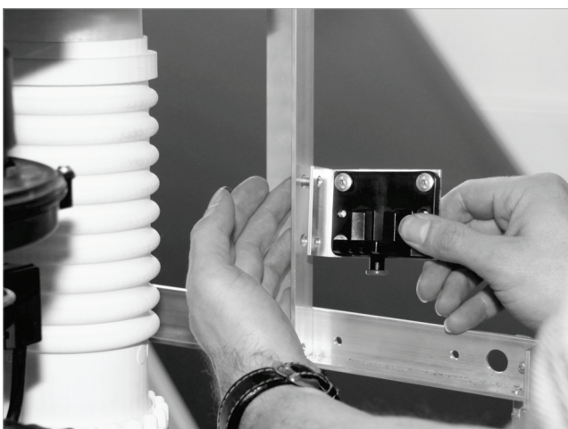
Afb. 64: Oliefilterhouder bevestigen
