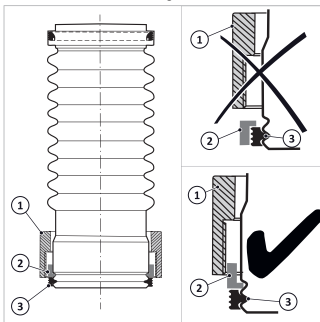
Afb. 58: Schroefkoppeling opgestoken
