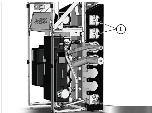
Afb. 67: De olieleiding door de derde reductie leiden.
