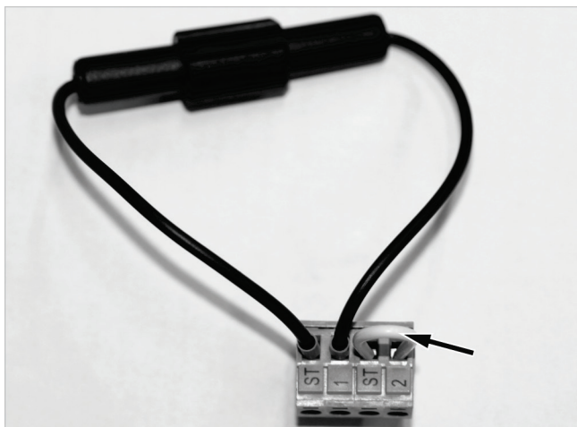
Afb. 42: Busstekker met zekering (zwart) voor brander SX-LN-3 (aansluiting ASTB zie pijl)
