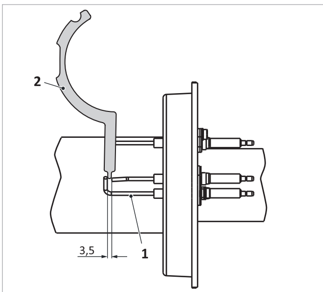
Afb. 111: Afstand elektrode naar de massa op de ontstekingselektrode
