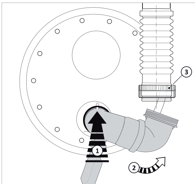
Afb. 62: De rookgasbocht monteren
