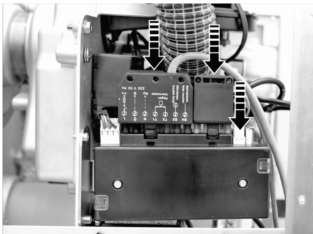
Afb. 71: Stekker opsteken
