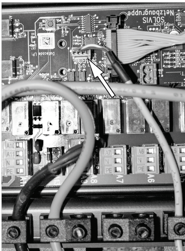
Afb. 48: De busstekker aansluiten.
