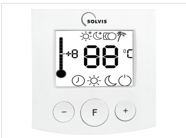
Afb. 91: Ruimtebedieningselement BE-SC-2
