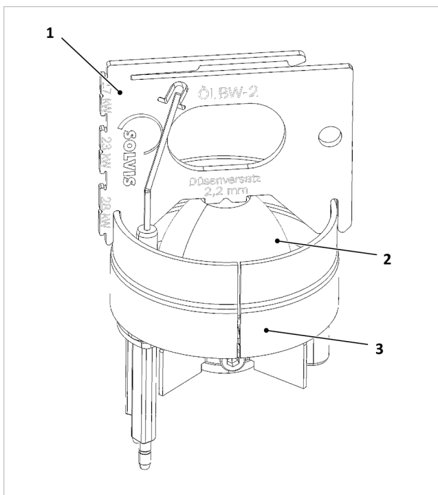
Afb. 117: Mengkop met aangebracht kaliber
