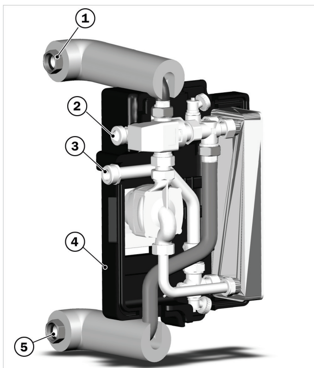
Afb. 77: WWS-24 - Aansluitingen
