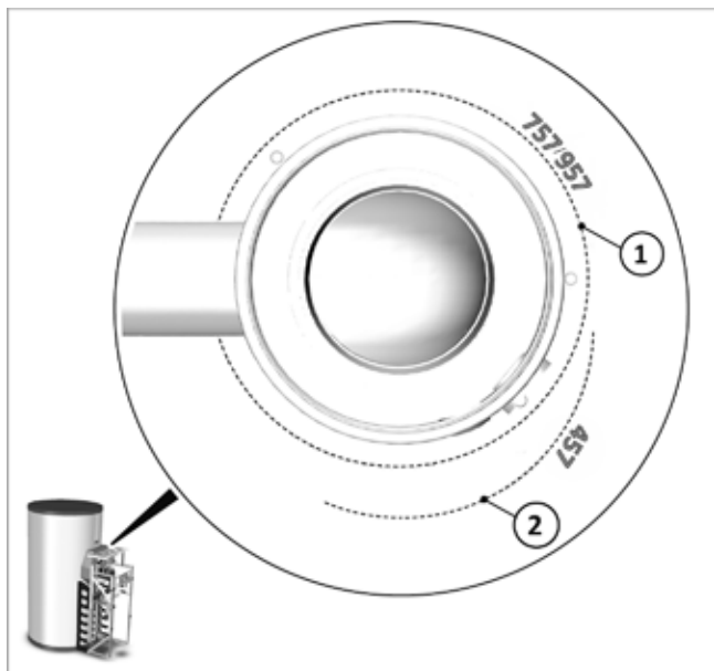
Afb.57: Positie Rookgasafvoeraansluitstuk
