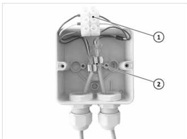
Afb. 94: Modbus-verbindingsdoos bevestigen
