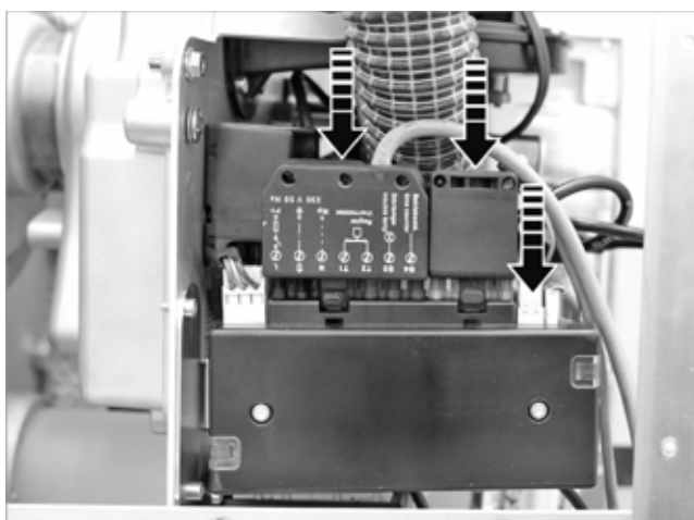
Afb. 71: Stekker opsteken
