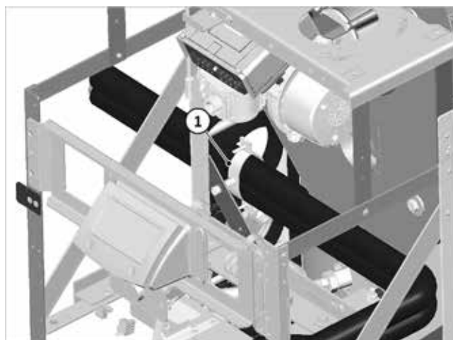
Afb. 86: Buizen bevestigen
