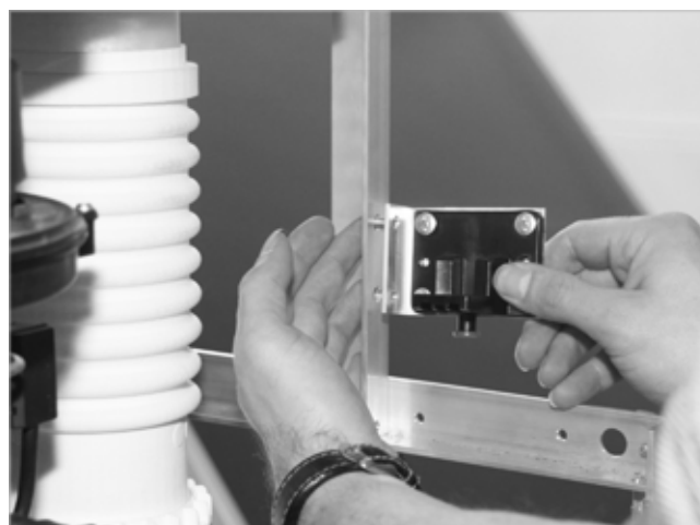
Afb. 64: Oliefilterhouder bevestigen
