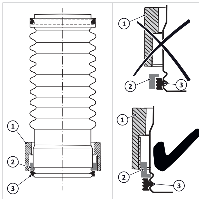
Afb. 37: Schroefkoppeling opgestoken
