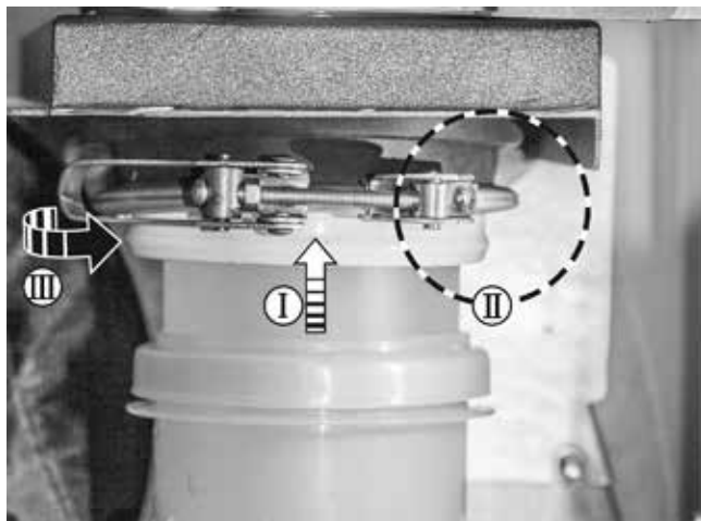
Afb. 36: Klem monteren
