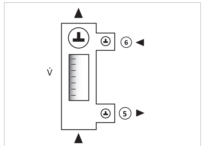
Afb. 104: Flowmeter V in spoelstand 2
