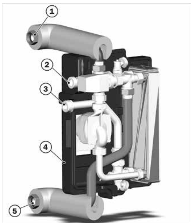
Afb. 77: WWS-24 - Aansluitingen
