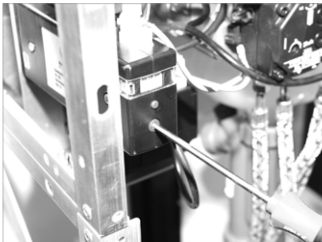
Afb. 100: Op de gewenste trap instellen
