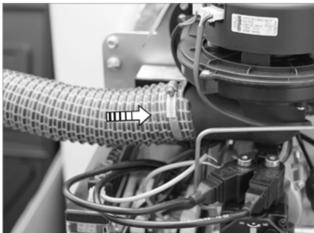
Afb. 56: Aanzuigluslang op de ventilator aansluiten
