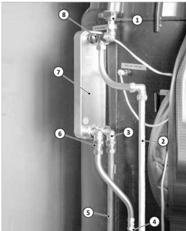
Abb. 3: Umbausatz montiert
