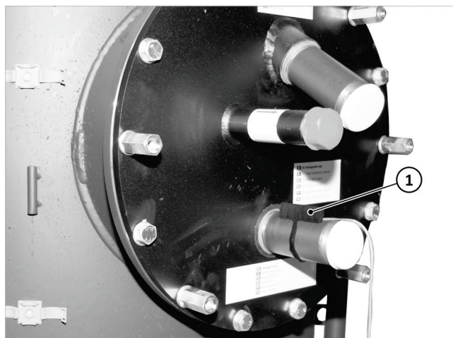
Abb. 4: Sensor S4 (1) montiert
