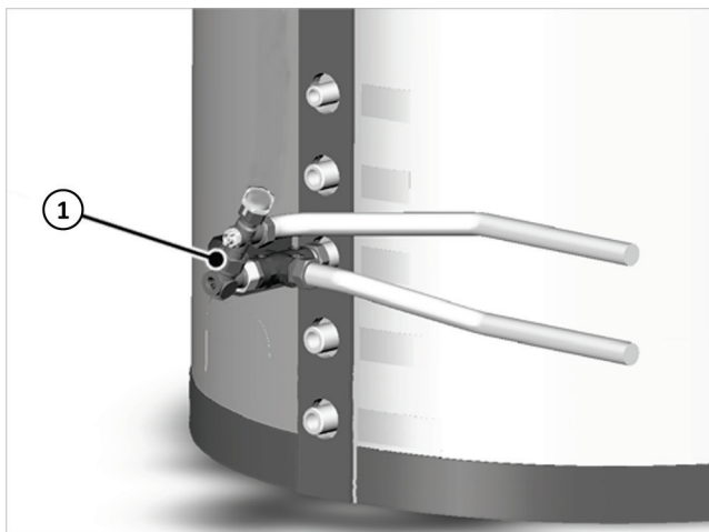
Abb. 7: Umschaltventil montiert
