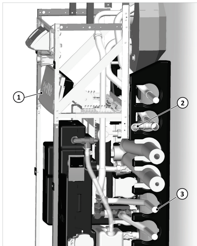
Fig.14: collegamento idraulico del circuito di riscaldamento
