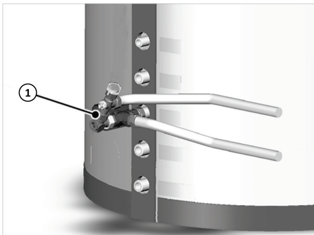
Fig. 7: Montaggio della valvola di commutazione
