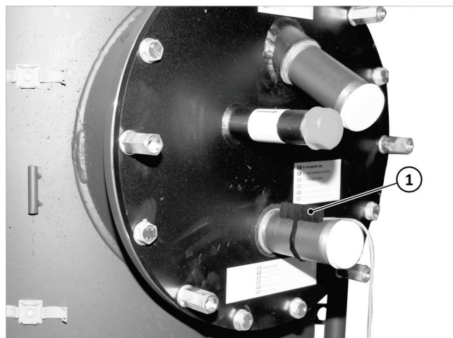
Fig. 4: Sensore S4 (1) montato
