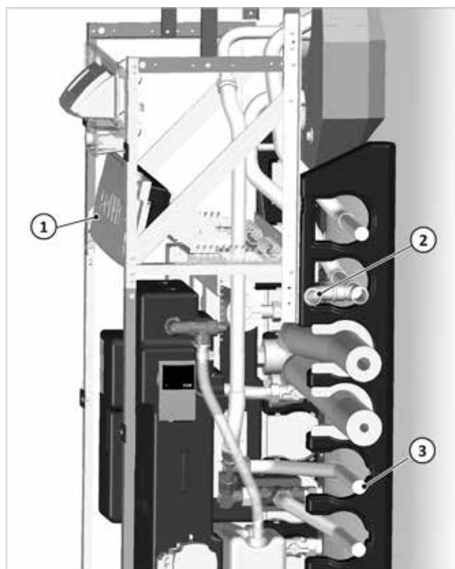
Fig.14: Integración hidráulica de circuitos de calefacción
