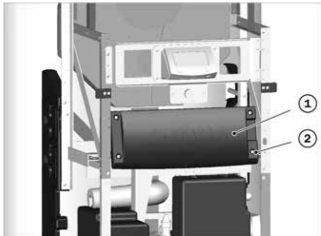
Fig. 27: Fijar la tapa del módulo de red
