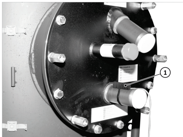
Afb. 4: Sensor S4 (1) gemonteerd
