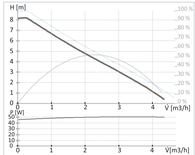
Fig. 22: Curva caratteristica pompa IMP NMT Mini PWM 15/80-130 (velocità costante)
