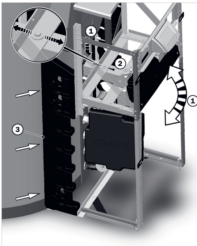
Afb.11: Laadmodule uitlijnen
