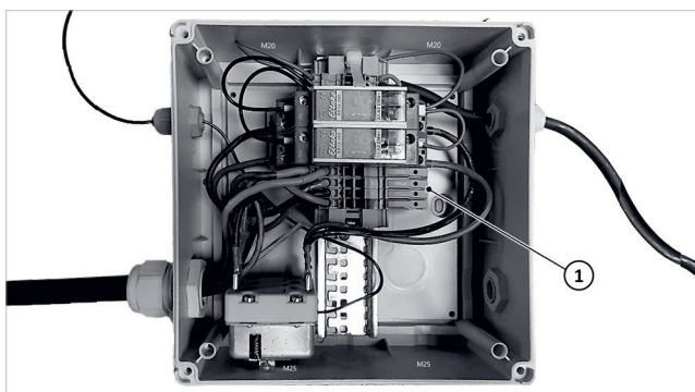
Afb. 18: Aansluitbox
