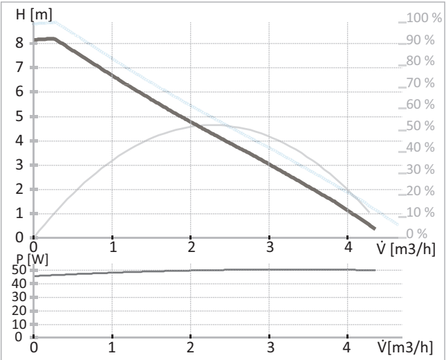
Afb. 22: Pompkarakteristiek IMP NMT Mini PWM 15/80-130 (constant toerental)
