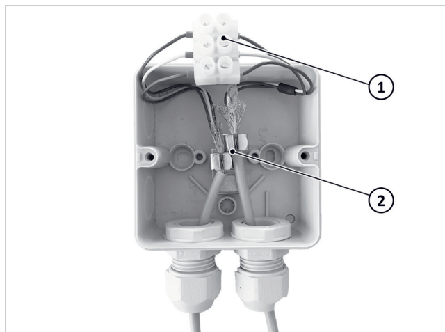
Afb. 16: Modbus-verbindingsdoos bevestigen
