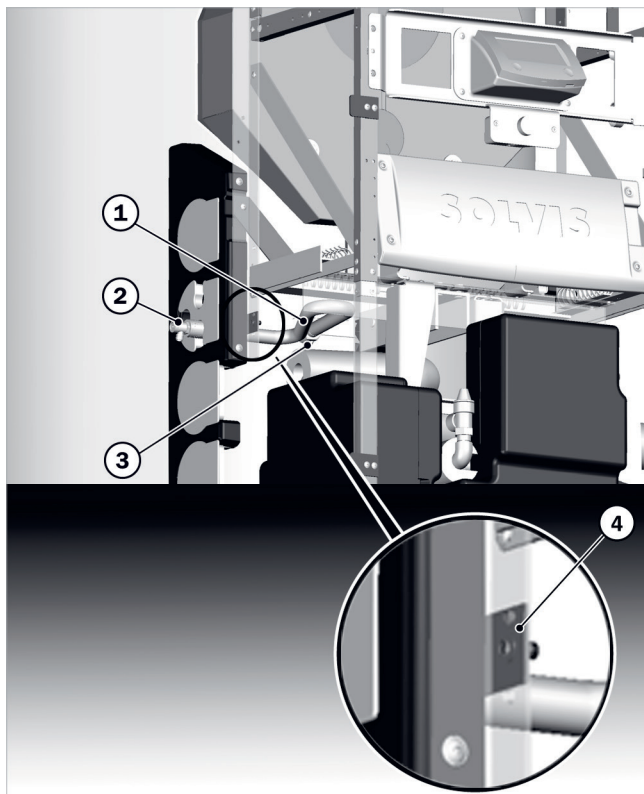
Afb.14: Aansluiting ontlufter van flexibele geribde buis voorzien
