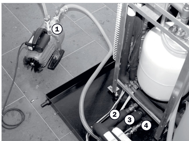
Afb. 1: Pomp aansluiten
