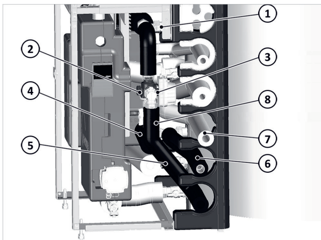
bb.6: Omschakelklep monteren (WP-aanvoer naar rechts)
