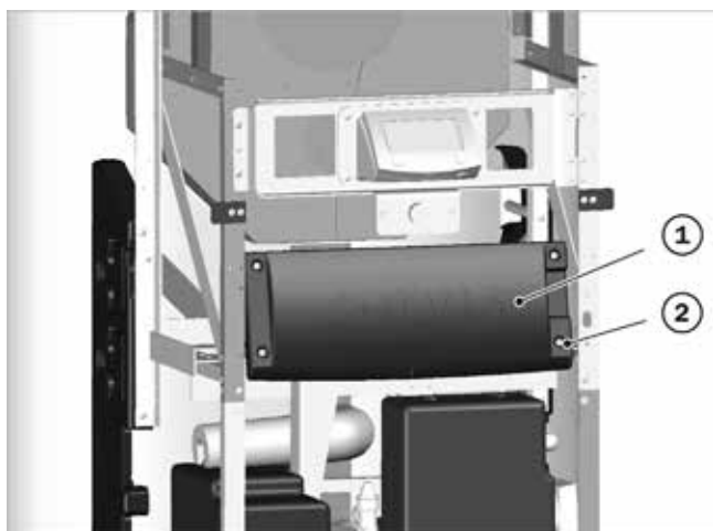
Afb. 19: Deksel van de netwerkkaart bevestigen
