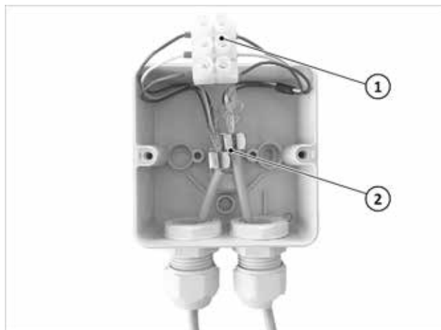
Afb. 16: Modbus-verbindingsdoos bevestigen
