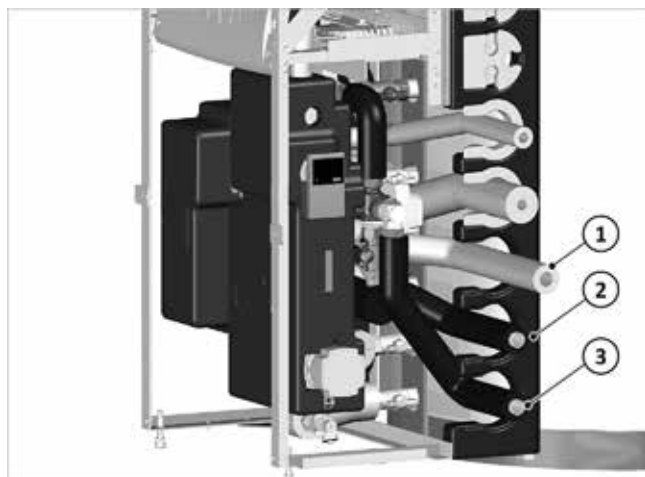
Afb. 15: hydraulische aansluiting warmtepomp
