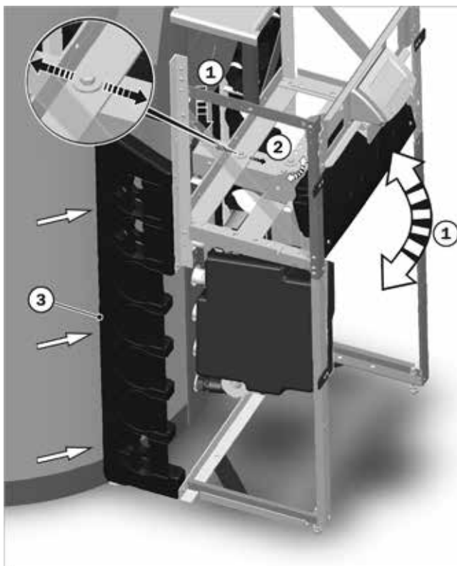
Afb.11: Laadmodule uitlijnen
