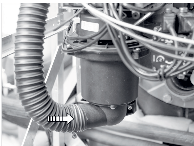
Fig. 59: Fissaggio del tubo flessibile per l'aria di alimentazione nel soffiante
