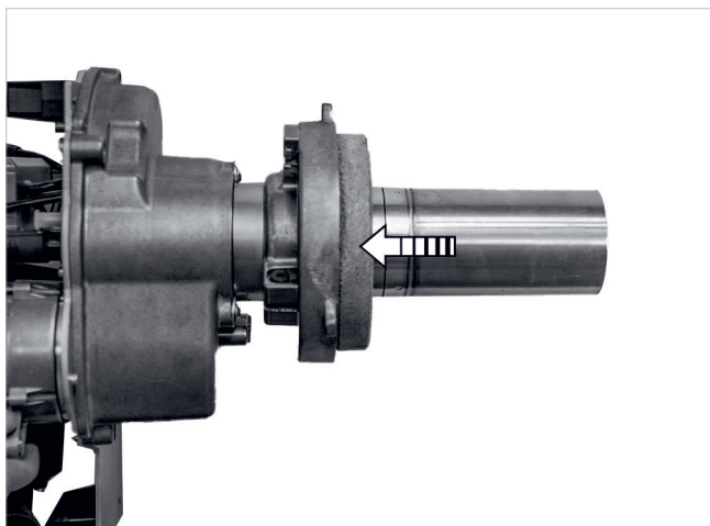
Fig. 56: applicazione del portello caldaia con isolante refrattario
