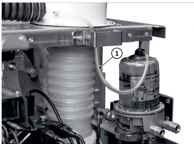
Fig. 71: tubo flessibile di sfiato montato
