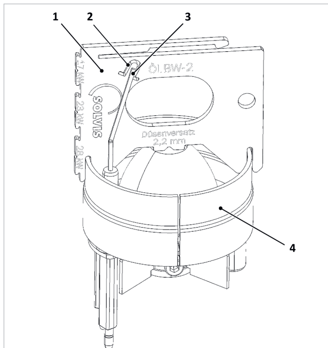
Fig. 54: Controllo della posizione degli elettrodi di accensione
