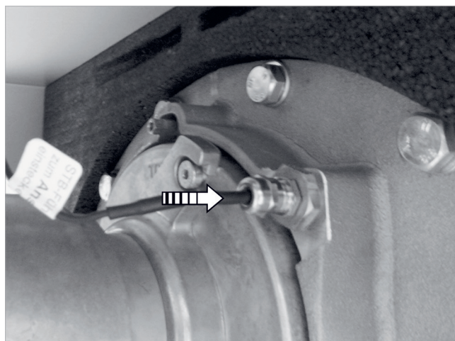
Fig. 72: inserire e avvitare eSTB
