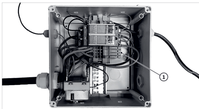
Fig. 98: Scatola di connessione
