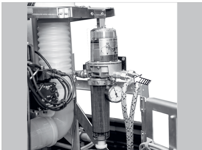
Fig. 69: allacciamento della tubazione dell'olio
