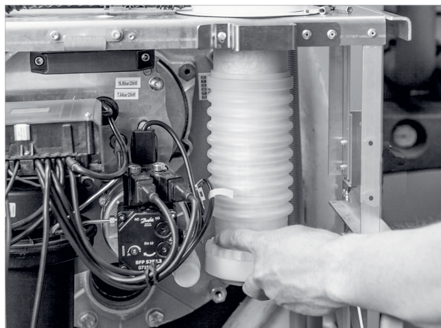
Fig. 64: Orientamento perpendicolarmente verso il basso del raccordo per lo scarico dei fumi
