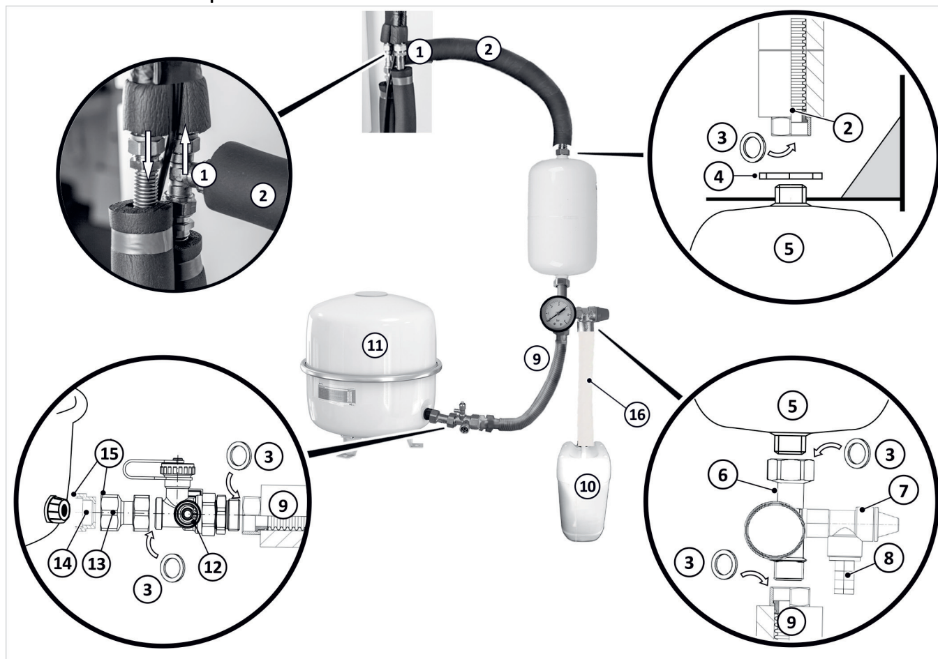
Fig. 90: Collegamento Solar-MAG
