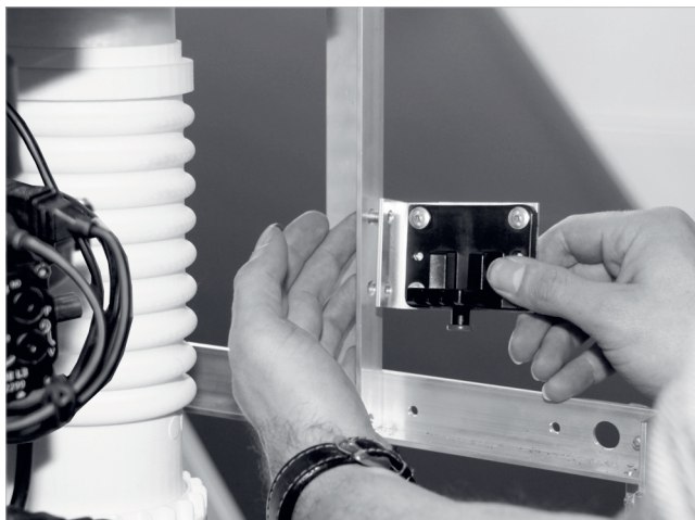
Fig. 67: Fissaggio del supporto del filtro dell'olio
