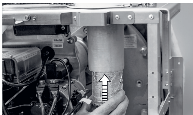
Fig. 62: Montaggio fonoassorbente per la parte interna del tubo
