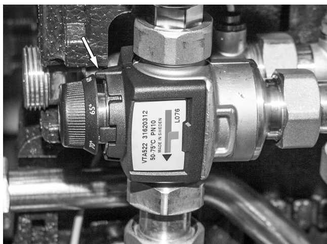
Fig. 102: Impostazione TMV
