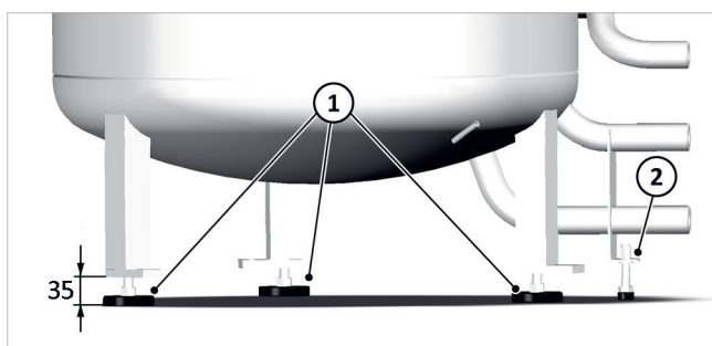
Fig.2: installazione dell'accumulatore
