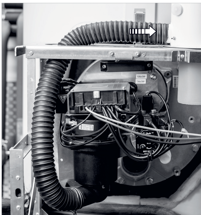
Fig. 60: Montaggio del tubo flessibile per l'aria di alimentazione
