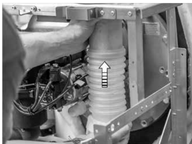
Fig. 63: Montaggio raccordo per lo scarico dei fumi
