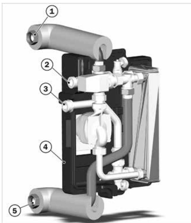
Fig.80: WWS-24 - collegamenti
