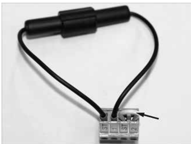
Fig. 46: Connettore femmina con fusibile (nero) per bruciatore SX-LN-3 (per il collegamento ASTB vedere freccia)
