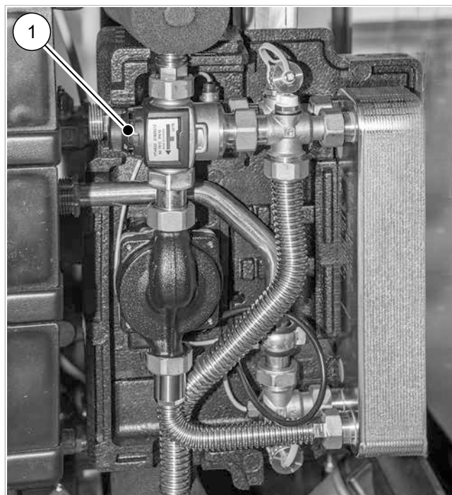
Fig. 101: Valvola di miscelazione termica (1) in WWS-30, SolvisMax
