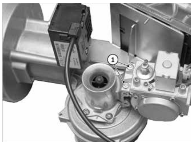
Fig. 25: smontaggio della valvola combinata del gas
