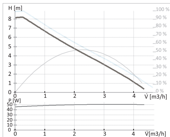
Fig. 133: Curva caratteristica pompa IMP NMT Mini PWM 15/80-130 (velocità costante)
