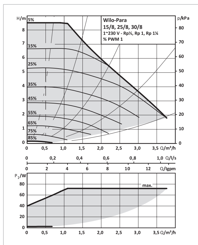
Fig. 132: Curva caratteristica della pompa Wilo-PARA 15/8
