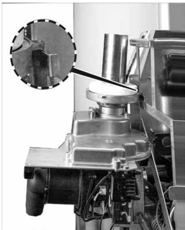
Fig. 117: bruciatore in posizione di parcheggio
