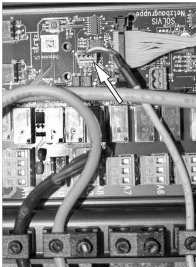
Fig. 52: Collegamento spina del bus
