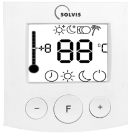
Fig. 94: elemento di regolazione ambiente BE-SC-2
