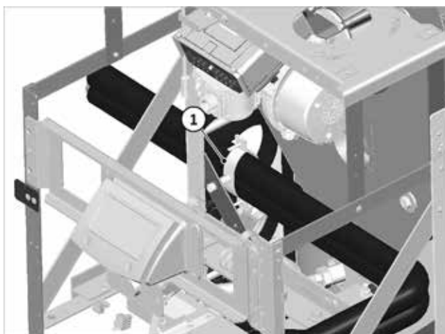
Fig. 89: fissaggio dei tubi
