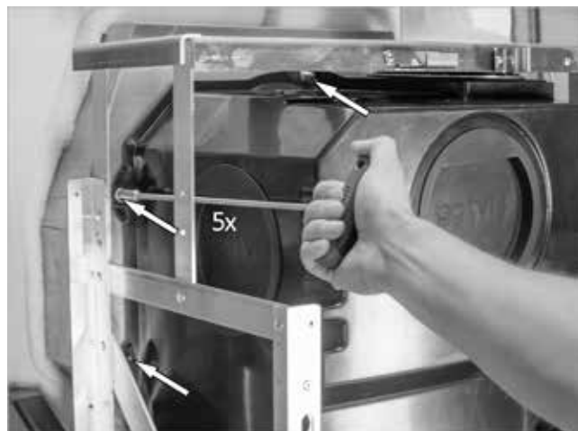
Fig. 49: Serraggio della copertura della camera di aspirazione
