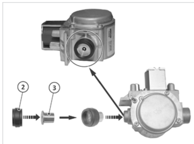
Fig. 26: montaggio dell'ugello per gas liquido
