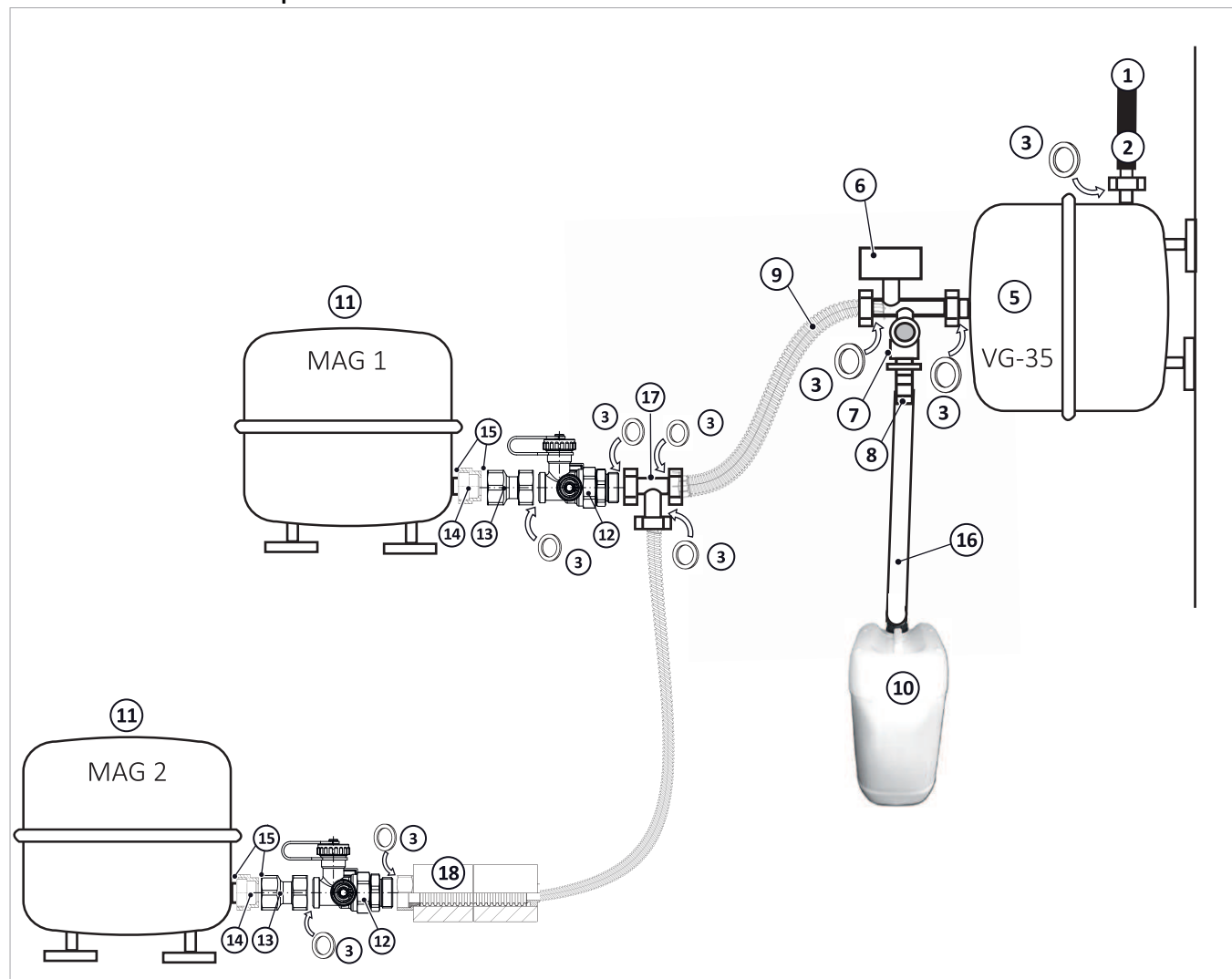
Fig. 91: Collegamento di due Solar-MAG per mezzo del vaso di espansione del set di estensione (EW-AG)
