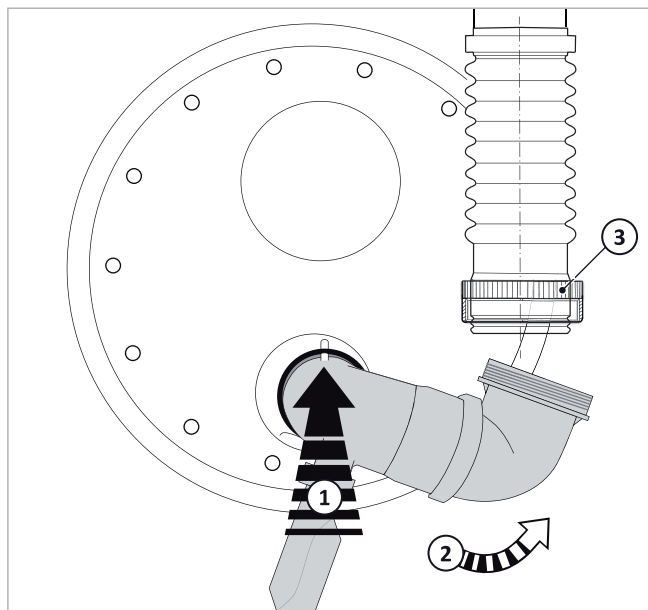
Fig. 65: montare la curva della tubazione fumi
