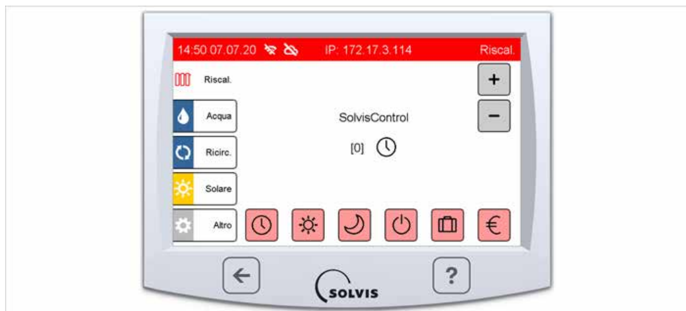
Fig. 130: SolvisControl con menu "Riscaldamento"
