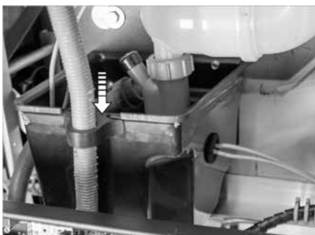
Fig. 48: Fissaggio della tubazione del gas alla vasca per mezzo delle clip di fissaggio
