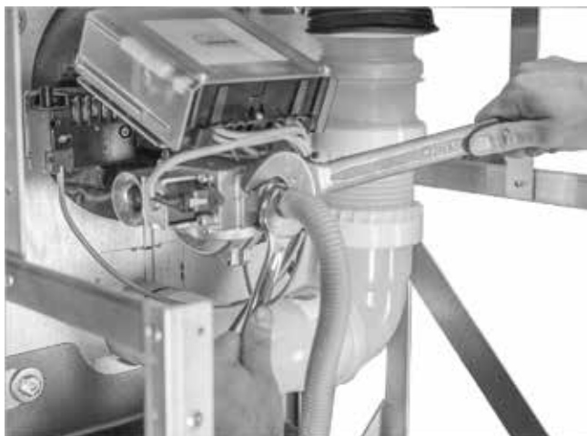
Fig. 47: collegamento della condotta del gas
