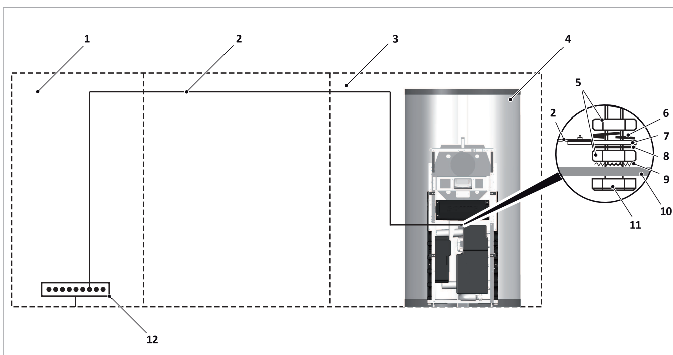
Fig. 92: compensazione di potenziale di SolvisMax
