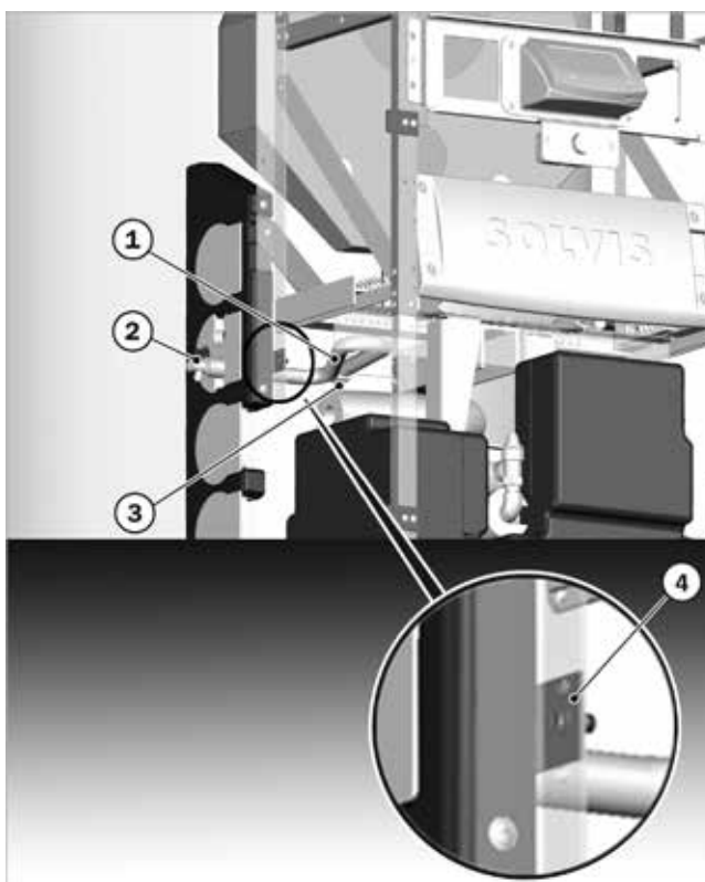
Fig.24: collegamento per lo sfiato con tubo ondulato applicato
