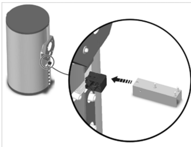
Fig.9: supporto dell'avancorpo
