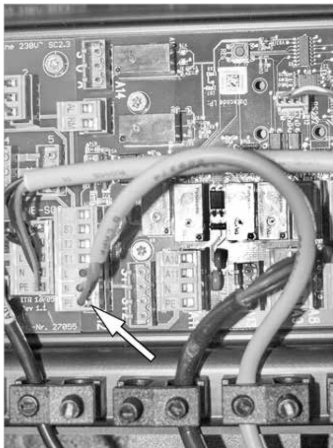
Fig. 51: Collegamento della spina del bruciatore a gas a A 12
