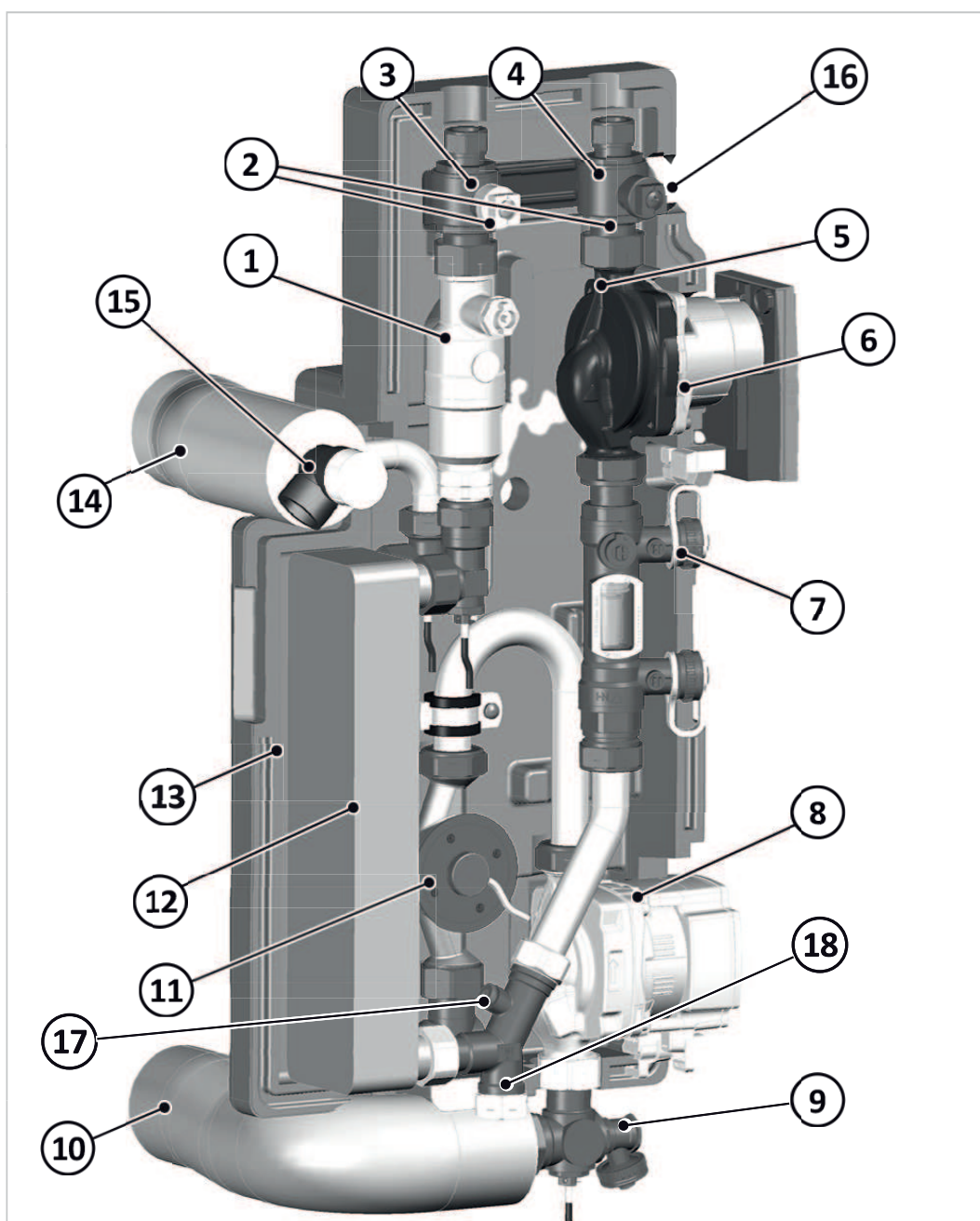
Fig.84: panoramica dei componenti della stazione di trasmissione del calore solare
