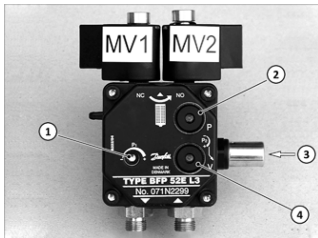
Fig. 104: Impostazione della pressione pompa nella pompa del gasolio
