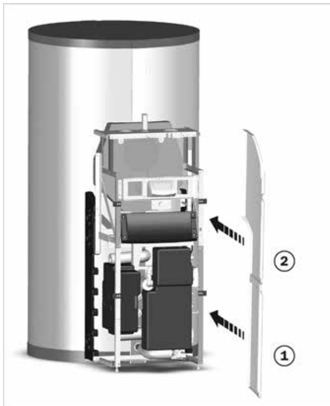
Fig. 110: infilare l'elemento laterale inferiore (1) per primo
