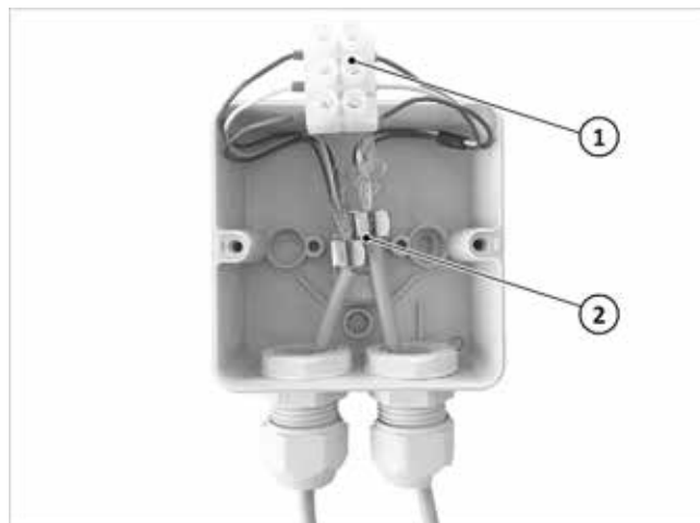
Fig. 97: fissaggio scatola di distribuzione Modbus
