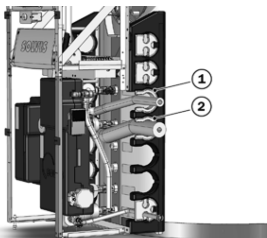
Fig. 83: Stazione acqua calda, passaggio tubi per l'acqua potabile (a destra)
