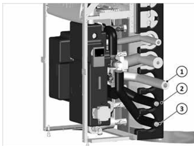
Fig. 78: Collegamento idraulico pompa di calore
