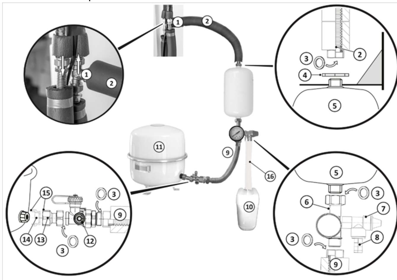
Fig. 90: Collegamento Solar-MAG
