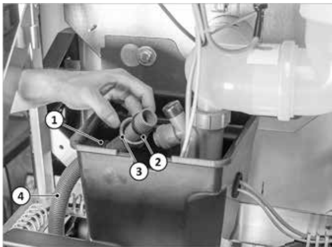
Fig. 44: Inserimento e fissaggio del tubo flessibile della condensa attraverso l'apertura
