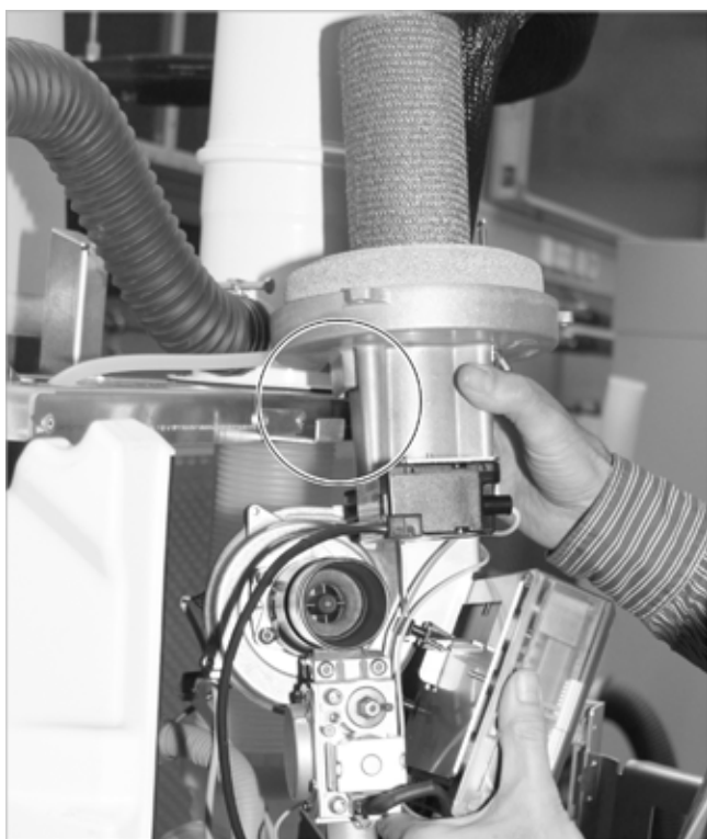
Fig. 112: bruciatore in posizione di manutenzione sulla console
