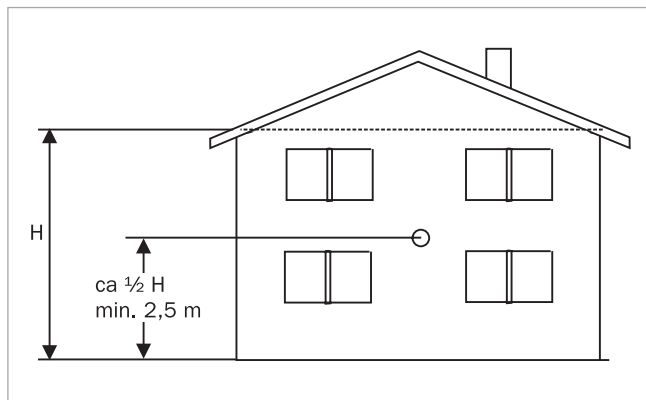
Fig. 93: Posizione del sensore esterno
