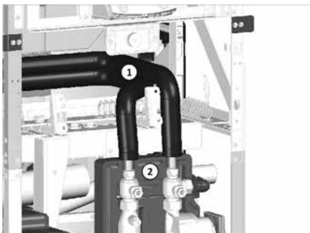
Fig. 87: guidare il set di tubi verso la parte posteriore
