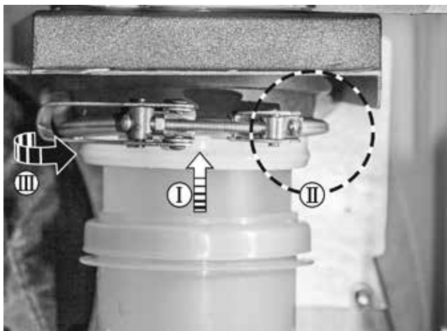
Fig. 40: Montaggio della fascetta
