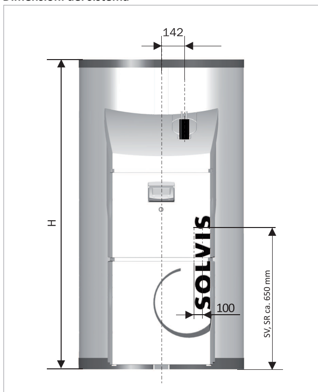
Fig. 126: Vista frontale
