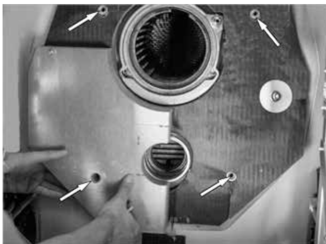
Fig. 29: Montaggio dell'isolamento anteriore della flangia
