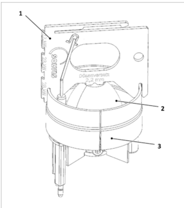
Fig. 122: Testa del miscelatore con calibro applicato
