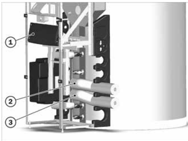
Fig. 79: collegamento idraulico del circuito di riscaldamento
