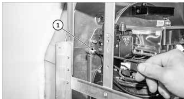
Fig. 118: Viti a serraggio rapido nell'inserto del bruciatore
