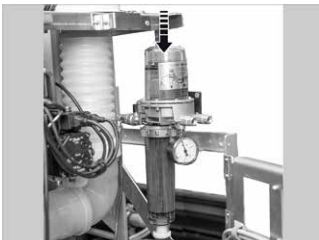
Fig. 68: inserimento del filtro dell'olio
