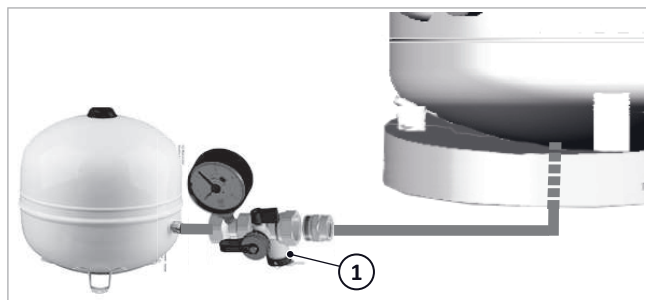
Fig. 100: Valvola KFE al gruppo di collegamento MAG
