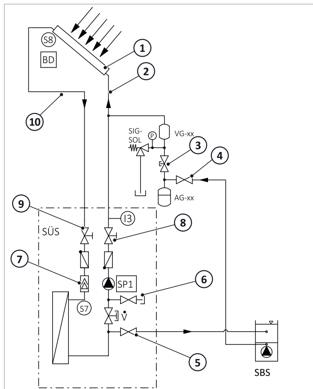
Fig. 106: Stazione di trasmissione del calore solare: Lavaggio dello scambiatore di calore
