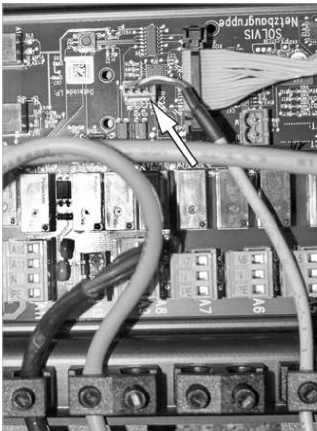
Fig. 74: Collegamento spina del bus
