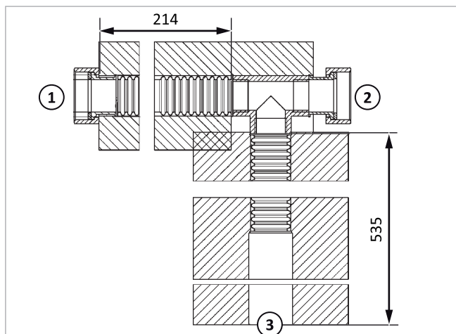
Fig. 86: Tubo di collegamento caldaia a combustibile solido (RO-FBK-RL)
