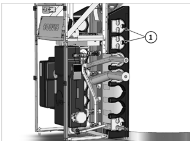
Fig. 70: passaggio della tubazione dell'olio attraverso la riduzione da tre
