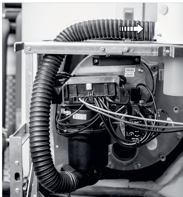
Fig. 60: Montaje del tubo de entrada de aire
