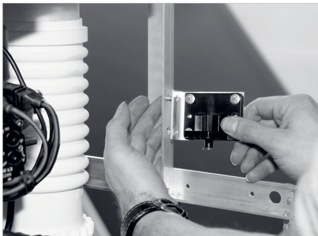
Fig. 67: Fijación del soporte del filtro de gasóleo
