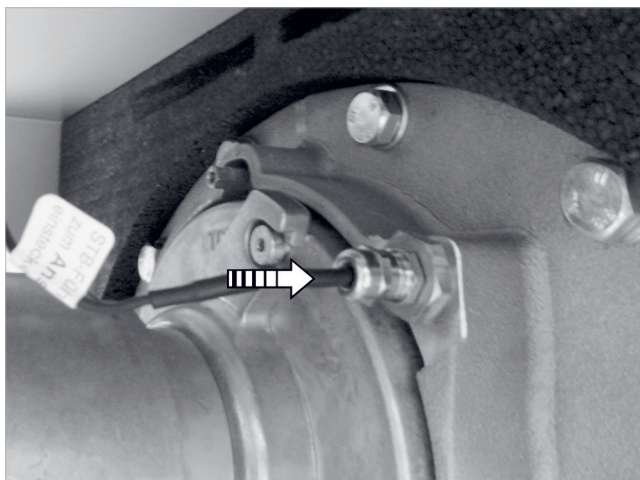
Fig. 72: Inserción y atornillado del eSTB
