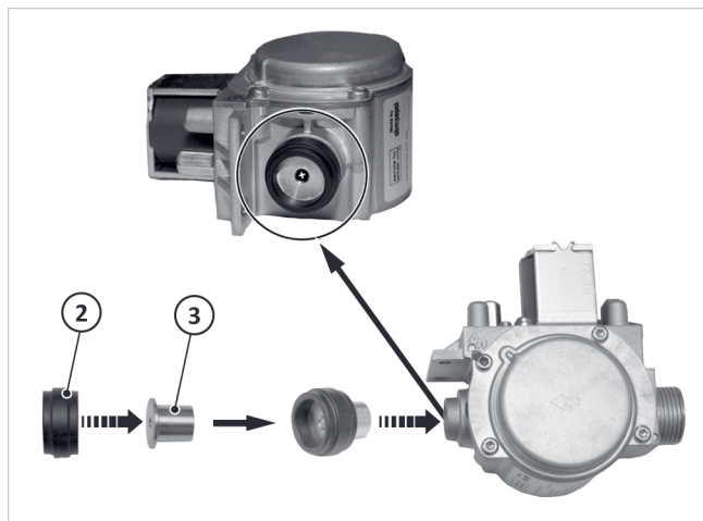
Fig. 26: Montar la tobera de gas líquido
