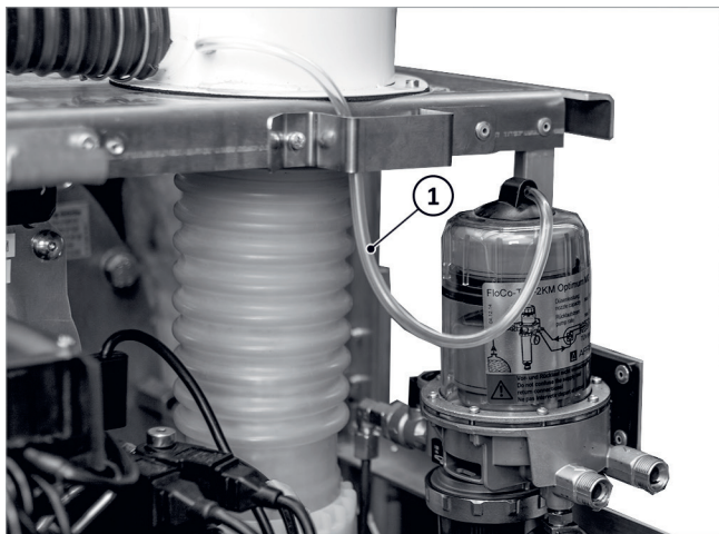
Fig. 71: Manguera de purga de aire montada
