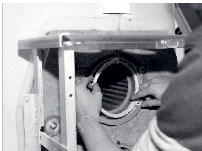
Fig. 53: Colocar el cordón de cierre hermético, extremo arriba
