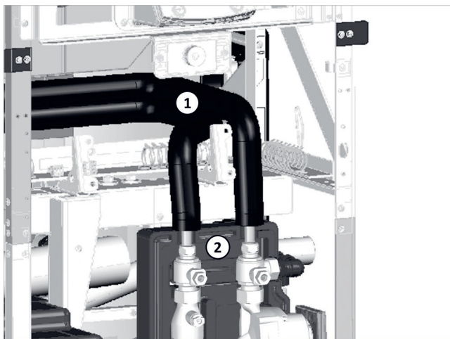
Fig. 87: Guiar los tubos hacia atrás
