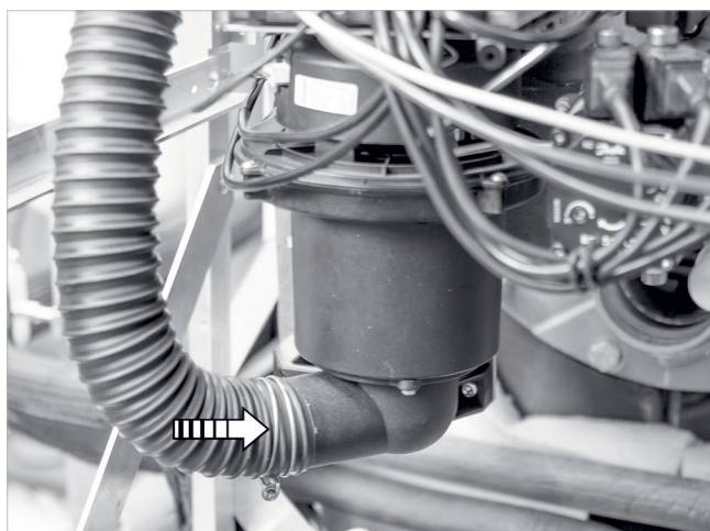
Fig. 59: Fijar el tubo de entrada de aire al ventilador
