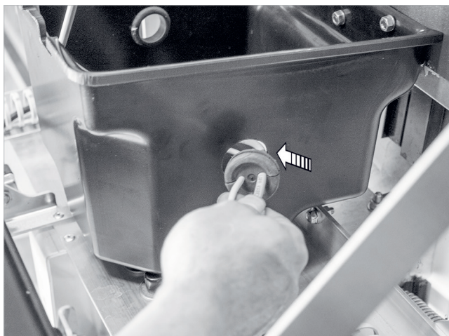
Fig. 36: Insertar herméticamente el paso de cables
