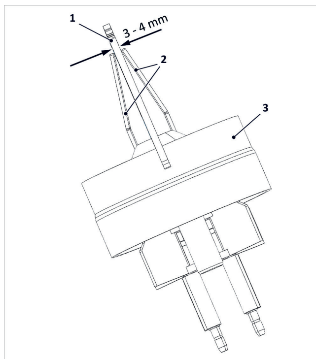
Fig. 124: Comprobar la distancia de los electrodos de encendido
