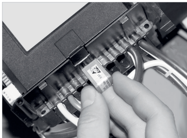
Fig. 28: Montar la tarjeta de chip del quemador
