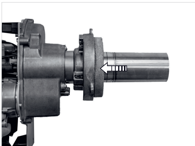
Fig. 56: Colocación del ladrillo de la puerta de la caldera
