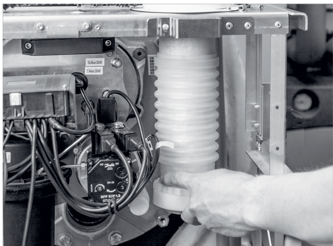
Fig. 64: Alineación recta de la pieza de tubo de conexión de salida de humos
