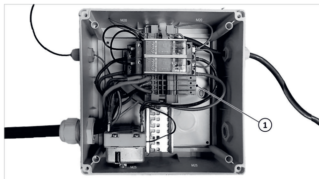
Fig. 98: Caja de conexión
