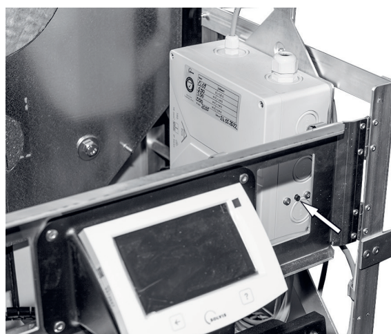
Fig. 125: Botón de desbloqueo caja de conexión HPT
