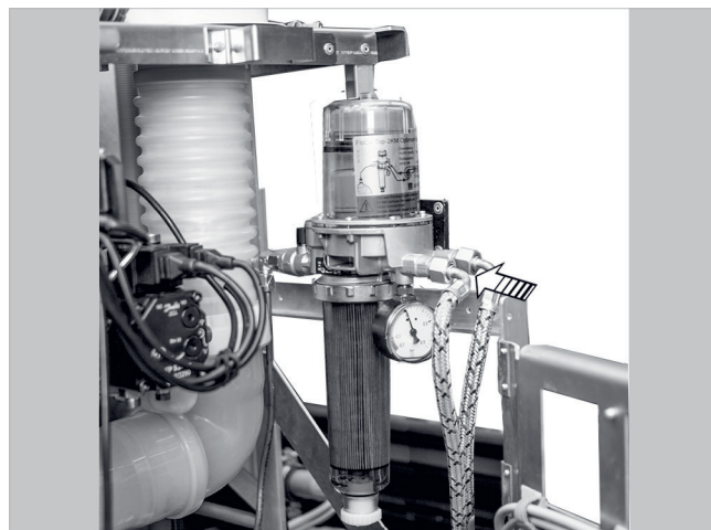
Fig. 69: Conexión de las tuberías de gasóleo
