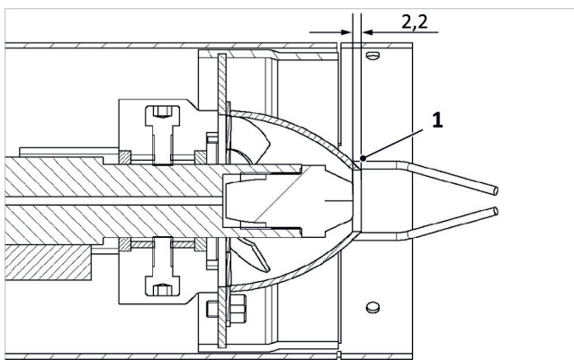
Fig. 121: Sección transversal del cabezal de mezcla
