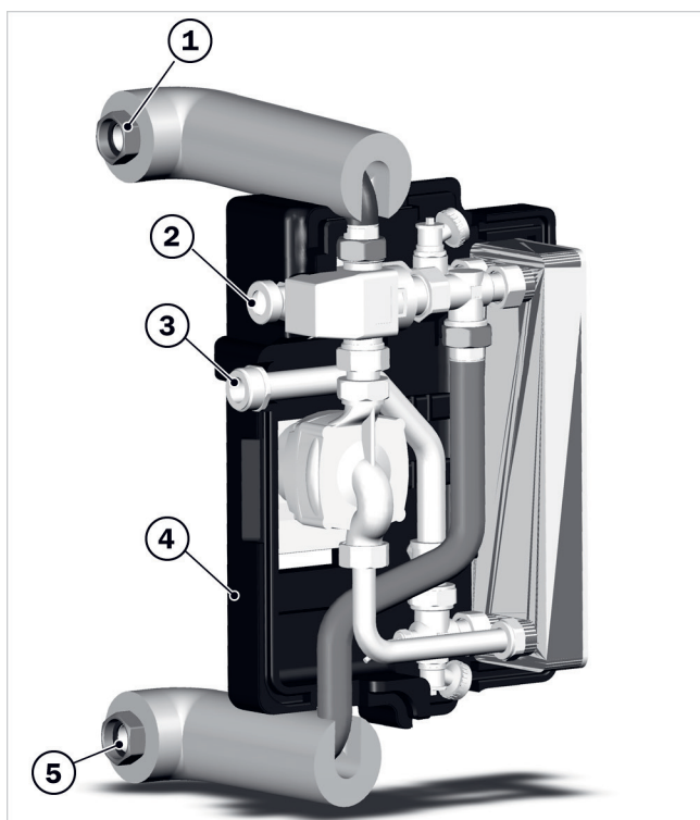
Afb.80: WWS-24 - Aansluitingen
