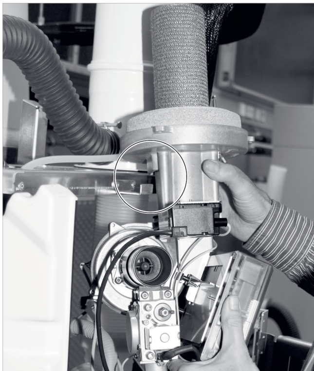
Afb. 112: Brander in onderhoudspositie aan de console
