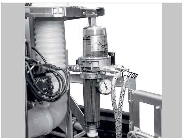
Afb. 69: Olieleidingen aansluiten
