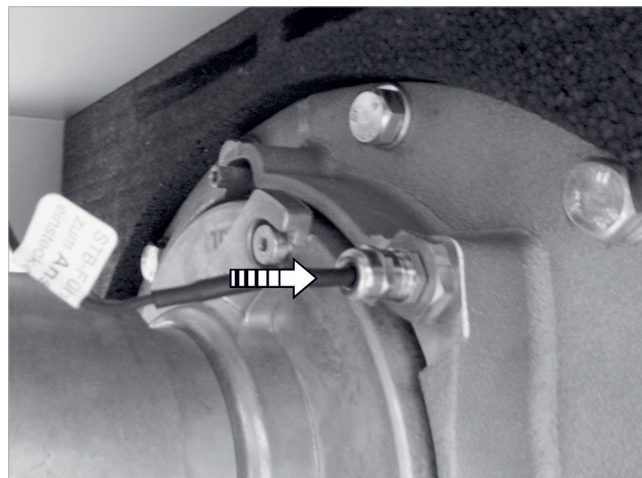
Afb. 72: eSTB insteken en vastschroeven
