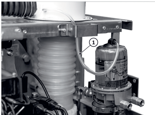
Afb. 71: Ontluchtingsslang gemonteerd
