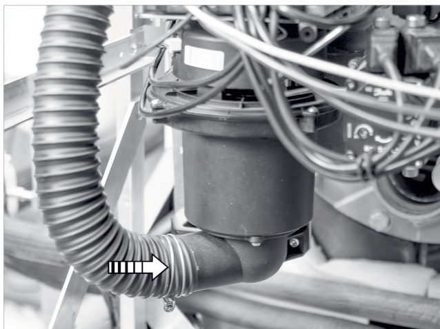
Afb. 59: Toevoerluchtslang op de ventilator aansluiten
