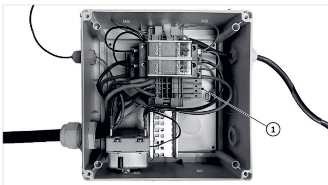
Afb. 98: Aansluitbox
