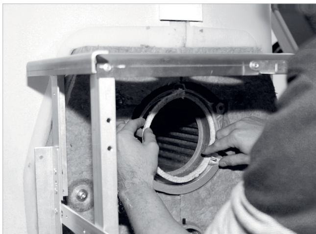
Afb. 53: Branderpakingsnoer plaatsen, kopse kanten boven
