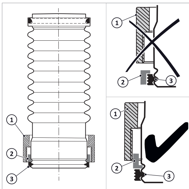
Afb. 61: Schroefkoppeling opgestoken
