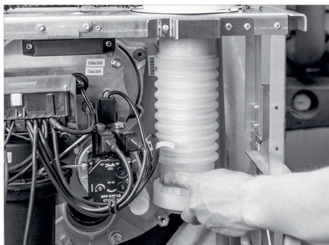
Afb. 64: Rookgasaansluitleidingstuk recht uitlijnen
