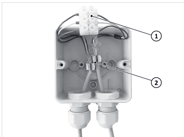
Afb. 97: Modbus-verbindingsdoos bevestigen
