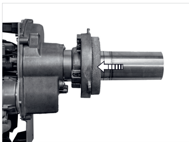
Afb. 56: Keteldeurisolatie plaatsen
