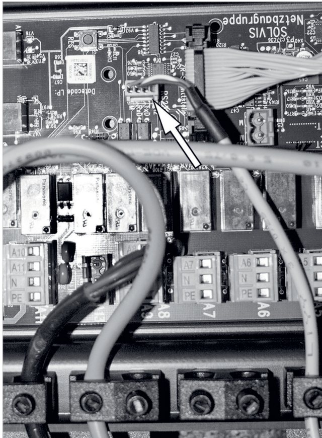
Afb. 74: De busstekker aansluiten.
