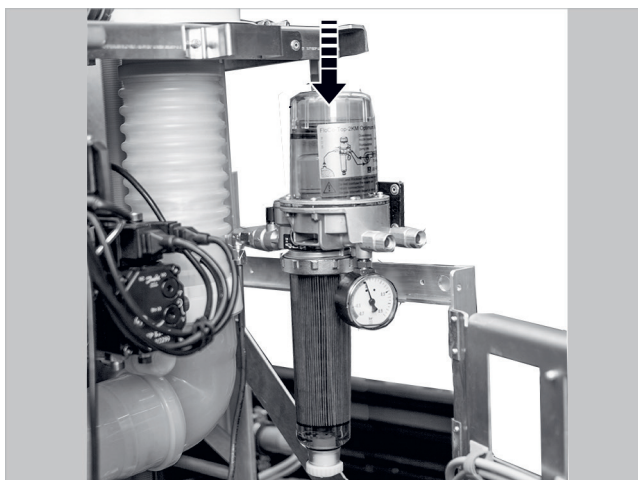
Afb. 68: Oliefilter opsteken
