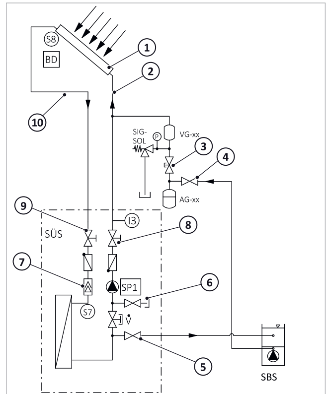
Afb. 106: Zonniewarmte-overdrachtsgroep: Spoelen van de warmtewisselaar
