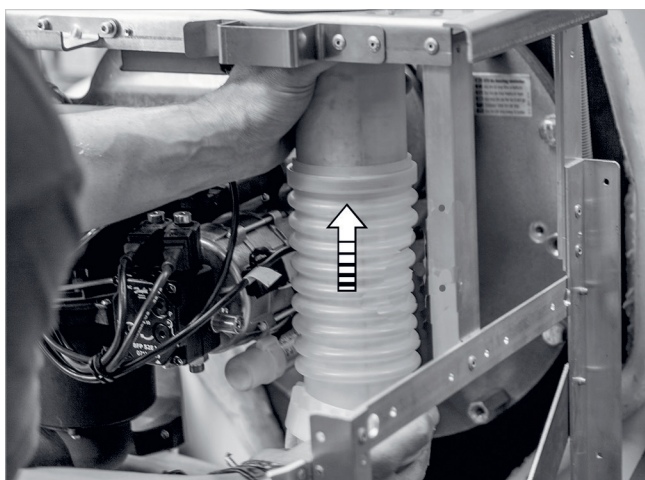
Afb. 63: Rookgasaansluitleidingstuk opsteken
