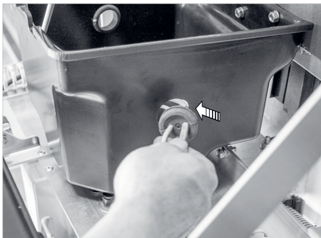
Afb. 36: Branderkabel luchtdicht doorvoeren
