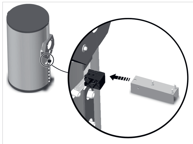
Afb.9: Opbouwhouder voorzijde
