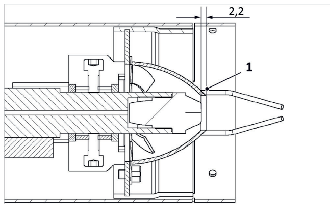
Afb. 121: Dwarsdoorsnede van mengkop
