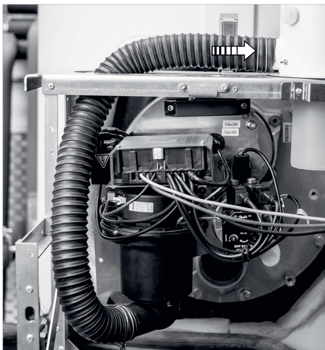
Afb. 60: Toevoerluchtslang monteren
