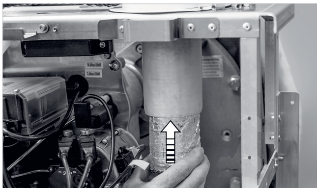
Afb. 62: Inwendige geluiddemper plaatsen
