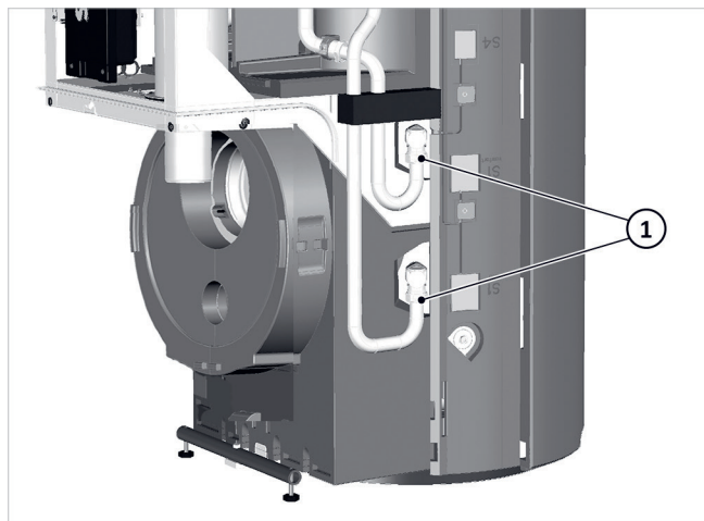
Fig. 31: Controllare/serrare gli attacchi della SCR
