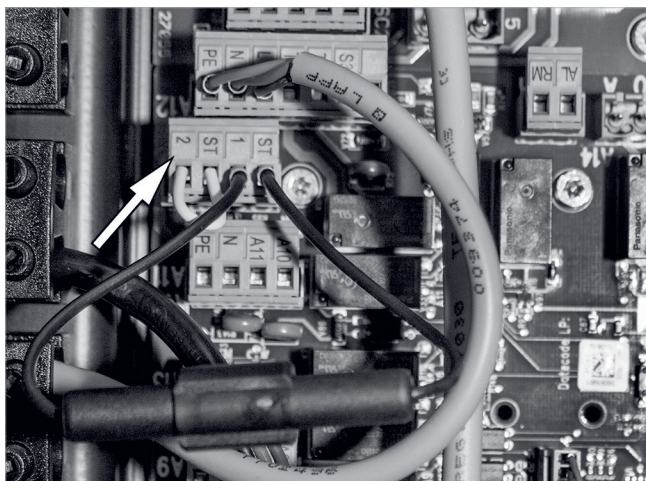
Fig. 57: Inserir la presa di collegamento
