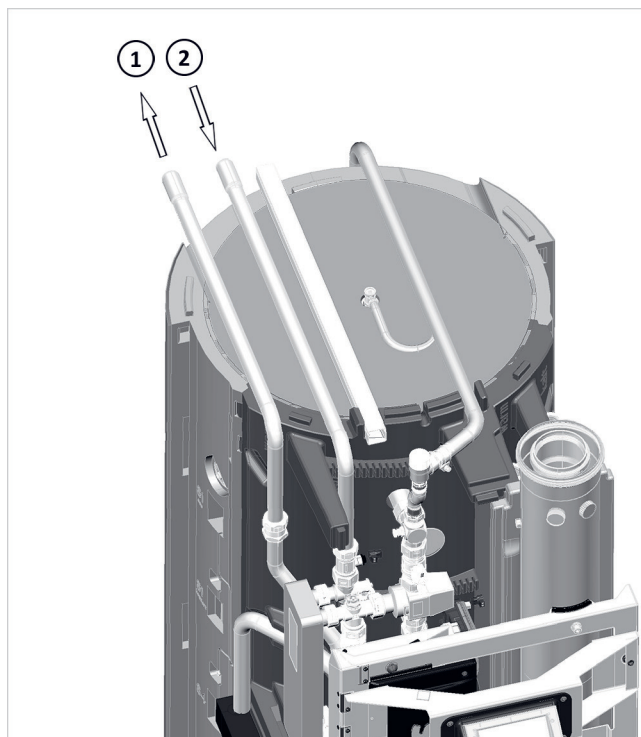
Fig. 29: Attacco posteriore TWW/TWW
