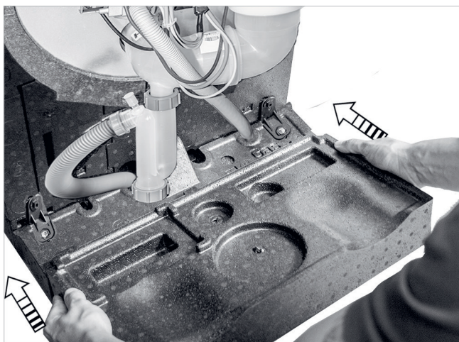
Fig. 93: Innestare la parte anteriore della base
