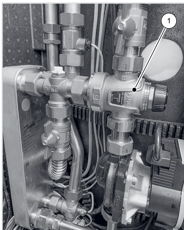
Fig. 111: Valvola di miscelazione termica (1) SolvisBen in WWS
