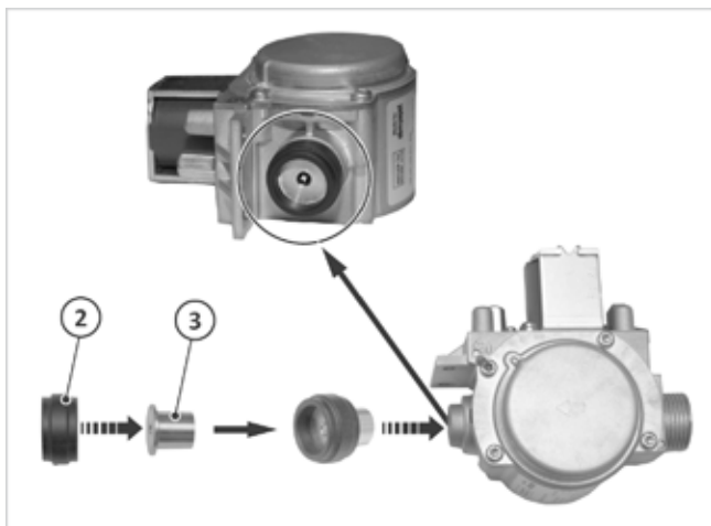
Fig. 42: Montar la tobera de gas líquido
