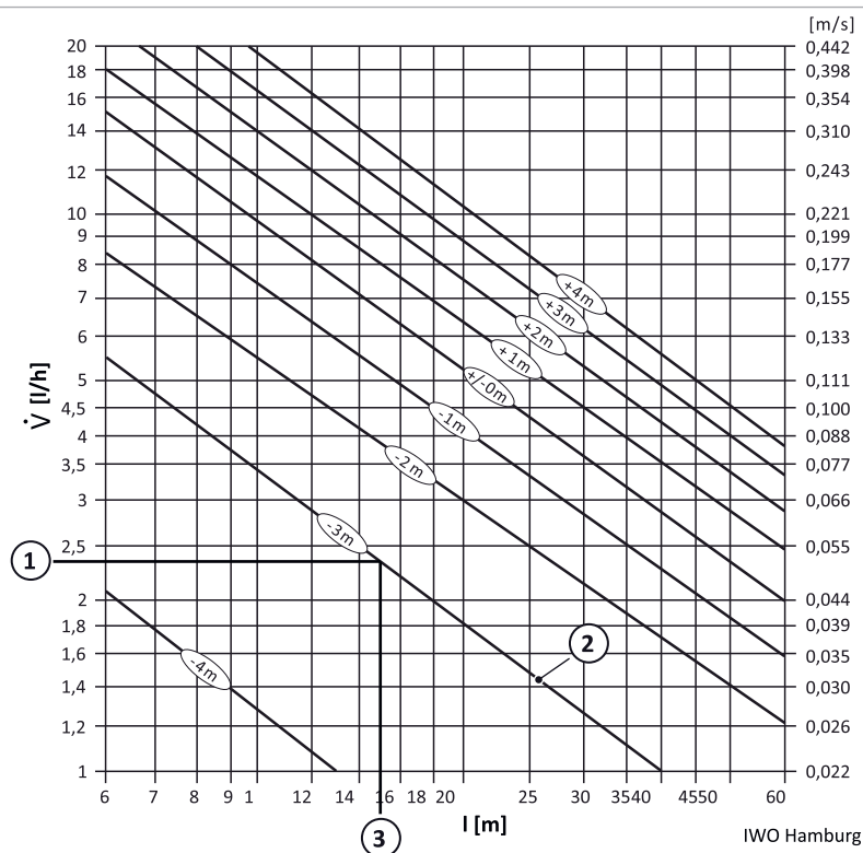
Fig. 82: Longitud máxima de tuberías del sistema de un ramal en función de la altura de bombeo
