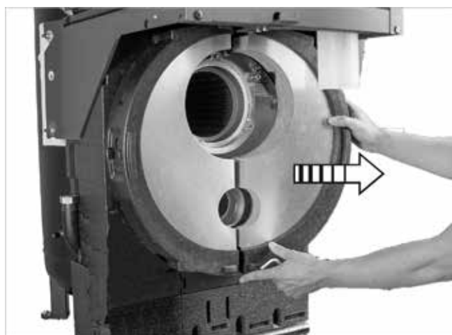
Fig. 6: Desmontaje del aislamiento delantero de la brida
