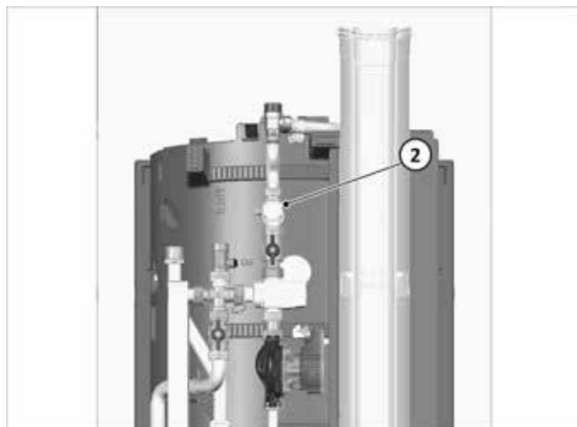
Fig. 27: Control/reapriete de la unión roscada del avance
