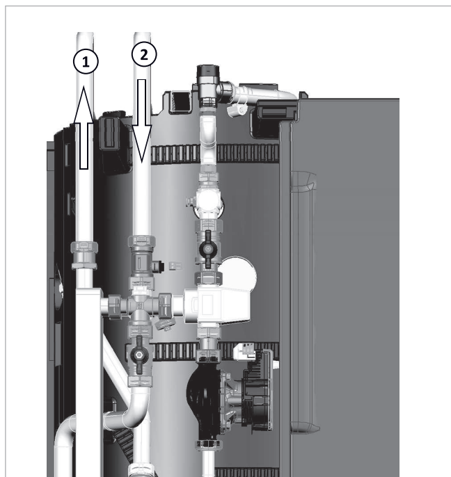
Fig. 28: Conexión de agua potable caliente/fría desde arriba
