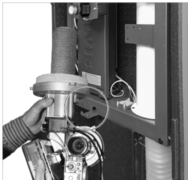
Fig. 136: Enganche del quemador en la consola (posición de mantenimiento)
