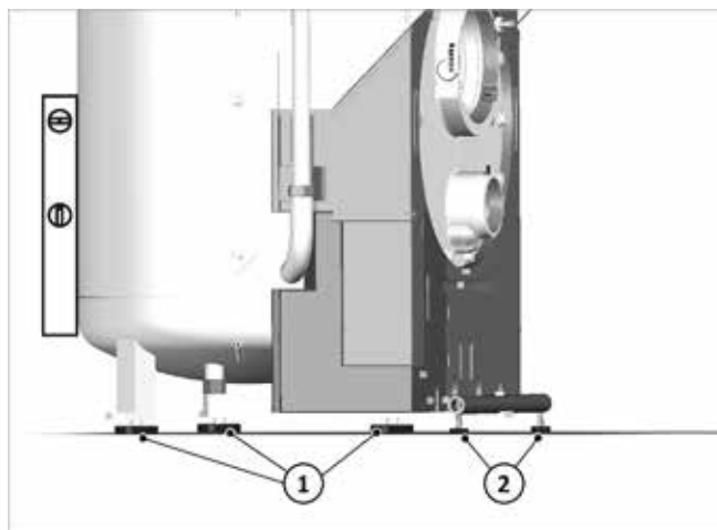
Fig. 5: Colocación del acumulador
