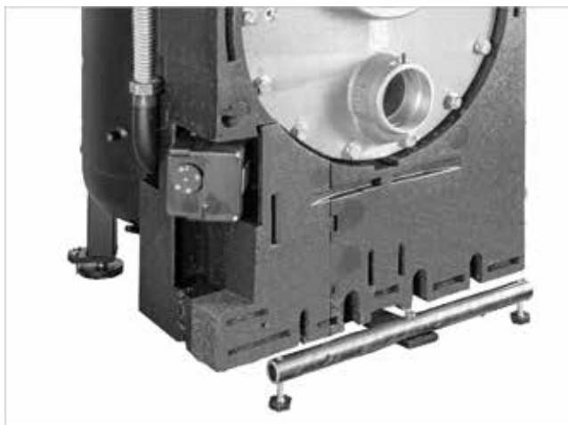
Afb. 11: Gemonteerd elektrische verwarmingselement
