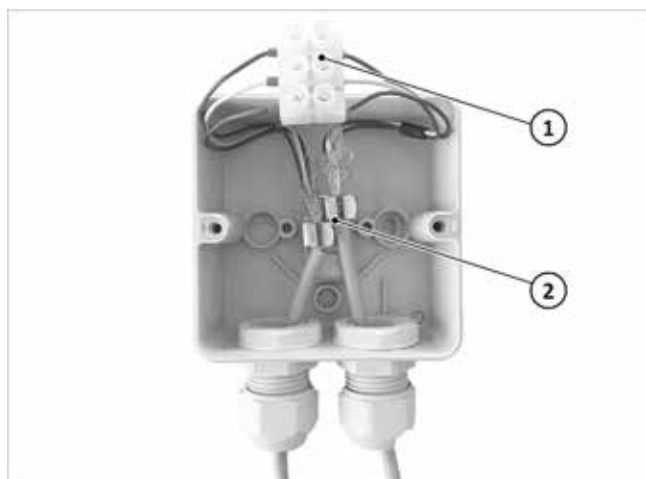
Afb. 106: Modbus-verbindingsdoos bevestigen
