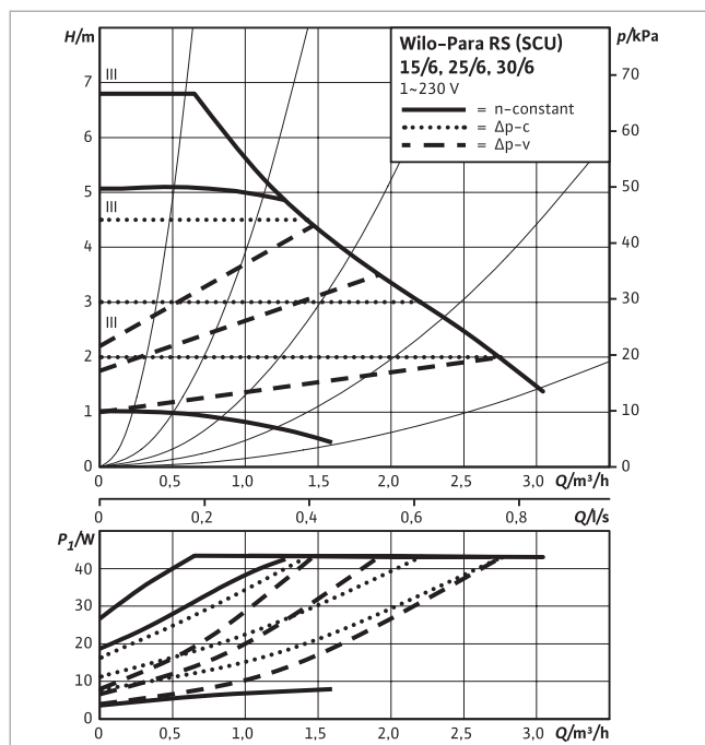
Afb. 148: Pompkarakteristiek Wilco-Para 15/6 SCU
