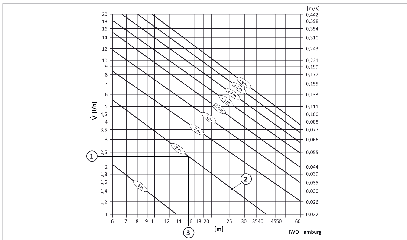
Afb. 82: Maximale leidinglengte in een één-leidingsysteem afhankelijk van de opvoerhoogte
