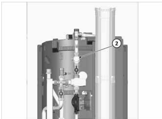
Afb. 27: De schroefkoppeling van de aanvoerleiding controleren/vast-draaien
