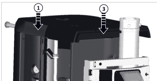
Afb. 125: Koppelingsprofiel links en voor
