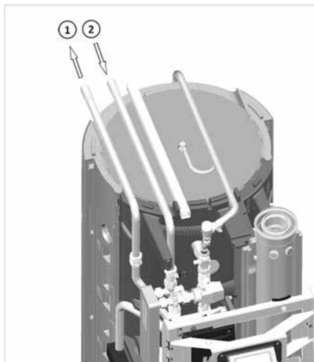
Afb. 29: TWW-/TWK-aansluiting achter
