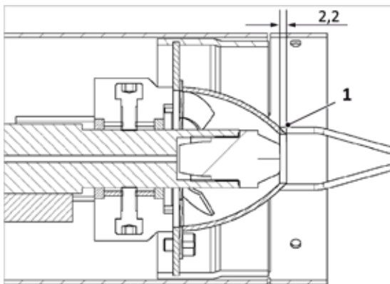
Afb. 142: Dwarsdoorsnede van mengkop
