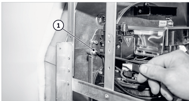
Afb. 139: Snelsluitbouten op het branderinzetstuk
