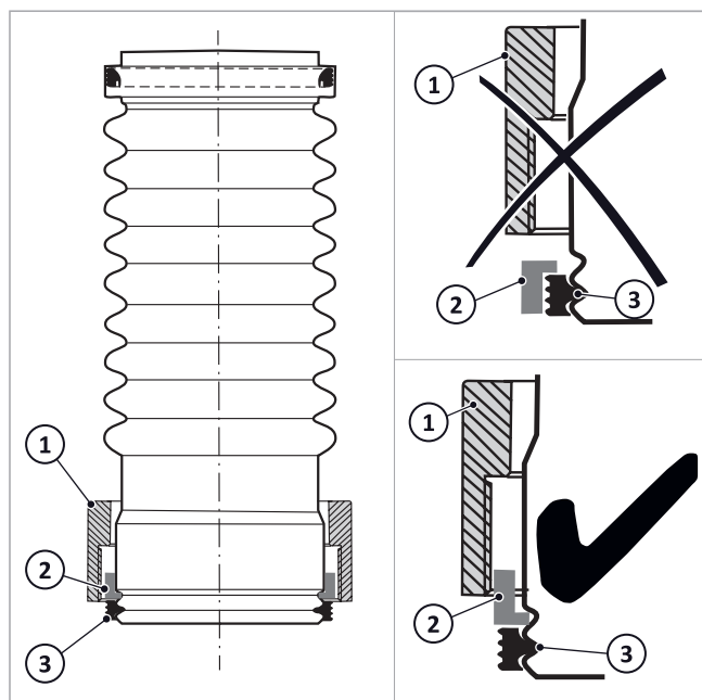
Afb.83: Schroefkoppeling opgestoken
