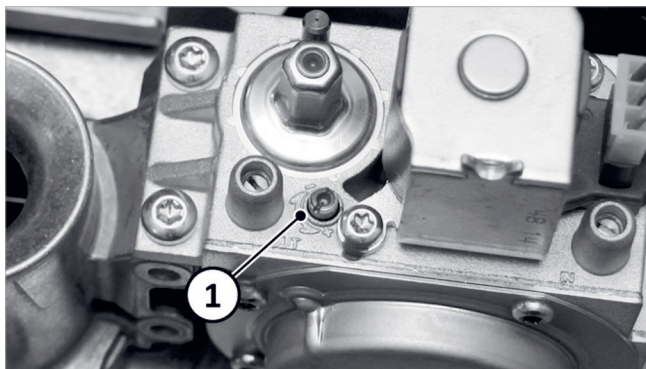
Afb. 43: Brander instellen
