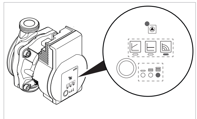
Afb. 117: Basisinstelling (constant toerental, grafiek III)
