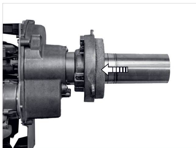
Afb. 67: Keteldeurisotatie plaatsen
