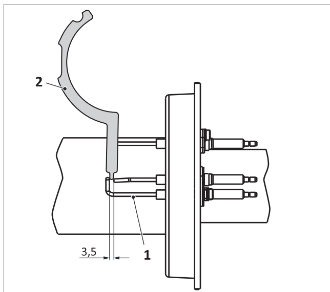
Afb. 138: Afstand elektrode naar de massa op de ontstekingselektrode
