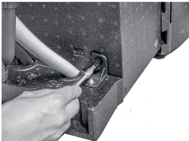
Afb. 92: Beugel bevestigen
