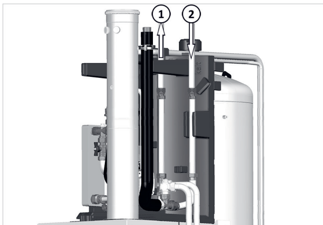
Afb. 39: H-VL/H-RL-aansluiting van bovenaf
