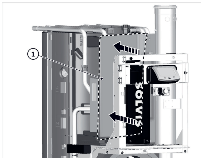
Afb. 107: Het voorste isolatiedeksel van de WWS erop steken
