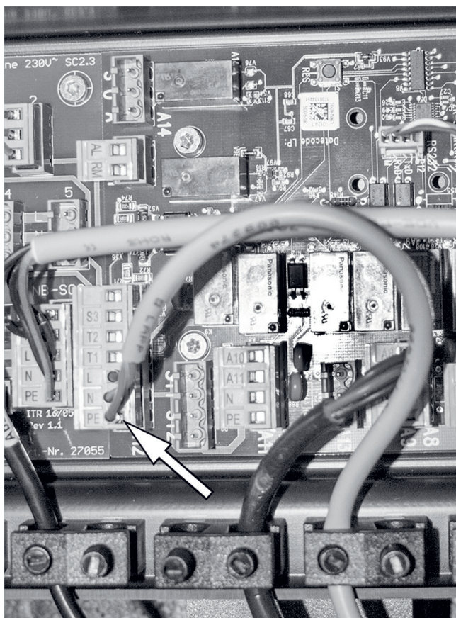
Afb. 73: Aansluiting branderstekker oliebrander op A12
