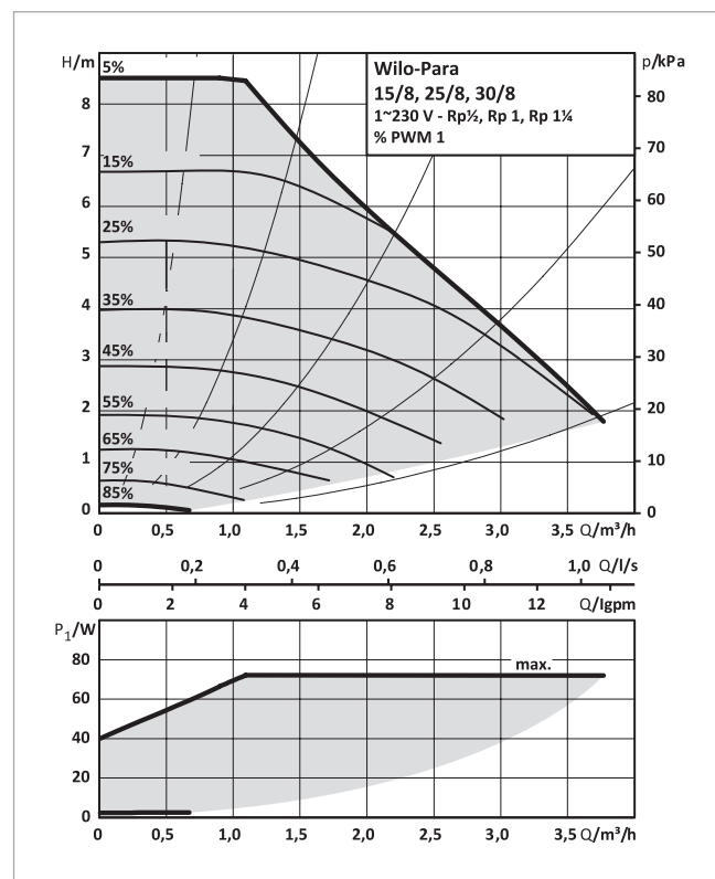
Afb. 149: Pompkarakteristieken Wilo PARA 15/8
