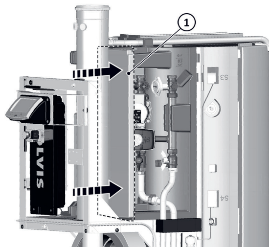
Afb. 108: Het voorste isolatiedeksel van de HKS erop steken
