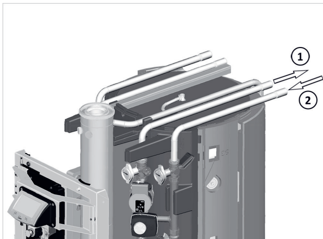
Afb. 34: H-VL/H-RL-aansluiting van achteren
