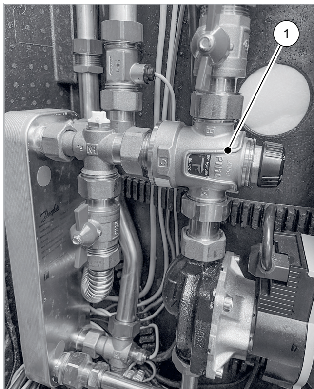
Afb. 111: Thermostatische mengklep (1) in de WWS SolvisBen
