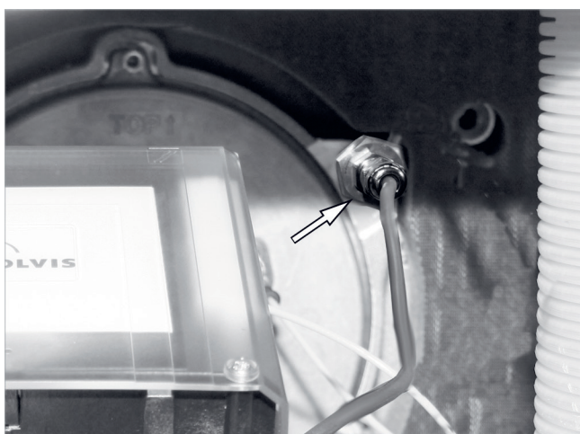
Afb. 69: eSTB insteken
