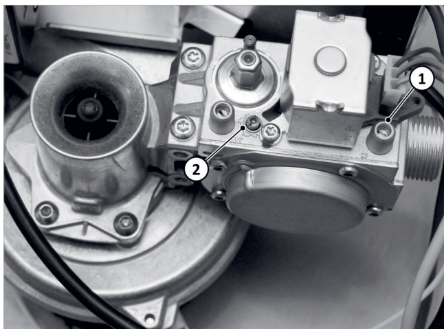
Afb. 113: Brander instellen
