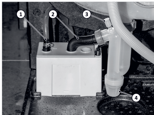
Afb. 87: Condenspomp, aangesloten
