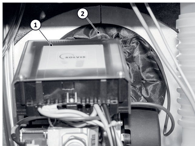
Afb. 97: De branderuitsparing is met een kraag geïsoleerd.
