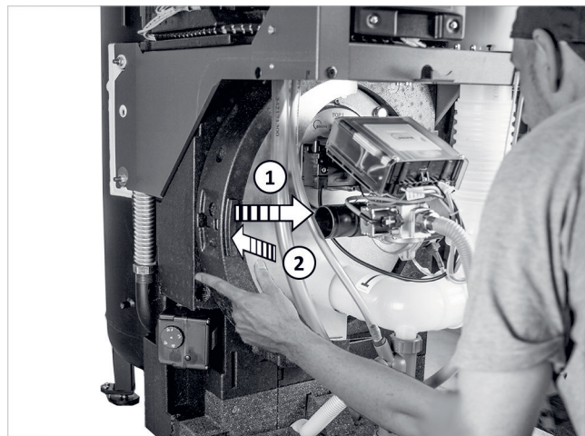
Afb. 96: Inbouw voorste flensisolatie
