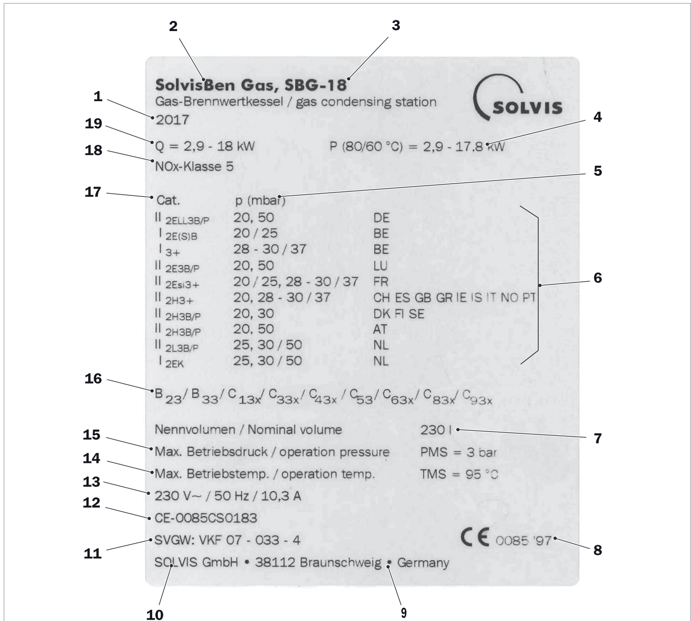
Afb. 154: Voorbeeld typeplaatje SolvisBen Gas
