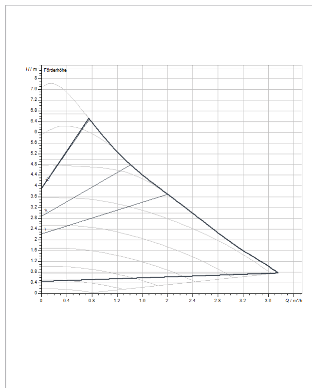
Afb. 150: Pompkarakteristieken Varios PICO-STG 15/1-7
