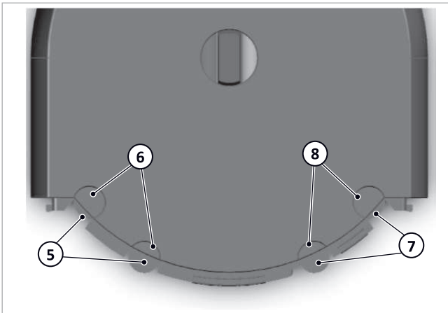
Afb. 119: Opensnijden van de leidingdoorvoeren
