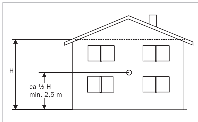
Afb. 102: Positie van de buitensensor
