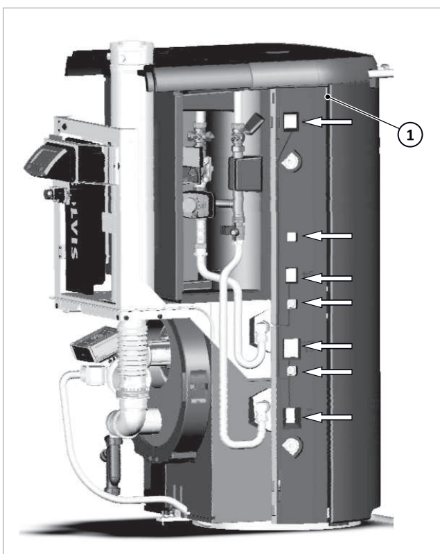
Afb. 127: Vliesstoppen rechter kant
