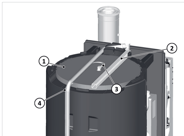
Afb. 18: Rond deksel en kabelkanalen plaatsen
