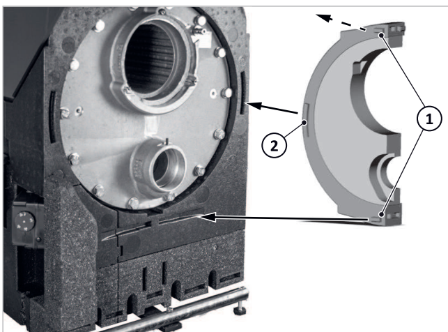
Afb. 95: Voorste flensisolatie (rechts, achteraanzicht) met vergrendelingsveren
