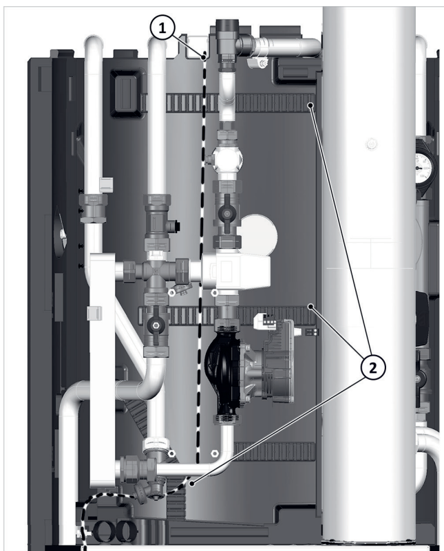
Afb. 99: Kabelgeleiding door de WWS-isolatie
