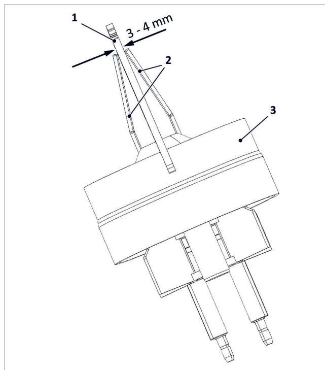
Afb. 145: De afstand van de ontstekingselektroden controleren
