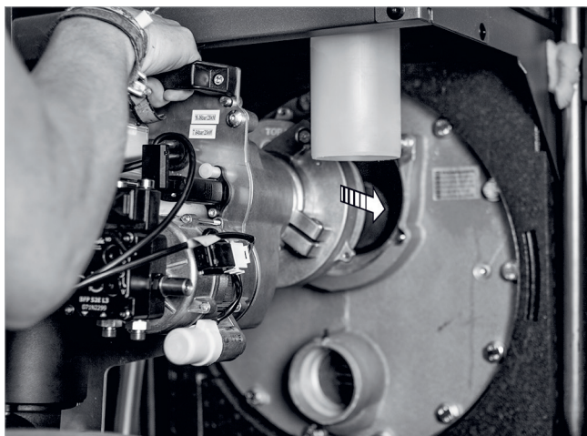
Afb. 68: Brander monteren
