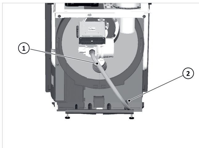
Afb. 58: Gasleiding naar beneden leggen
