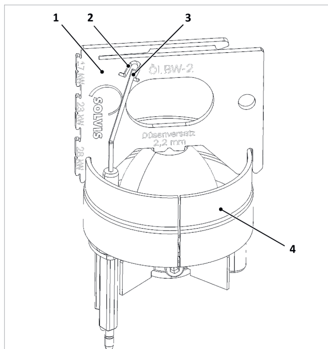
Afb. 144: Ontstekingselektroden controleren
