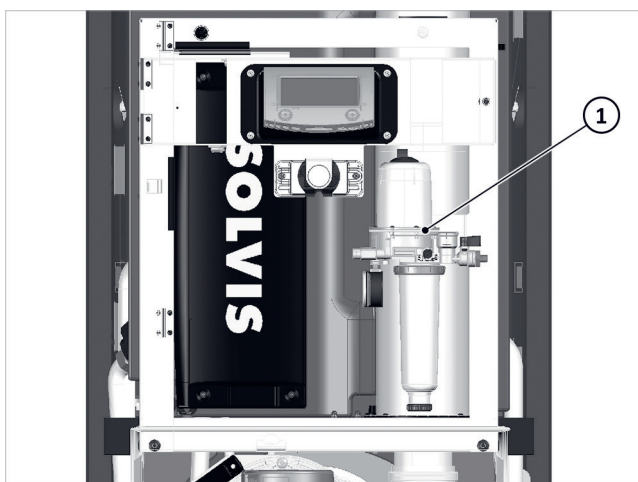
Afb. 75: Oliefilter op houder gestoken
