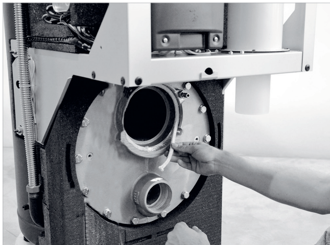
Afb. 64: Branderpakkingsnoer aanbrengen
