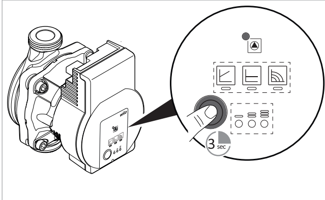
Afb. 115: Ontluchting starten
