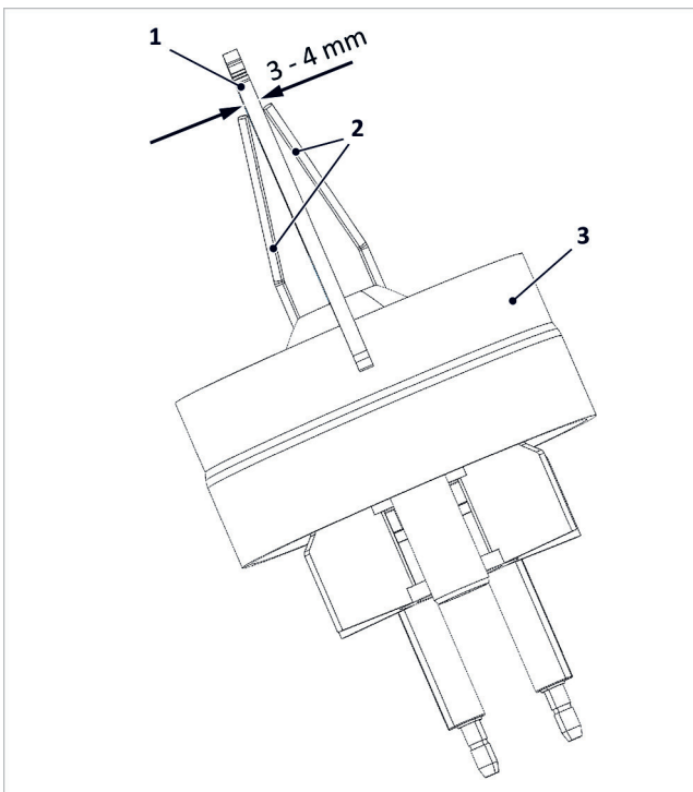
Afb. 66: De afstand van de ontstekingselektroden controleren
