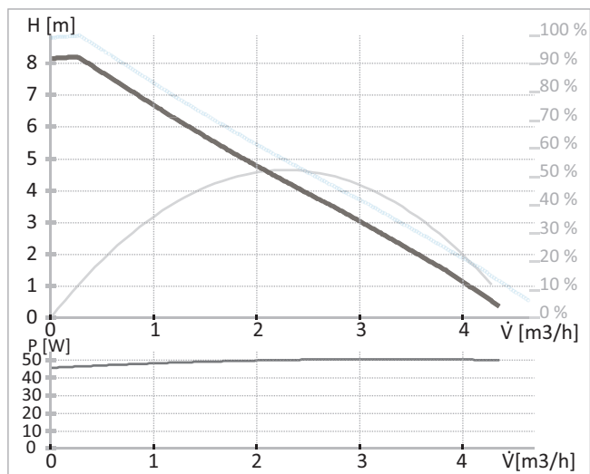
Afb. 151: Pompkarakteristiek IMP NMT Mini PWM 15/80-130 (constant toerental)
