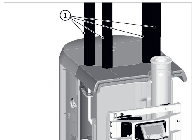
Afb. 123: Bovenste isolatiedelen met de aansluitingen van bovenaf
