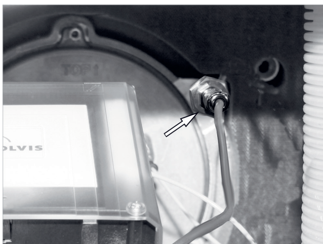
Afb. 50: eSTB insteken
