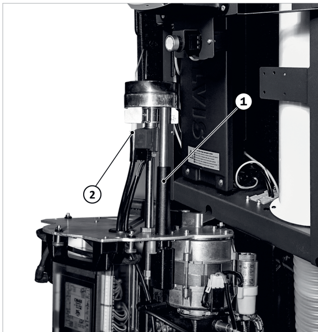
Afb. 140: Brander op console inhaken
