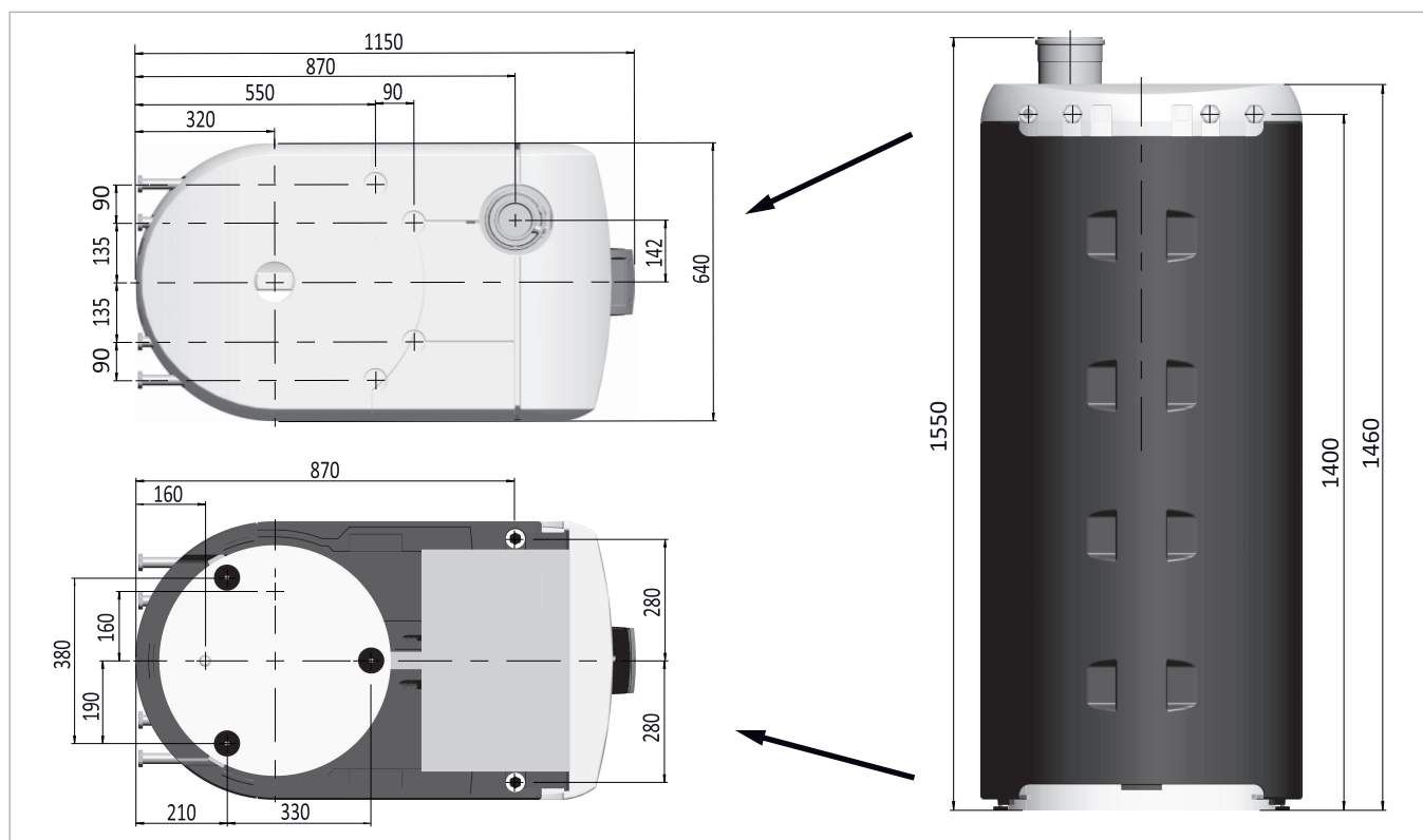
Afb. 146: Aanzichten SolvisBen (alle afmetingen in mm)
