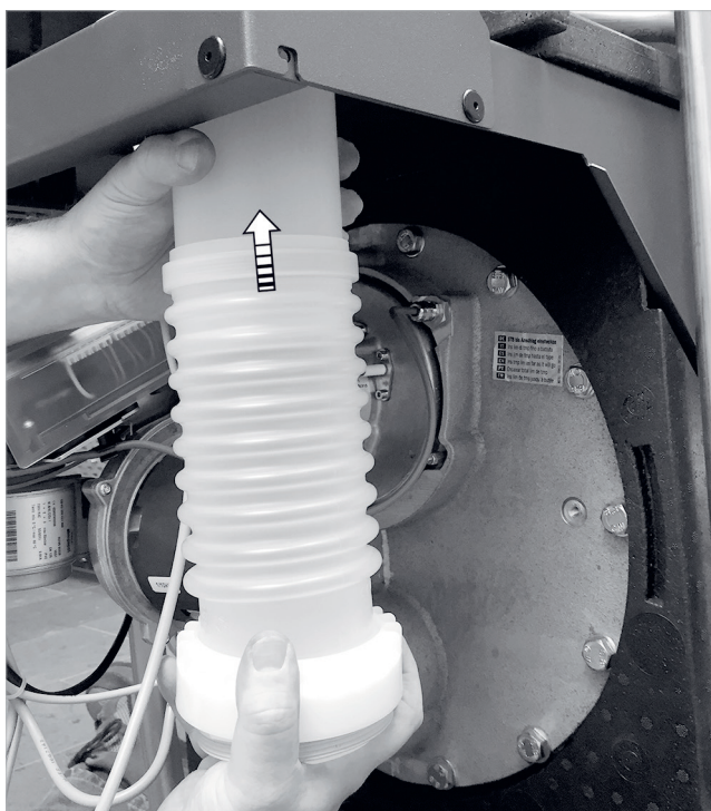
Afb.84: Het aansluitstuk voor rookgas op de rookgaspijp steken.
