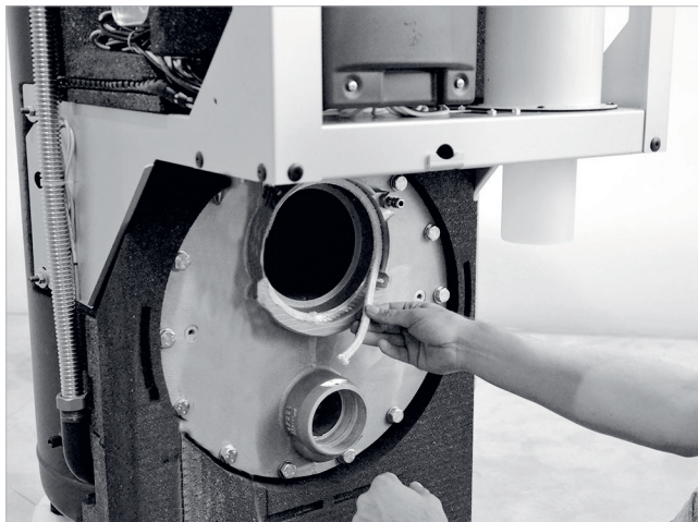
Afb. 46: Branderpakingsnoer aanbrengen
