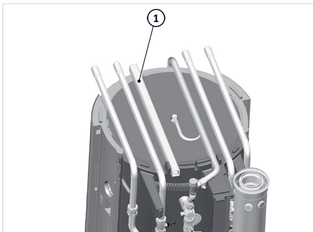
Afb. 98: Kabelkanaal
