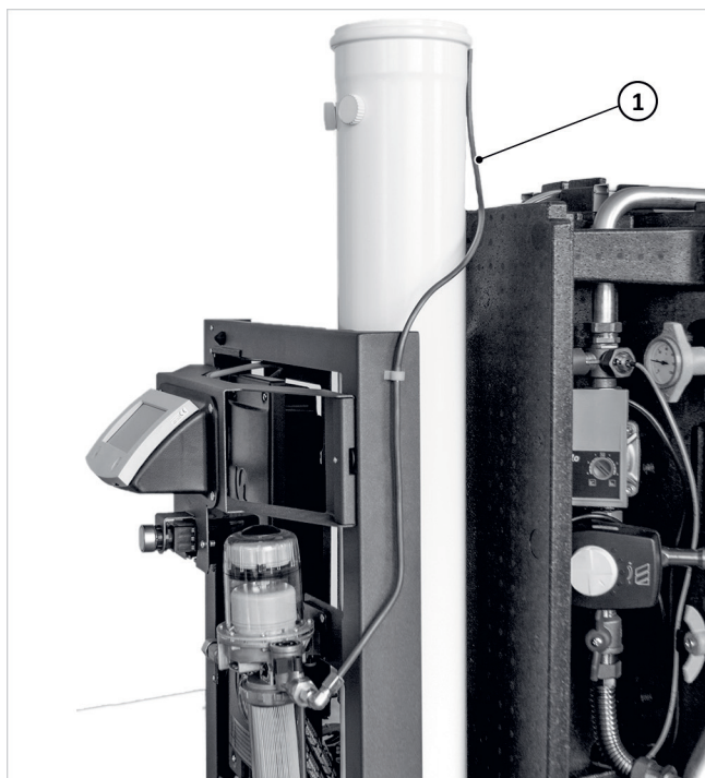
Afb. 77: Olietoevoerleiding achter afvoerbuis leiden
