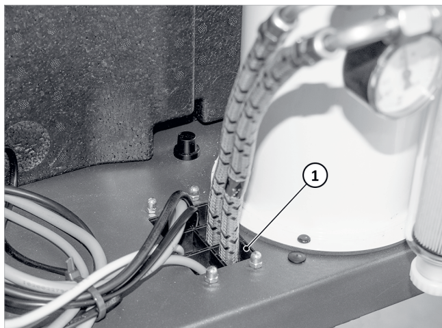
Afb. 76: Doorvoer olieleiding in basisplaat
