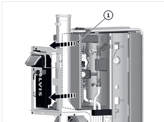
Afb. 30: Het voorste isolatiedeksel van de HKS verwijderen
