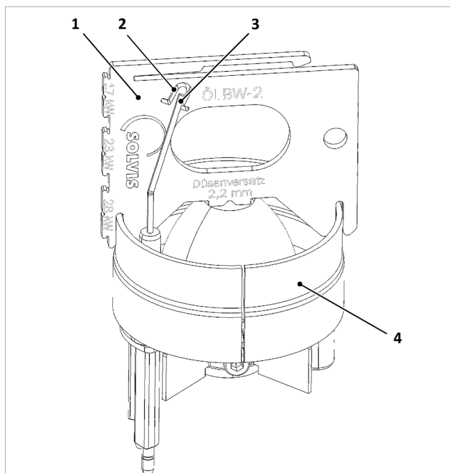
Afb. 65: Stand van de ontstekingselektroden controleren
