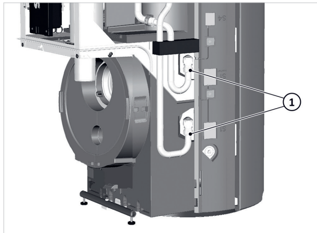
Afb. 31: De aansluitingen van de HKS controleren/vastdraaien
