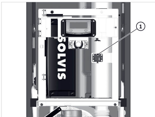
Afb. 74: Oliefilterhouder bevestigen
