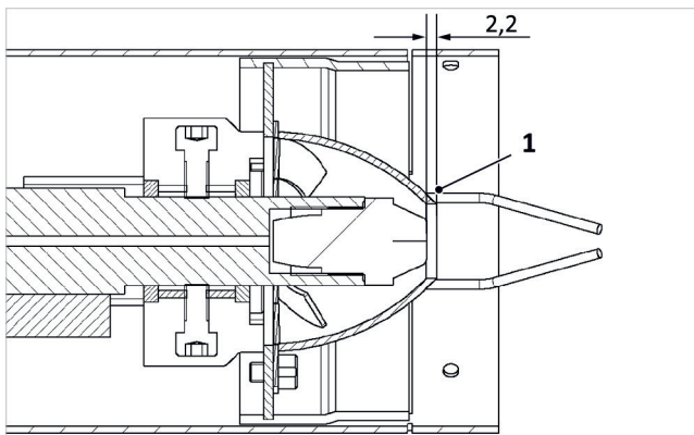
Afb. 142: Dwarsdoorsnede van mengkop
