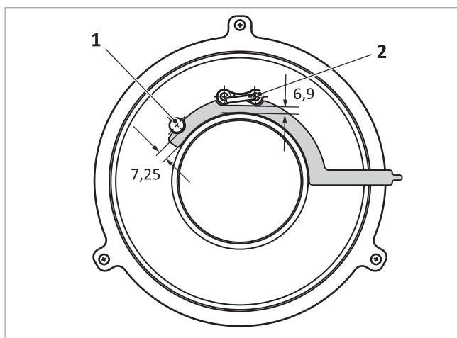
Afb. 137: Afstanden ionisatie- en ontstekingselektrode naar brandervezel-laag
