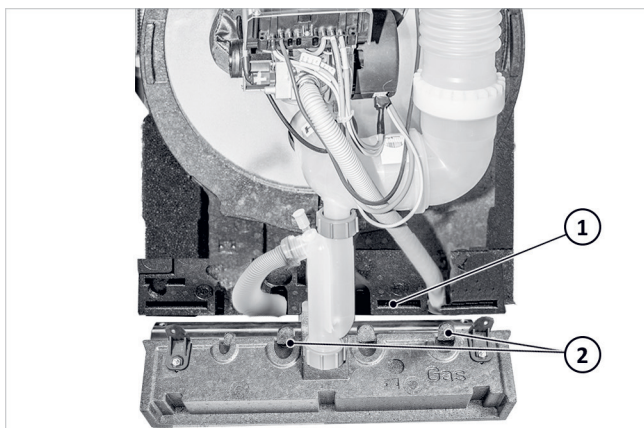
Afb. 90: Leidingen door het vloerdeel geleiden
