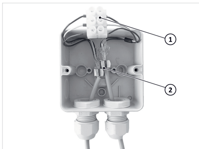
Afb. 106: Modbus-verbindingsdoos bevestigen
