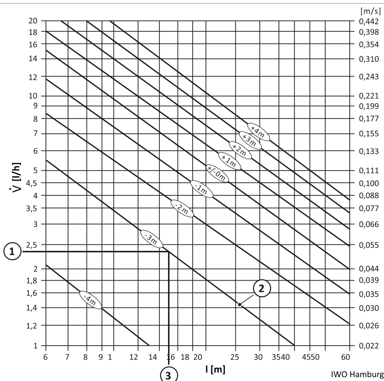
Afb. 82: Maximale leidinglengte in een één-leidingsysteem afhankelijk van de opvoerhoogte
