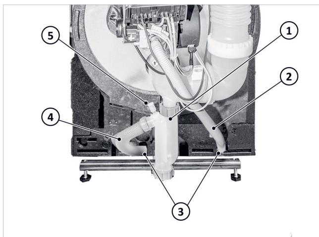
Afb. 86: Toevoer- en afvoerleidingen zonder condenspomp
