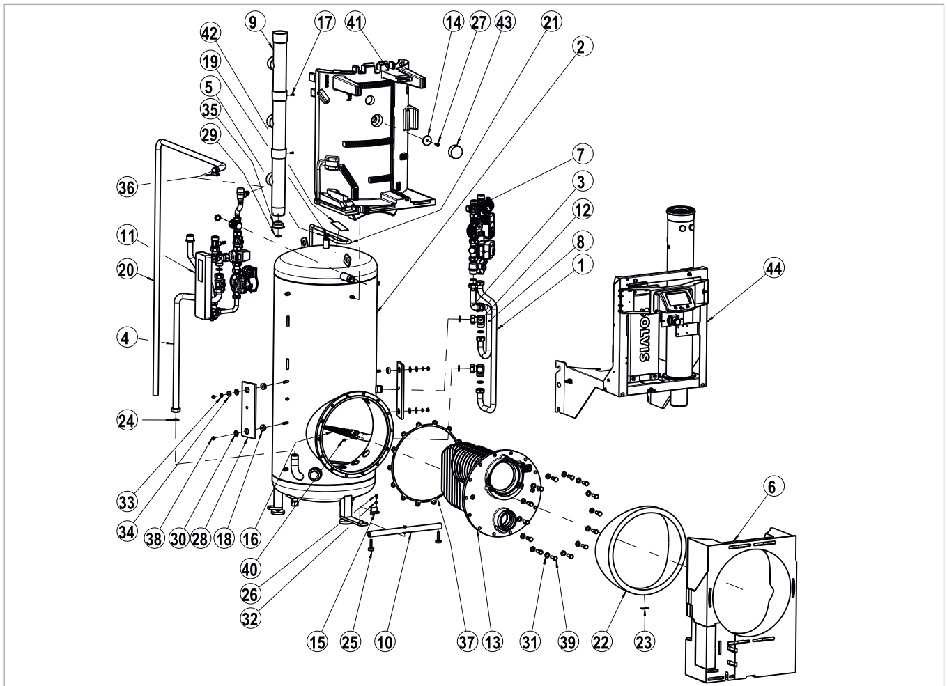
Afb. 153: Overzicht vervangende onderdelen SolvisBen met WWS en HKS (voor alle leverbare onderdelen zie → TNF-EST-BEN)
