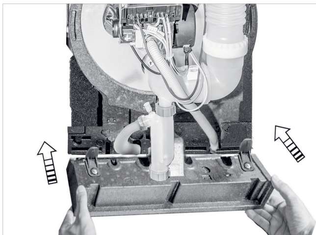
Afb. 91: Vloerdeel gelijkliggend inschuiven.
