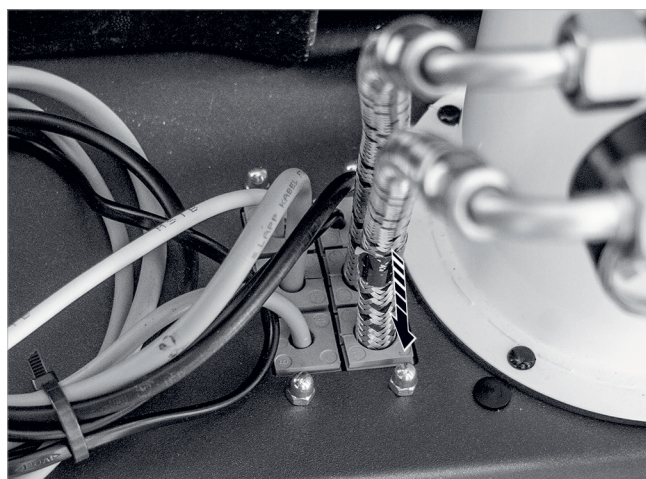
Afb. 81: Tules in de inlay drukken
