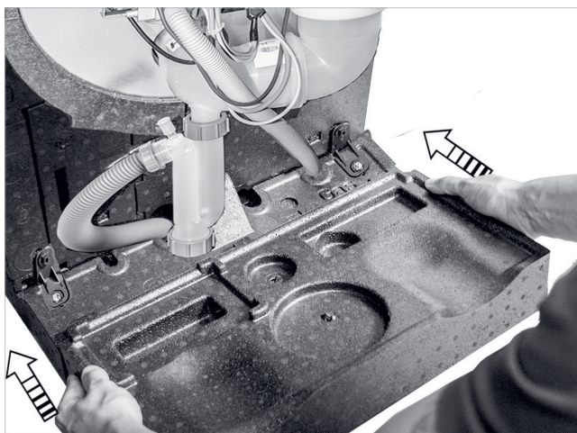
Afb. 93: Voorste vloerdeel monteren
