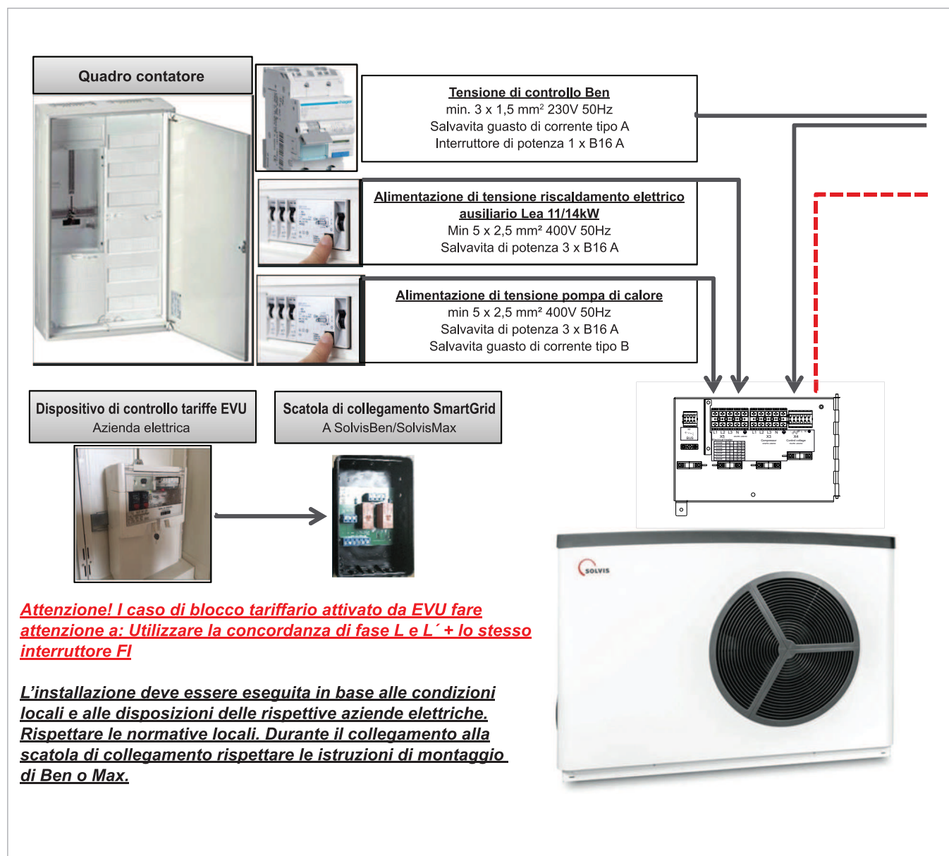
Fig. 1: Supporto di montaggio per SolvisBen WP con SolvisLea Eco 11/14 kW e collegamento a EVU - Parte 1
