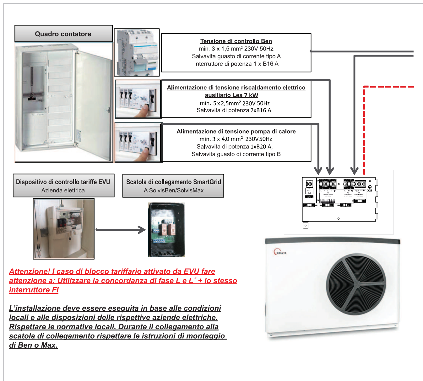
Fig. 3: Supporto di montaggio per SolvisBen WP con SolvisLea Eco 7 kW e collegamento a EVU - Parte 1
