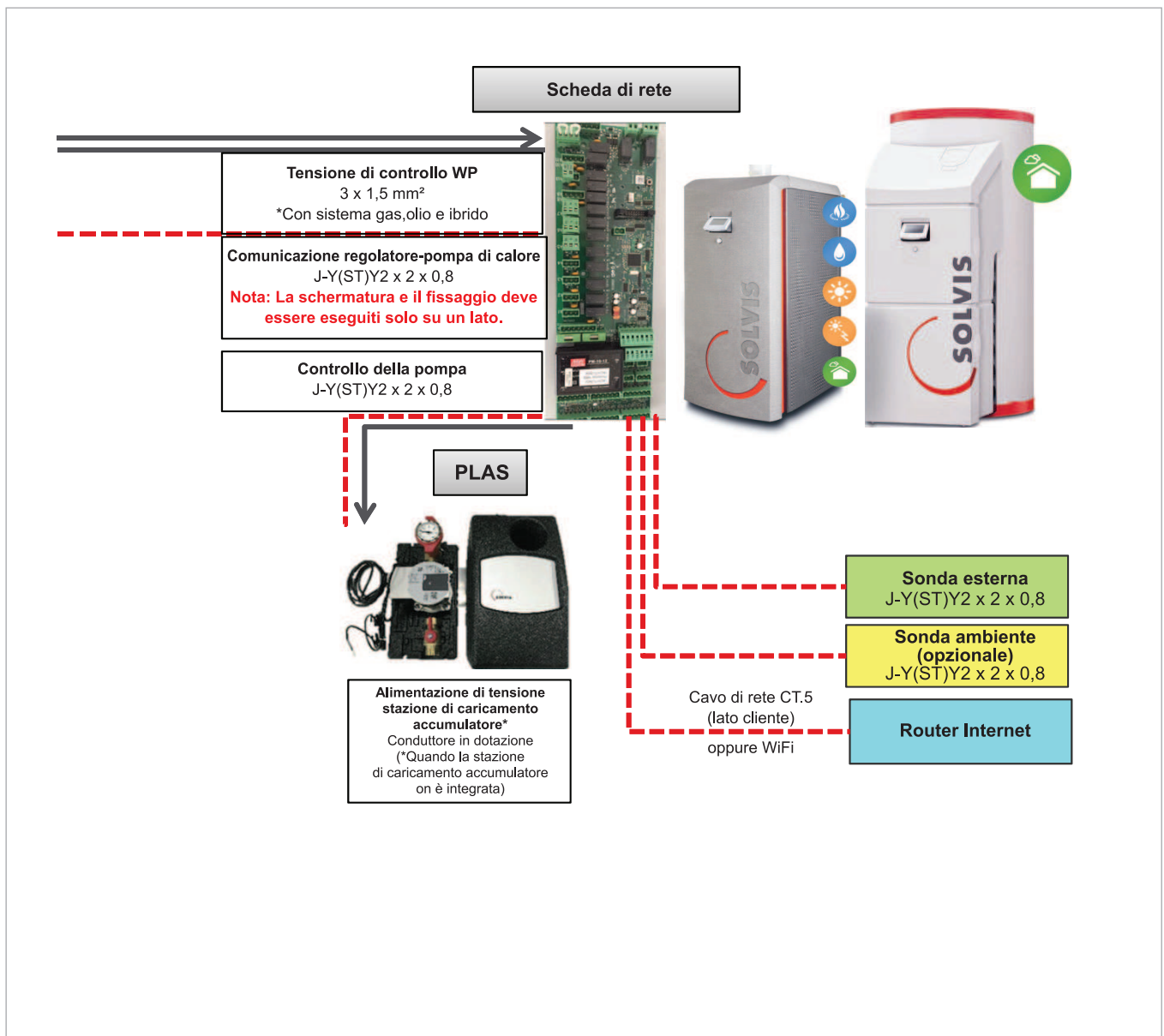
Fig. 4: Supporto di montaggio per SolvisBen WP con SolvisLea Eco 7 kW e collegamento a EVU - Parte 2
