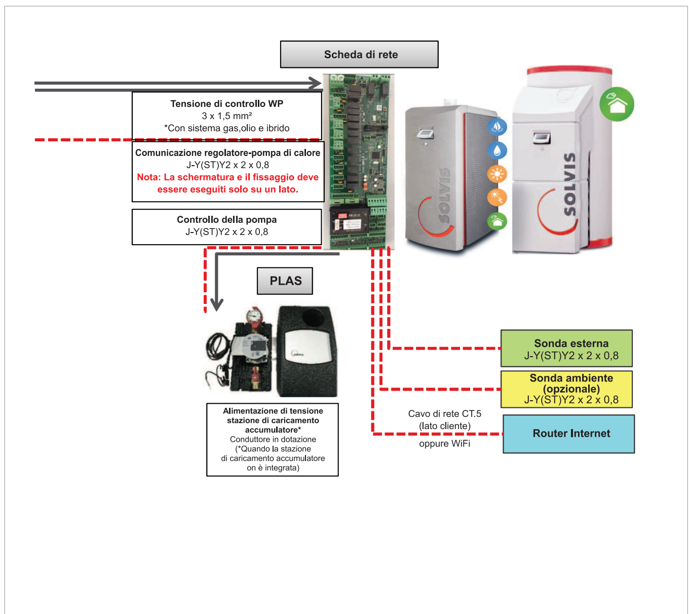
Fig. 2: Supporto di montaggio per SolvisBen WP con SolvisLea Eco 11/14 kW e collegamento a EVU - Parte 2
