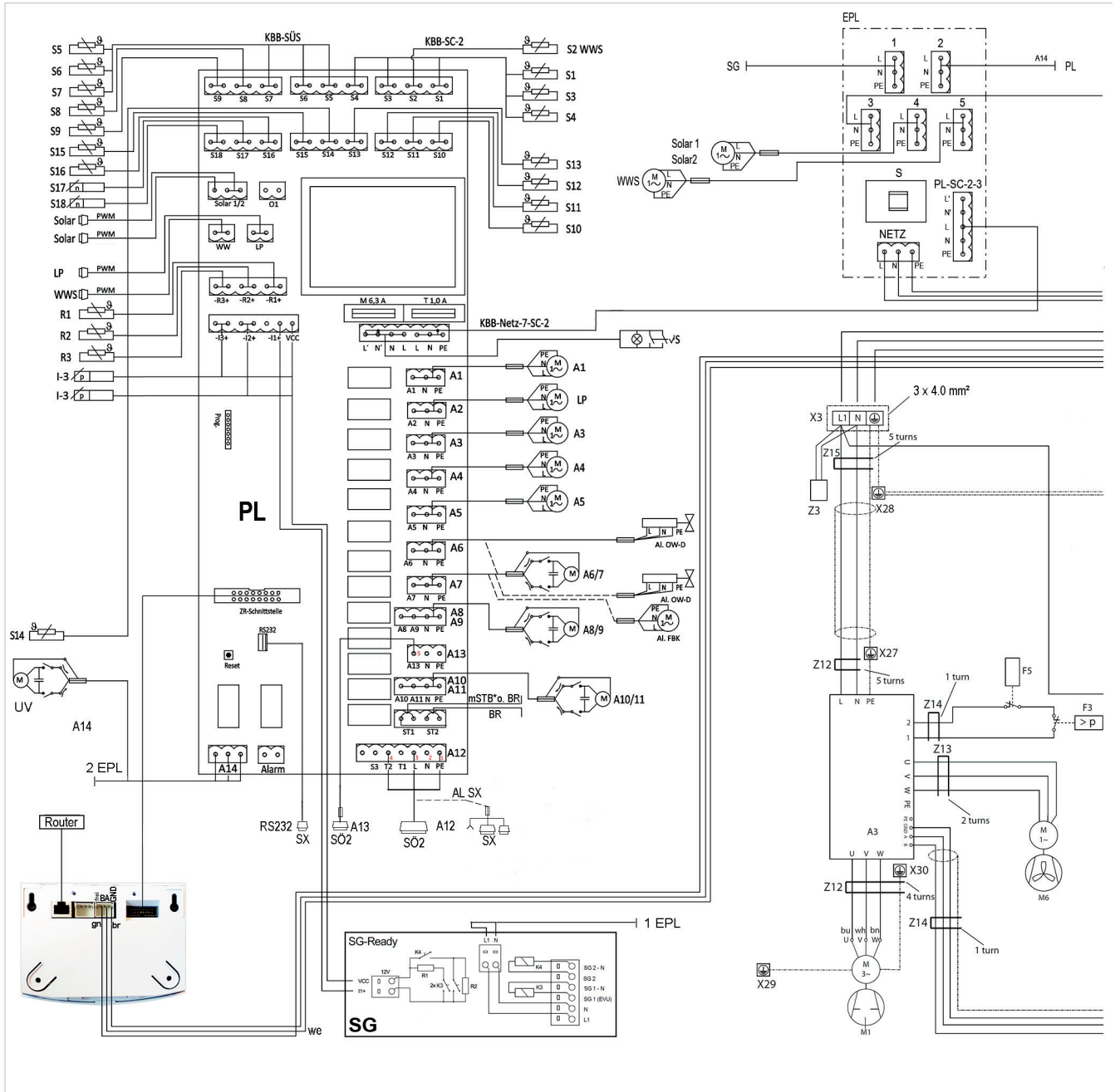
Fig. 24: Schema elettrico SolvisLea Eco - Parte 1
