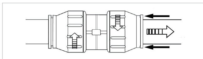
Fig. 10: Allentare un collegamento a innesto
