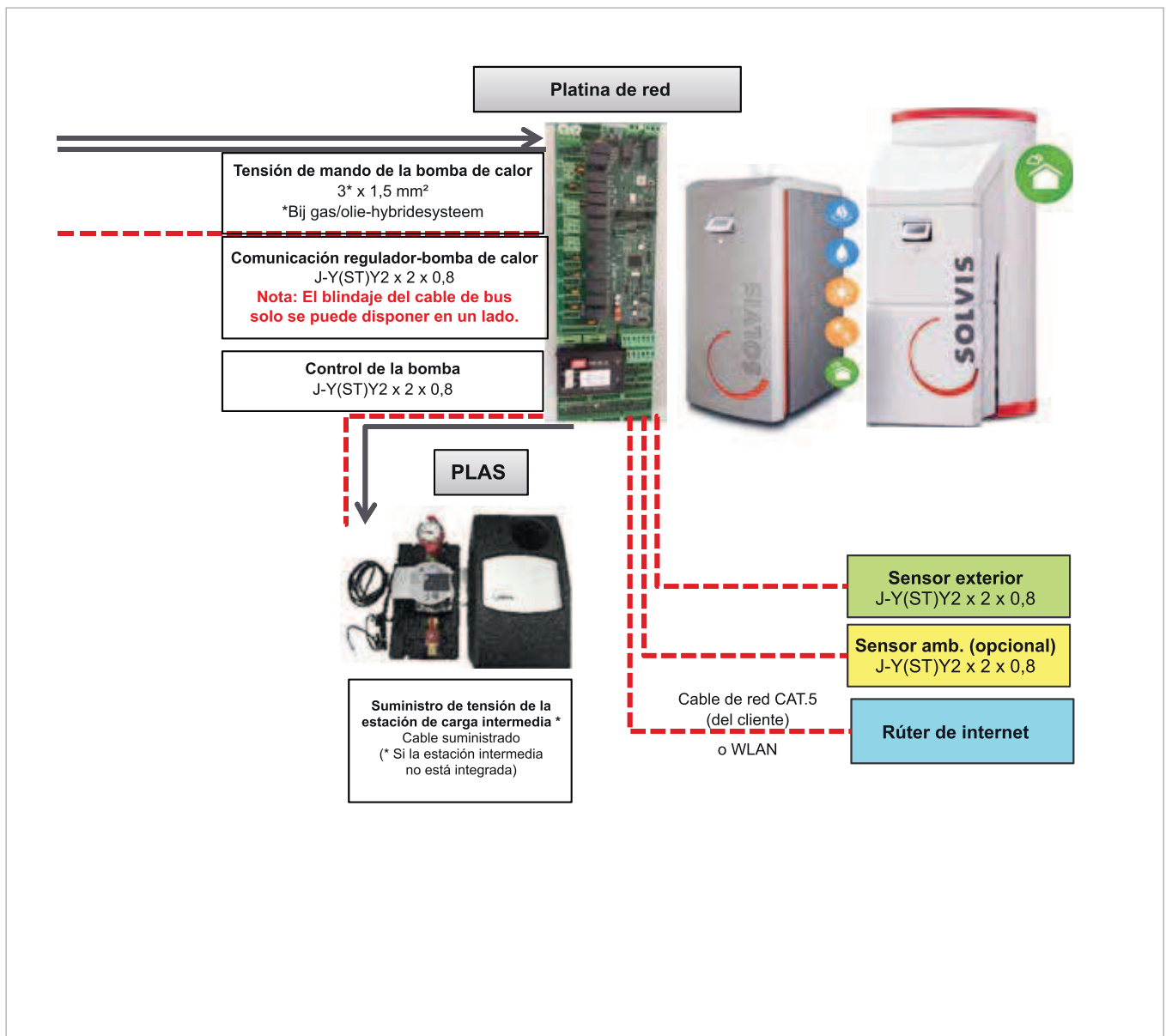
Fig. 4: Instrucciones de montaje de SolvisBen WP con SolvisLea Eco 7 kW y conexión EVU, parte 2
