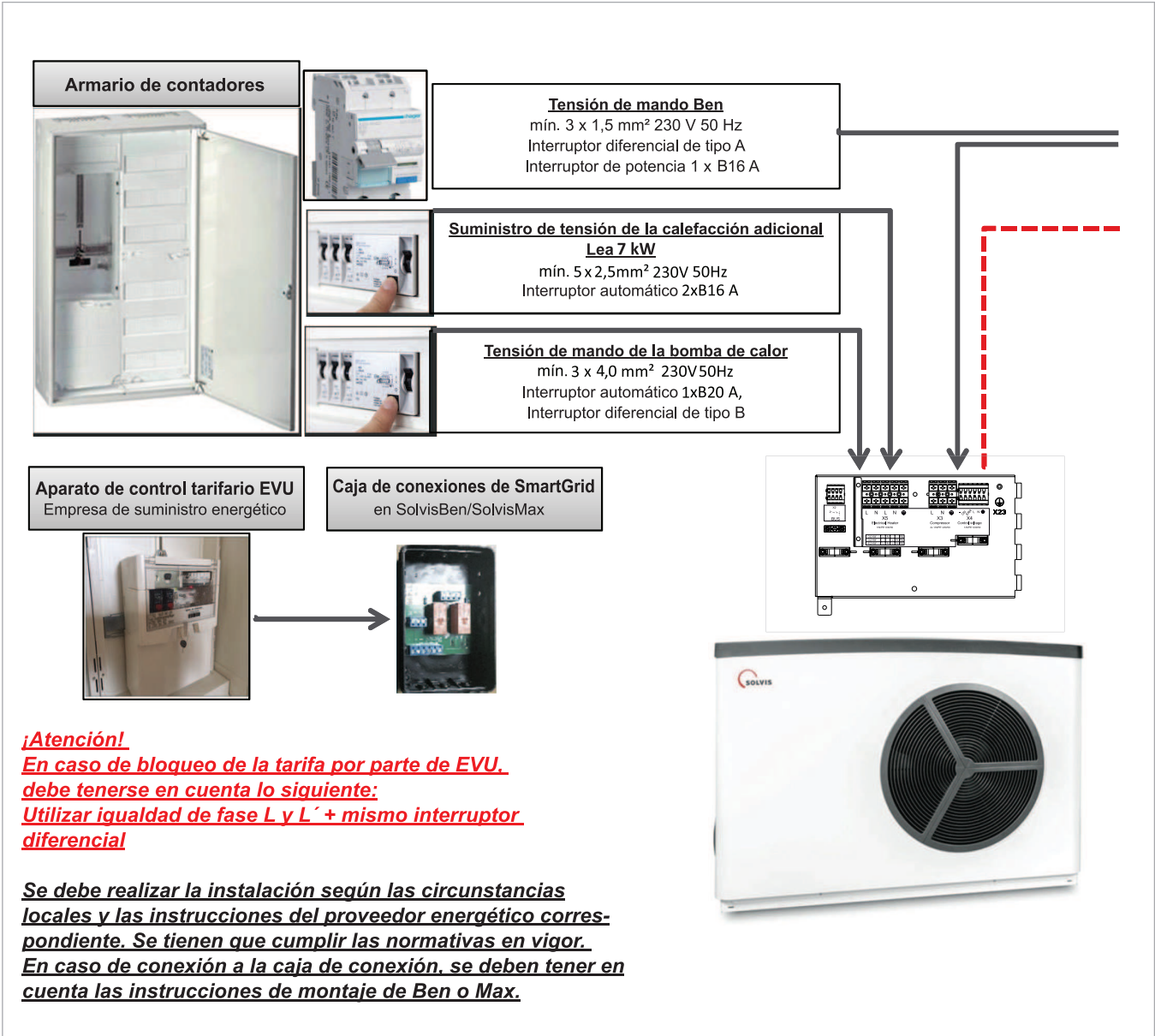
Fig. 3: Instrucciones de montaje de SolvisBen WP con SolvisLea Eco 7 kW y conexión EVU, parte 1
