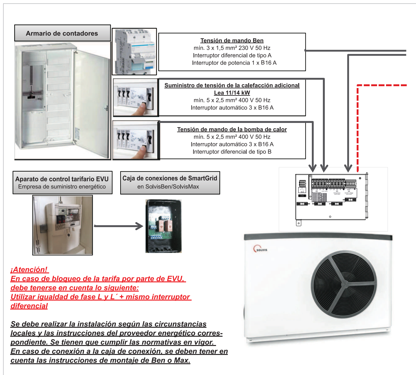
Fig. 1: Instrucciones de montaje de SolvisBen WP con SolvisLea Eco 11/14 kW y conexión EVU, parte 1
