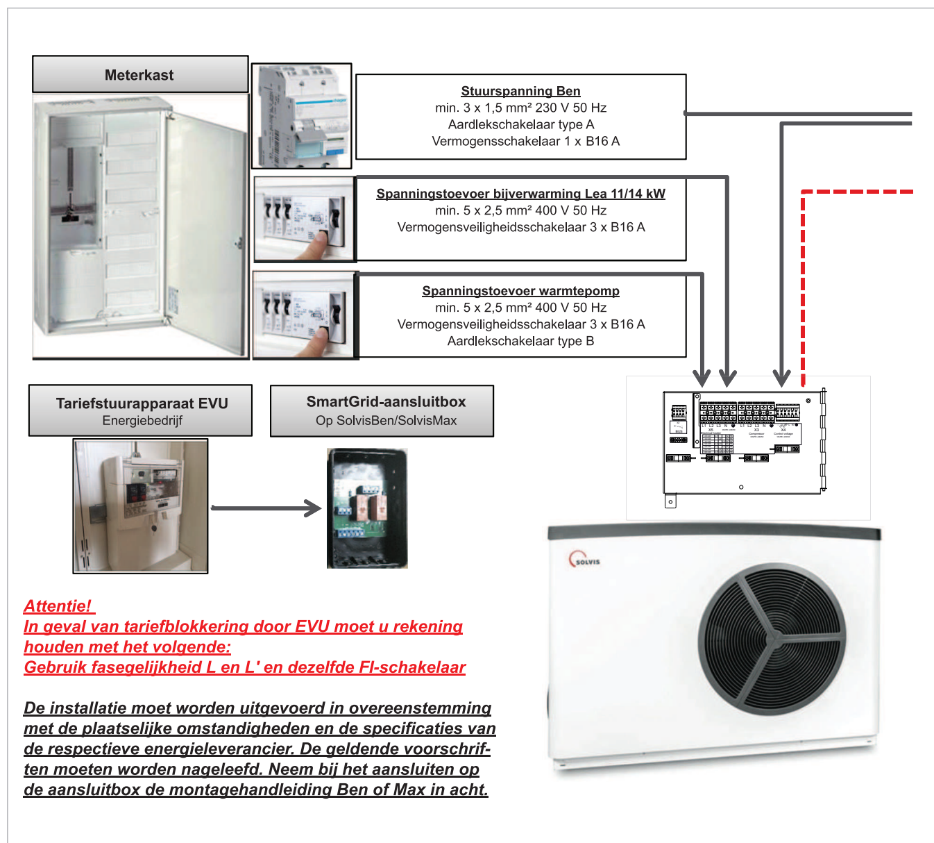
Afb. 1: Montagehulp SolvisBen WP met SolvisLea Eco 11/14 kW en EVU-verbinding - Deel 1
