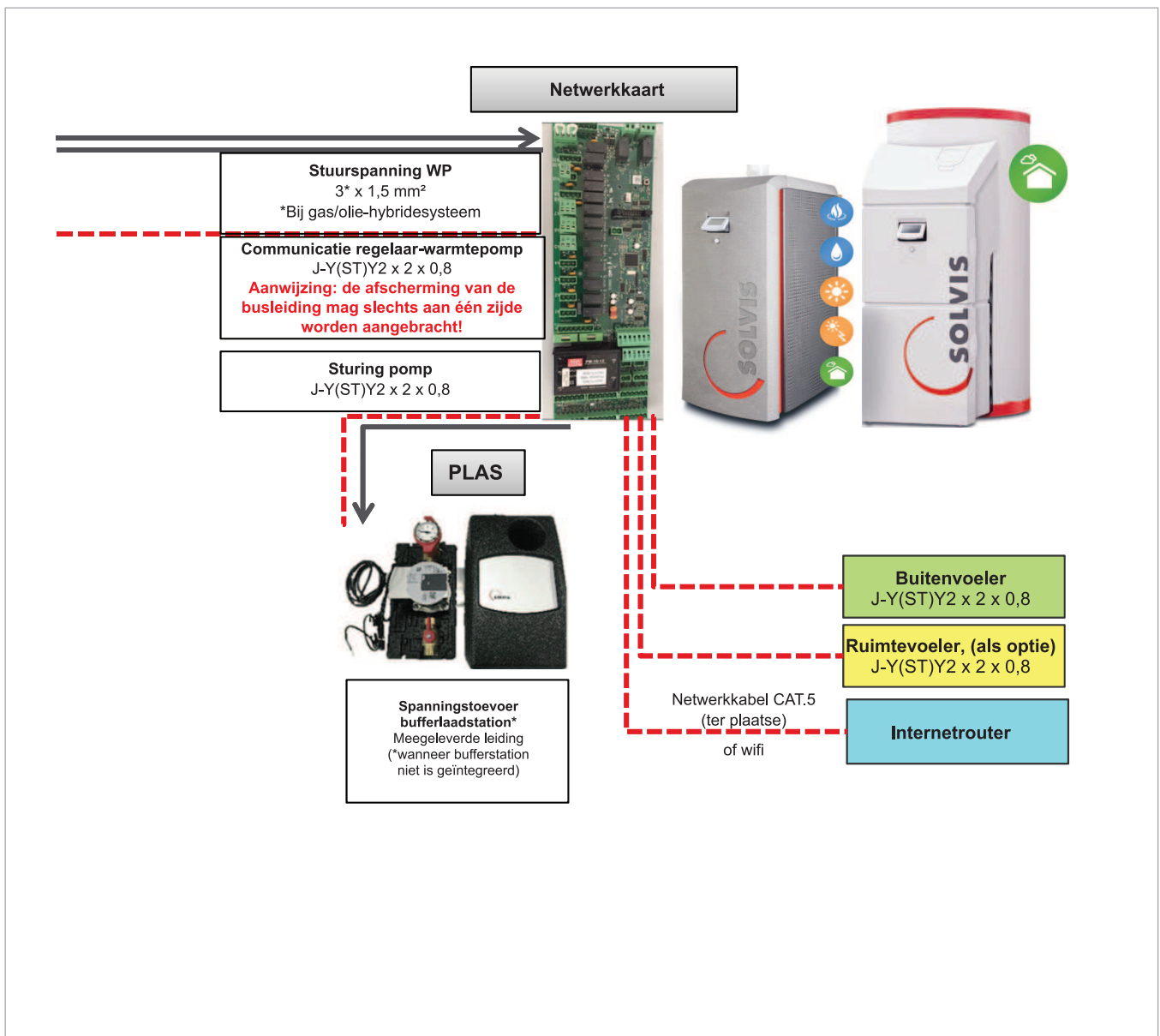
Afb. 4: Montagehulp SolvisBen WP met SolvisLea Eco 7 kW en EVU-verbinding - Deel 2
