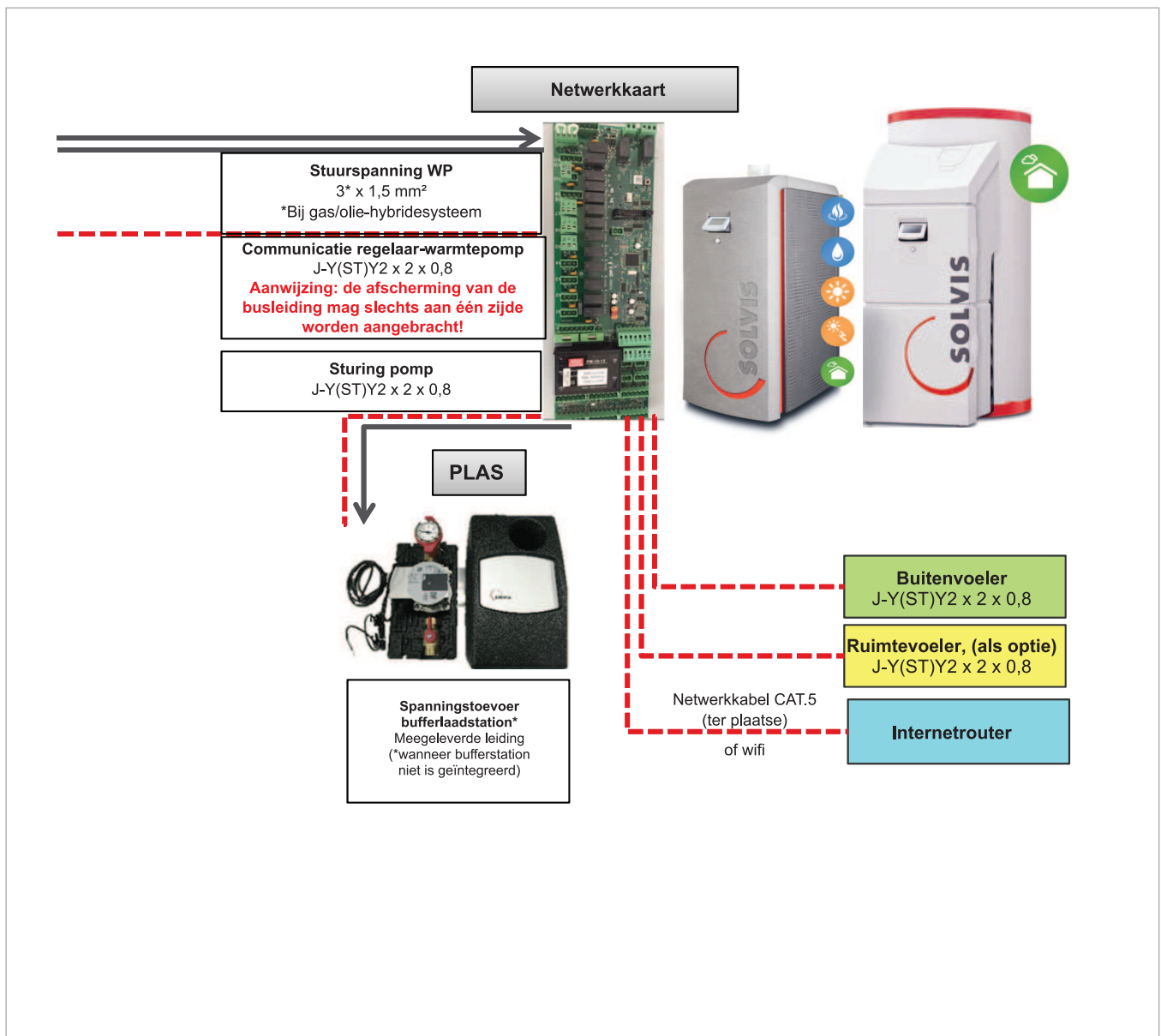
Afb. 2: Montagehulp SolvisBen WP met SolvisLea Eco 11/14 kW en EVU-verbinding - Deel 2
