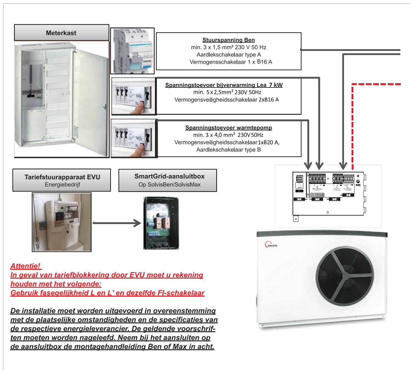
Afb. 3: Montagehulp SolvisBen WP met SolvisLea Eco 7 kW en EVU-verbinding - Deel 1
