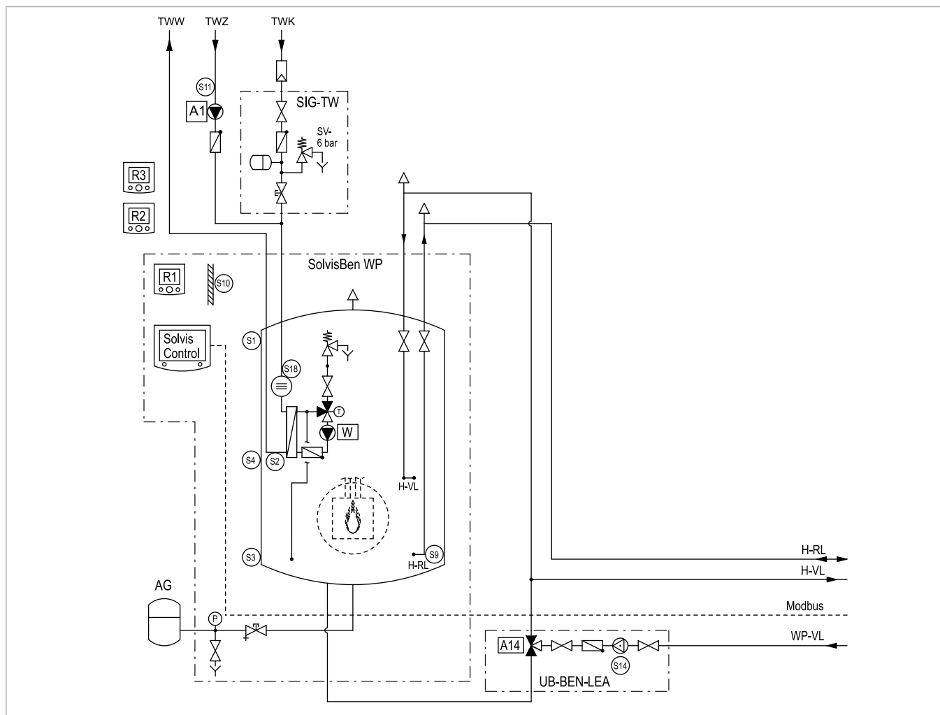
Fig. 19: SolvisBen WP tre circuiti di riscaldamento misti e pompa di calore SolvisLea - Parte 1
