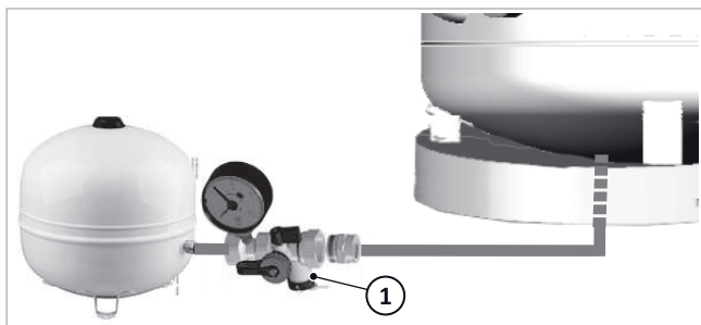
Fig. 15: Valvola KFE al gruppo di collegamento MAG
