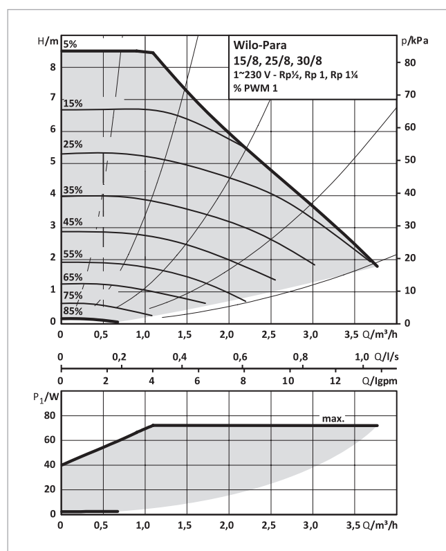
Fig. 16: Curva caratteristica della pompa Wilo-PARA 15/8
