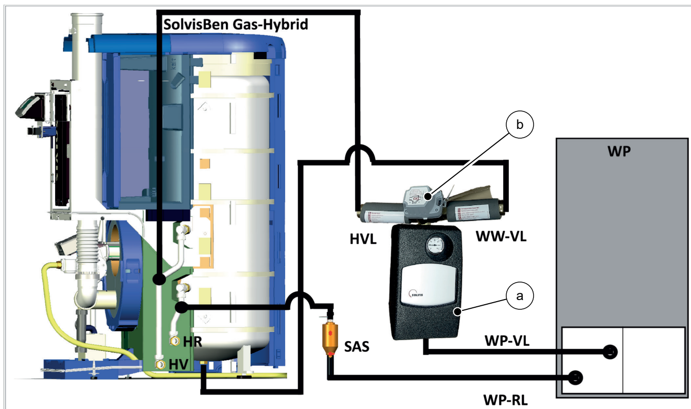
Fig. 8: Panoramica collegamento SolvisLea a SolvisBen GAS-Hybrid senza stazione di riscaldamento integrata (HKS)
