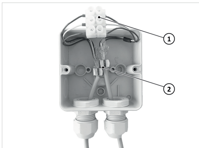
Fig. 12: fissaggio scatola di distribuzione Modbus
