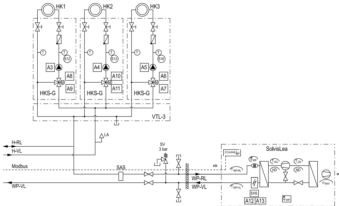
Fig. 20: SolvisBen WP 3 stazione circuito di riscaldamento misto e pompa di calore SolvisLea - Parte 2
