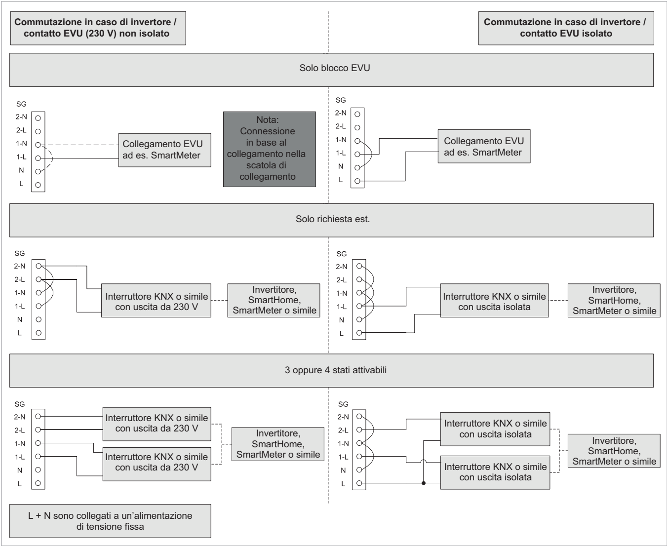
Fig. 24: opzioni di collegamento SmartGrid per la scheda di rete di SolvisControl 3
