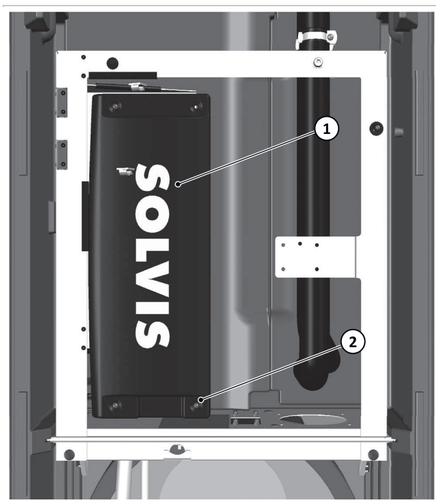
Fig. 14: fissaggio del coperchio della scheda di rete
