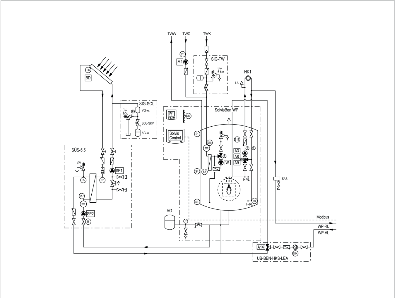
Fig. 17: SolvisBen Lino con stazione circuito di riscaldamento integrata, impianto solare e pompa di calore SolvisLea - Parte 1
