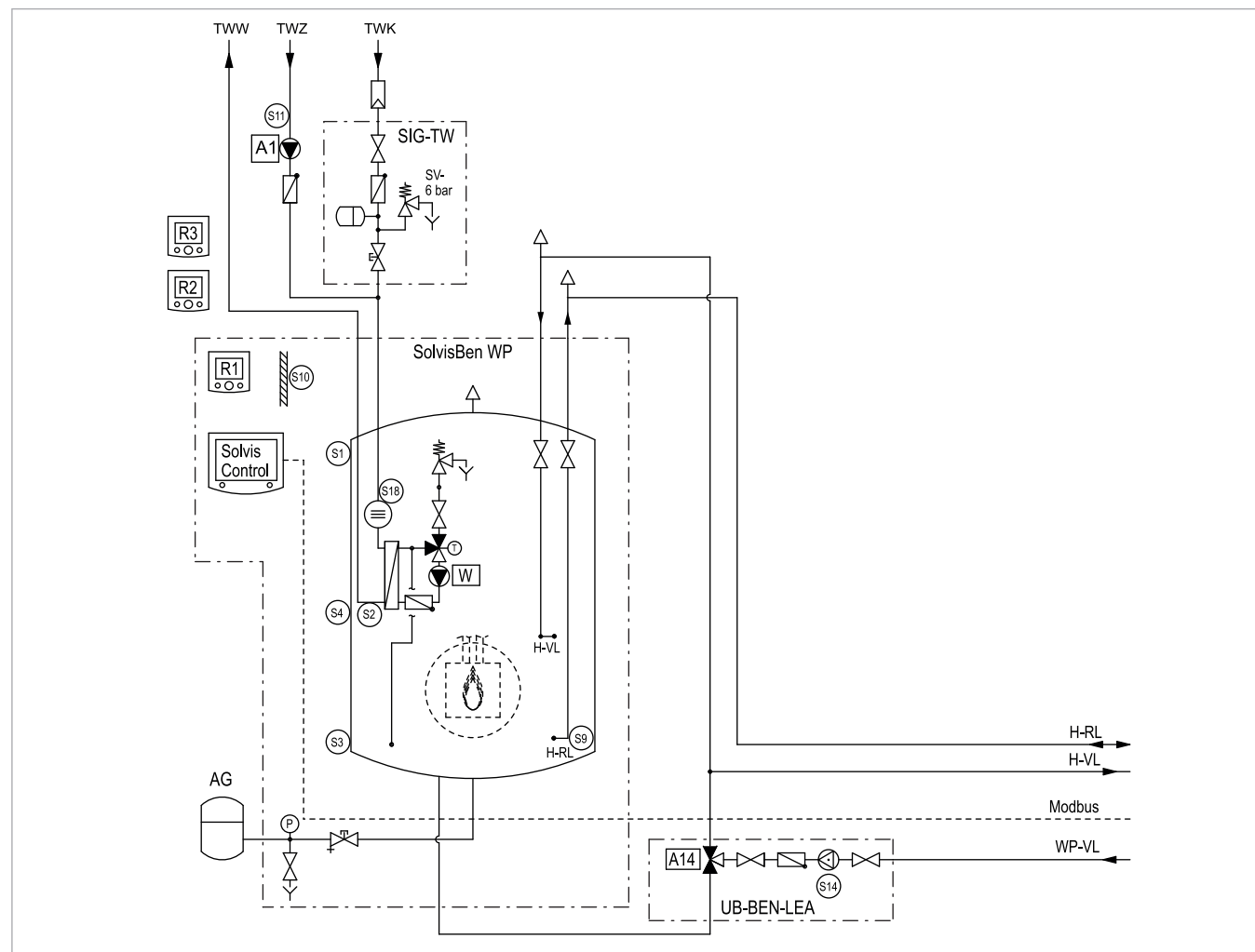
Fig. 19: SolvisBen WP tre circuiti di riscaldamento misti e pompa di calore SolvisLea - Parte 1
