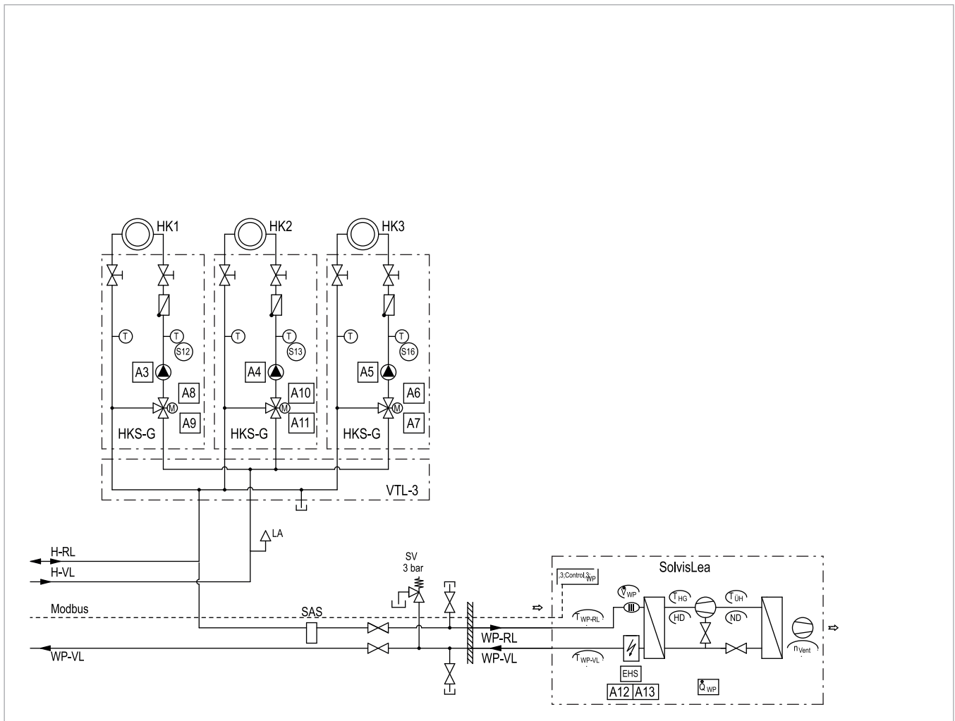
Fig. 20: SolvisBen WP 3 stazione circuito di riscaldamento misto e pompa di calore SolvisLea - Parte 2
