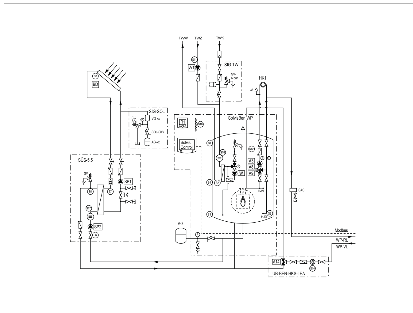
Afb. 17: SolvisBen WP met geïntegreerd verwarmingsgroepsstation, zonne-energiesysteem en warmtepomp SolvisLea - deel 1
