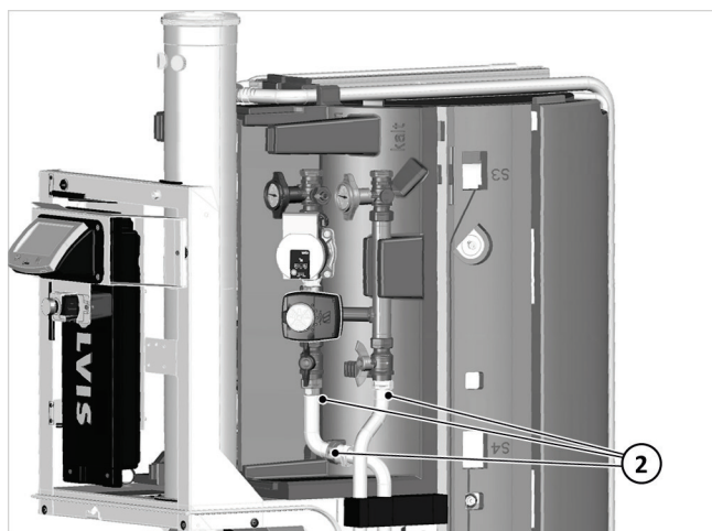
Afb. 5: Stukken leiding (2) verwijderen
