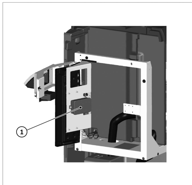
Afb. 13: Achterpaneel van de M&R-groep
