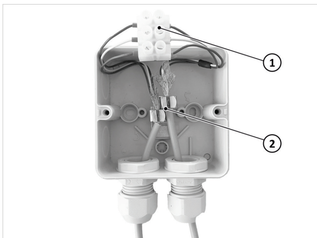
Afb. 12: Modbus-verbindingsdoos bevestigen
