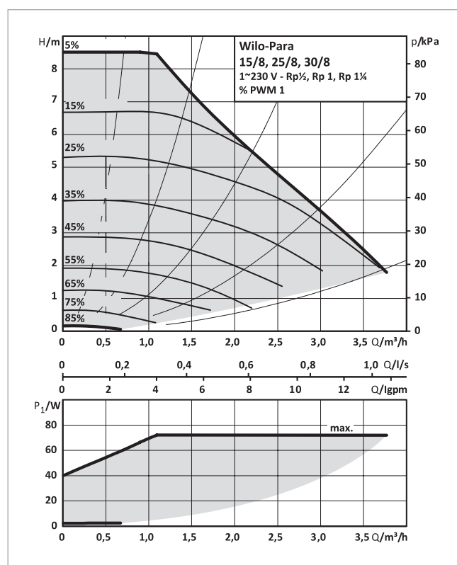
Afb. 16: Pompkarakteristieken Wilo PARA 15/8
