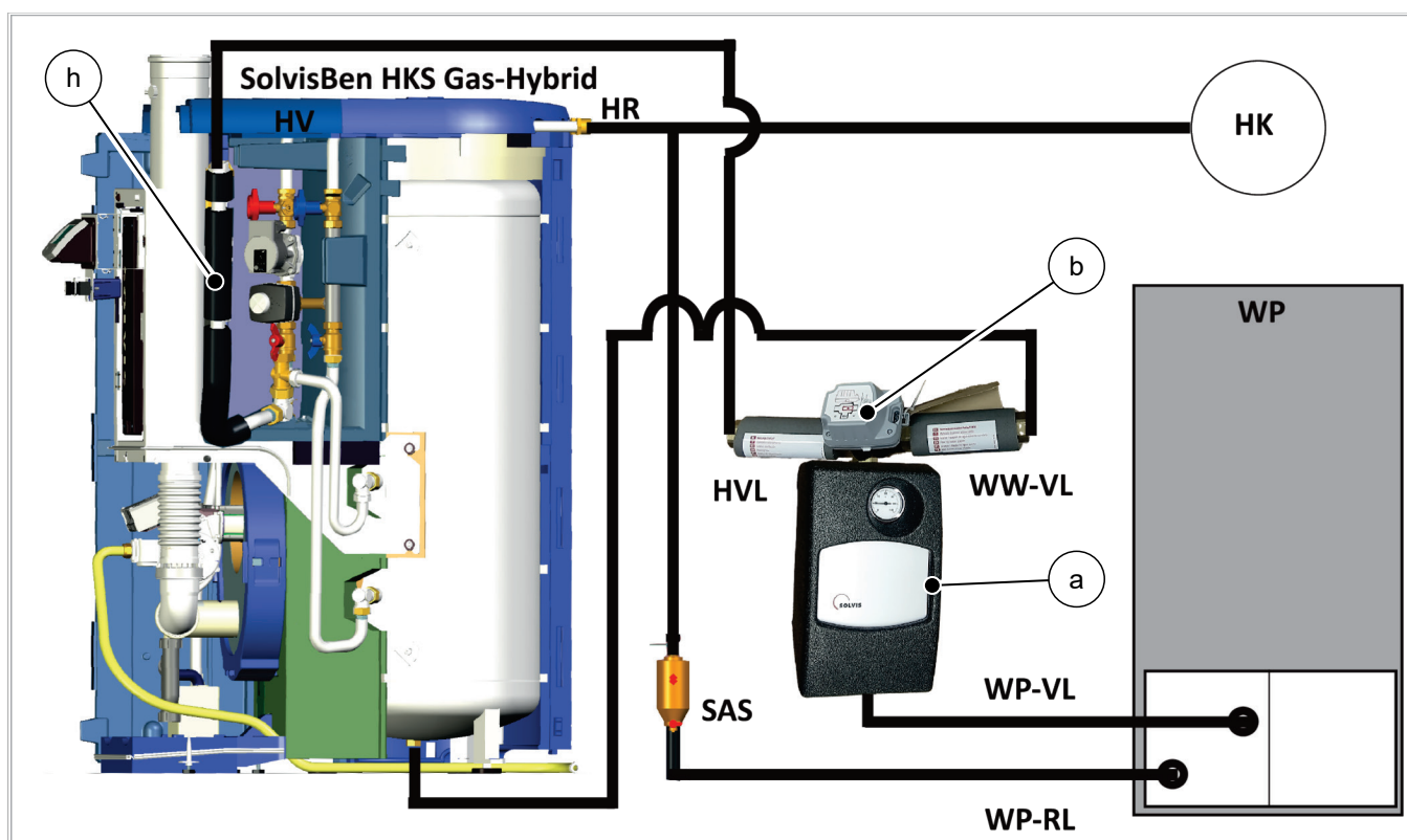
Afb. 9: Overzicht aansluiting SolvisLea aan SolvisBen HKS Gas-hybride
