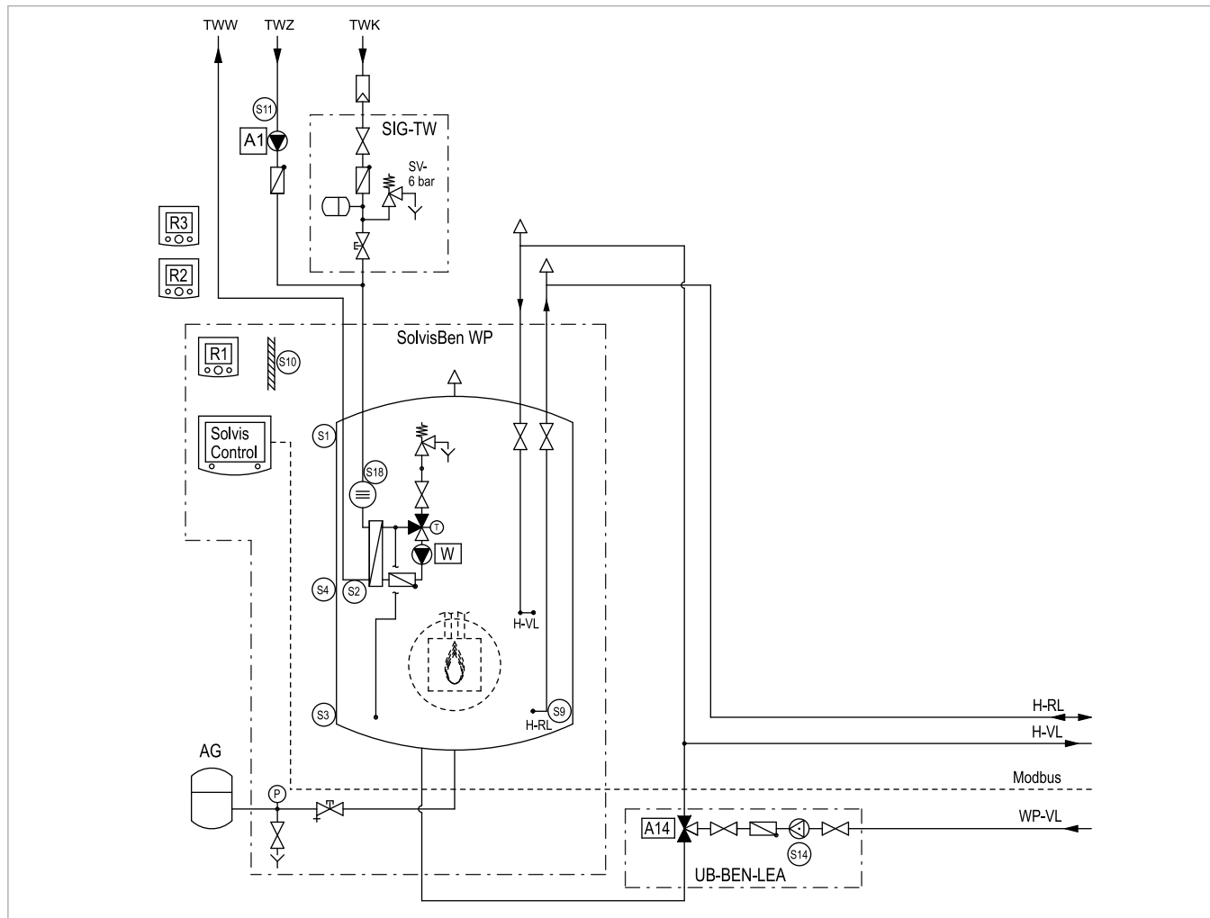
Afb. 19: SolvisBen WP drie met gemengde verwarmingsgroepen en warmtepomp - deel 1
