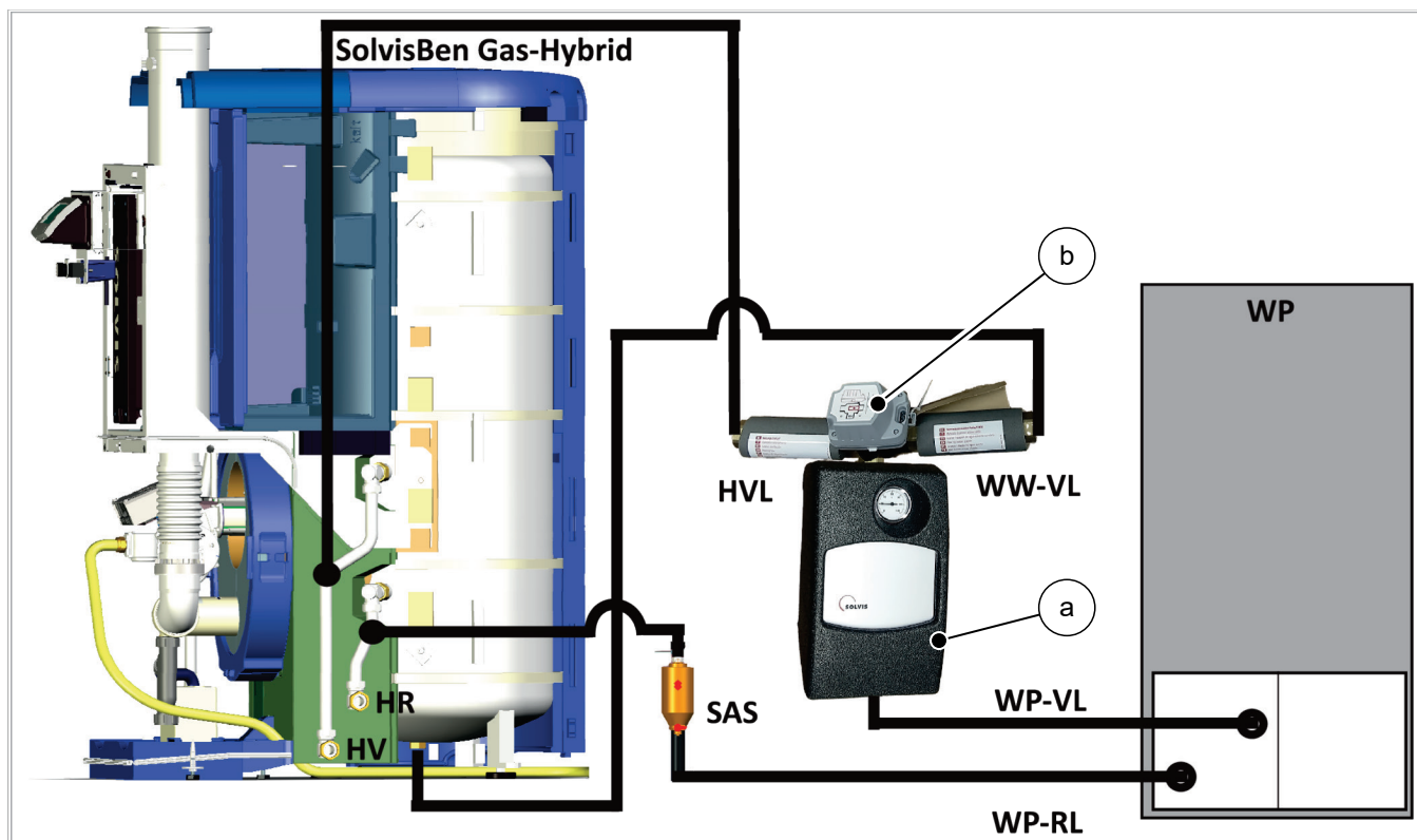
Afb. 8: Overzicht aansluiting SolvisLea aan SolvisBen GAS-hybride, zonder geïntegreerde verwarmingscircuitstation (HKS)
