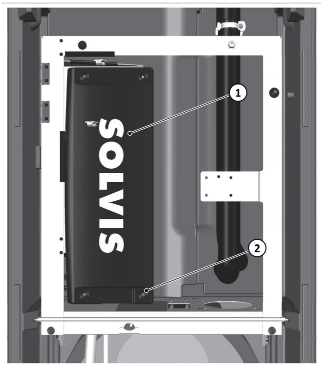
Afb. 14: Deksel van de netwerkkaart bevestigen
