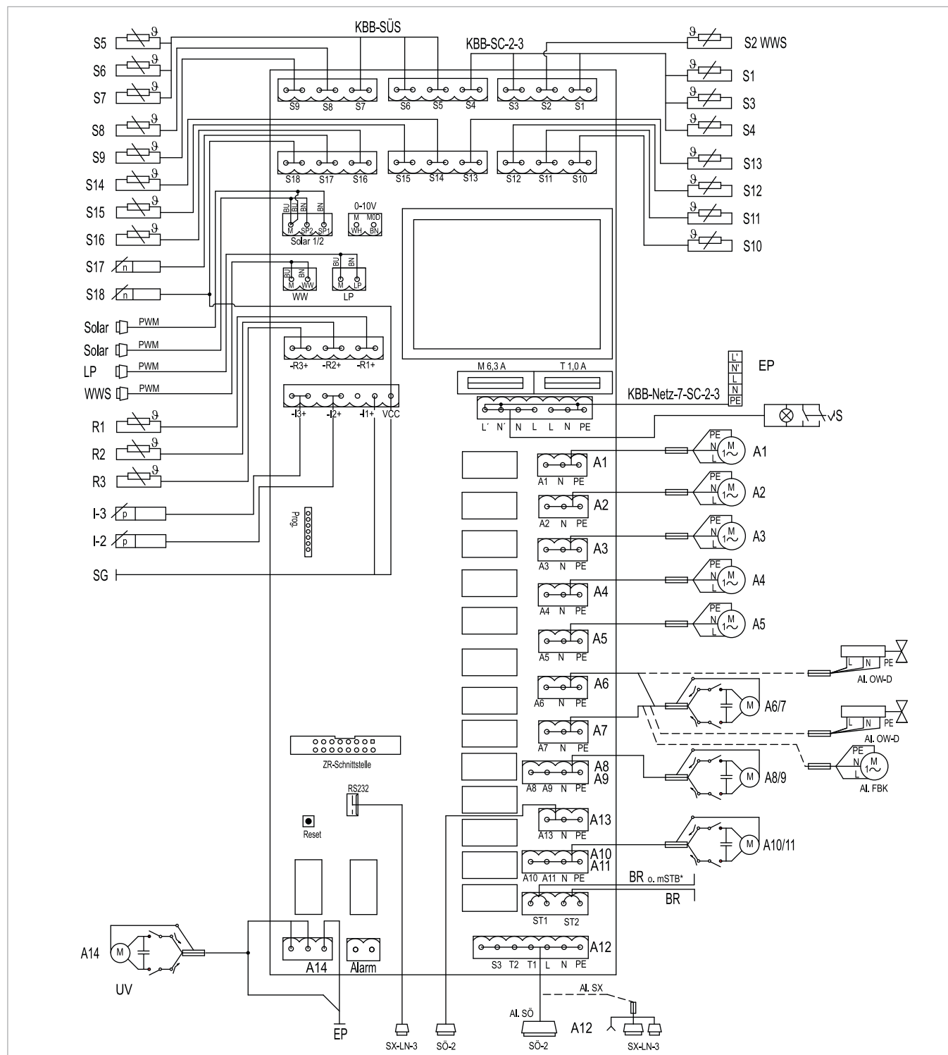
Afb. 22: Netwerkkkaart SolvisControl 3 voor SolvisBen Gas-/Olie-Hybrid
