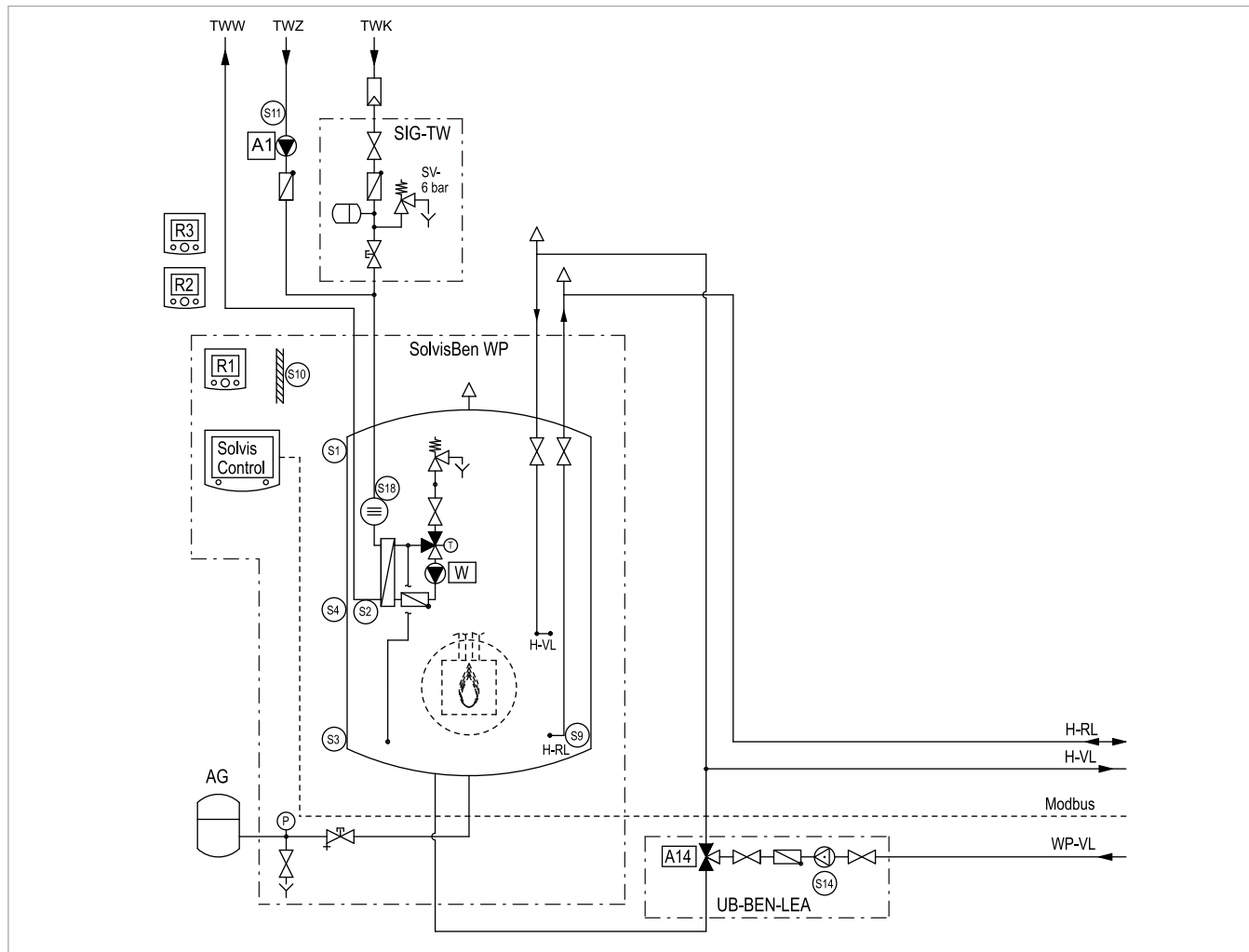
Afb. 19: SolvisBen WP drie met gemengde verwarmingsgroepen en warmtepomp - deel 1
