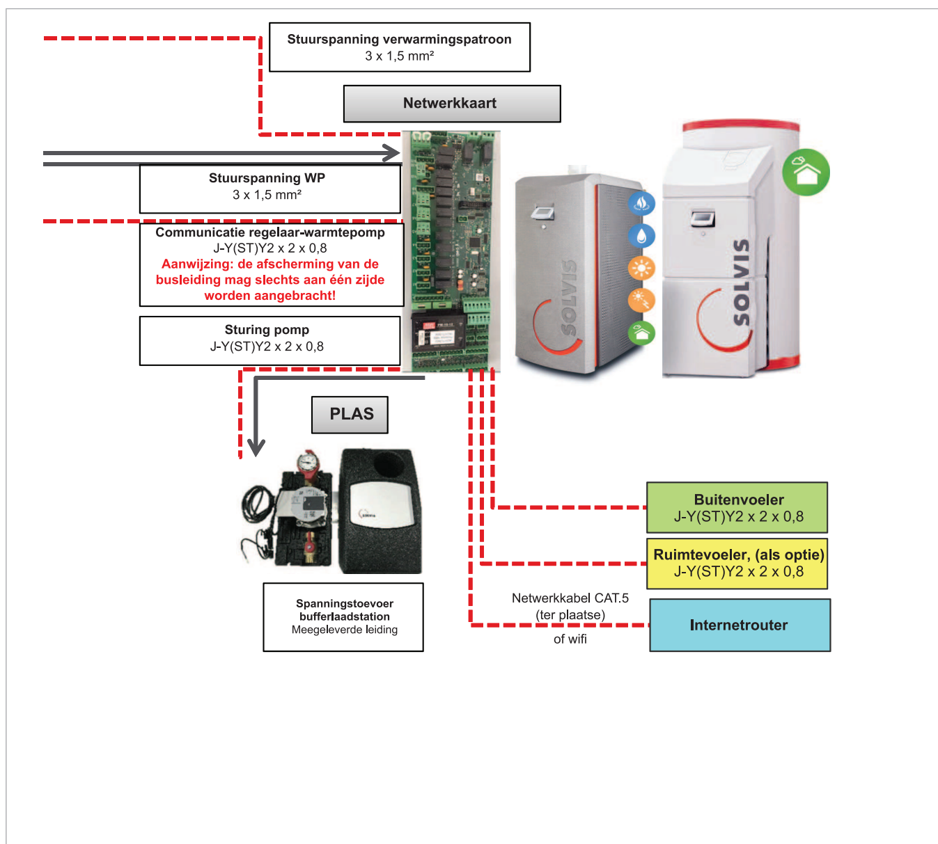
Afb. 4: Montagehulp SolvisBen/SolvisMax WP HPT met SolvisLea Eco 8 kW en EVU-verbinding - Deel 2
