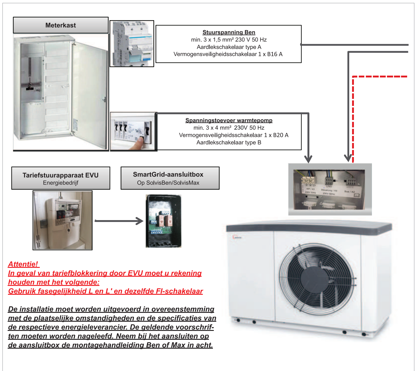
Afb. 1: Montagehulp SolvisBen/SolvisMax Hybrid met SolvisLea Eco 8 kW en EVU-verbinding - Deel 1
