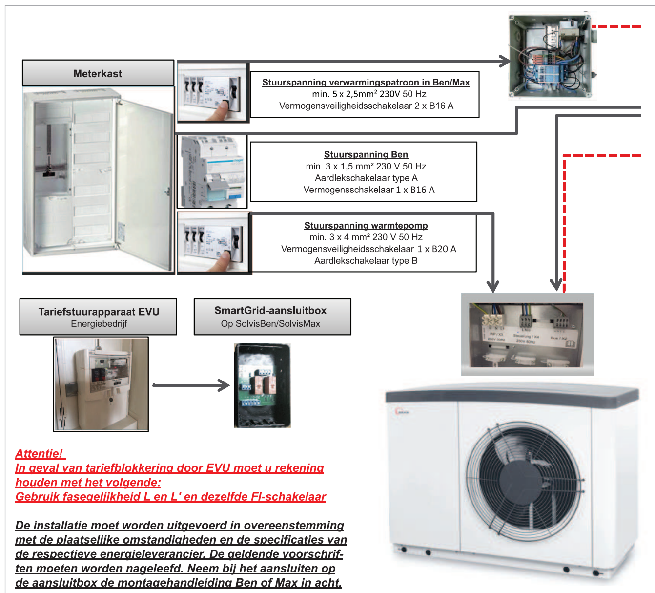
Afb. 3: Montagehulp SolvisBen/SolvisMax WP HPT met SolvisLea Eco 8 kW en EVU-verbinding - Deel 1
