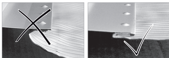
Fig. 44: Errato (sinistra), corretto (destra)
