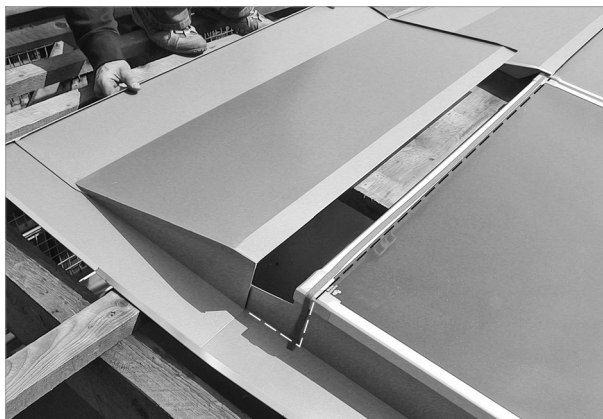
Fig. 80: applicare la lamiera superiore sulla lamiera laterale e spingerla contro il collettore
