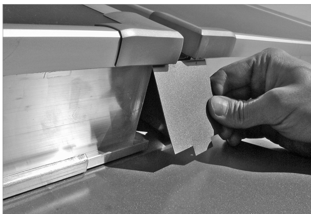
Fig. 89: applicare le piccole lamiere davanti alle intercapedini dei collettori
