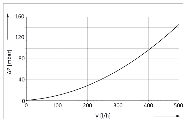
Fig. 98: curva della perdita di pressione SolvisCala C-254-C
