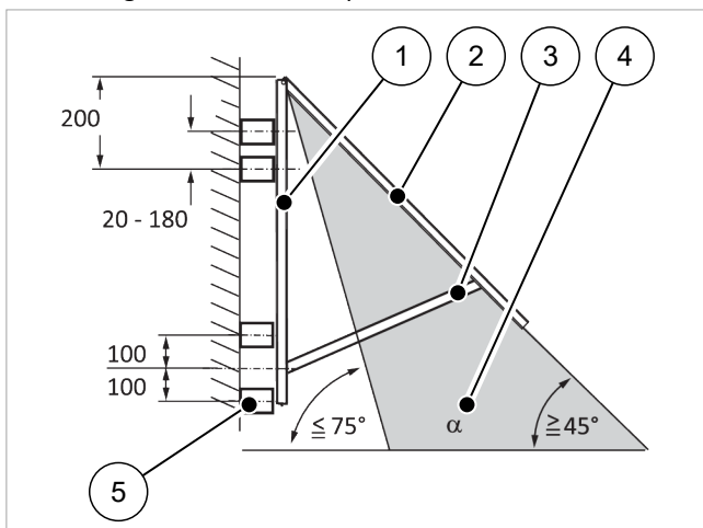
Fig. 32: montaggio dei supporti sulla parete
