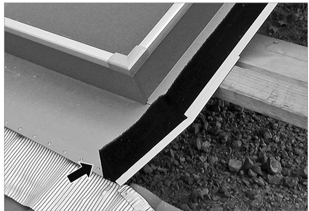
Fig. 86: cuneo antineve incollato
