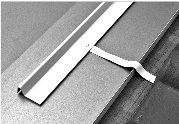
Fig. 84: applicare il sollevamento per le tegole e piegare le strisce di lamiera
