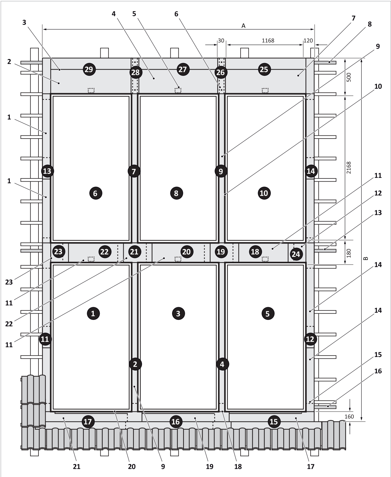
Fig. 43: dimensioni del campo del collettore a incasso con sei SolvisCala (quote in mm, le dimensioni del collettore sono misurate alla base)
