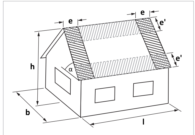
Fig. 41: Aree perimetrali del tetto
