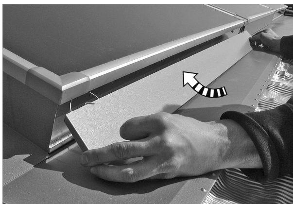
Fig. 90: applicare le lamiere di copertura lunghe davanti al lato frontale dei collettori
