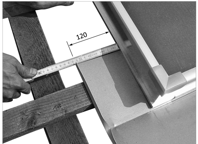
Fig. 50: applicare il primo collettore a sinistra e stabilire la distanza laterale
