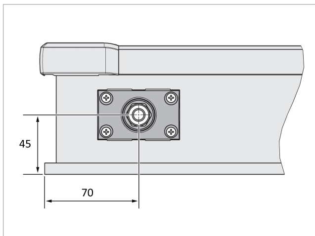
Abb. 97: position dell'allacciamento SolvisCala C-254-C
