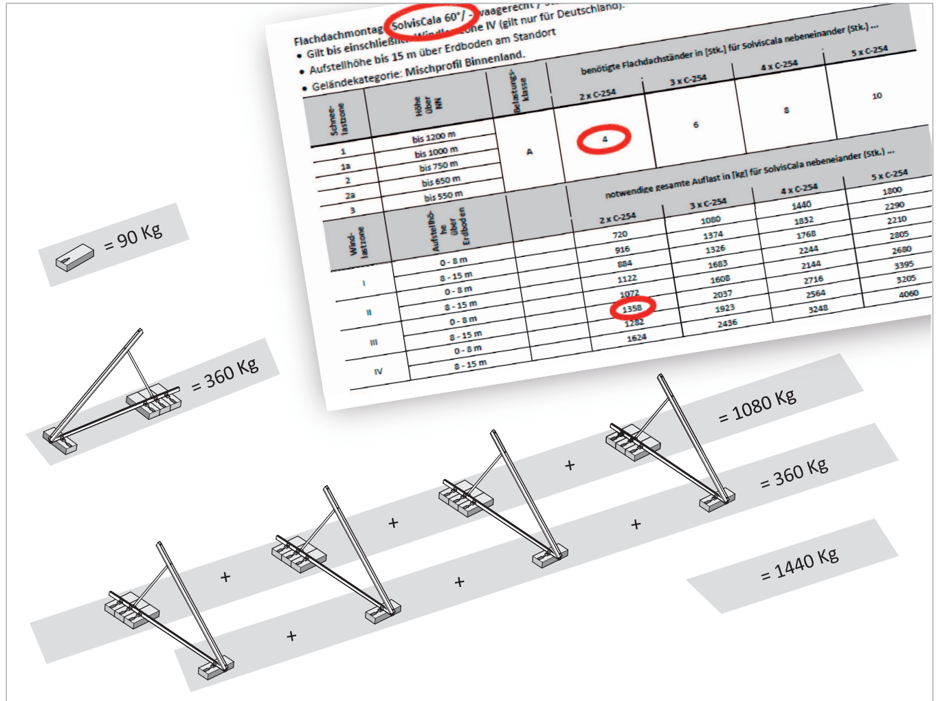
Fig. 27: esempio di distribuzione del carico
