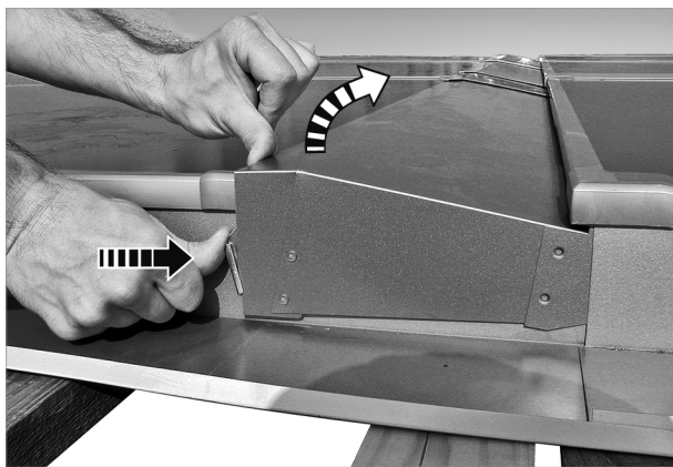
Fig. 78: ...quindi premere contro la leva e ribaltare la lamiera intermedia
