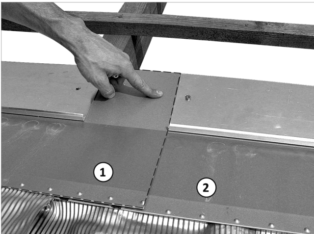
Fig. 48: montaggio, allineamento e serraggio della lamiera successiva da sinistra
