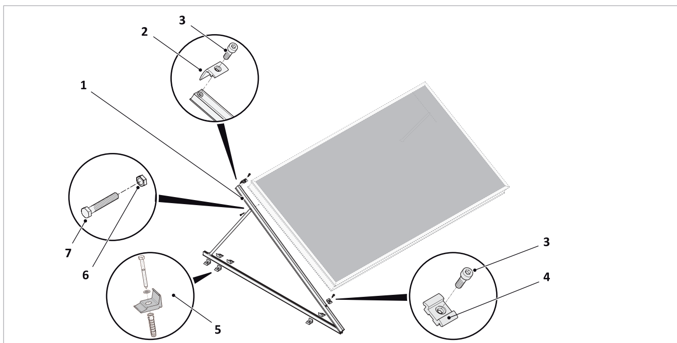
Abb. 24: Kit supporti per tetto piano per SolvisCala montaggio orizzontale (collettore non compreso nella fornitura)
