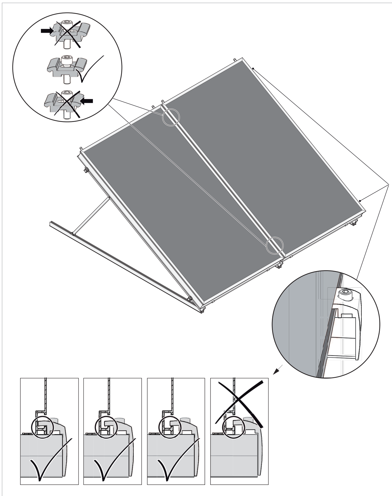
Fig. 40: fissaggio dei dispositivi di bloccaggio dei bordi e centrali
