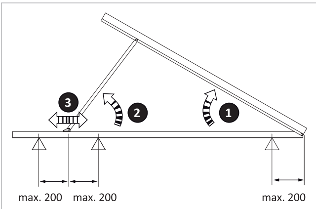
Fig. 30: schema del supporto per tetto piano
