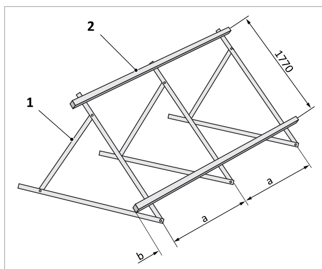
Fig. 28: dimensioni delle distanze supporti per tetto piano
