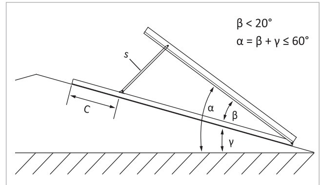
Fig. 31: angolo sulle superfici leggermente inclinate
