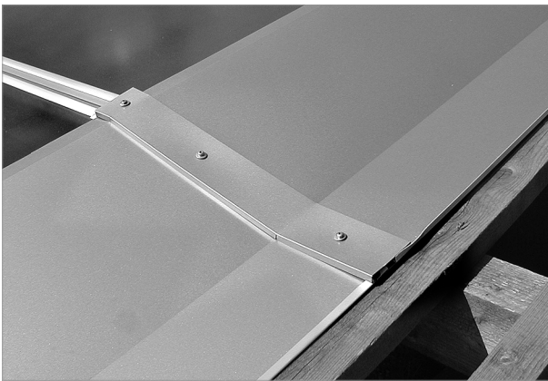
Fig. 83: avvitare la lamiera superiore con quella inferiore
