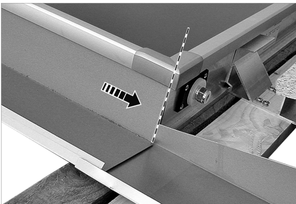
Fig. 66: spingere la lamiera laterale inferiore fino al bordo inferiore del telaio del collettore
