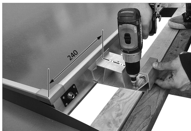
Fig. 61: avvitare i distanziali dei collettori, a sinistra e a destra, con la distanza rispetto al bordo esterno
