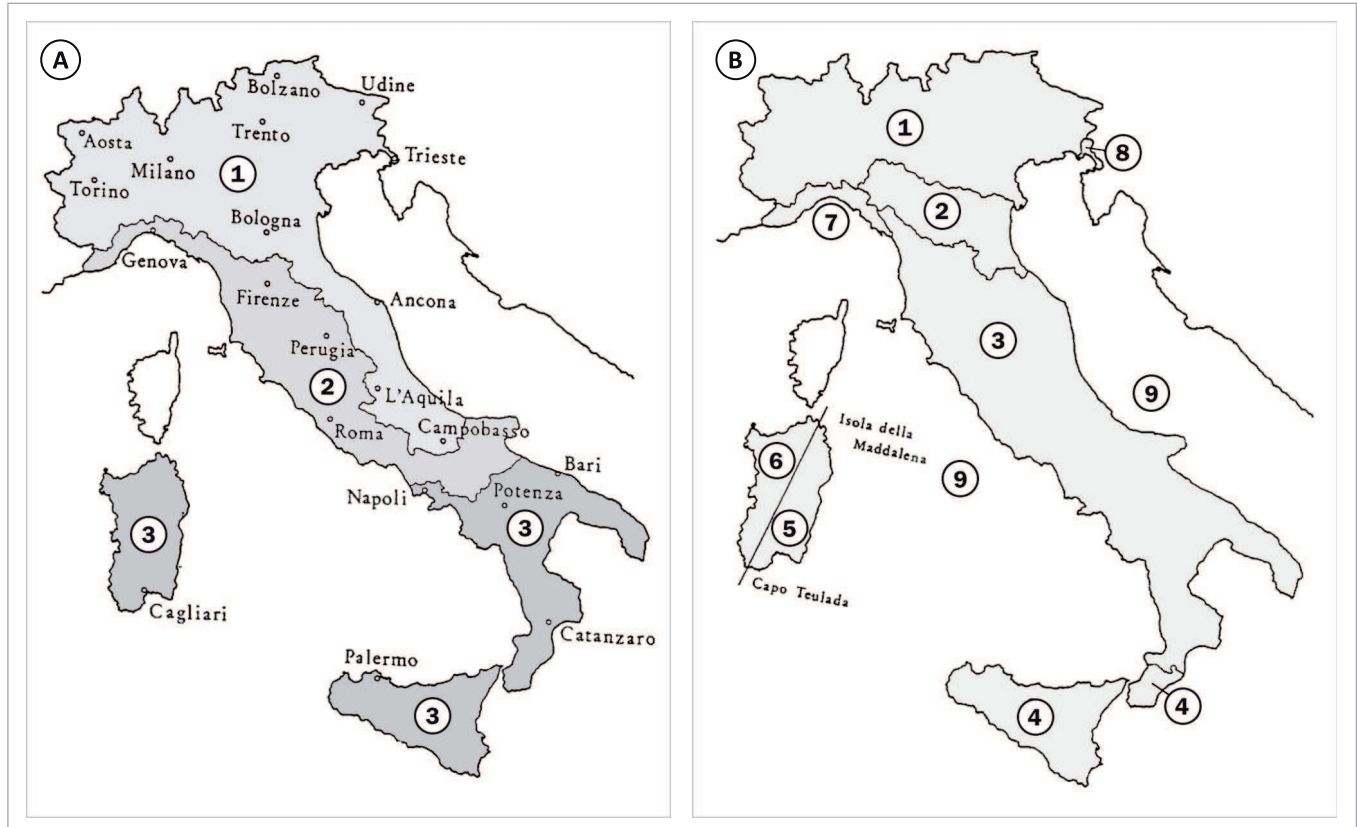
Fig. 100: distribuzione delle zone di carico di neve e di vento in Italia
