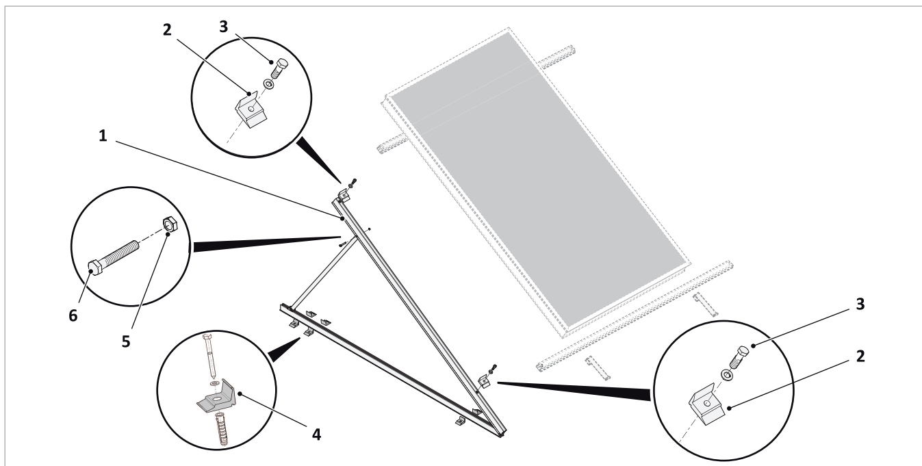
Fig. 23: Kit di montaggio su tetto piano per SolvisCala, montaggio sul bordo (collettore e traverse non compresi nella fornitura).
