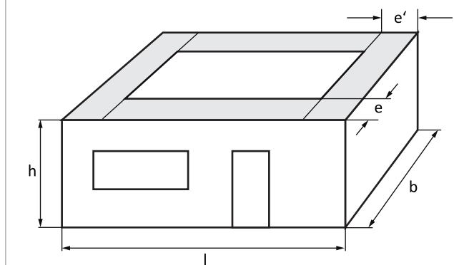
Fig. 25: distanze minime dallo spigolo dell'edificio
