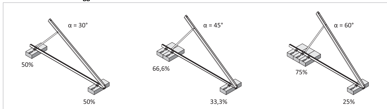
Fig. 26: distribuzione del carico aggiuntivo con angolo di inclinazione \alpha = 30^\circ / 45^\circ / 60^\circ
