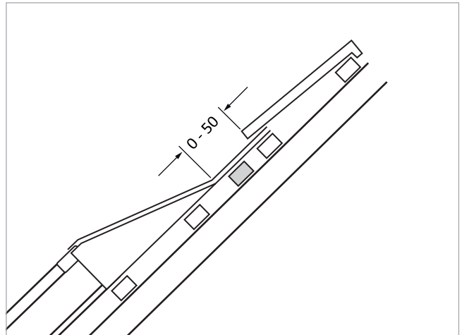
Fig. 85: copertura superiore (vista laterale)
