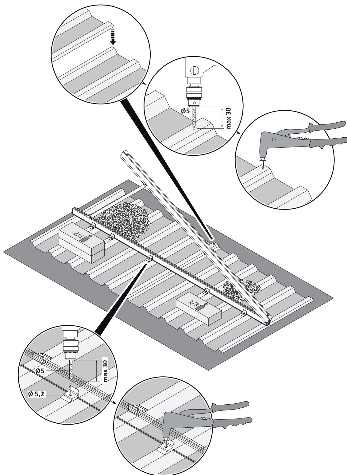
Fig. 38: montaggio del supporto per tetto piano su lamiera trapezoidale
