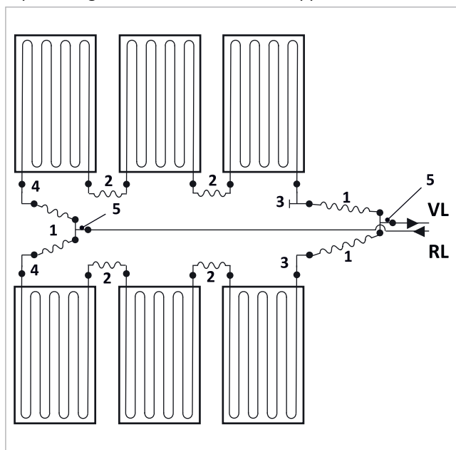
Fig. 14: SolvisCala 254 Eco, collegamento in parallelo sovrapposto
