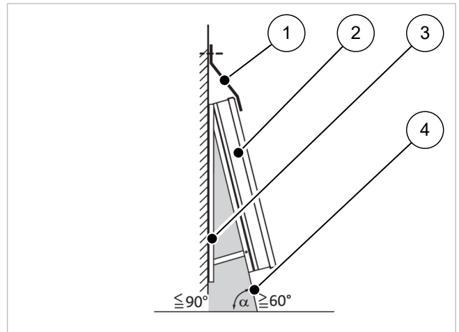
Fig. 33: Collettore con lamiera di copertura
