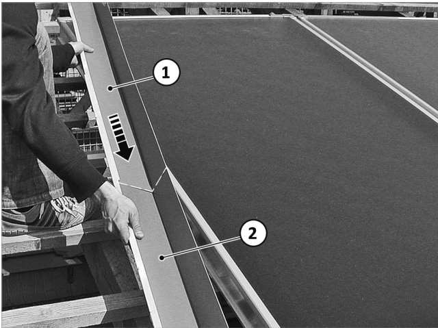
Fig. 55: spinta della parte della lamiera laterale superiore sopra la parte della lamiera laterale inferiore
