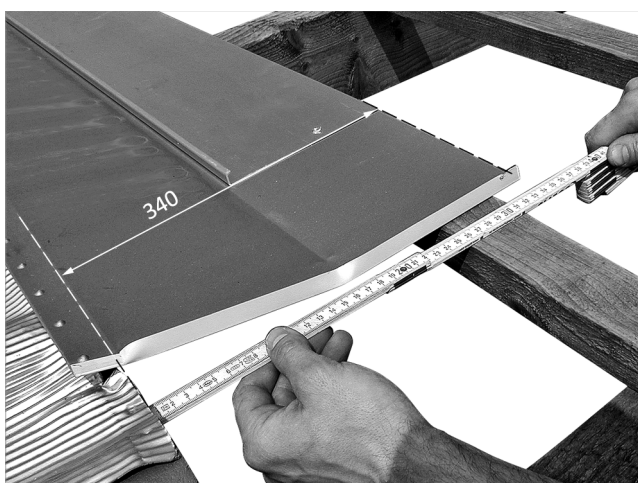
Fig. 46: determinare la posizione della lamiera del grembiule di piombo
