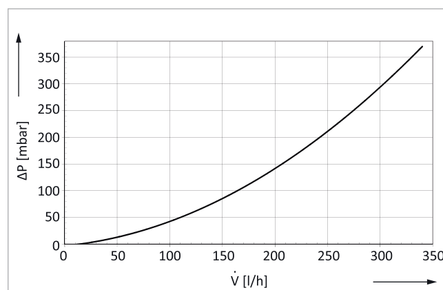
Fig. 99: Curva perdita di pressione SolvisCala C-254-E
