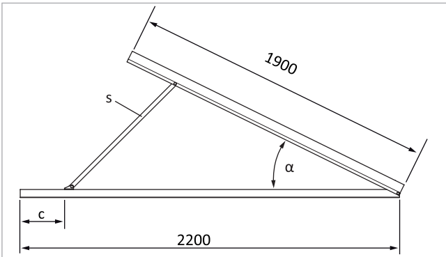
Fig. 29: supporti per tetto piano, dimensioni e angolo di inclinazione
