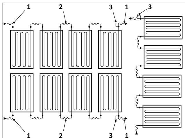
Fig. 13: SolvisCala 254 Eco, collegamento in serie affiancato e sovrapposto
