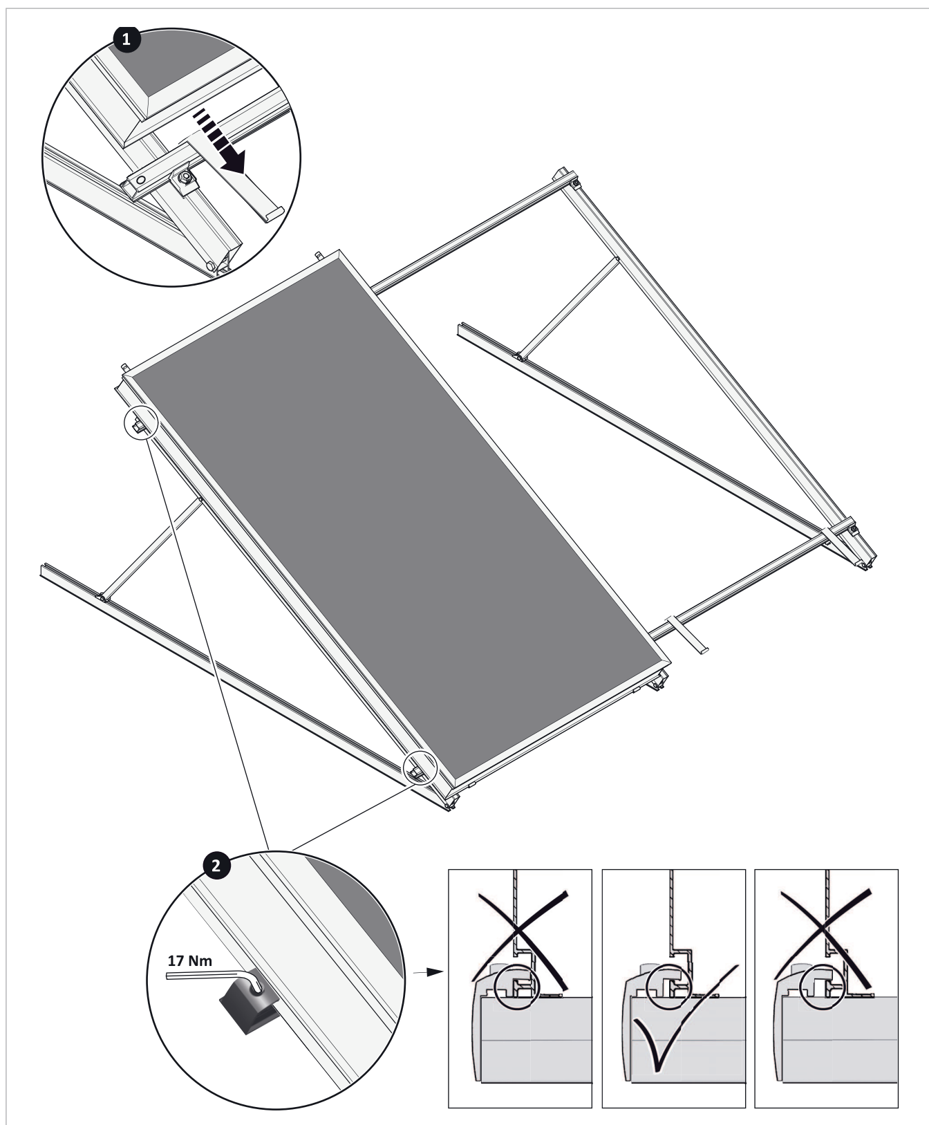
Fig. 39: fissaggio di un collettore ai supporti per tetto piano
