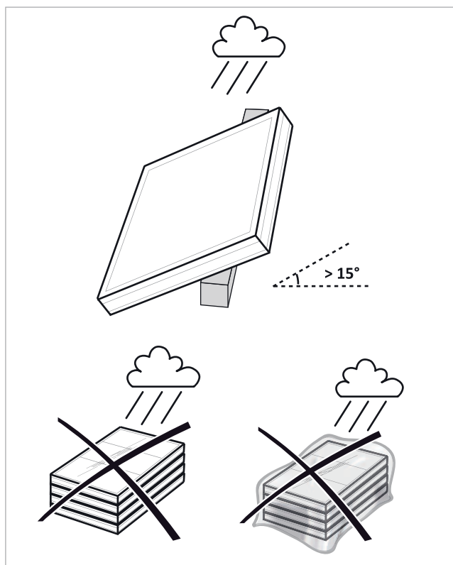
Fig. 1: Stoccaggio di SolvisCala all'aperto
