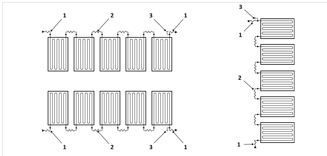
Fig. 10: SolvisCala 254 Control, collegamento in serie affiancato e sovrapposto
