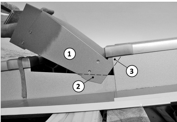
Fig. 76: inserire, applicare e premere la lamiera intermedia-angolo nella scanalatura
