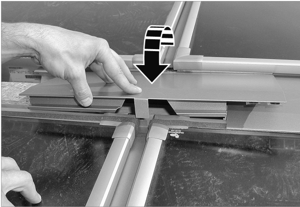
Fig. 74: inserimento, applicazione e pressione della lamiera a incrocio nella scanalatura
