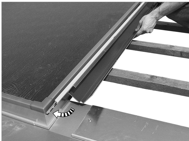
Fig. 52: inserire la lamiera di giunzione
