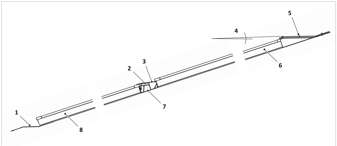
Fig. 42: sezione attraverso un campo collettori con due file
