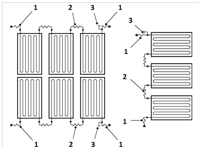
Fig. 12: SolvisCala 254 Eco, collegamento in serie affiancato e sovrapposto
