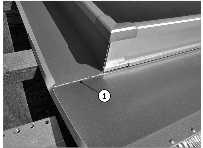
Fig. 58: spinta della lamiera inferiore laterale verso il basso fino alla piega
