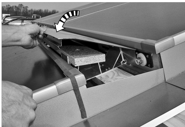
Fig. 70: inserire, applicare e premere la prima lamiera intermedia nella scanalatura
