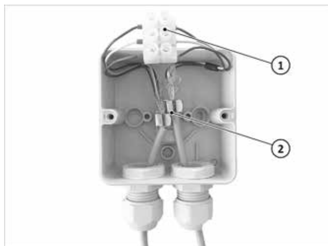
Abb. 18: Modbus-Verbindungsdose befestigen
