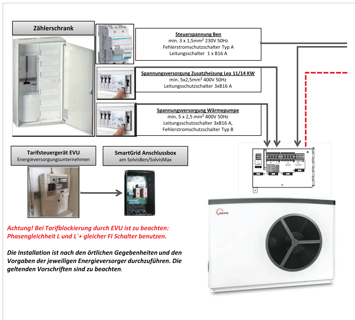
Abb. 1: Montagehilfe SolvisBen WP mit SolvisLea 11/14 kW und EVU-Anbindung - Teil 1
