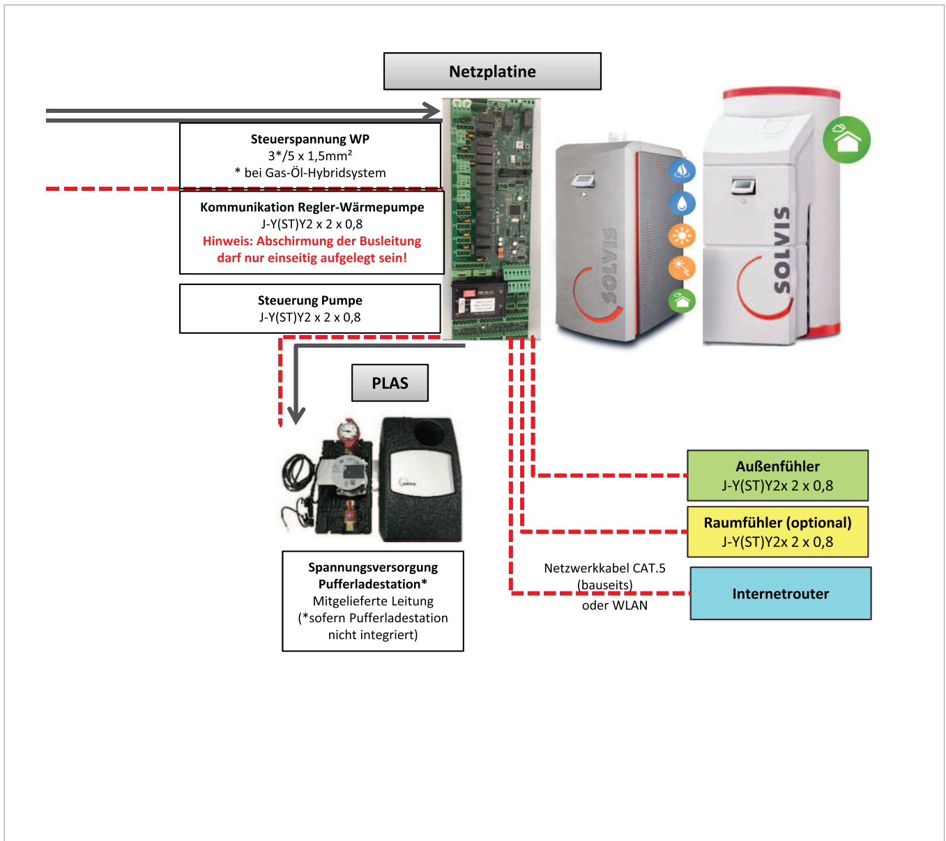
Abb. 2: Montagehilfe SolvisBen WP mit SolvisLea 11/14 kW und EVU-Anbindung - Teil 2
