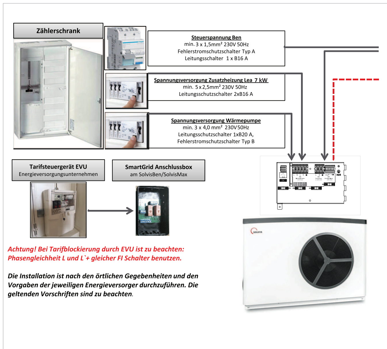
Abb. 3: Montagehilfe SolvisBen WP mit SolvisLea 7 kW und EVU-Anbindung - Teil 1
