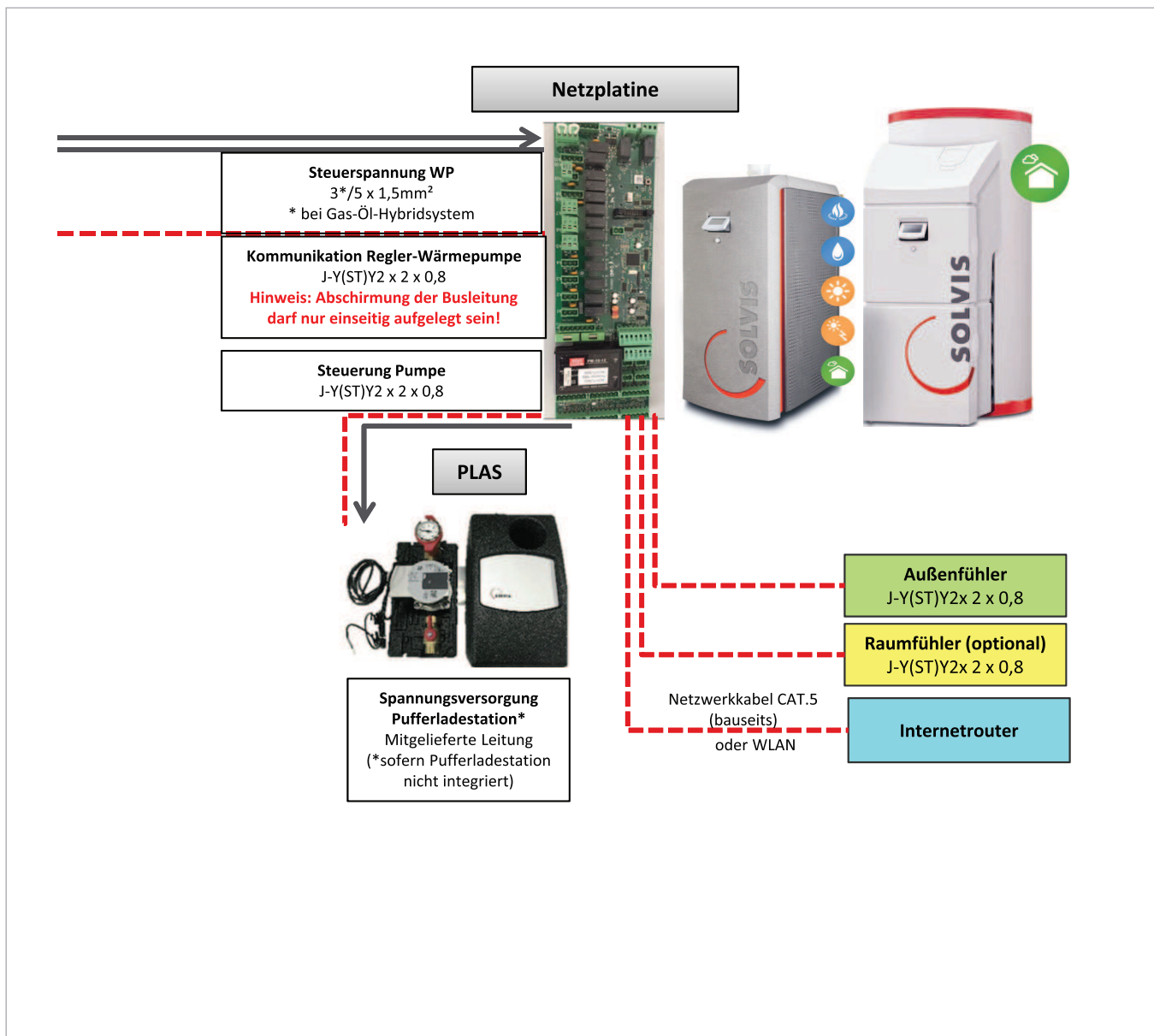
Abb. 4: Montagehilfe SolvisBen WP mit SolvisLea 7 kW und EVU-Anbindung - Teil 2
