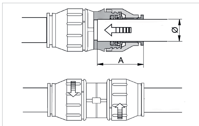
Fig. 8: Insertar y bloquear el tubo
