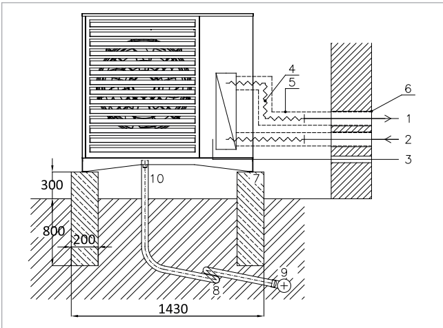
Fig. 6: SolvisMia montado en cimientos corridos
