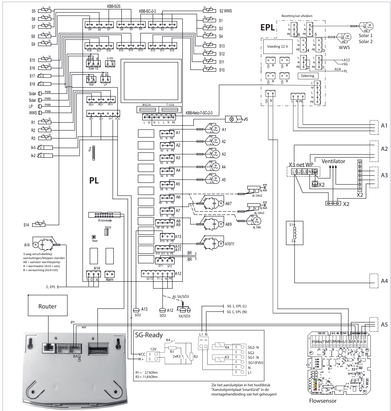
Afb. 23: Stroomingsschema SolvisMia 8 hybride systeem - deel 1
