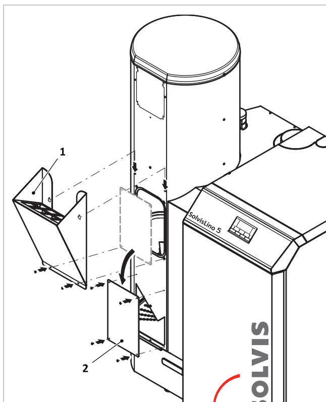
Abb. 179: Pelletschütte und Revisionsdeckel montieren
