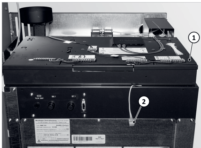
Abb. 41: Deckel vom Schaltfeld aufklappen
