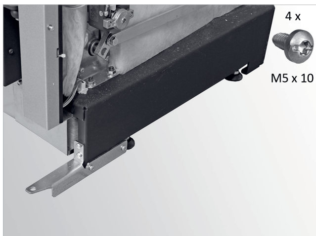
Abb. 84: Türscharnier unten anschrauben
