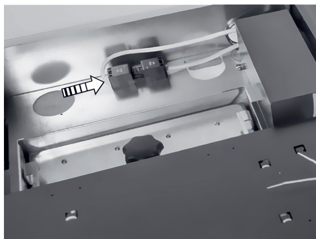
Abb. 121: Netzstecker einstecken
