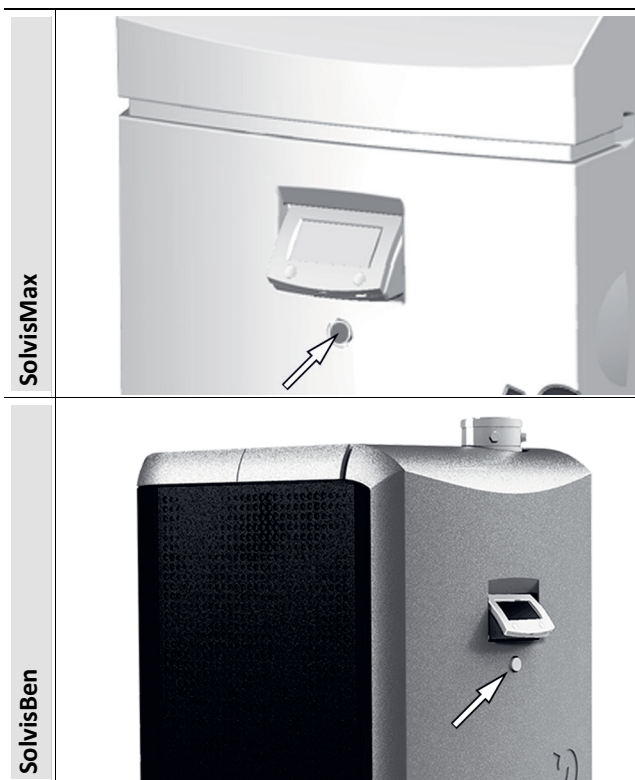
Abb. 120: Anlage einschalten
