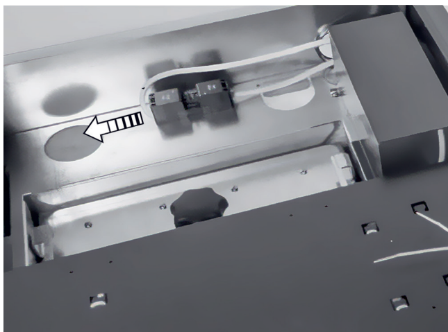
Abb. 132: Gerätenetzstecker ziehen
