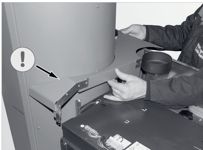
Abb. 46: Verkleidung vorsichtig auflegen
