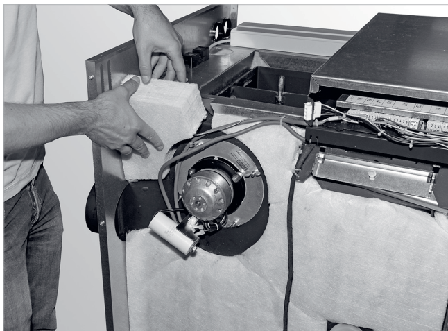
Abb. 25: Isolierung anbringen
