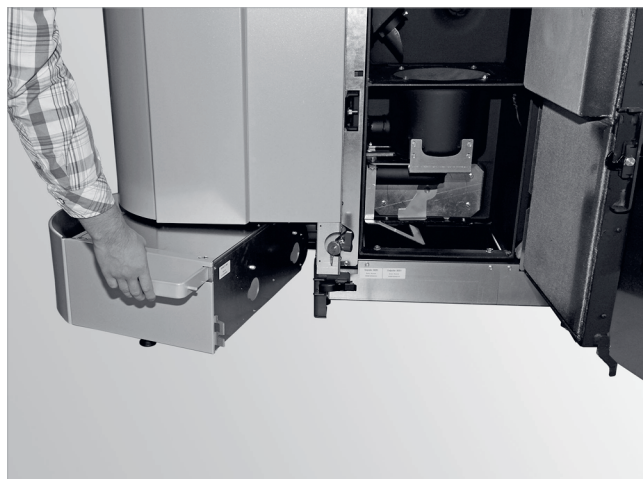
Abb. 101: Aschebehälter einschieben (LI-5-xx-GS)
