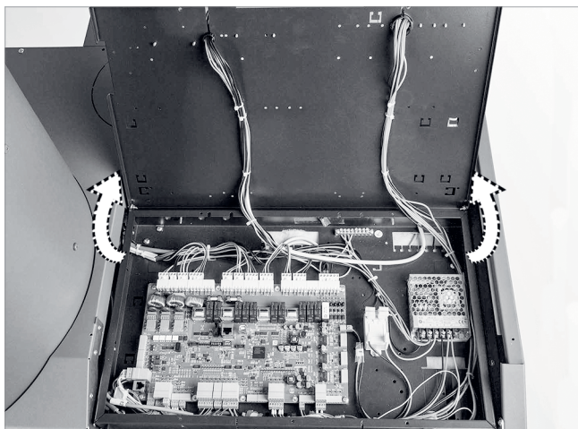
Abb. 111: Deckel nach oben klappen
