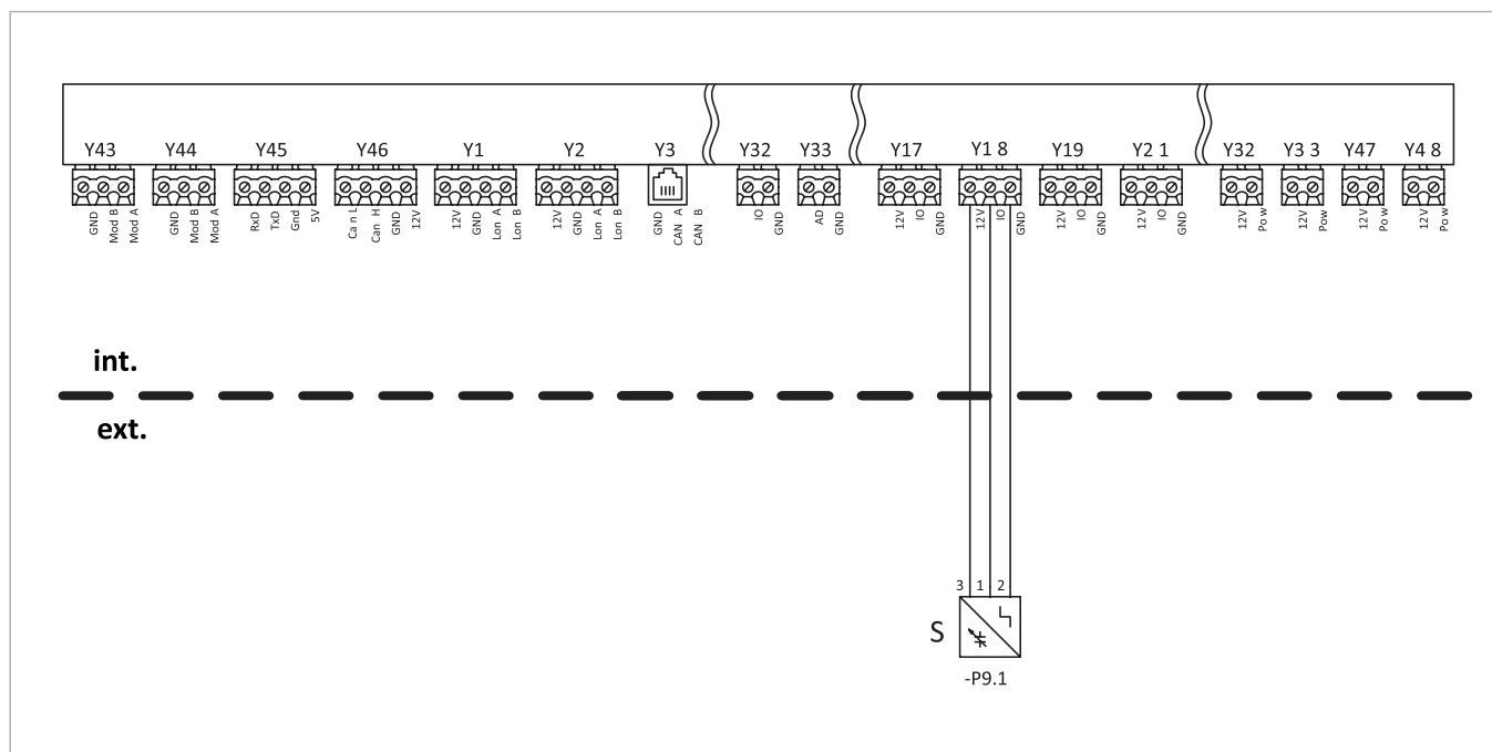
Abb. 198: Anschlussplan Absperreinheit
