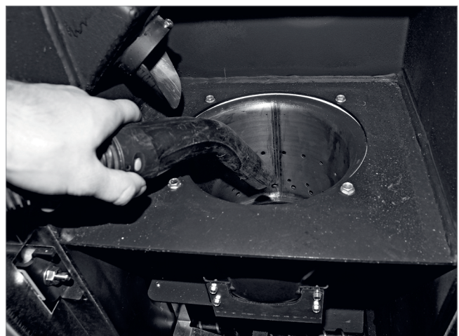
Abb. 150: Brennertopf aussaugen
