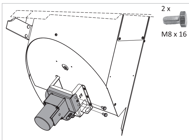
Abb. 63: Schneckenmotor anschrauben
