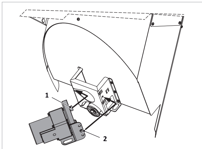
Abb. 62: Schneckenmotor einhängen
