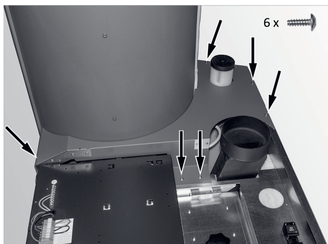
Abb. 47: Verkleidung befestigen
