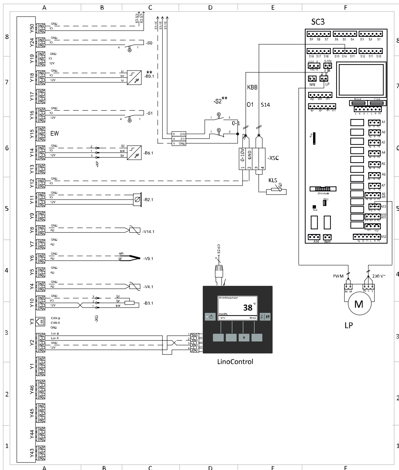
Abb. 192: Grundschaltbild SolvisLino 4 / SolvisLino 5 (Plan E2)
