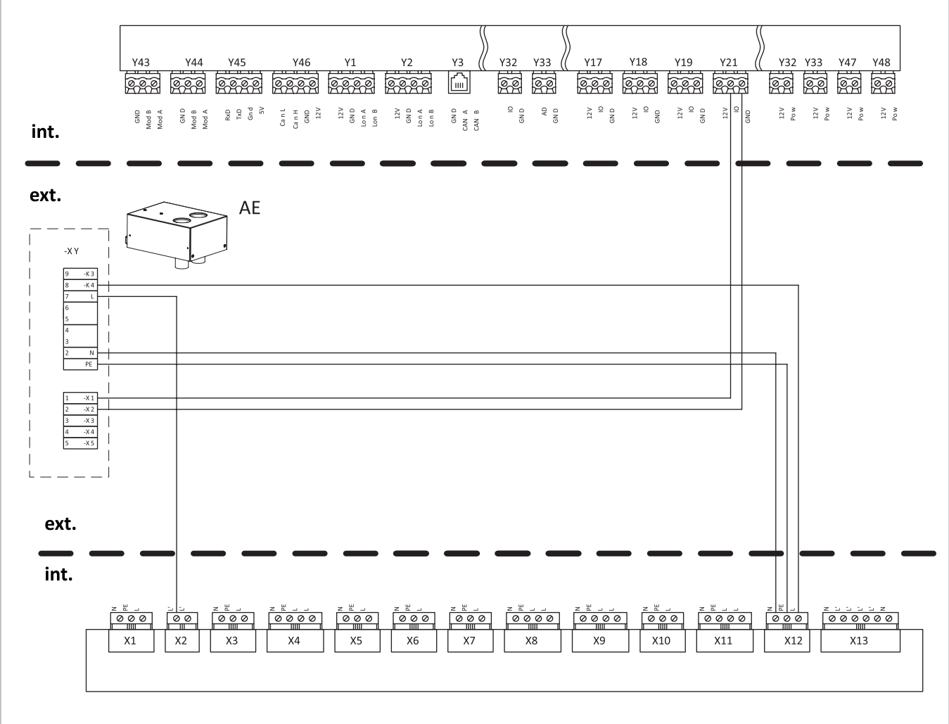
Abb. 197: Anschlussplan Absperreinheit
