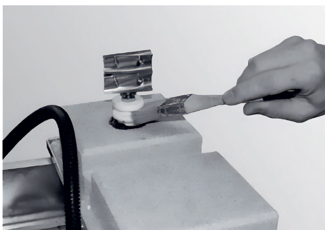
Abb. 162: Elektrode des Feinstaubabscheiders mit Pinsel reinigen
