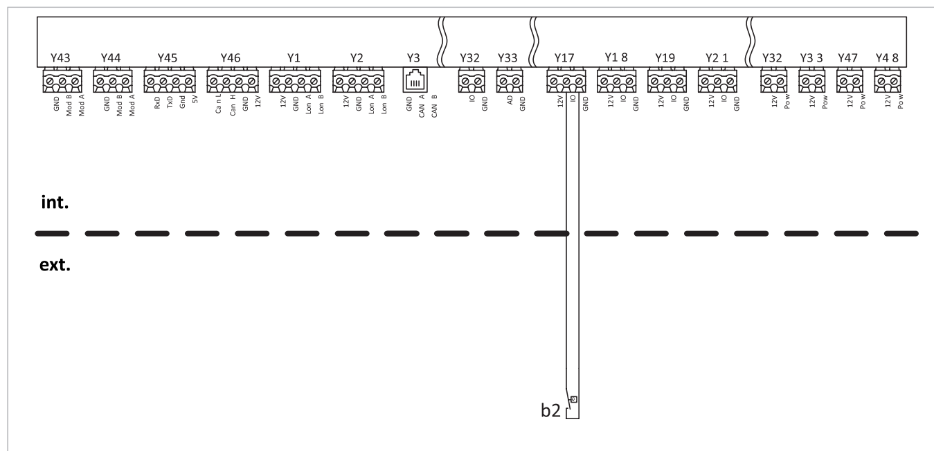
Abb. 200: Anschlussplan Rauchgasthermostat
