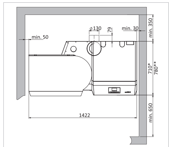
Abb. 190: Mindestabstand Rauchgasrohr hinten (Maße in mm)
