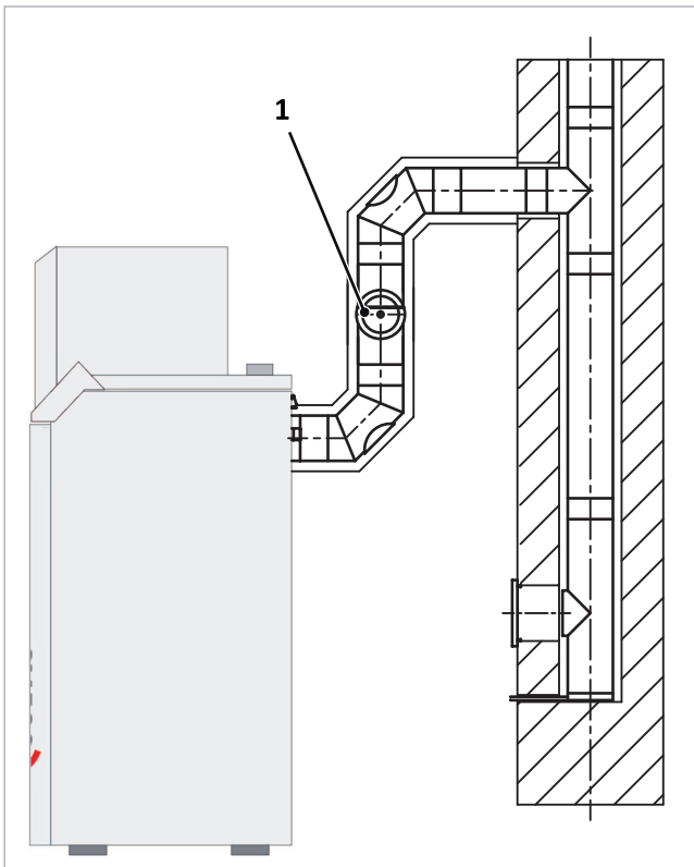
Abb. 1: SolvisLino mit Energiespar-Zugregler
