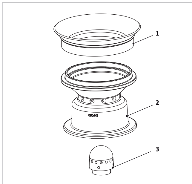
Abb. 155: Zusammenbau Brennertopf
