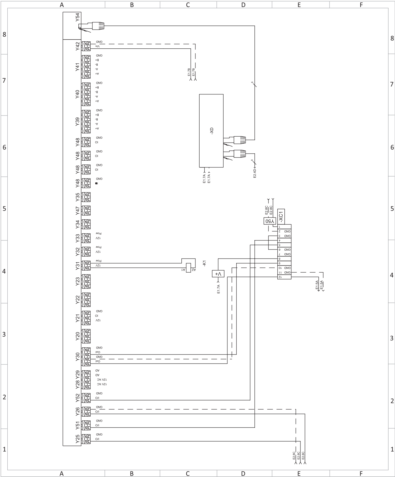
Abb. 193: Grundschriftbild SolvisLino 4 / SolvisLino 5 (PLan E3)
