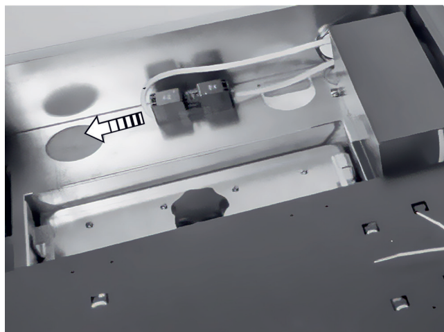
Abb. 172: Geräte-Netzstecker abziehen
