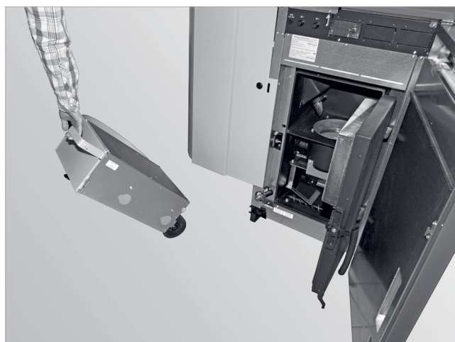
Abb. 173: Aschebehälter entfernen
