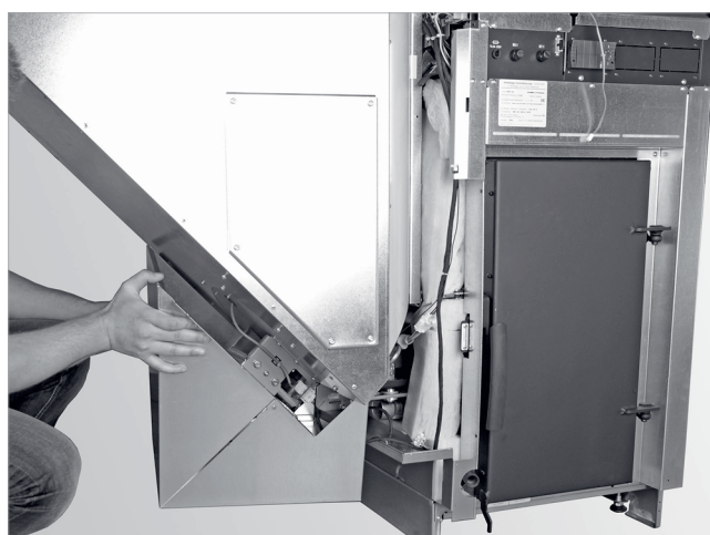
Abb. 66: Abdeckung einhängen
