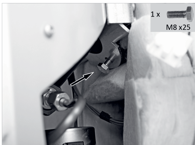
Abb. 31: Vorratsbehälter festschrauben
