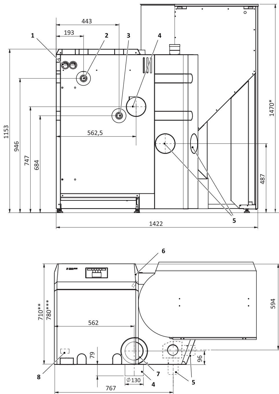
Abb. 186: Ansichten SolvisLino 5 mit Vorratsbehälter (LI-5-xx-VO)
