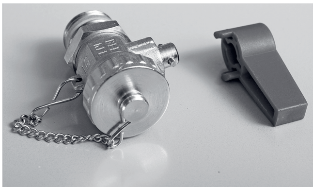
Abb. 26: Griff bei Füll- und Entleerhahn abziehen
