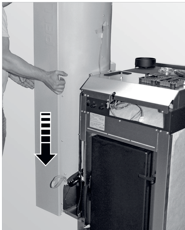
Abb. 33: Blende abnehmen
