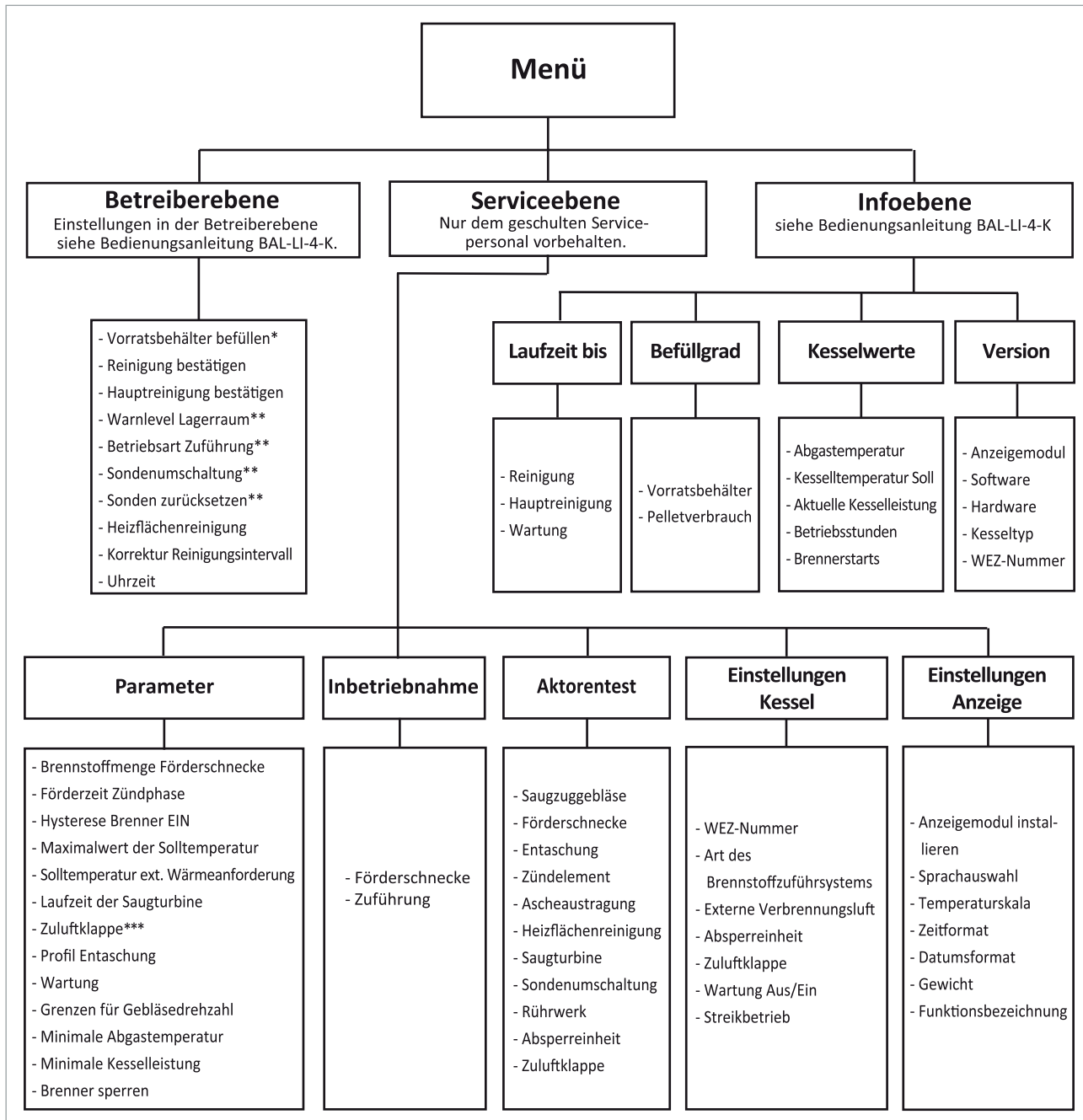
Abb. 118: Struktur in der Betreiber-, Service- und Infoebene
