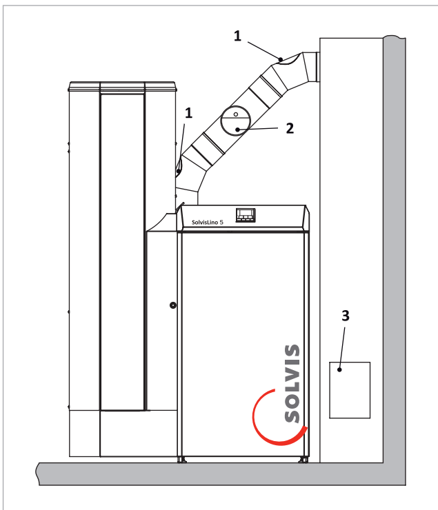
Abb. 168: Reinigungsöffnungen (Ansicht ohne Isolierung)
