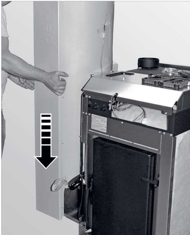
Abb. 175: Blende abnehmen (Bajonettverschluss)
