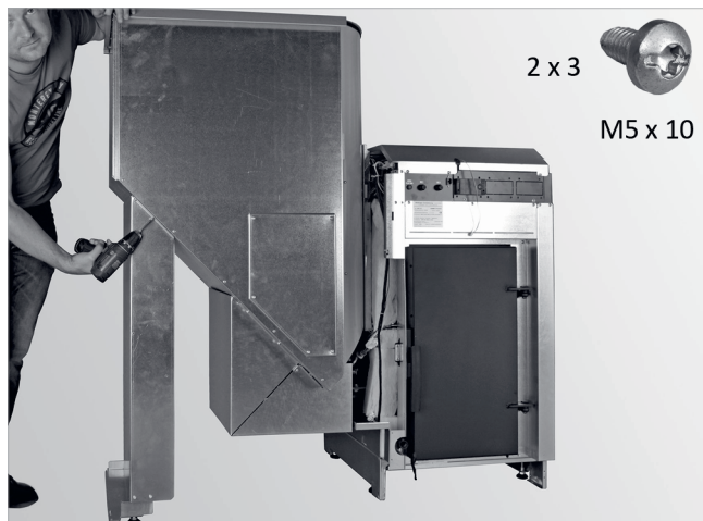
Abb. 68: Stellfuß anschrauben
