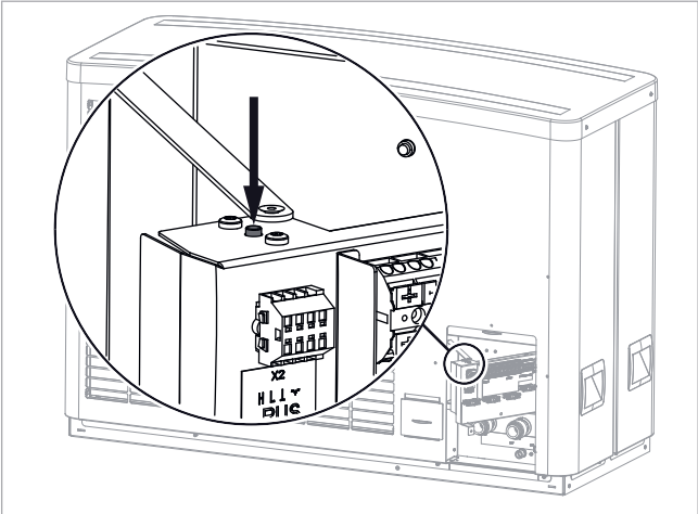
Fig. 30: Solvis Lea: Botón de reset de la calefacción adicional/de emergencia
