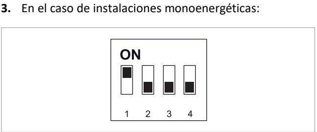
Fig. 33: interruptor deslizable de tipo BC en instalaciones monoenergéticas
