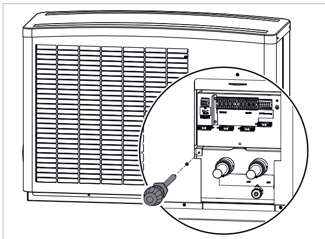
Fig. 23: Aflojar el tornillo del área de conexión
