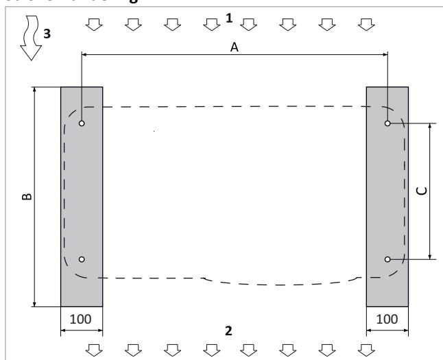
Afb. 11: Fundering voor standconsole SolvisLea (bovenaanzicht)
