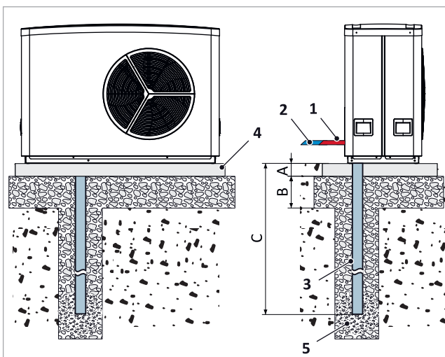
Afb. 6: Fundering voor SolvisLea
