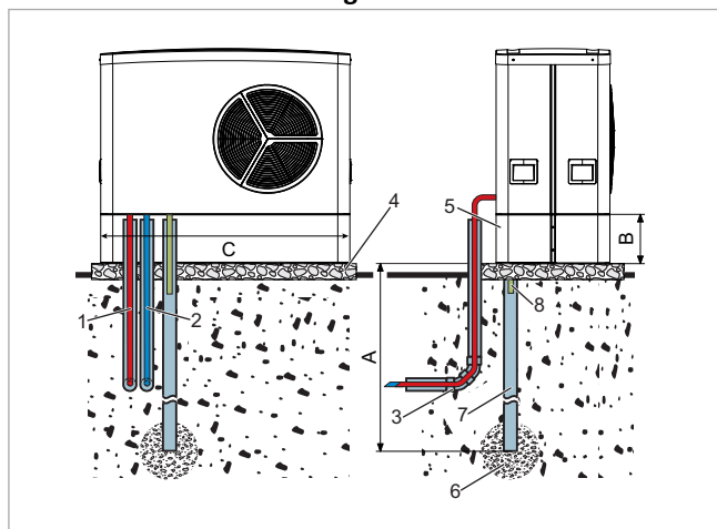
Afb. 10: Condensafvoer voor montageconsole
