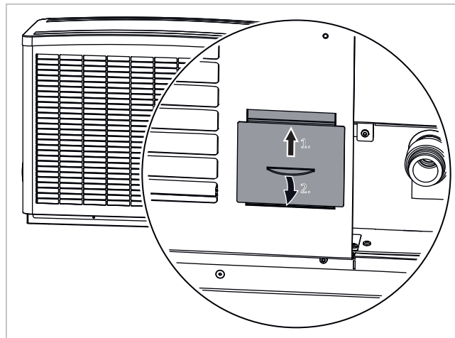
Afb. 31: Revisieschacht openen
