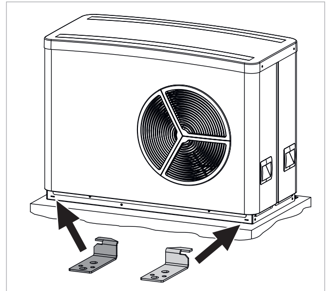
Afb. 9: Schroefkoppeling op fundering
