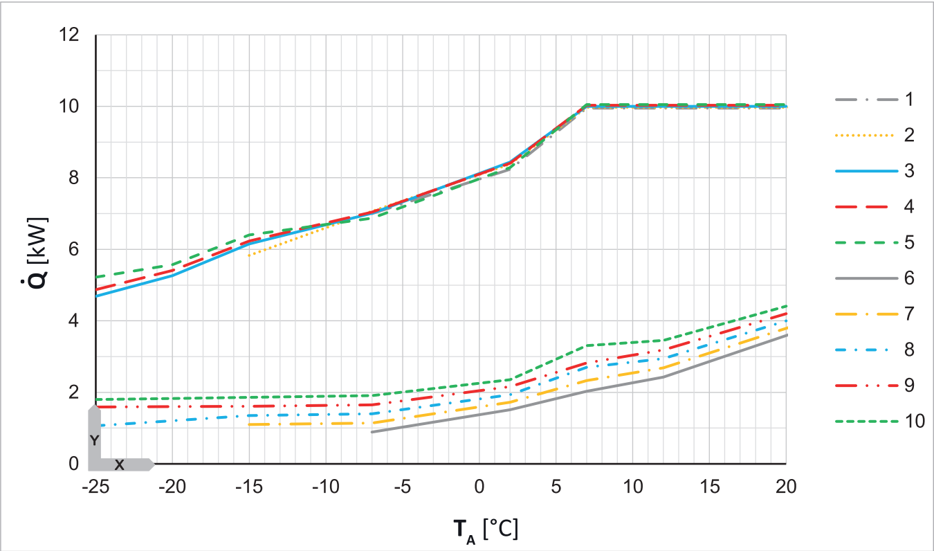
Afb. 38: Diagram prestatiegegevens van de SolvisLea 8,3 Premium
