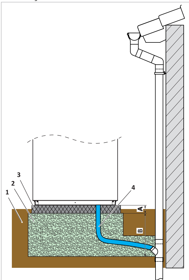
Afb. 8: Condensafvoer in valbuis of afvoer
