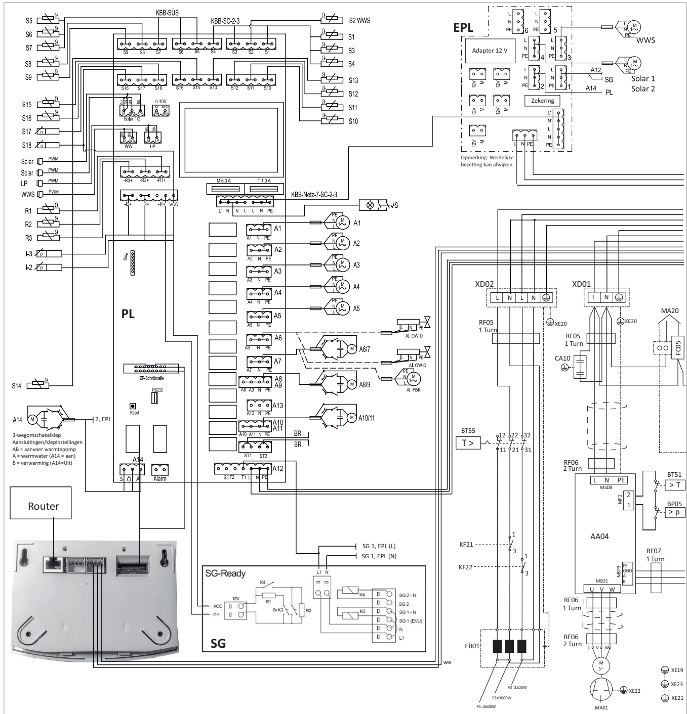
Afb. 39: Stroomloopbaan SolvisLea 8,3 Premium - deel 1
