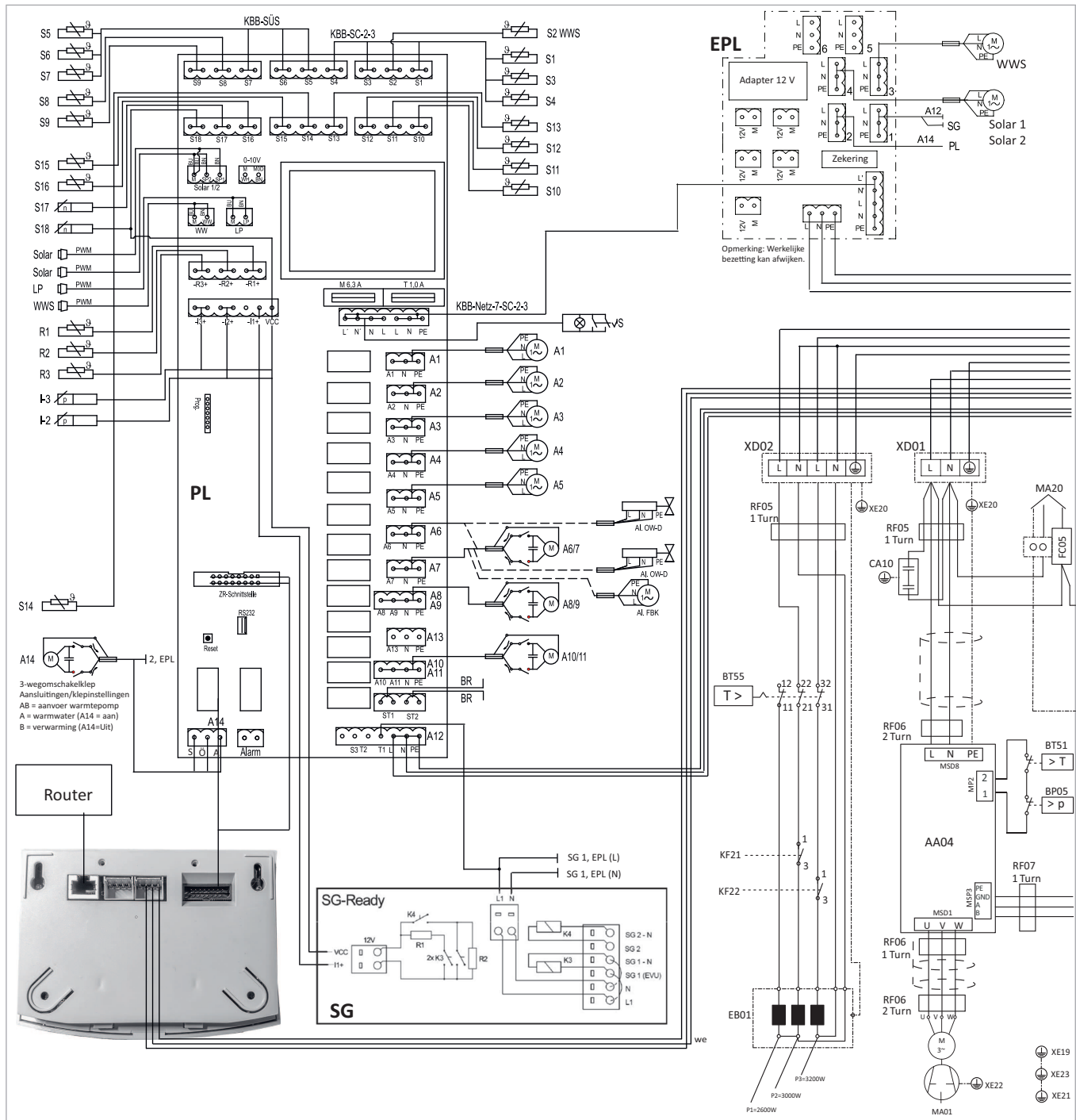
Afb. 41: Stroomschema SolvisLea 8,3 Premium hybride systeem - deel 1
