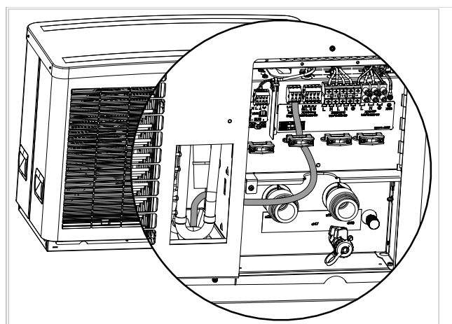
Afb. 28: Op XD06 aansluiten
