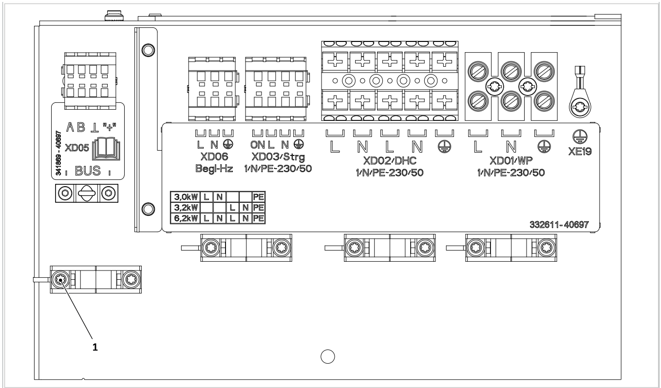
Afb. 26: SolvisLea 8,3 Premium: Aansluitdeel
