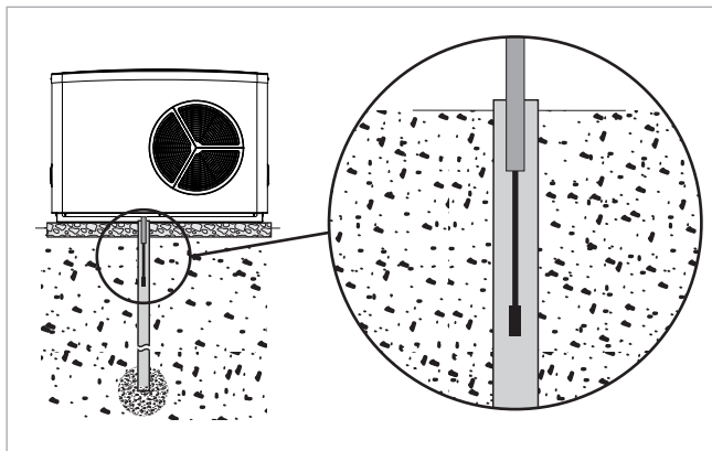
Afb. 27: Buisverwarming in condensafvoerbuis
