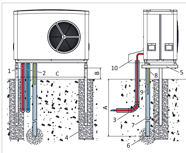
Afb. 13: SolvisLea op standconsole gemonteerd
