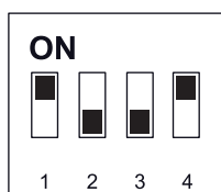
Afb. 32: Schuifschakelaar WP-type bij hybride installaties
