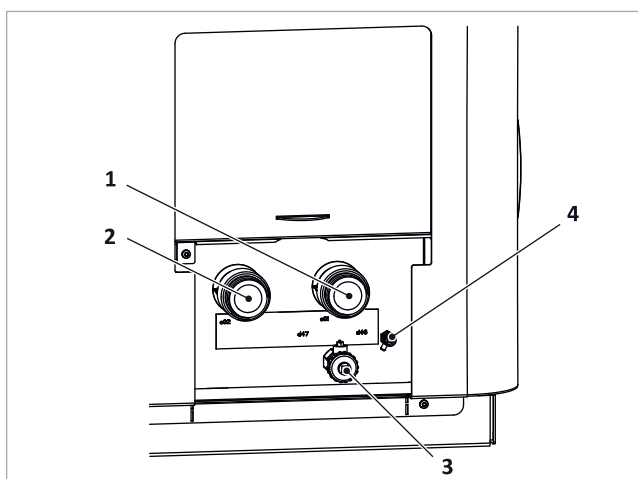
Afb. 17: SolvisLea: Hydraulische aansluiting
