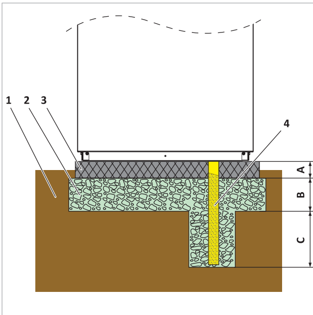
Afb. 7: Condensafvoer in grindbed
