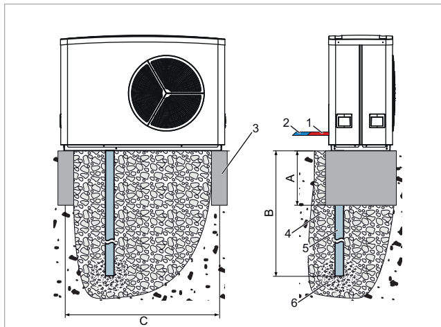
Afb. 12: SolvisLea gemonteerd op strokenfundering
