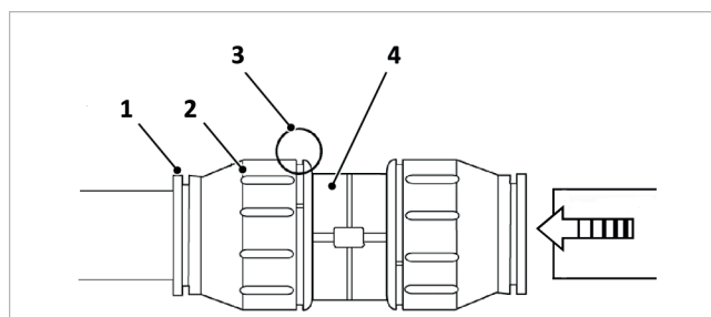
Afb. 14: Stekkerverbinding ontgrende
