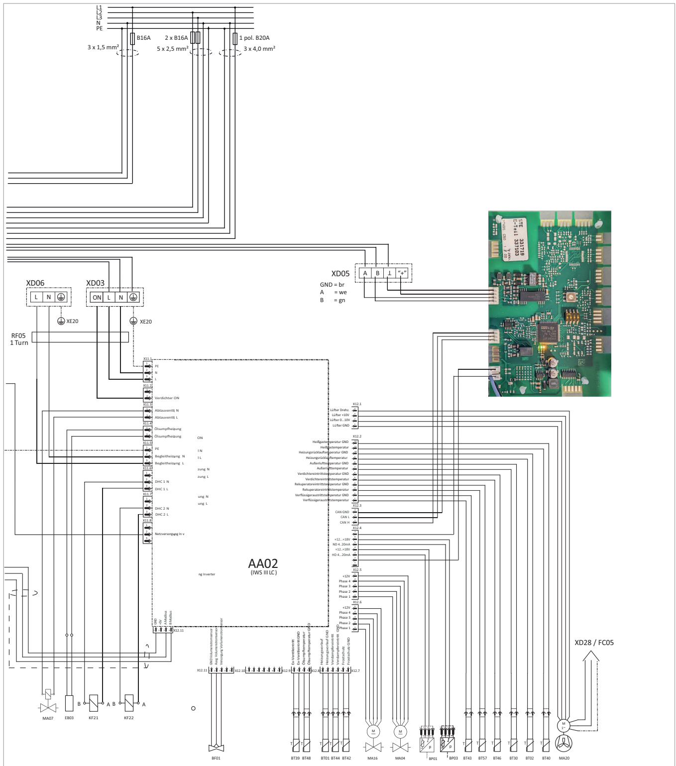
Afb. 40: Stroomloopbaan SolvisLea 8,3 Premium - deel 2
