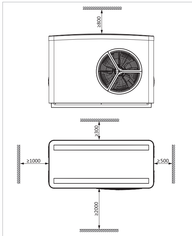
Afb. 4: Tussenafstanden ten opzichte van de wand, SolvisLea
