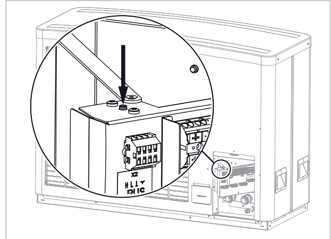
Afb. 30: Solvis Lea: Resetknop nood- en bijverwarming
