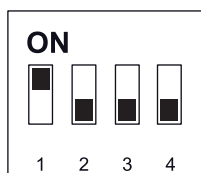
Afb. 33: Schuifschakelaar WP-type bij mono-energetische installaties
