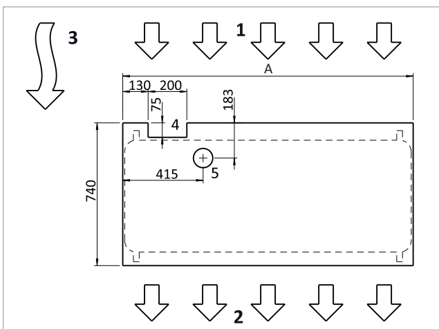
Afb. 5: Fundering voor SolvisLea (bovenaanzicht)
