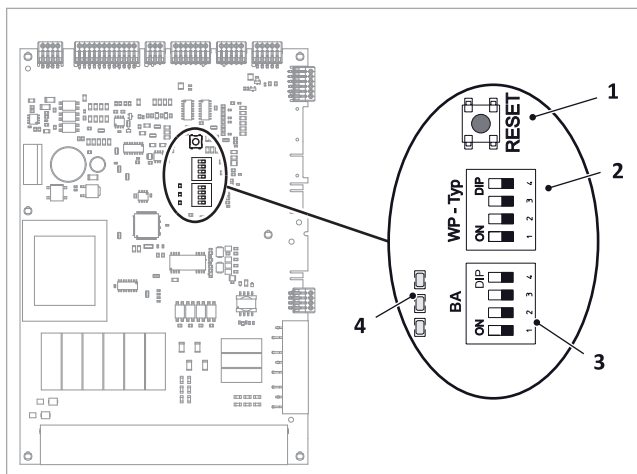
Afb. 35: IWS van de SolvisLea Eco / SolvisLea 8,3 Premium
