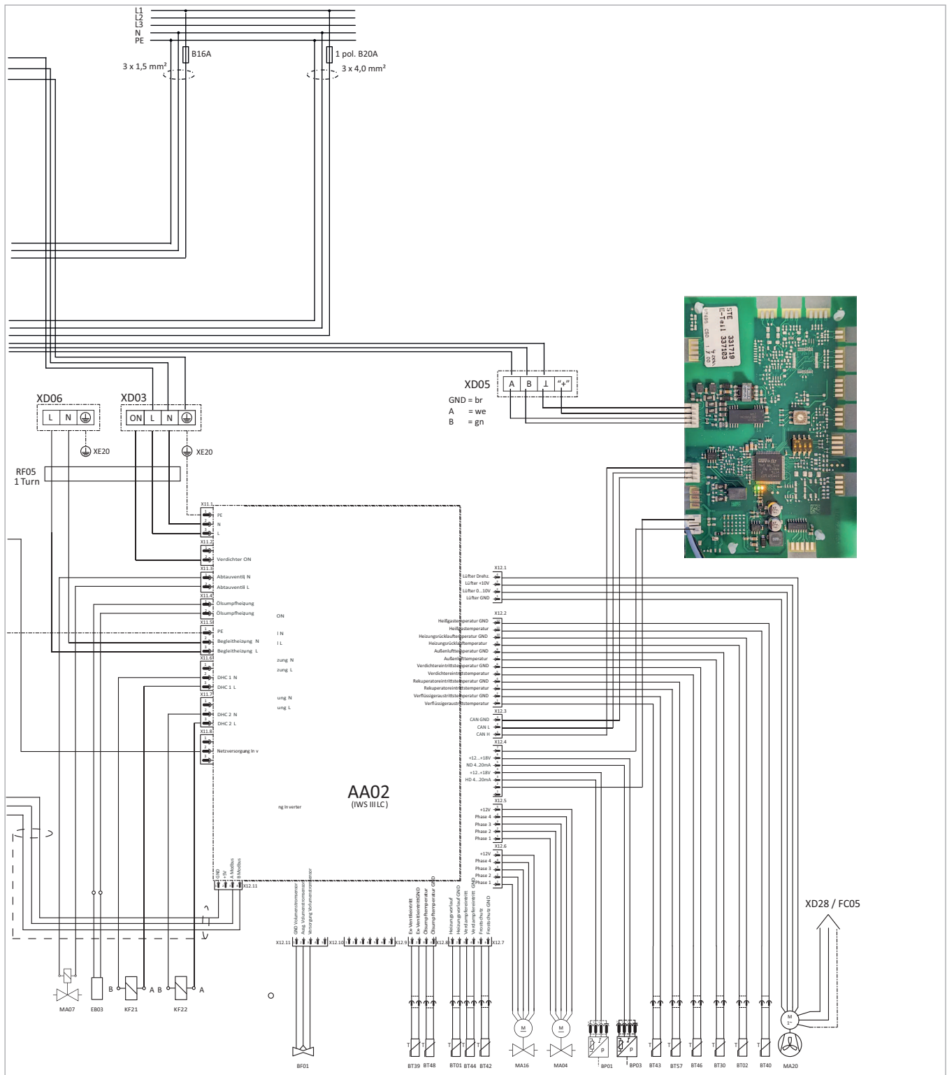
Afb. 42: Stroomschema SolvisLea 8,3 Premium hybride systeem - deel 2
