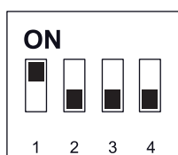
Afb. 33: Schuifschakelaar WP-type bij mono-energetische installaties
