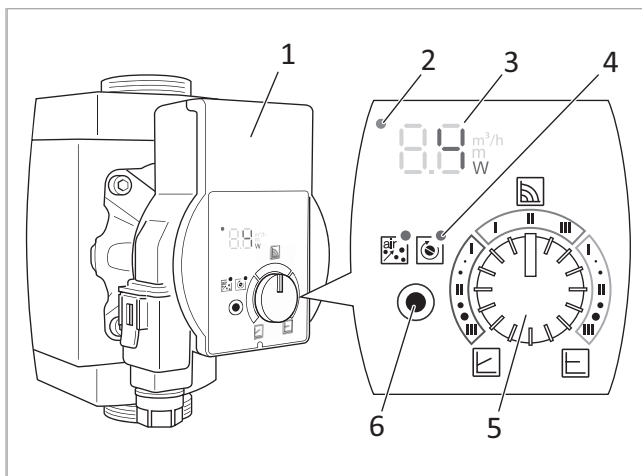
Abb. 18: Übersicht der Funktionen der Wilo-Yonos PICO plus
