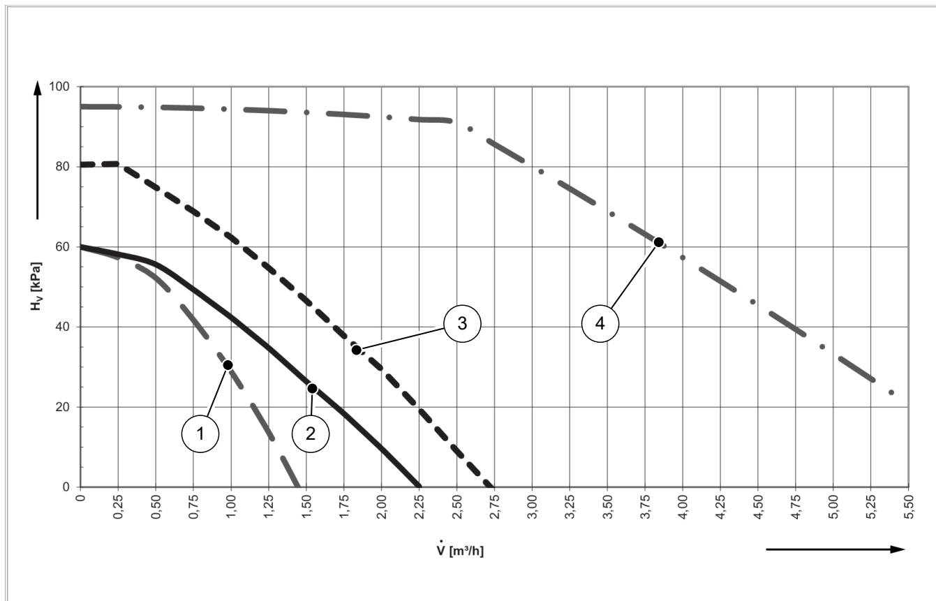
Abb. 25: Verfügbare externe Förderhöhen für bauseitige Heizkreise
