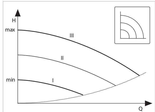
Abb. 22: Einstellung für Konstant-Drehzahl
