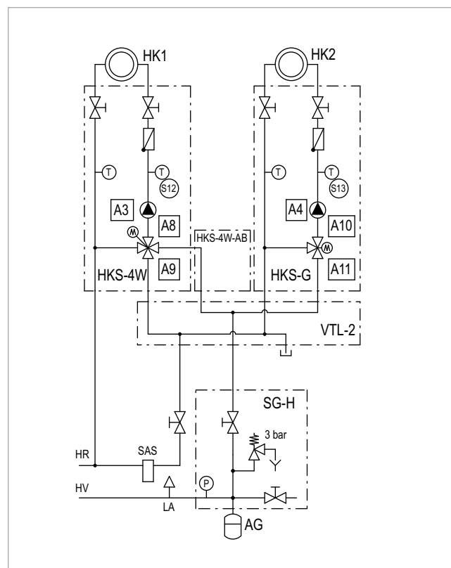
Abb. 27: HKS-4W: Zwei gemischte Heizkreise (unterschiedliche Temperaturniveaus)
