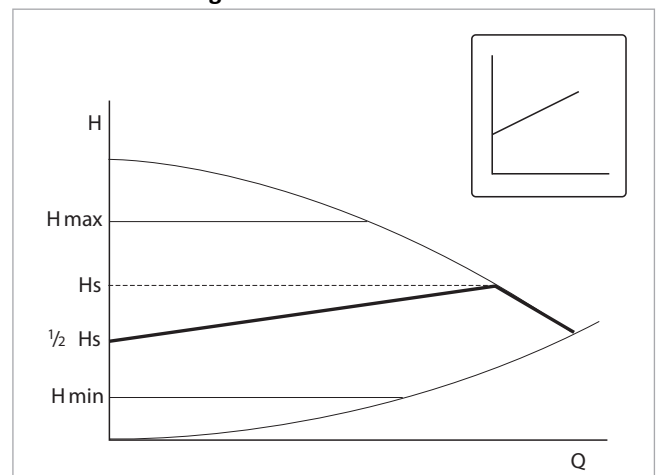
Abb. 20: Einstellung für Radiatorenheizung
