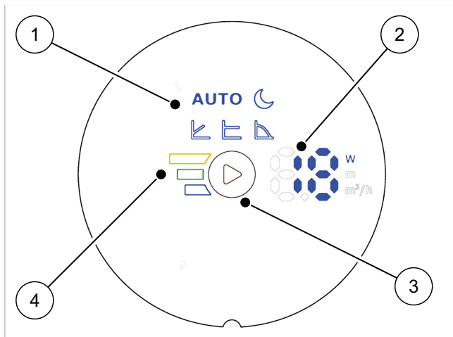
Abb. 24: Bedienfeld IMP NMT Mini Pro
