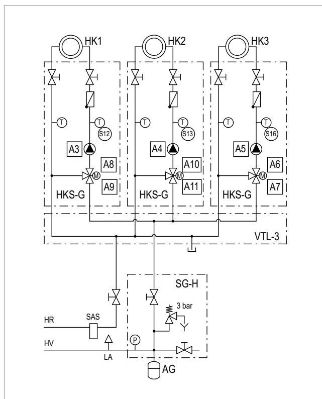
Abb. 26: HKS-G und HKS-B: Zwei gemischte Heizkreise und ein ungemischter, temperaturbegrenzter Heizkreis
