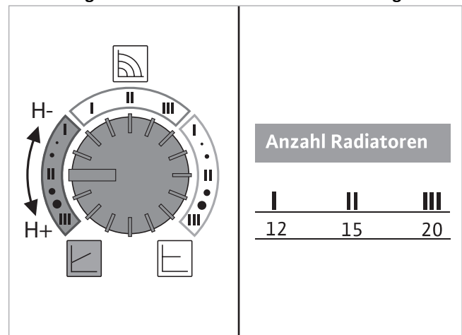
Abb. 23: Einstellung der Förderhöhe bei Radiatorenheizung
