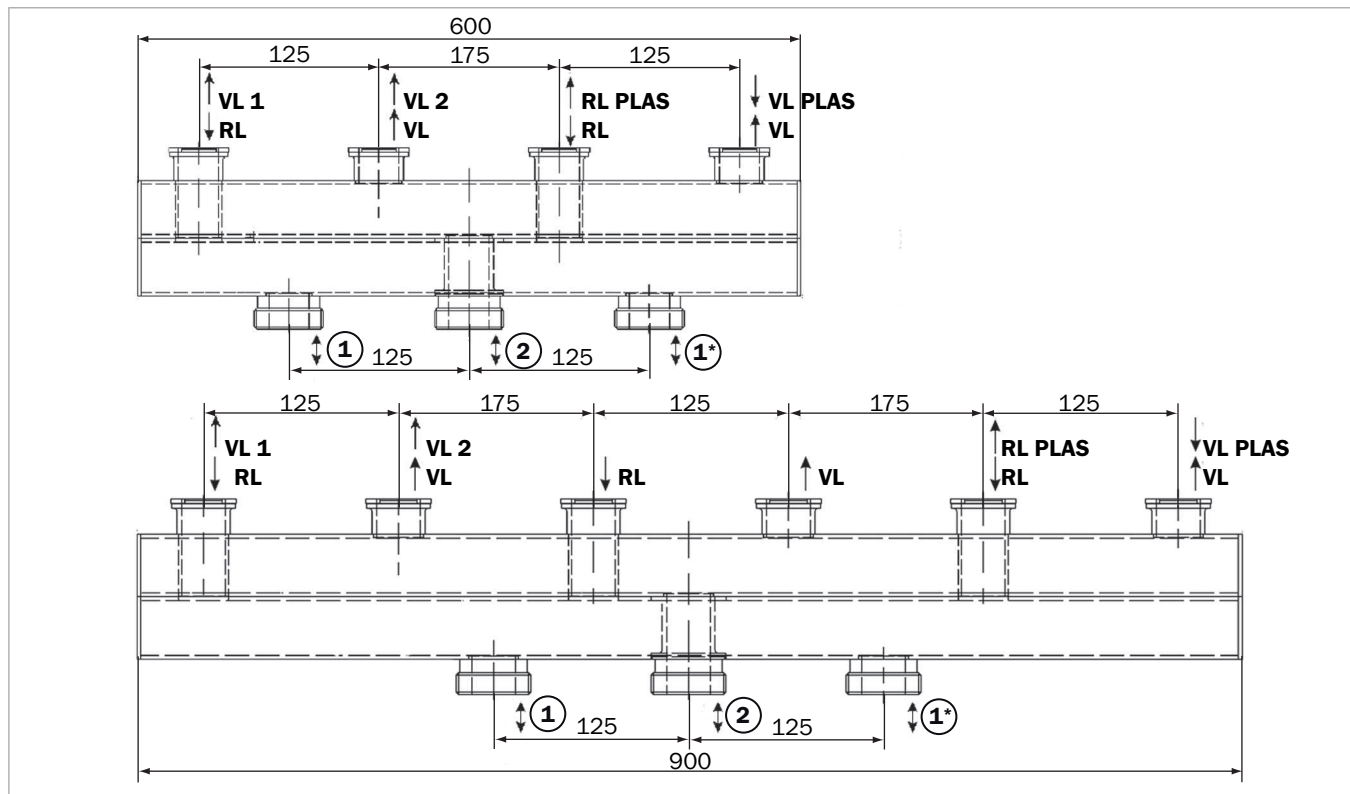
Abb. 28: Anschlüsse am Heizkreisverteiler
