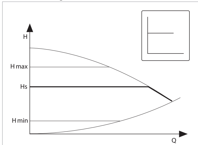
Abb. 21: Einstellung für Fußbodenheizung
