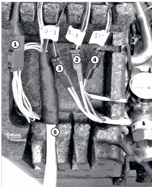
Fig. 4: Collegamenti al cavo di prolunga
