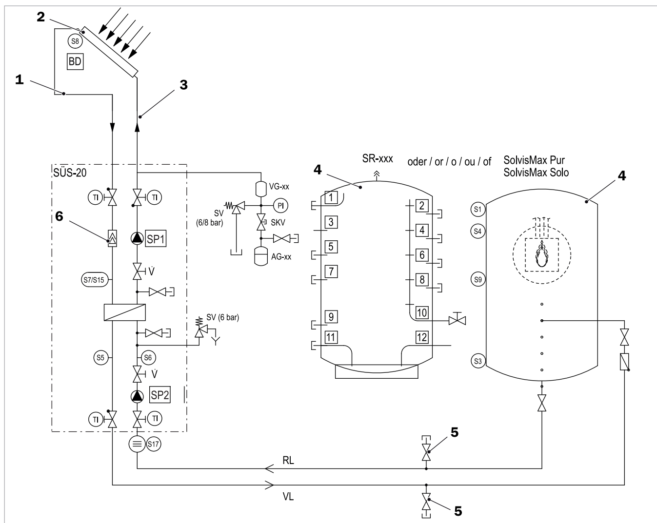
Fig. 16: Stazione di trasmissione del calore solare con impianto SolvisMax Pur (gas, olio oppure pompa di calore) e SolvisMax Solo
