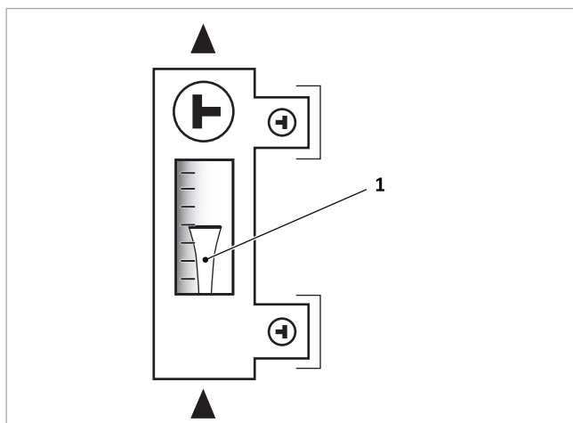
Fig. 12: lettura del flusso volumetrico nel bordo superiore del galleggiante (1)
