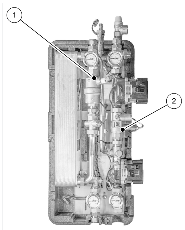
Fig. 13: Posizione delle valvole per la manutenzione
