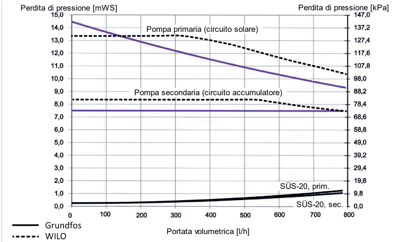
Fig. 15: Curva perdita di pressione del circuito primario SÜS-20
