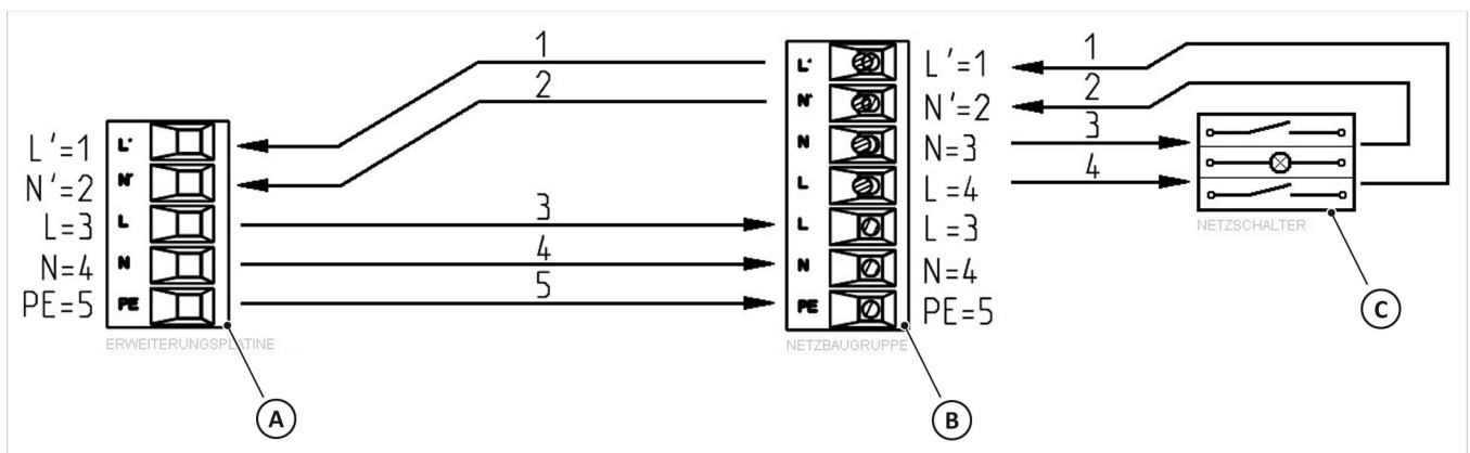
Fig. 2: Elektrische aansluiting
