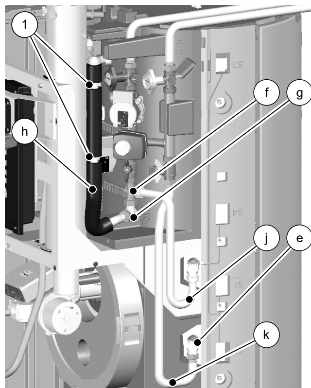
Afb. 6: Omgebouwde verwarmingspomp-aansluiting
