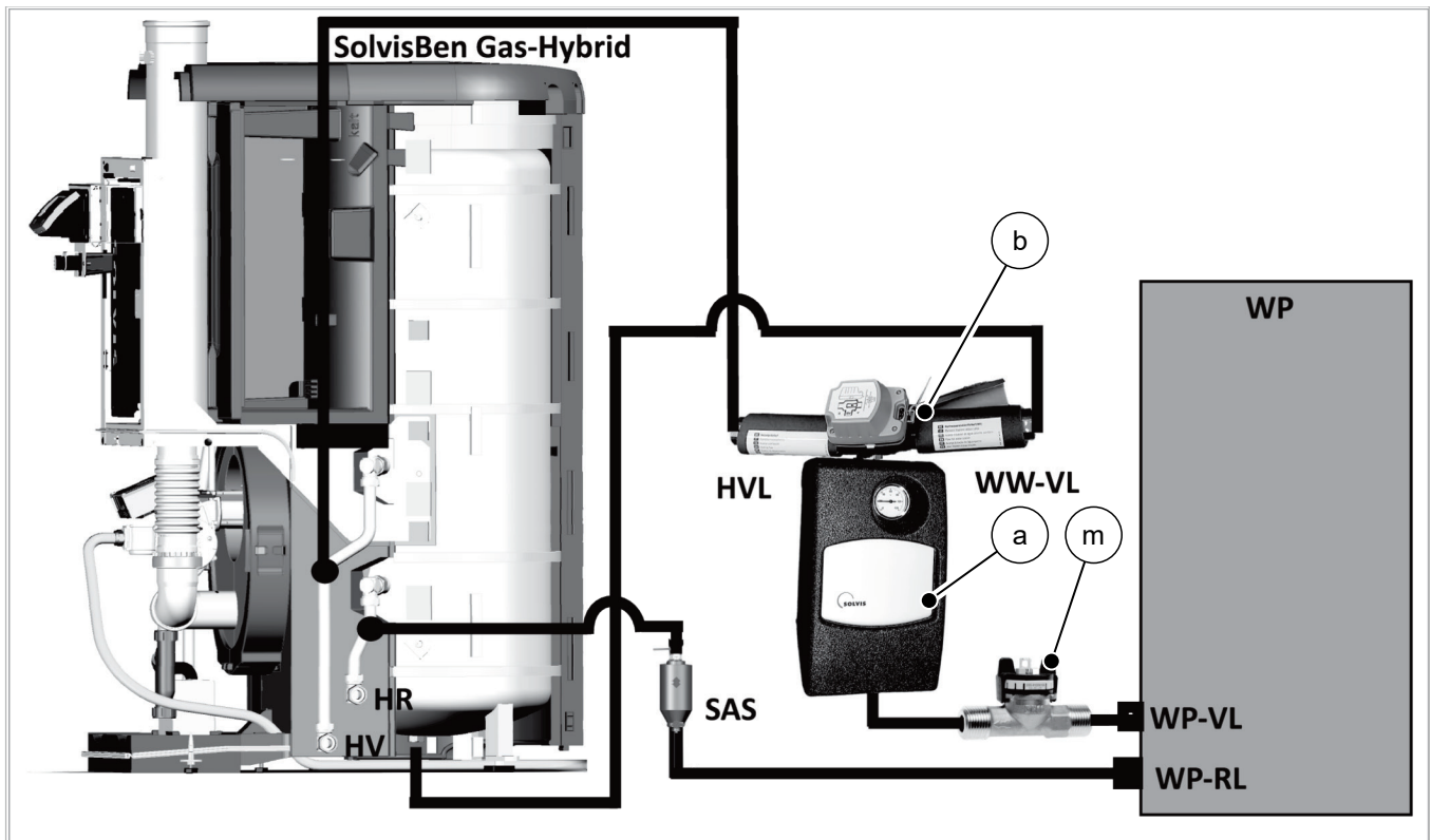
Afb. 8: Overzicht aansluiting SolvisMia aan SolvisBen GAS-hybride, zonder geïntegreerde verwarmingscircuitstation (HKS)
