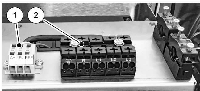
Afb. 18: SolvisMia aansluitdeel
