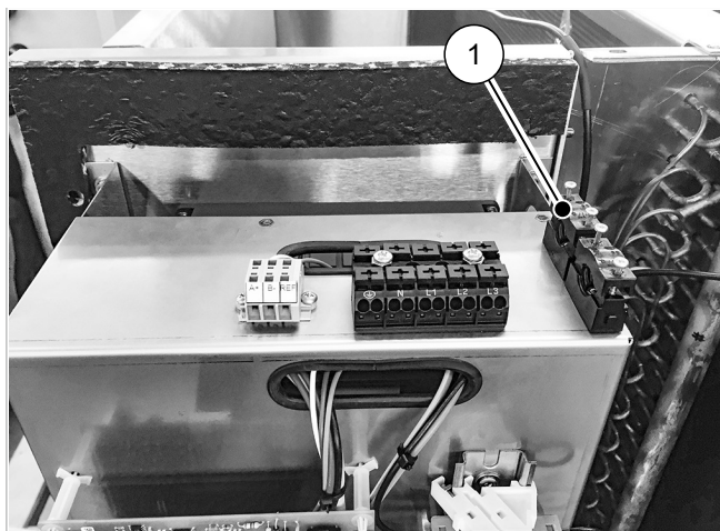
Afb. 17: Kabel doorvoeren
