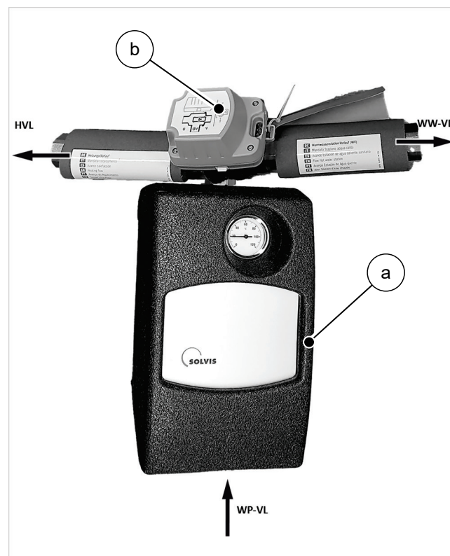
Afb. 3: Bufferlaadstation met omschakelklep
