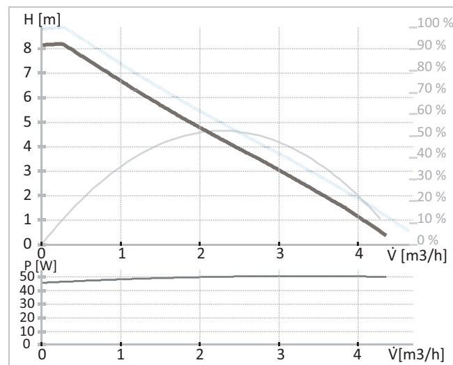
Afb. 24: Pompkarakteristiek IMP NMT Mini PWM 15/80-130 (constant toerental)
