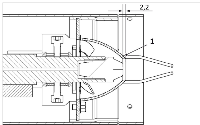
Fig. 143: Sección transversal del cabezal de mezcla
