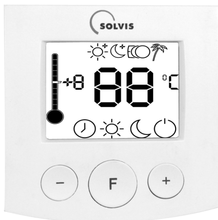
Fig. 113: Elemento de manejo ambiental BE-SC-2
