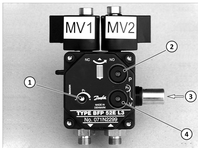
Fig. 125: Ajustar la presión de la bomba de gasóleo
