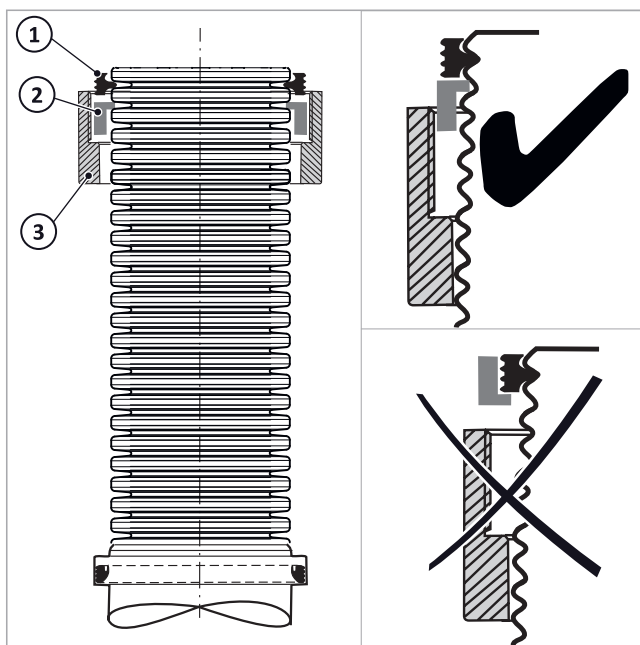
Fig. 81: Unión atornillada insertada en el tubo flexible
