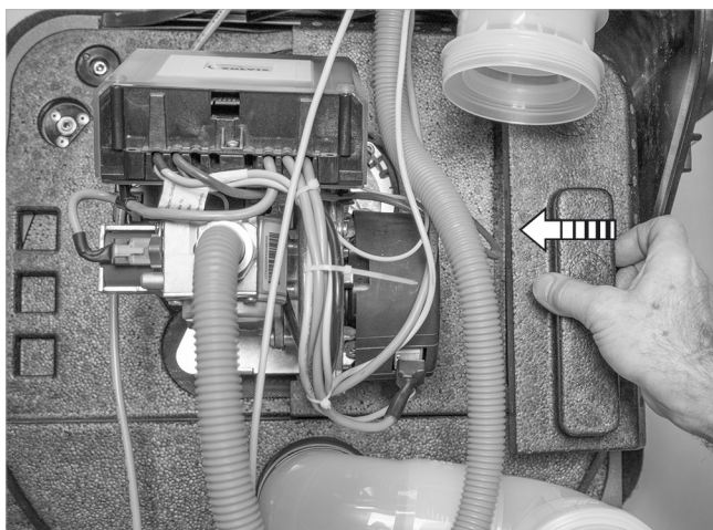
Fig. 93: Montaje del aislamiento de la brida delantera derecha (parte III)
