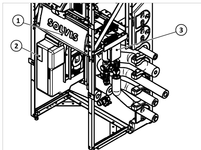
Fig. 117: Módulo de carga con SmartGrid Box
