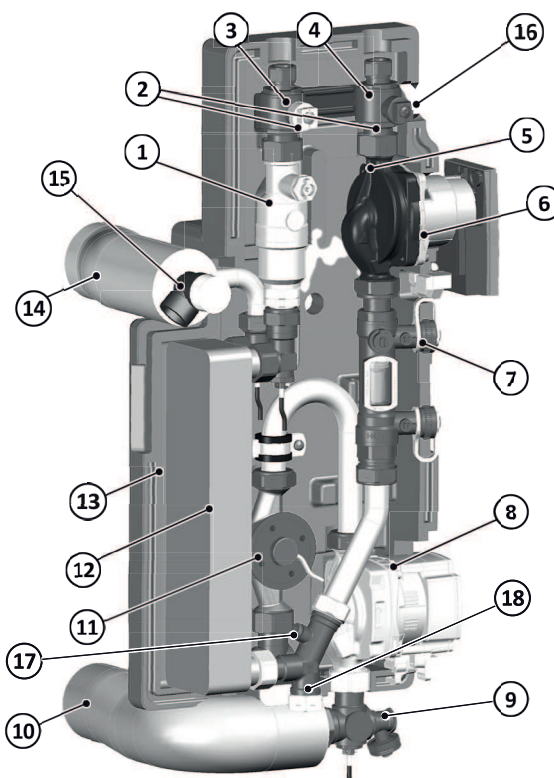
Fig. 104: Vista general de los componentes de la estación de transferencia de calor solar
