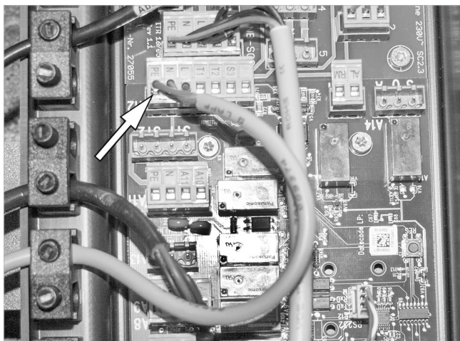
Fig. 47: Conexión del conector de quemador a gas en A12
