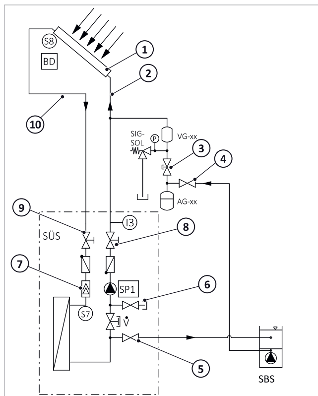
Fig. 127: Estación de transferencia de calor solar: Lavado del intercambiador de calor
