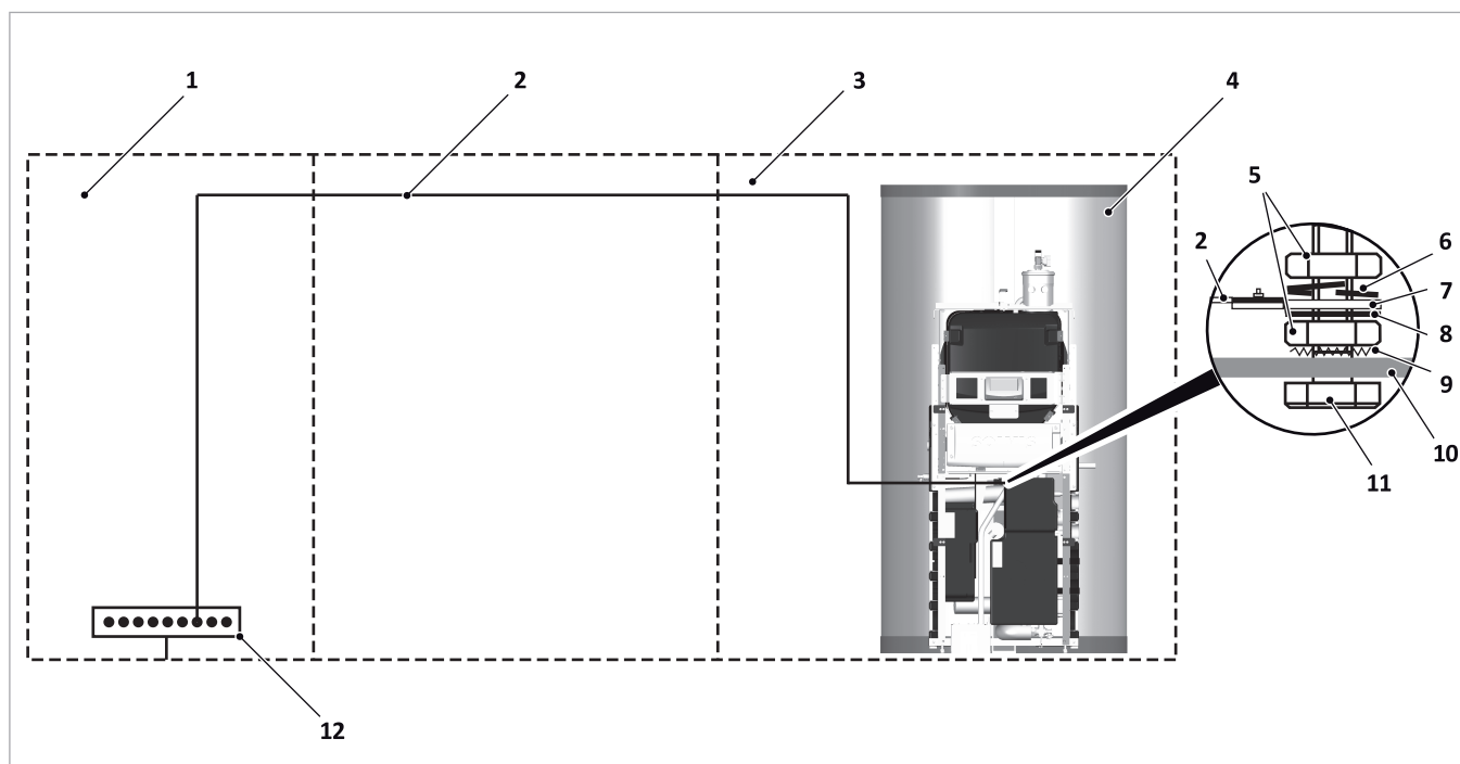
Fig. 111: Conexión equipotencial del SolvisMax
