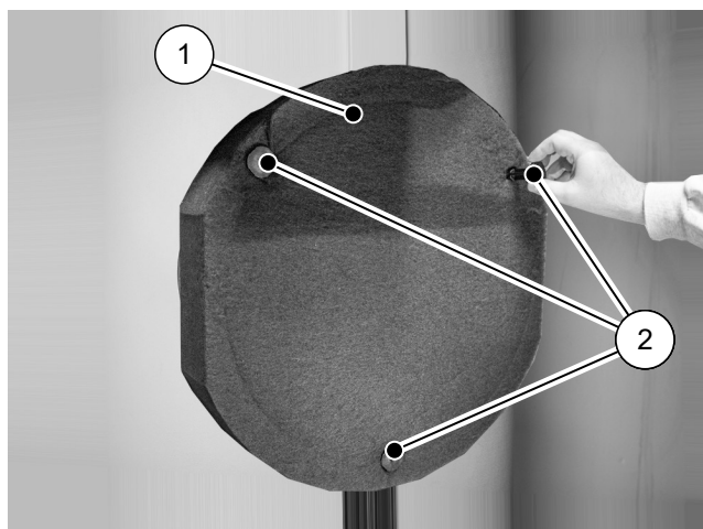
Fig. 9: Fijar el aislante de la brida Solo
