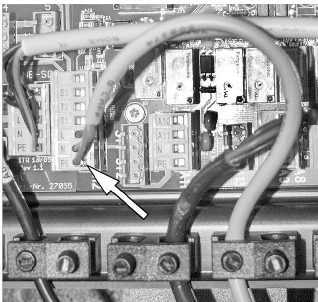
Fig. 70: Conexión del conector de quemador de gasóleo en A12
