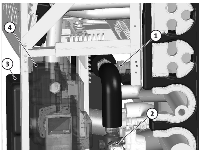
Fig. 26: Montaje de la válvula conmutadora (avance de la bomba de calor hacia la derecha)
