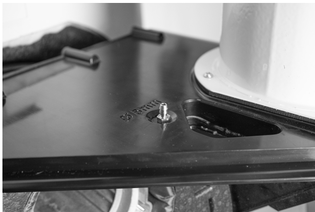
Fig. 54: Fijar la boquilla de vapor de aceite con la tuerca
