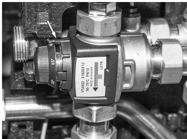
Fig. 122: Ajuste TMV
