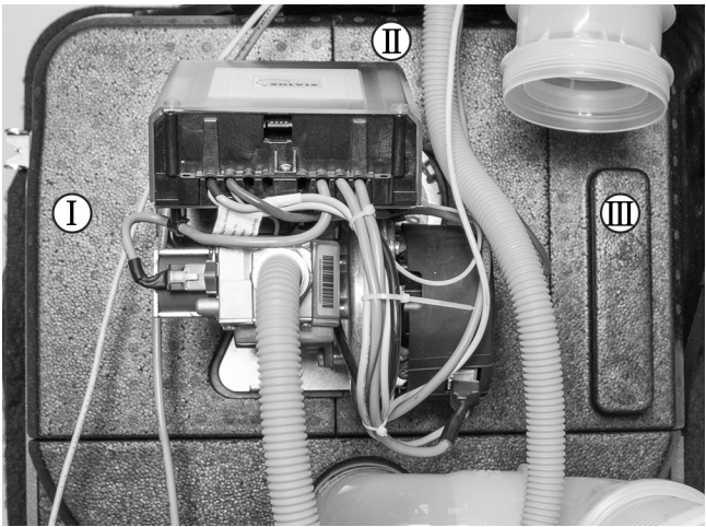
Fig. 89: Aislamiento de la brida delantera (3 piezas)
