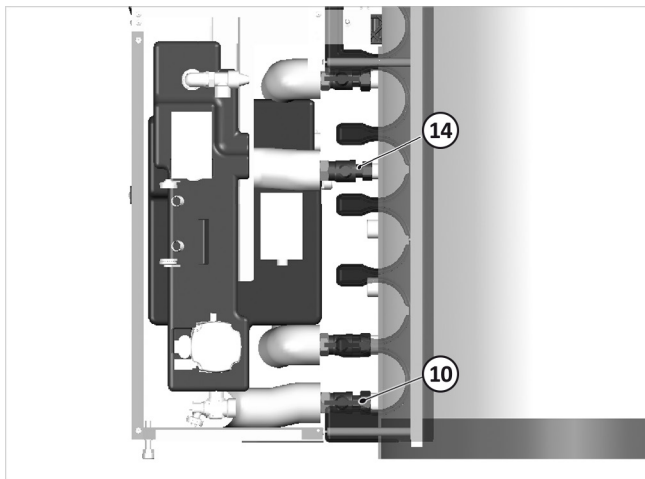
Fig. 105: Conectar la estación de transferencia de calor solar
