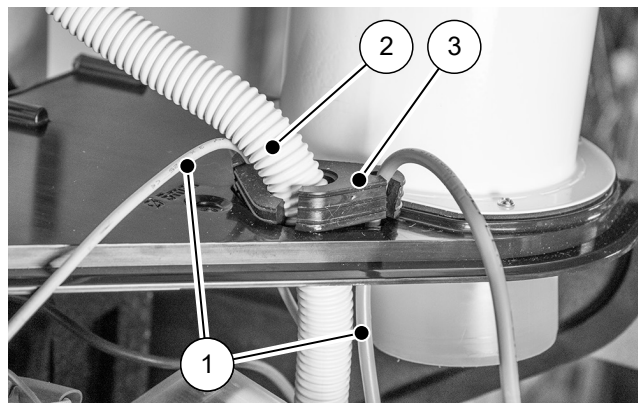
Fig. 46: Paso de cables en la cámara de aspiración
