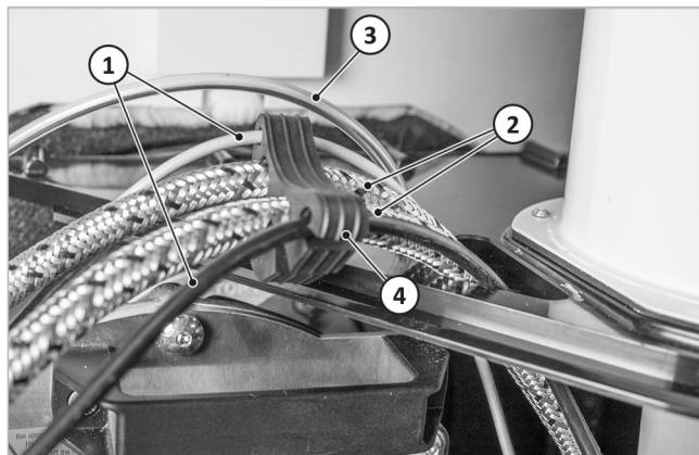
Fig. 69: Paso de conductos en la cámara de aspiración
