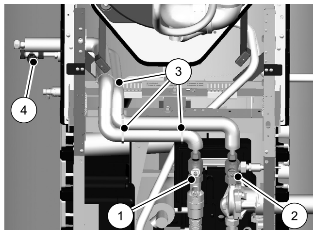
Fig. 108: Tender y fijar las tuberías solares
