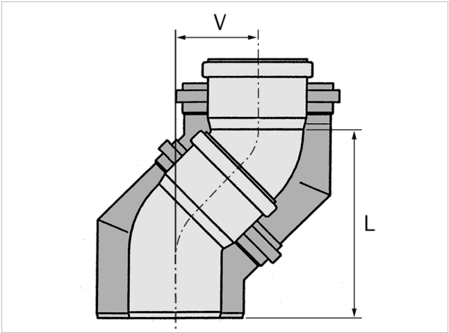
Fig. 88: Desplazamiento y longitud
