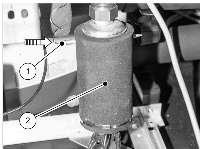
Fig. 32: Insertar el mSTB en el manguito
