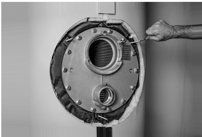
Fig. 7: Montar las barras roscadas
