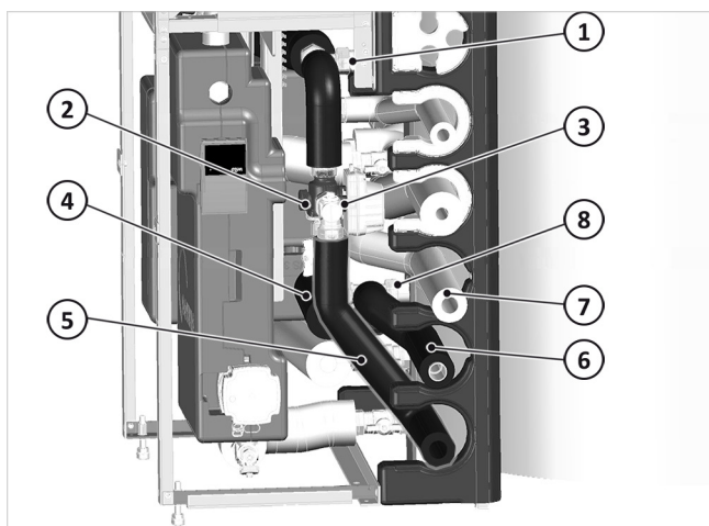
Fig. 28: Tubo de conexión de avance WP montado (hacia la derecha)
