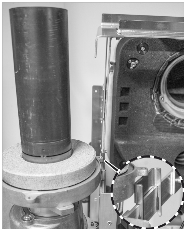
Fig. 139: Quemador en posición de estacionamiento
