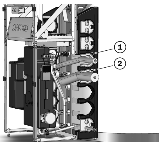
Fig. 103: Estación de agua caliente sanitaria, conducción de los tubos de agua potable (derecha)
