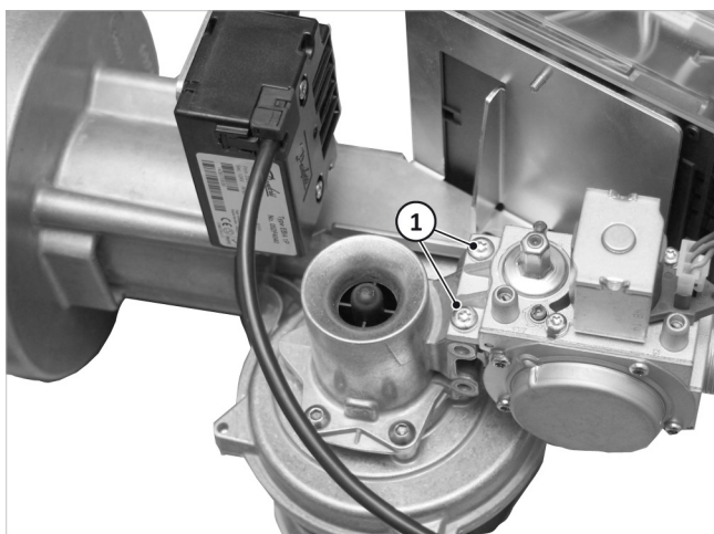
Fig. 33: Desmontar la válvula reguladora de gas
