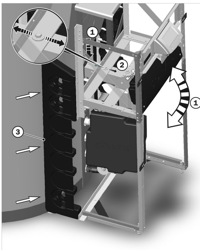
Fig. 18: Nivelar el módulo de carga
