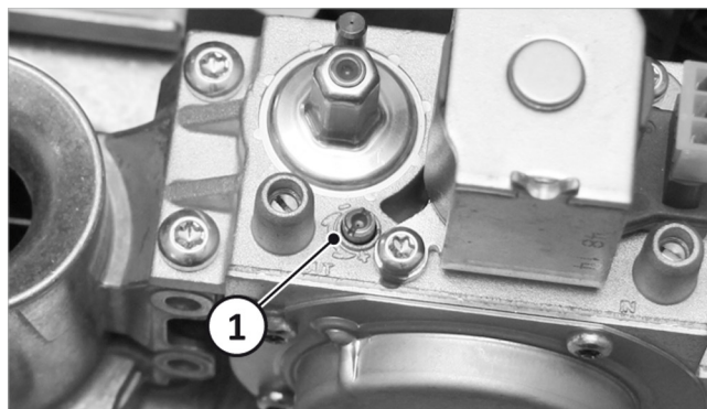
Fig. 35: Ajuste del quemador
