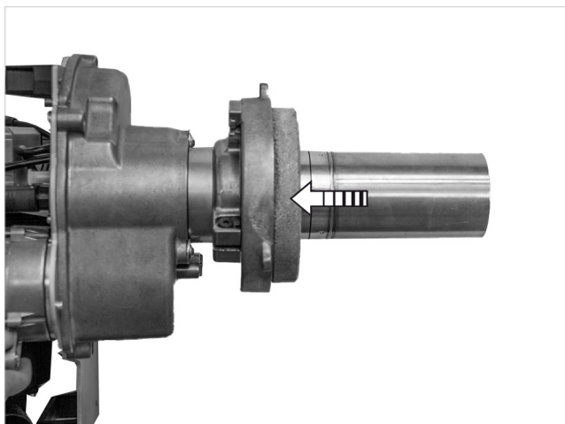
Fig. 59: Colocación del ladrillo de la puerta de la caldera
