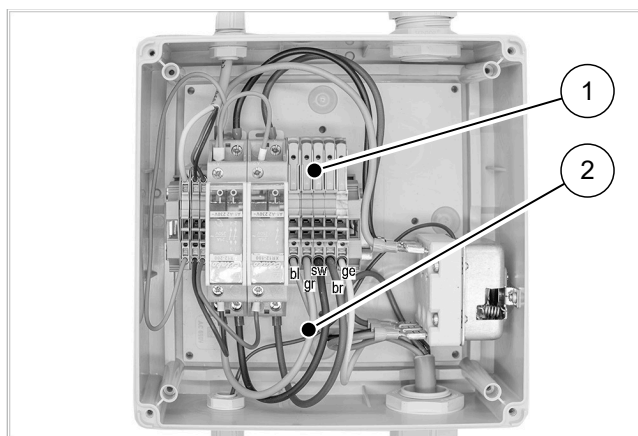
Fig. 118: Caja de conexiones, abierta
