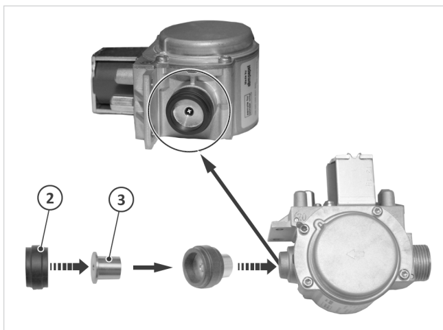
Fig. 34: Montar la tobera de gas líquido
