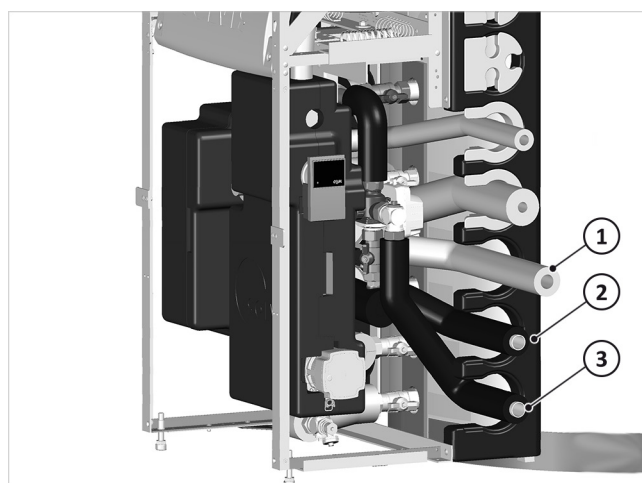
Fig. 98: Conexión hidráulica bomba de calor
