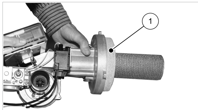
Fig. 41: Colocar el ladrillo de puerta de caldera
