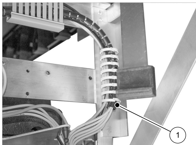
Fig. 21: Tender al mazo de cables hacia la placa de circuitos impresos de red
