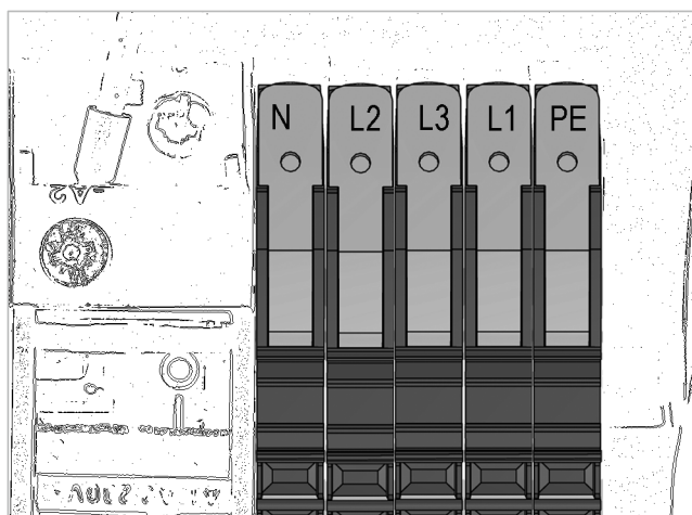
Fig. 119: Distribución de las conexiones de (1)
