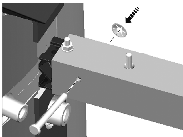
Fig. 16: Perno y arandela de fijación
