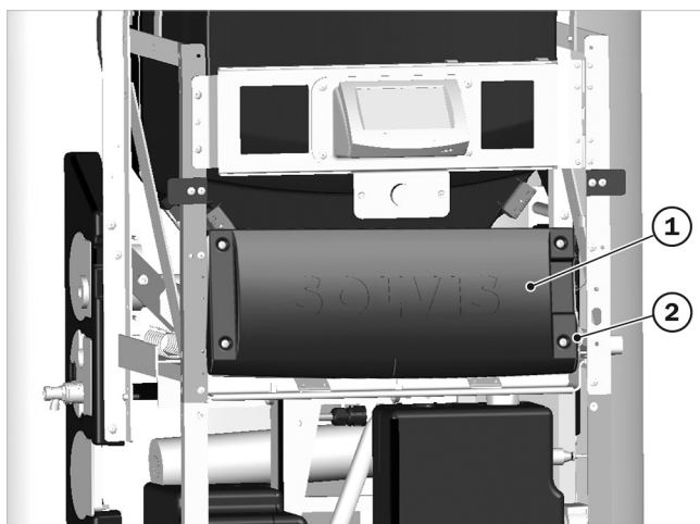
Fig. 120: Fijar la tapa de la placa de circuitos impresos de red
