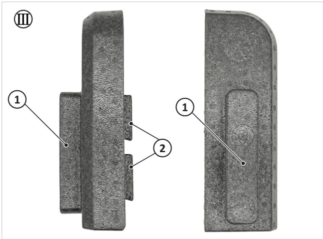
Fig. 90: Aislamiento de la brida delantera (III) con muelles de bloqueo
