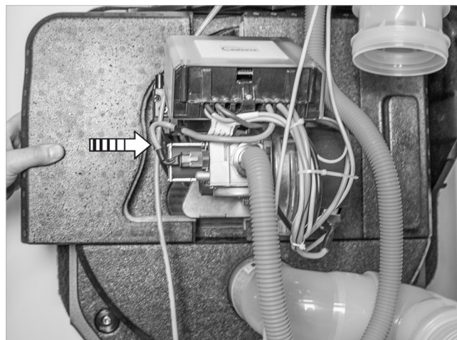
Fig. 94: Montaje del aislamiento de la brida delantera derecha (parte I)
