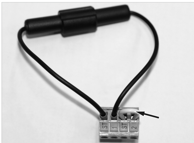
Fig. 50: Conector hembra con fusible (negro) para quemador SX-LN-3 (conexión ASTB véase flecha)
