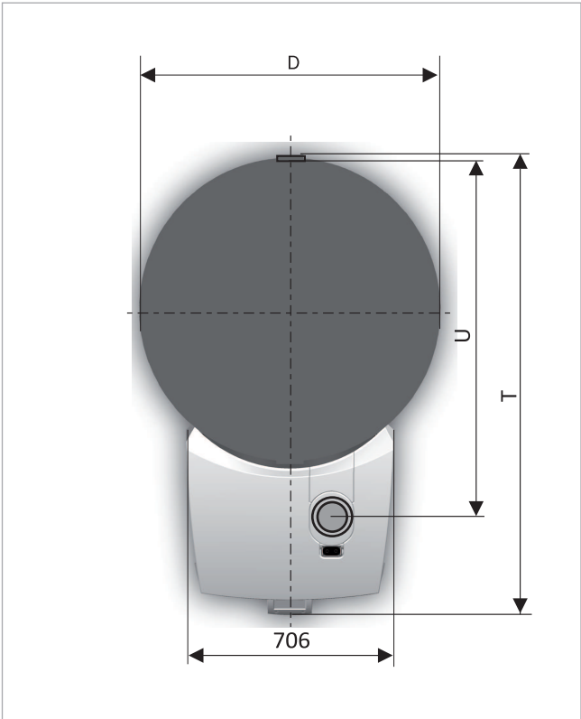
Fig. 149: Vista superior
