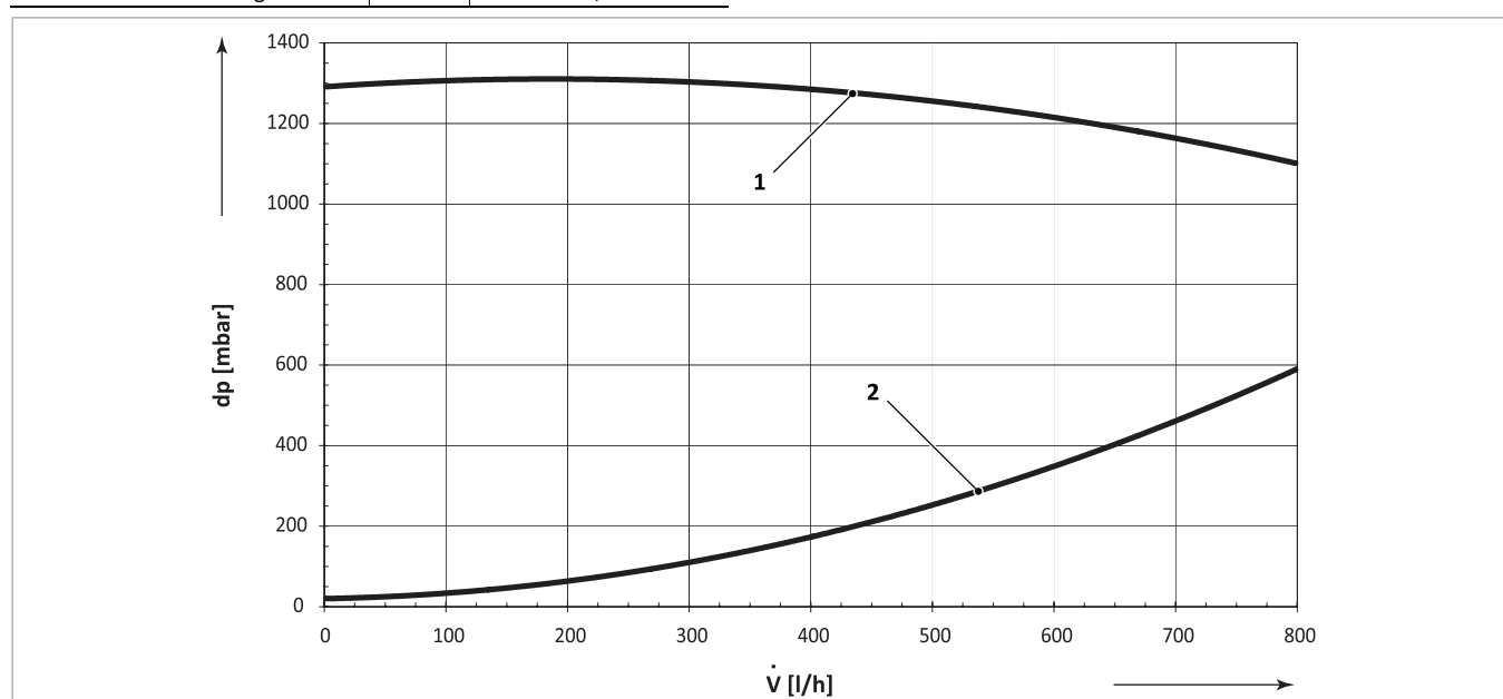
Fig. 153: Curva de pérdida de carga del circuito primario
