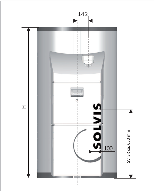
Fig. 148: Vista frontal
