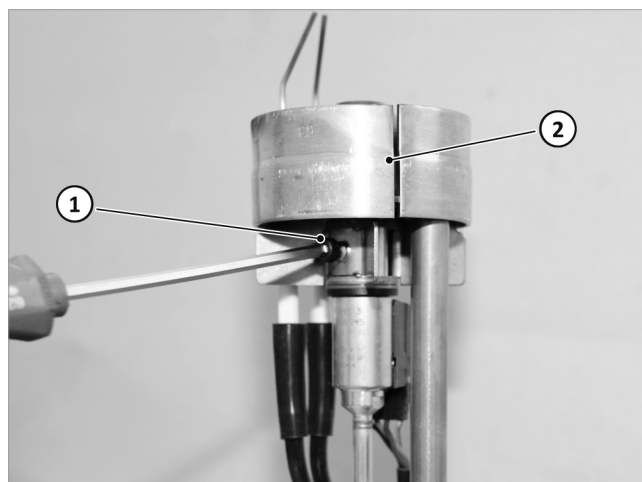
Fig. 142: Cabezal de mezcla en el portatoberas
