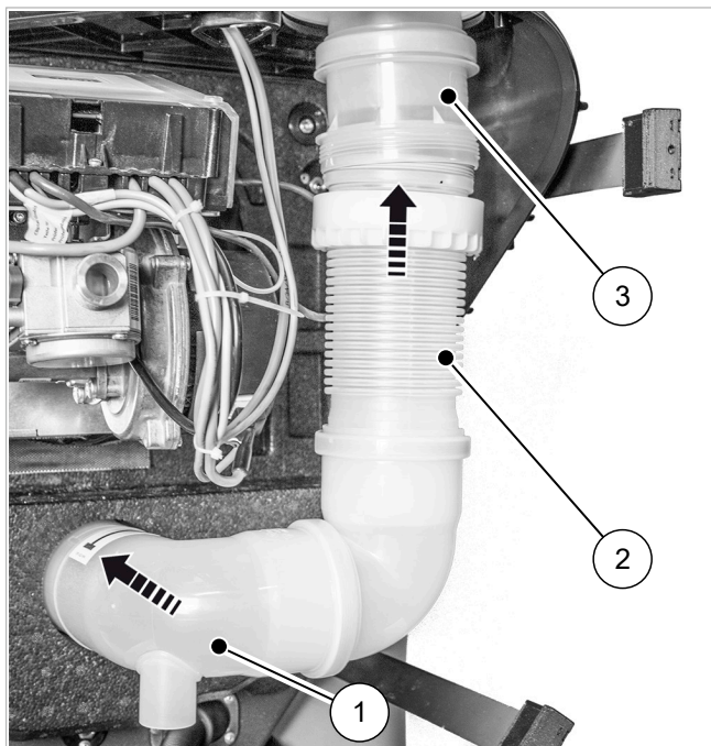
Fig. 77: Codo de salida de humos montado
