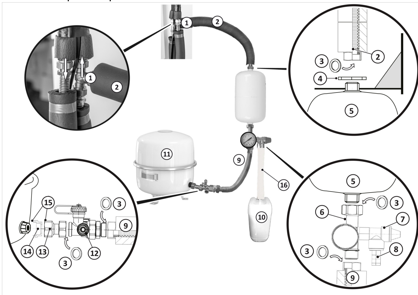
Fig. 109: Conexión de Solar-MAG
