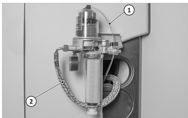
Fig. 68: Conexión de las tuberías de gasóleo
