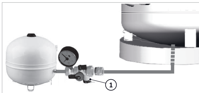
Fig. 123: Grifo KFE en el grupo de conexión MAG
