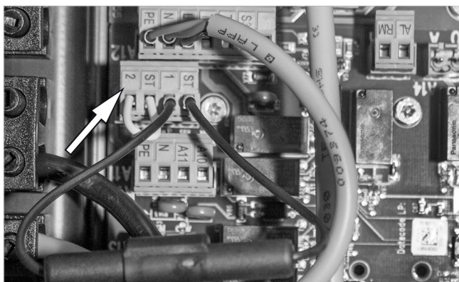
Fig. 72: Conexión de la regleta de hembrillas
