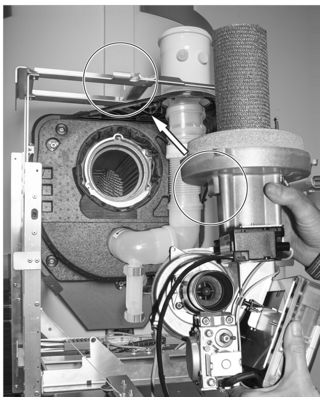
Fig. 134: Quemador en posición de mantenimiento en la consola
