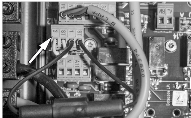
Fig. 49: Conexión de la regleta de hembrillas
