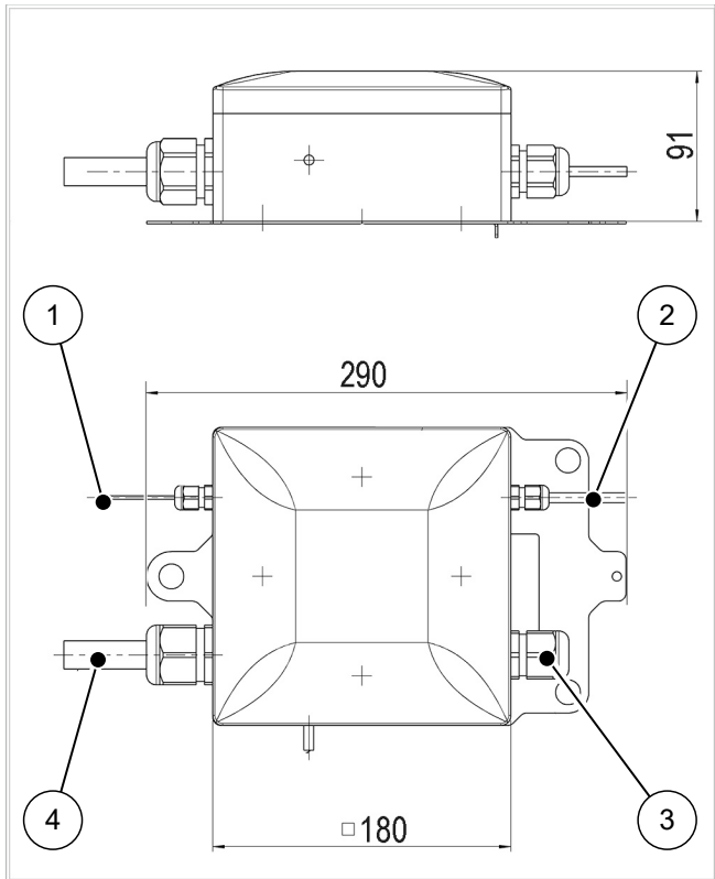
Fig. 154: Dimensiones de la caja de conexiones
