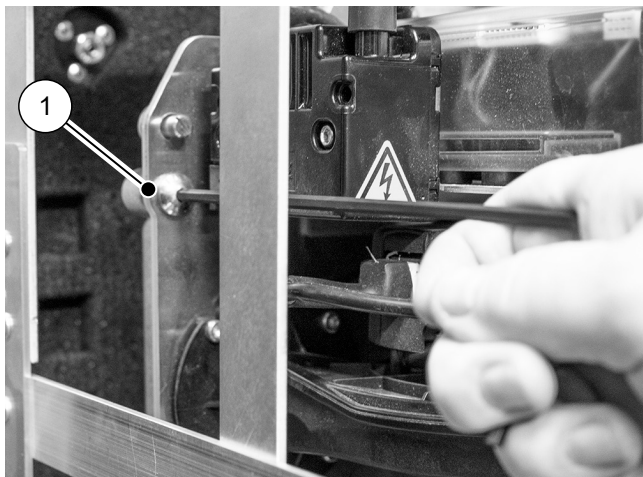
Fig. 140: Tornillos de cierre rápido en la unidad del quemador
