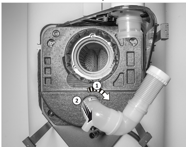
Fig. 83: Girar el codo de salida de humos (1) y extraerlo (2)
