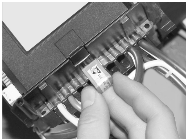
Fig. 36: Montar la tarjeta de chip del quemador
