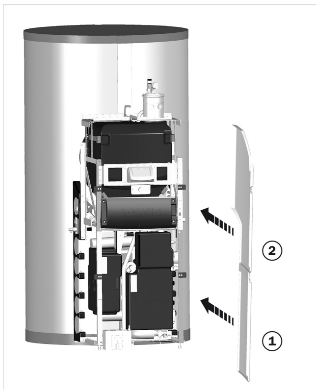
Fig. 132: Introduzca primero la pieza lateral inferior (1)
