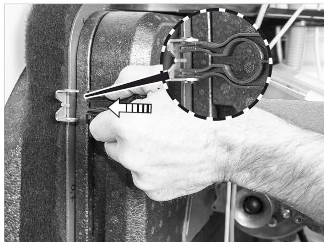
Fig. 95: Montaje del riel guía
