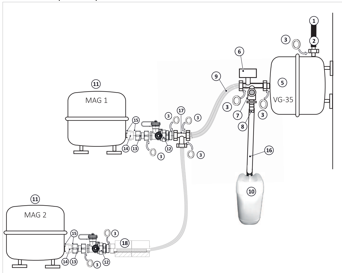
Fig. 110: Conexión de dos Solar-MAG por medio de un set de extensión de vaso de expansión (EW-AG)
