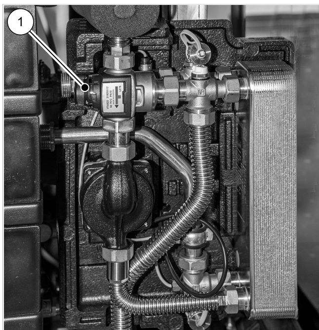
Fig. 121: Válvula mezcladora térmica (1) en una ACS-30, SolvisMax
