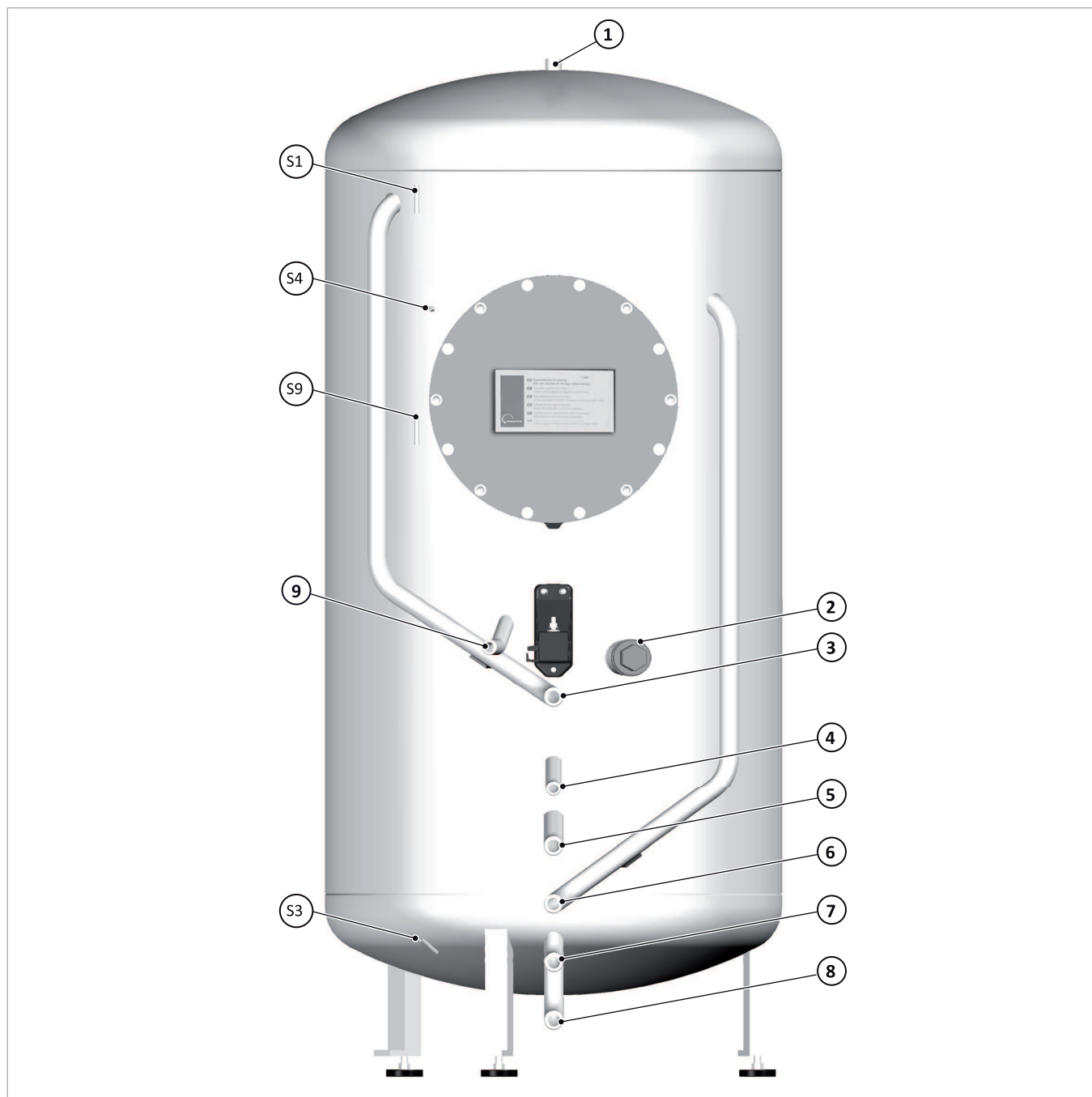
Fig. 156: Vista frontal del acumulador de estratificación
