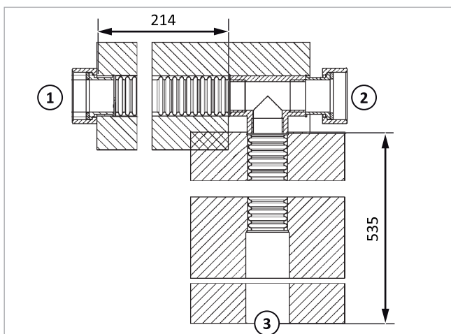
Fig. 106: Tubo de conexión de caldera de combustible sólido (RO-FBK-RL)
