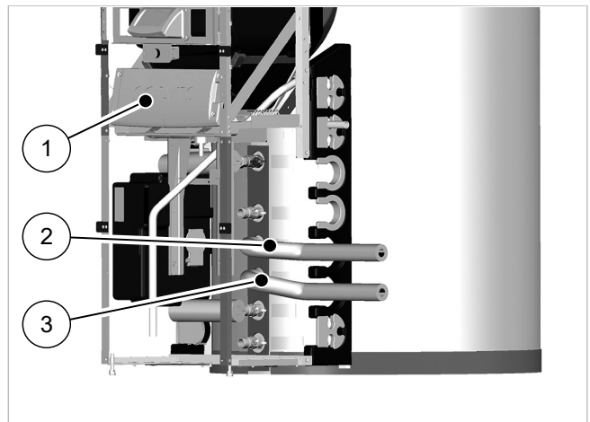
Fig. 99: Integración hidráulica de circuitos de calefacción
