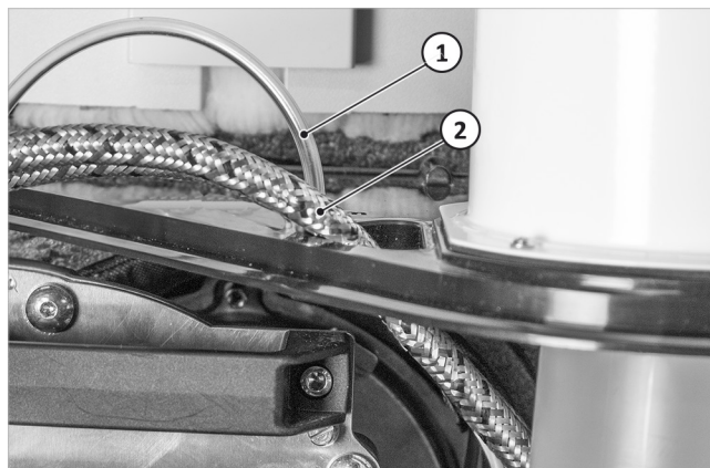
Fig. 66: Pasar las tuberías de gasóleo por la apertura
