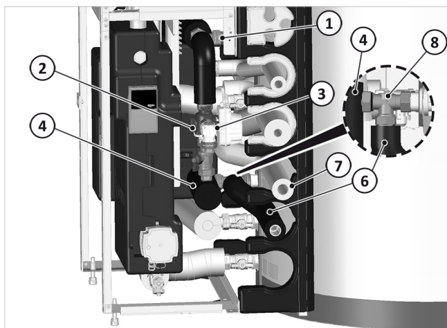
Fig. 27: Montaje de la válvula conmutadora (avance de la bomba de calor hacia la derecha)
