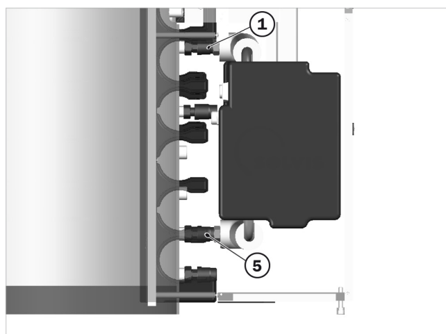
Fig. 101: Conexión de la estación de agua caliente sanitaria
