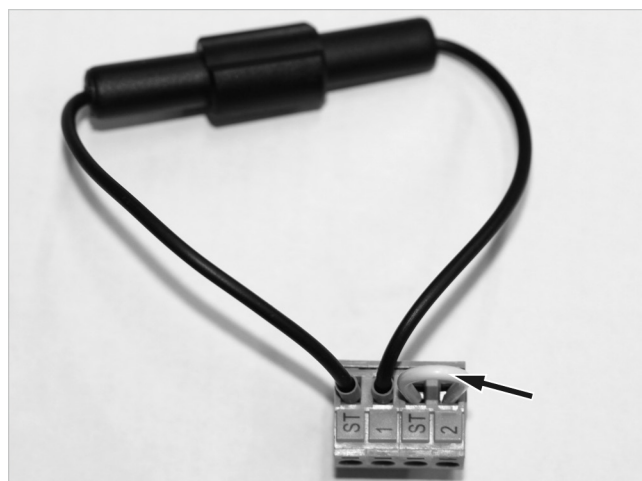
Fig. 73: Conector hembra con fusible (negro) para quemador SX-LN-3 (conexión ASTB véase flecha)
