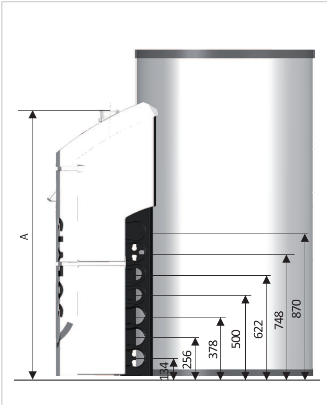
Fig. 150: Vista lateral
