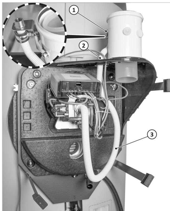
Fig. 44: Tubería de gas tendida hacia arriba
