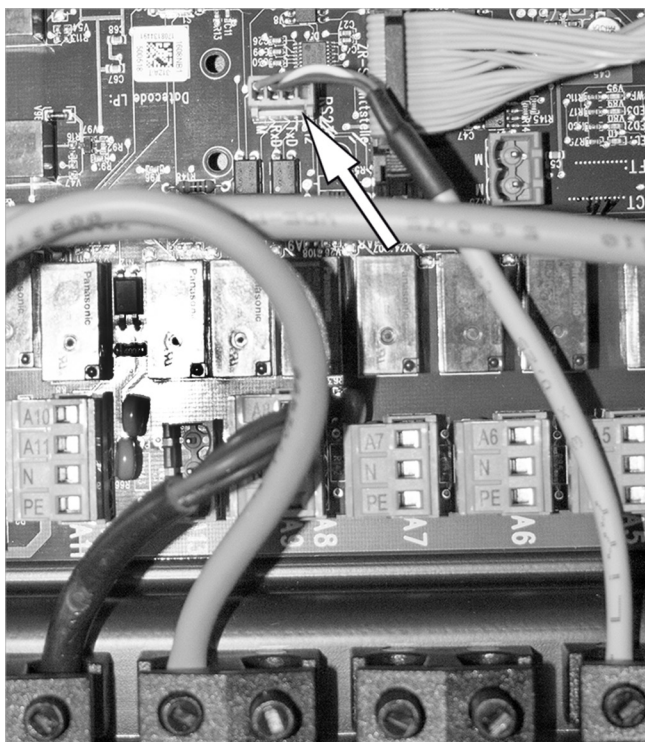
Fig. 71: Conexión del conector de bus
