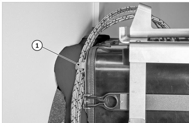
Fig. 67: Fijar las tuberías de gasóleo con la pestaña
