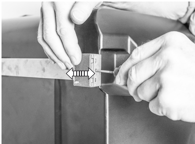
Fig. 97: Reajuste de los rieles de cierre en caso necesario
