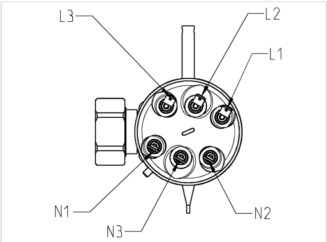
Fig. 155: Conexión del cartucho calefactor
