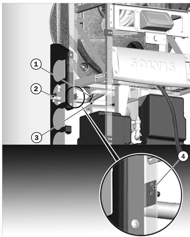
Fig. 23: Conectar el tubo ondulado a la conexión del purgador de aire
