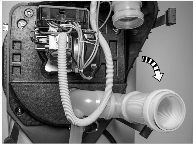
Fig. 91: Doble el tubo de escape hacia abajo.
