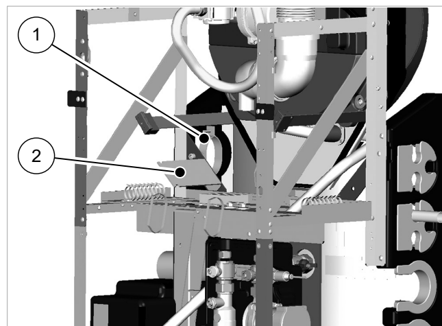
Fig. 107: Montar la abrazadera de tubo y la chapa de sujeción
