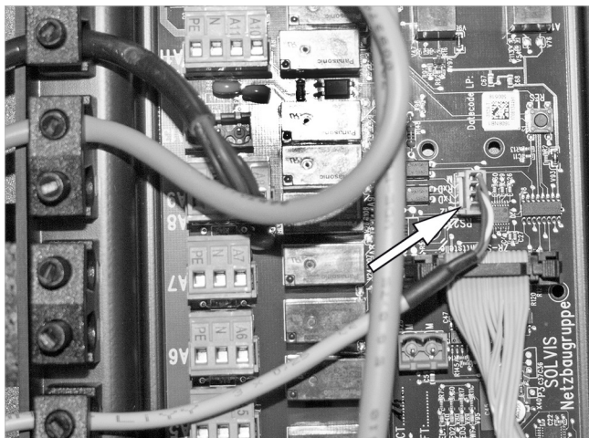
Fig. 48: Conexión del conector de bus
