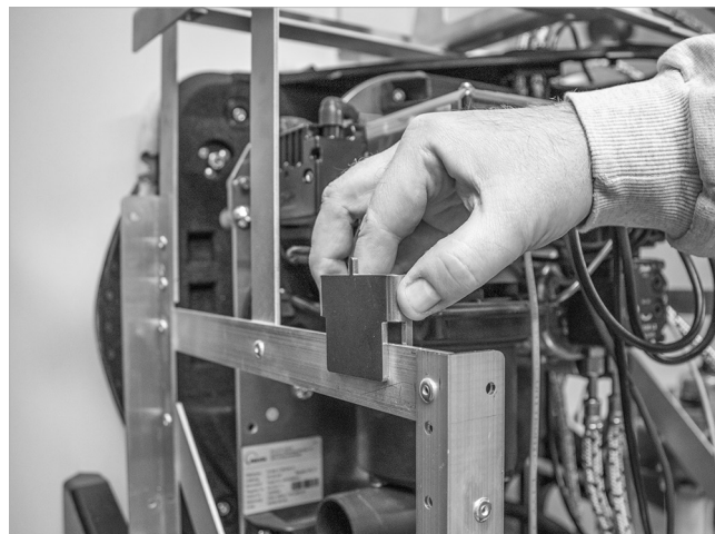
Fig. 138: Enganche del gancho alojador
