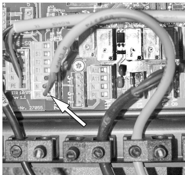
Fig. 76: collegamento della spina del bruciatore a olio ad A 12
