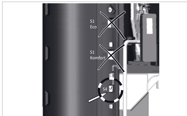
Fig. 24: Montaggio del sensore S4
