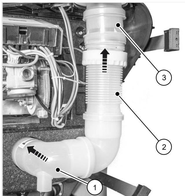
Fig. 80: Gomito di scarico montato
