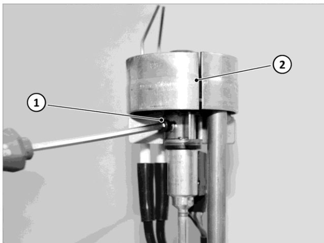
Fig. 147: Testa di miscelazione nel supporto ugello
