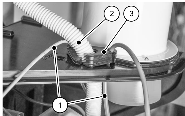
Fig. 56: Passaggio dei cavi sulla camera di aspirazione
