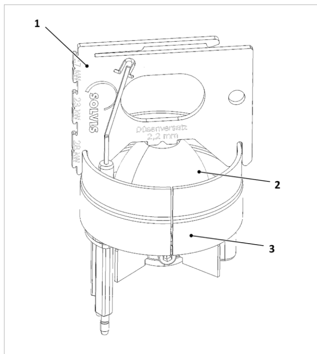
Fig. 149: Testa del miscelatore con calibro applicato
