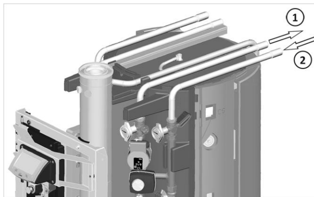
Fig. 36: Attacco H-VL/H-RL da dietro
