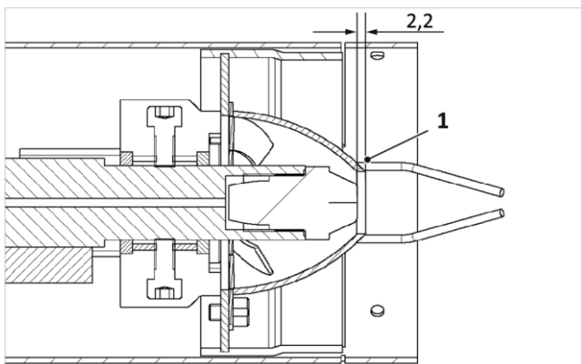
Fig. 148: Sezione attraverso la testa di miscelazione
