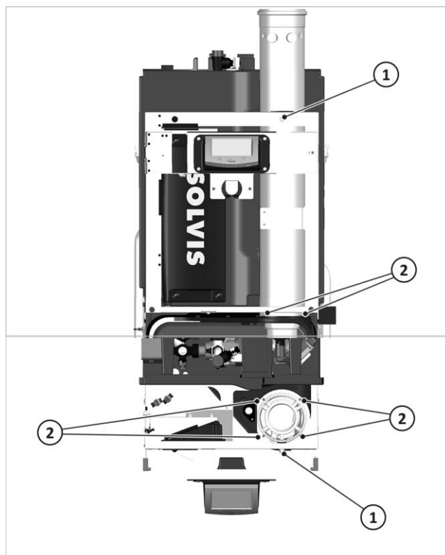
Fig. 6: Allentare le viti, rimuovere il tubo di scarico
