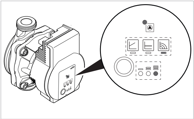
Fig. 123: Impostazione di base (N.giri costante, linea caratteristica III)
