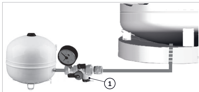
Fig. 116: Rubinetto KFE sul gruppo di collegamento MAG
