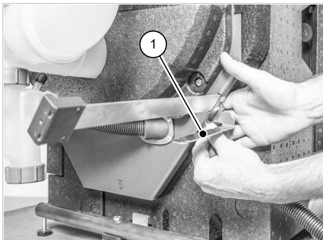
Fig. 89: Montaggio della staffa di fissaggio
