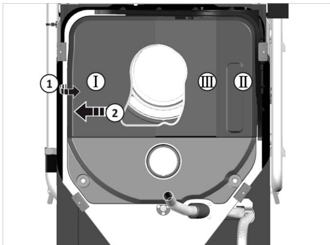
Fig. 47: Smontaggio dell'isolamento della flangia anteriore
