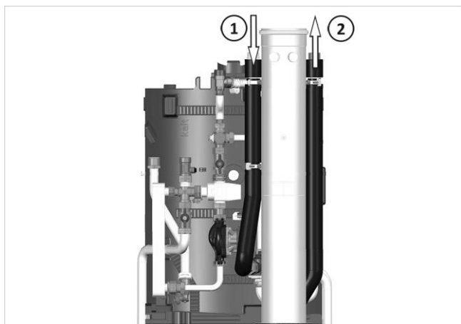
Fig. 42: attacco WP-VL / WP-RL dall'alto
