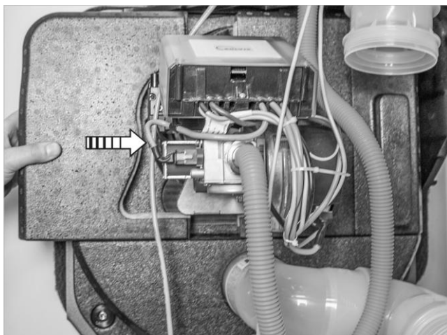
Fig. 100: Montaggio dell'isolamento della flangia anteriore destra (parte I)
