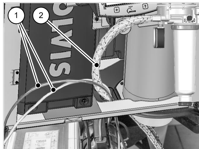
Fig. 75: Passaggio del tubo nella camera di aspirazione
