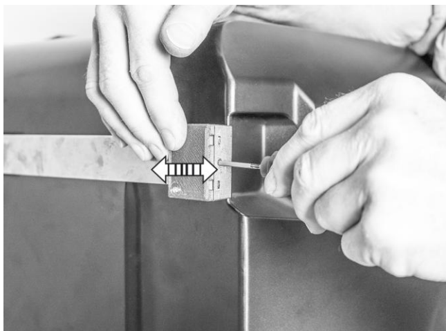
Fig. 103: Regolazione delle guide di bloccaggio se necessario
