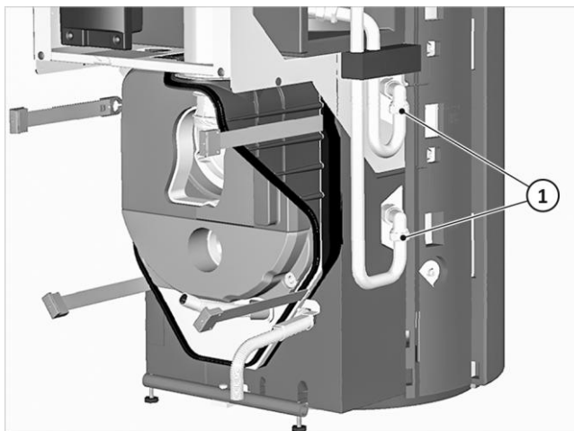
Fig. 33: Controllare/serrare gli attacchi della SCR
