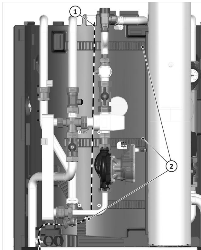
Fig. 105: guida cavi attraverso l'isolamento WWS
