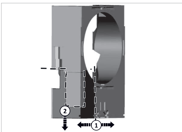
Fig. 11: Estrazione dell'isolamento della flangia
