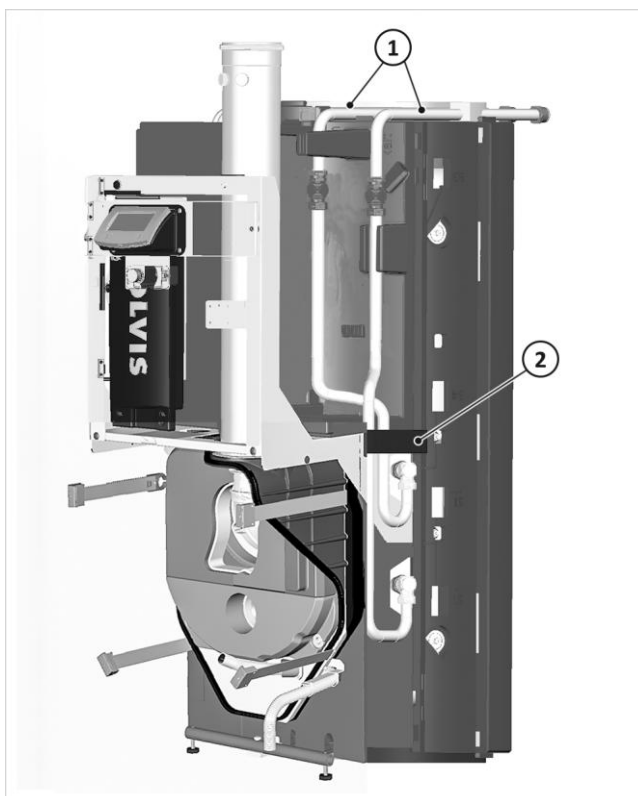
Fig. 40: Tubi posizionati sul retro
