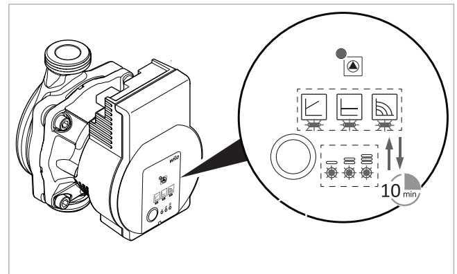
Fig. 122: Indicazione sfiato in funzione
