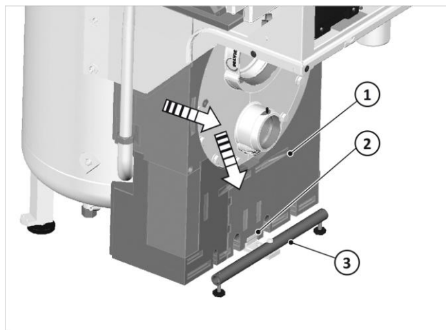
Fig. 9: smontaggio dell'isolamento posteriore della flangia
