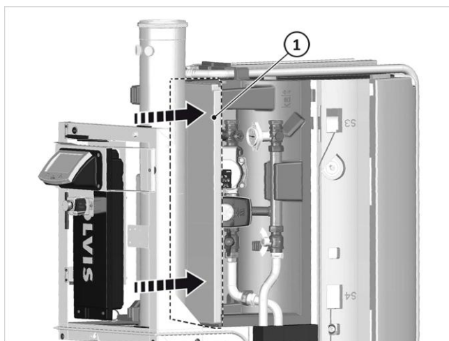
Fig. 114: Inserire il coperchio isolante anteriore della SCR
