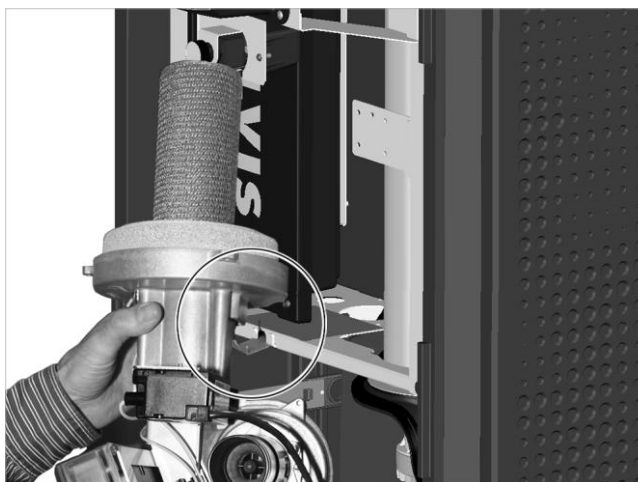
Fig. 142: Aggancio del bruciatore alla console (posizione di manutenzione)
