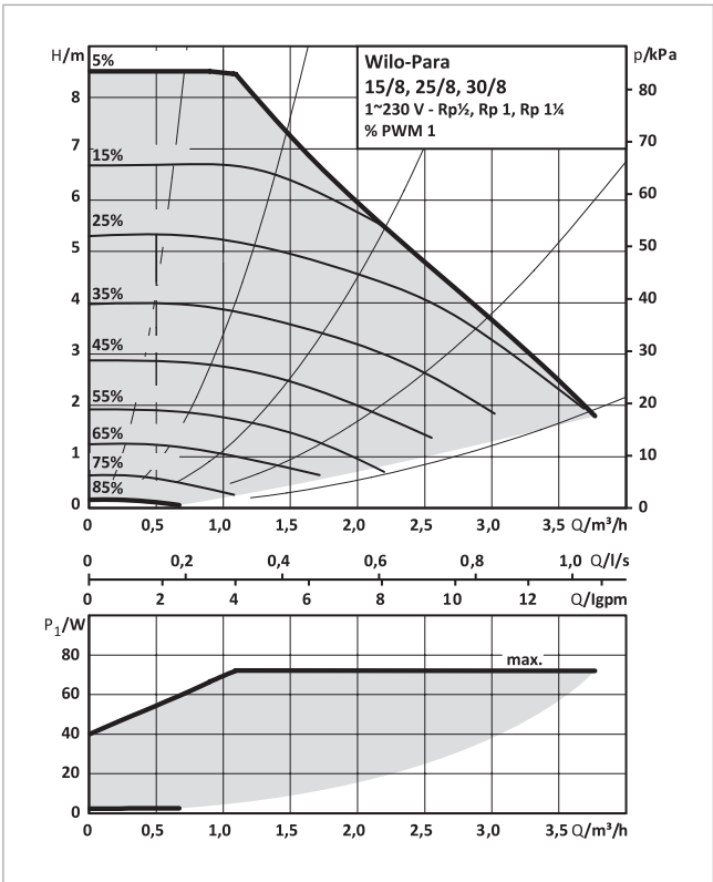
Fig. 155: Curva caratteristica della pompa Wilo-PARA 15/8
