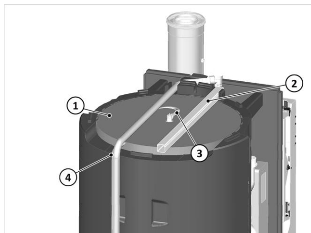
Fig. 20: Posizionare la lamiera circolare di copertura e le canaline guida
