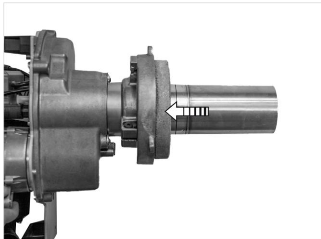
Fig. 64: applicazione del portello caldaia con isolante refrattario
