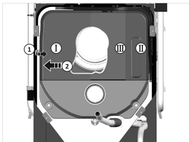
Fig. 7: Smontaggio dell'isolamento anteriore della flangia
