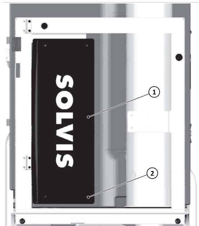
Fig. 115: Fissaggio del coperchio del gruppo di rete
