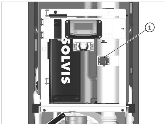
Fig. 69: Fissaggio del supporto del filtro del gasolio
