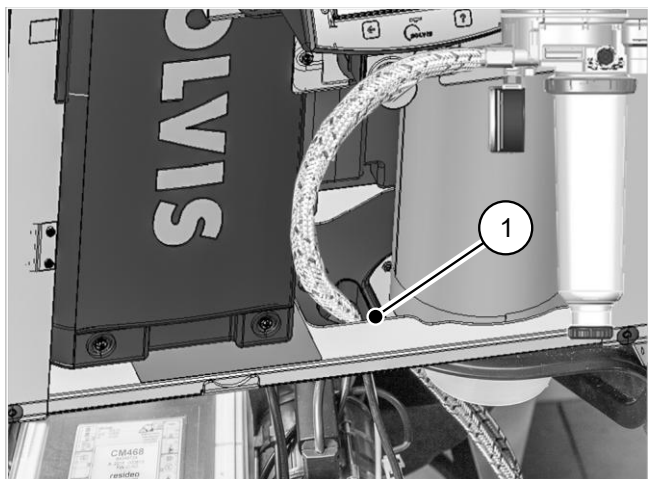
Fig. 71: Passaggio della linea dell'olio alla camera di aspirazione
