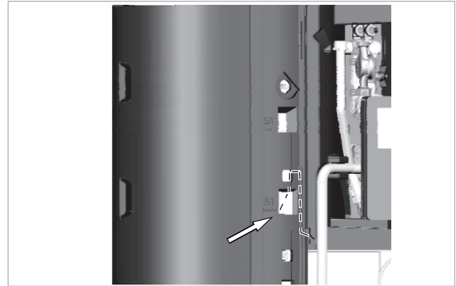
Fig. 26: Montaggio sensore S1 in posizione S1 - Comfort
