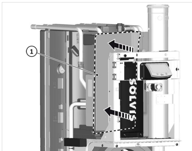
Fig. 113: Inserire il coperchio isolante anteriore della SAC
