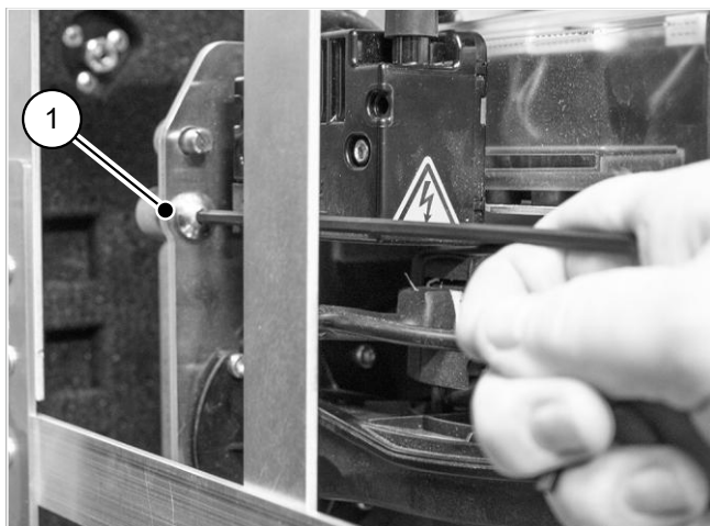
Fig. 145: Viti a serraggio rapido nell'inserto del bruciatore
