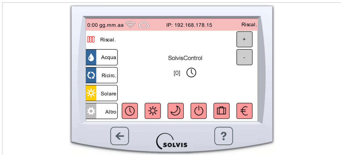
Fig. 153: SolvisControl con menu "Riscaldamento" (un circuito di riscaldamento)
