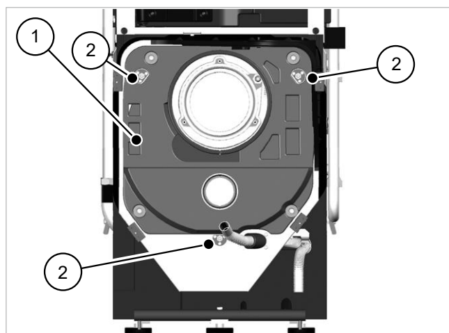
Fig. 14: Montaggio del pannello posteriore della camera di aspirazione
