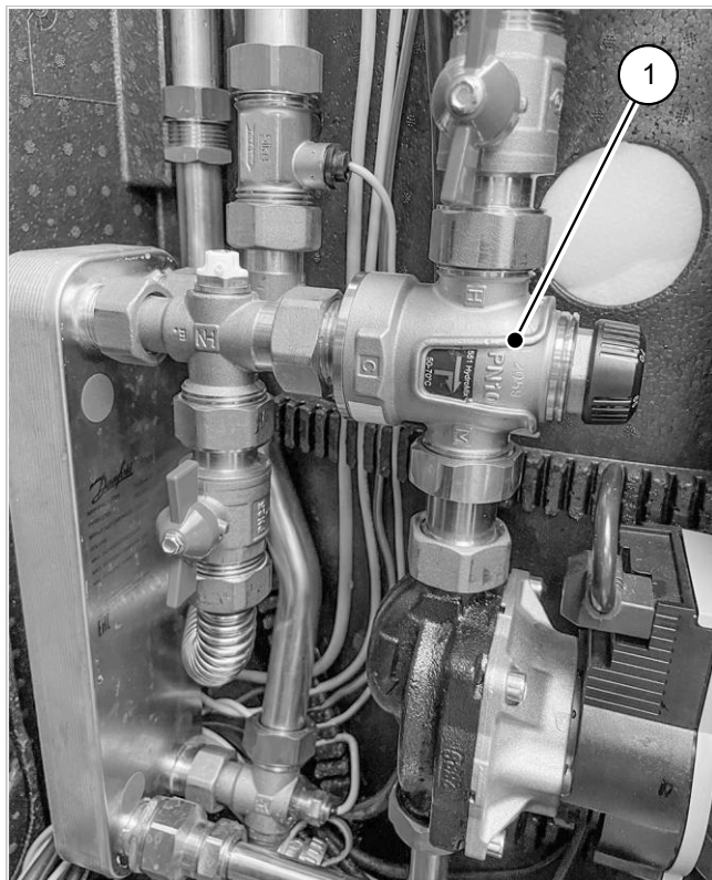
Fig. 117: Valvola di miscelazione termica (1) SolvisBen in WWS
