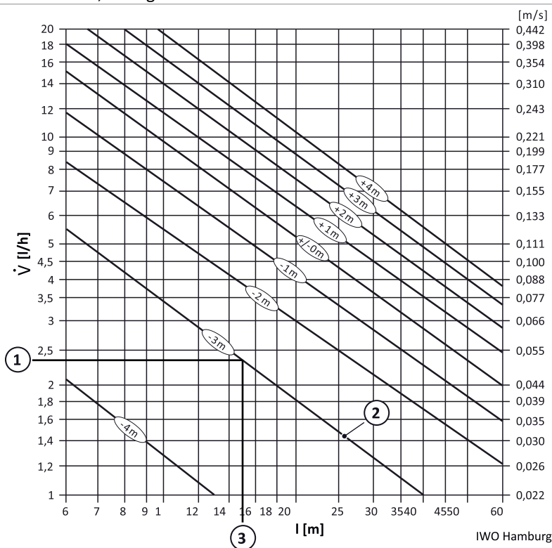
Fig. 78: Lunghezza massima della tubazione nel sistema a linea unica in funzione della prevalenza
