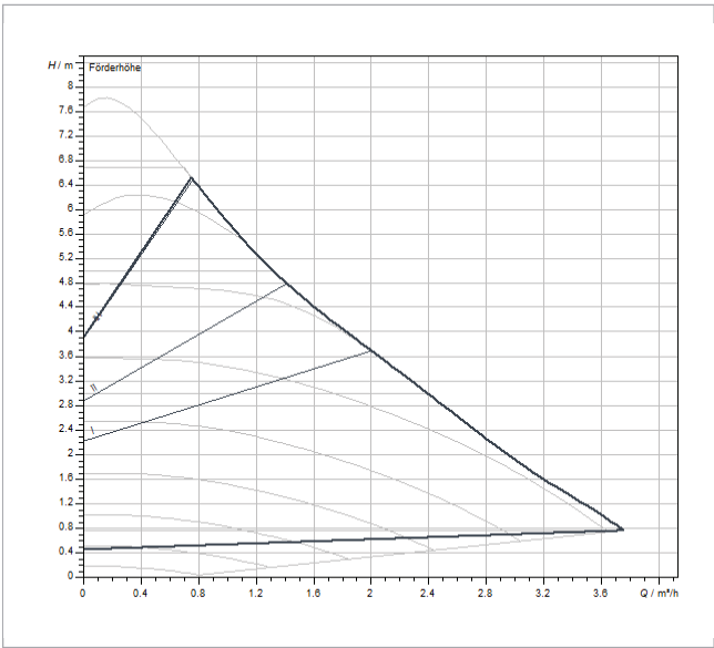
Fig. 156: Curve caratteristiche della pompa Varios PICO-STG 15/1-7
