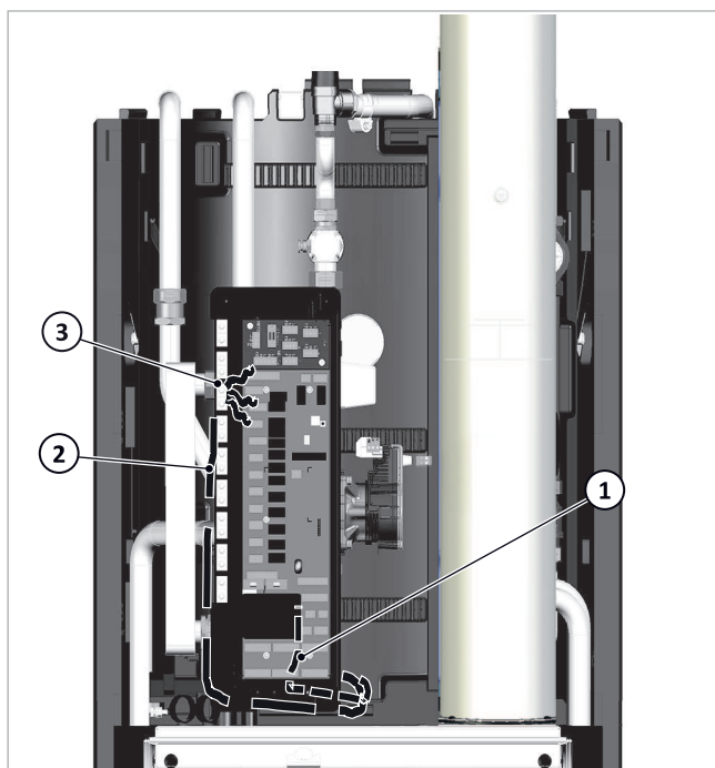
Fig. 106: posizionamento della scheda di rete
