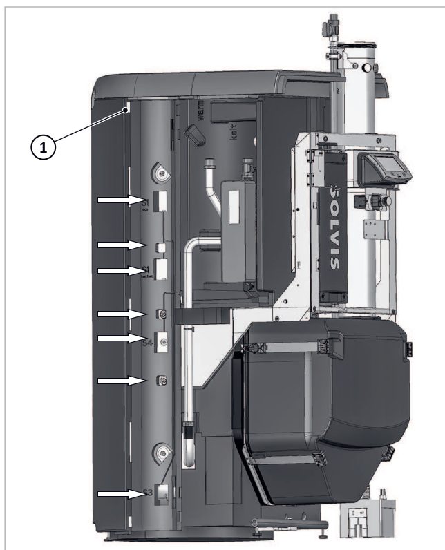
Fig. 134: Tappi in non tessuto lato sinistro
