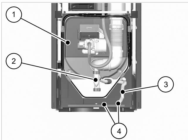
Fig. 91 : Linea di scarico della condensa senza pompa di condensa
