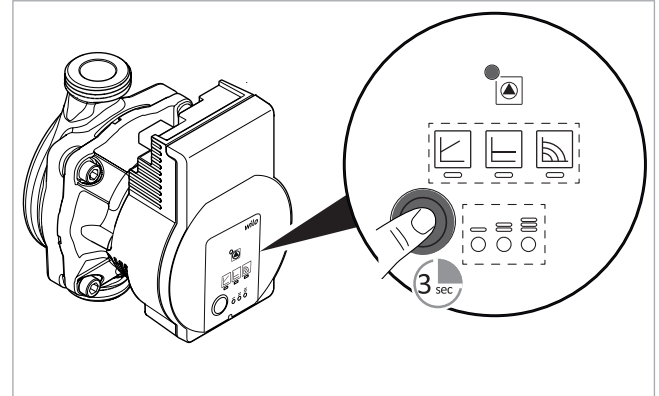
Fig. 121: iniziare l'operazione di sfiato
