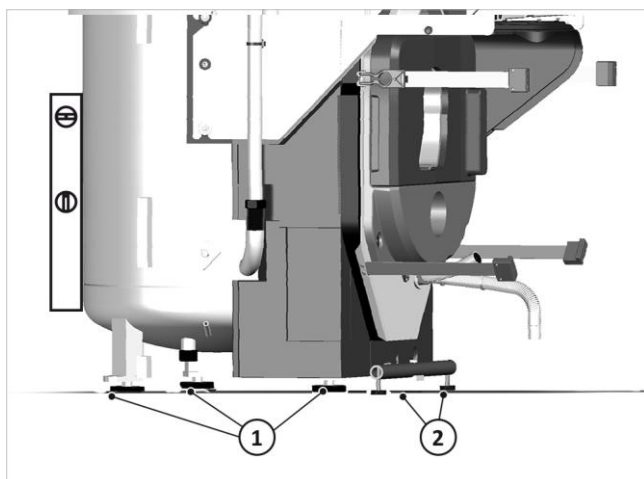
Fig. 5: installazione dell'accumulatore
