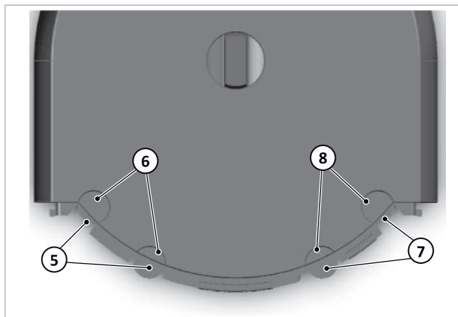
Fig. 125: Taglio dei passaggi delle tubazioni
