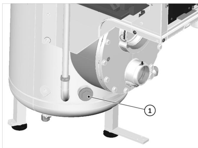
Fig. 10: Raccordo per riscaldatore elettrico a immersione
