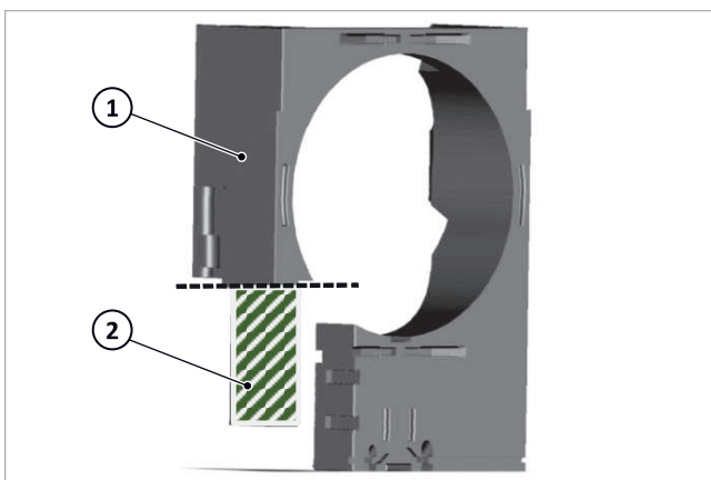
Fig. 12: Taglio dell'isolamento della flangia
