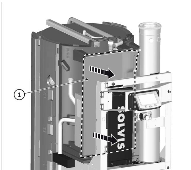
Fig. 27: Rimuovere il coperchio isolante anteriore della SAC
