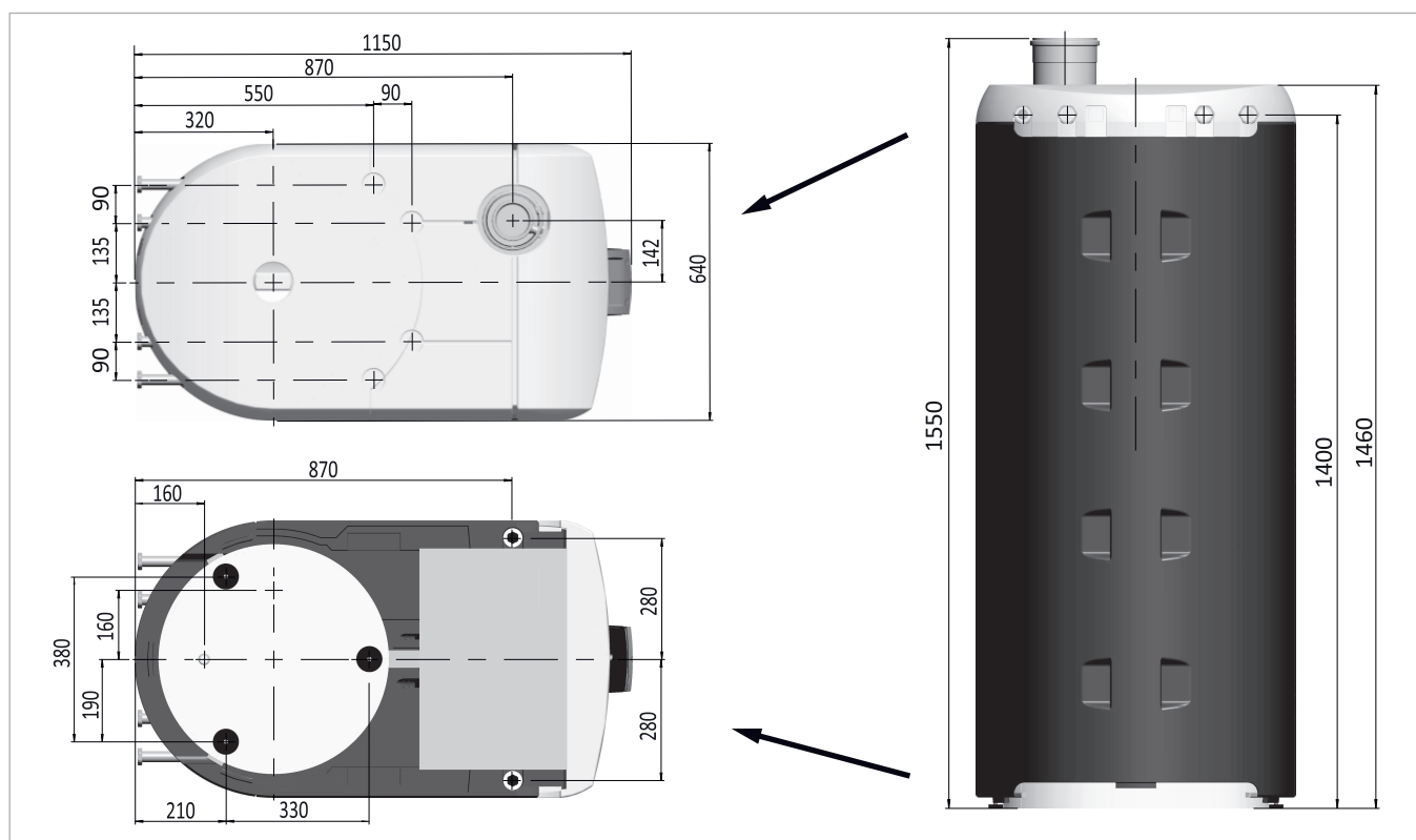
Fig. 152: Panoramiche SolvisBen (tutte le dimensioni in cm)
