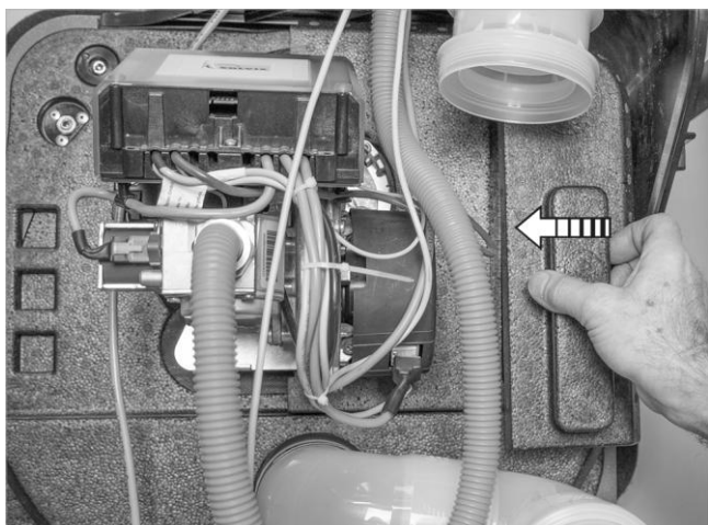
Fig. 99: Montaggio dell'isolamento della flangia anteriore destra (parte III)
