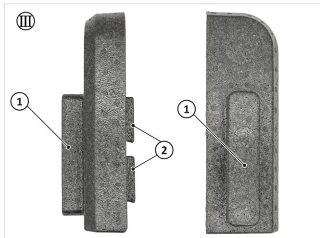
Fig. 96: Isolamento della flangia anteriore (III) con molle di bloccaggio
