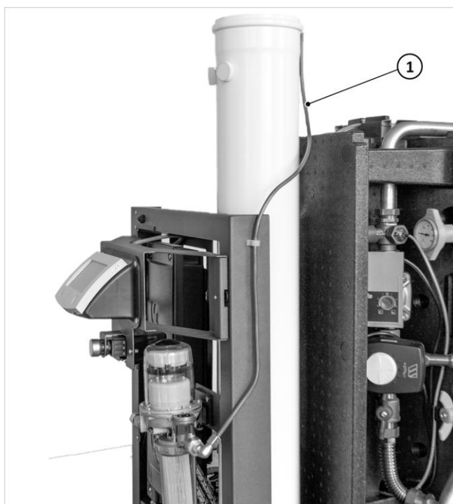
Fig. 72: Collegamento delle linee di alimentazione dell'olio
