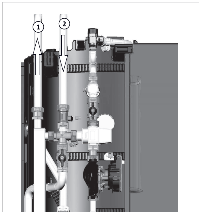
Fig. 30: attacco TWW/TWK dall'alto
