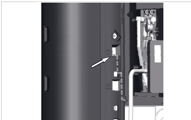
Fig. 25: Montaggio sensore S1 in posizione S1 - Eco
