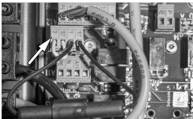
Fig. 59: Inserire la presa di collegamento
