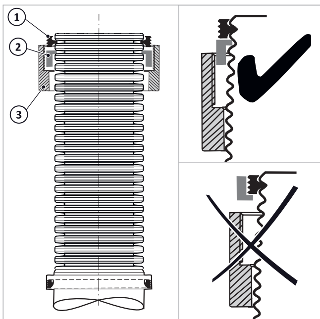
Fig. 84: Avvitamento infilato sul tubo flessibile
