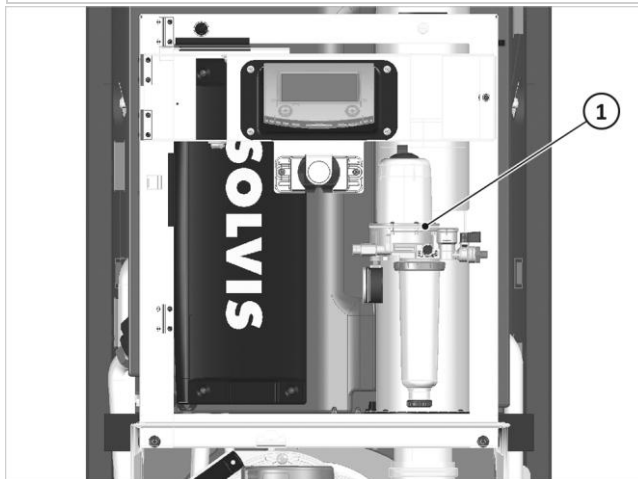
Fig. 70: Filtro del gasolio inserito nel supporto
