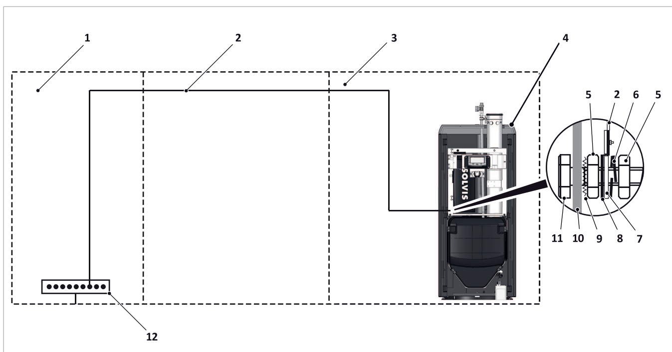
Fig. 107: Compensazione di potenziale di SolvisBen
