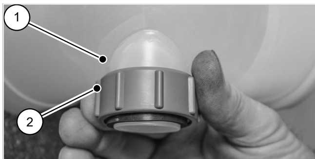
Fig. 87: Fissare il dado di raccordo e l'anello elastico
