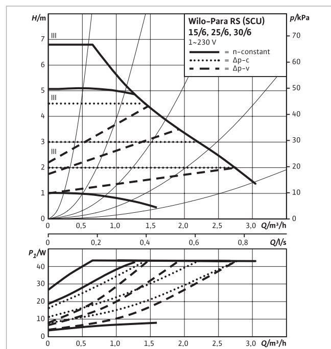
Fig. 154: Curva caratteristica della pompa Wilo-Para 15/6 SCU
