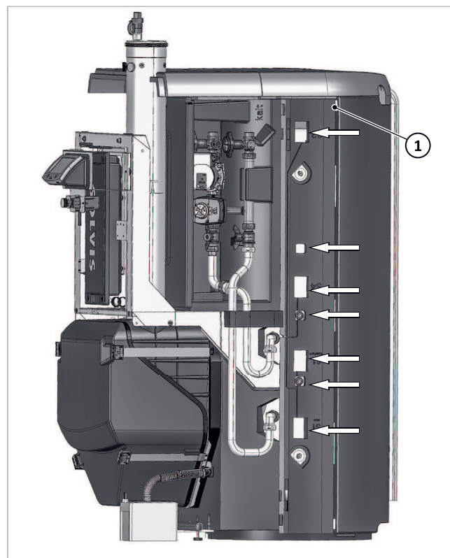
Fig. 133: Tappi in non tessuto lato destro
