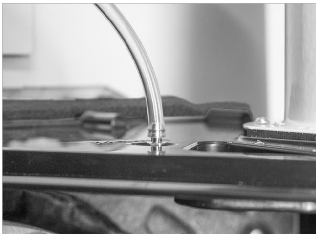
Fig. 68: Nipplo vapore olio montato
