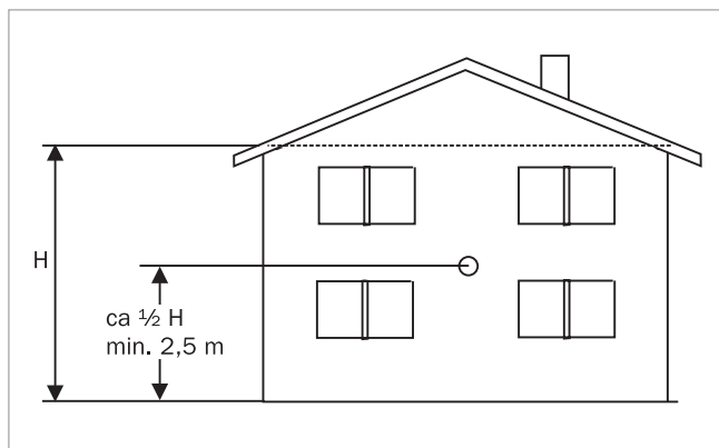
Fig. 108: Posizione del sensore esterno
