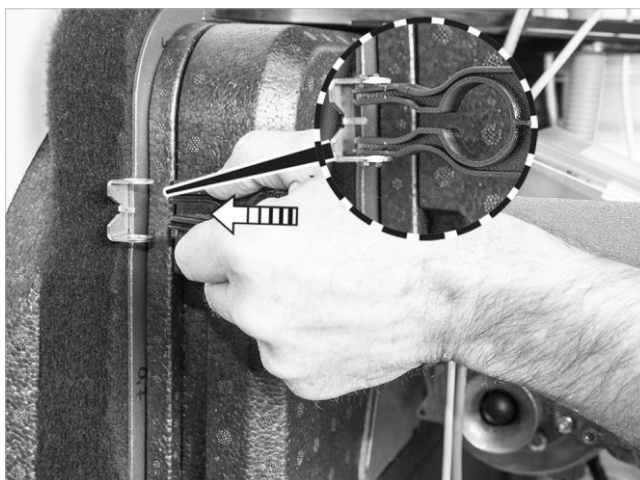
Fig. 101: Montaggio della guida
