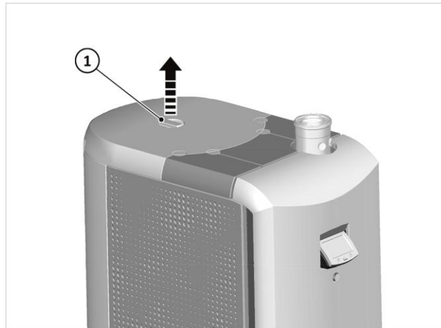
Fig. 140: Estrarre il coperchio di sfiato
