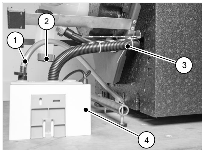
Fig. 92: Pompa della condensa collegata
