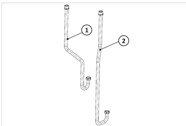
Fig. 39: attacco H-VL (1) / H-RL (2) per HKS esterna
