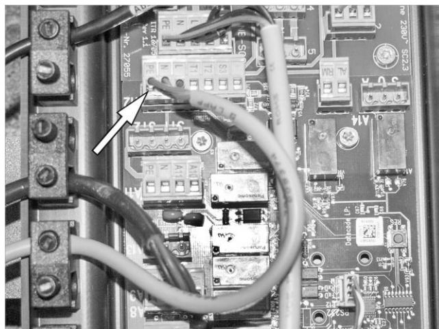
Fig. 57: Collegamento della spina del bruciatore a gas a A 12
