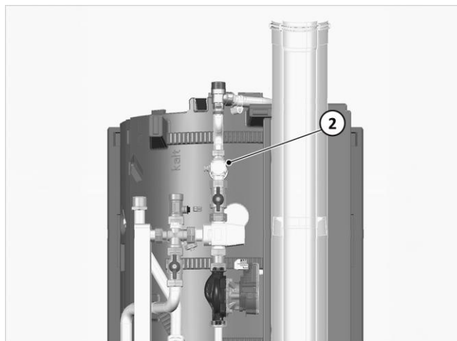
Fig. 29: Controllare/serrare il raccordo a vite della mandata
