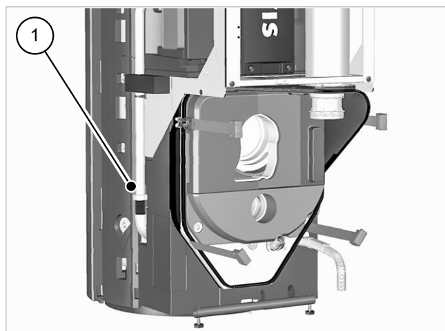
Fig. 28: Controllare/serrare il raccordo a vite del ritorno
