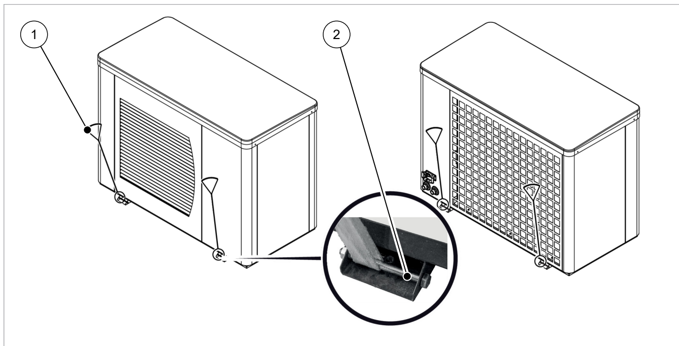
Abb. 3: Tragegurte mit Schrauben/Muttern an SolvisPia befestigen
