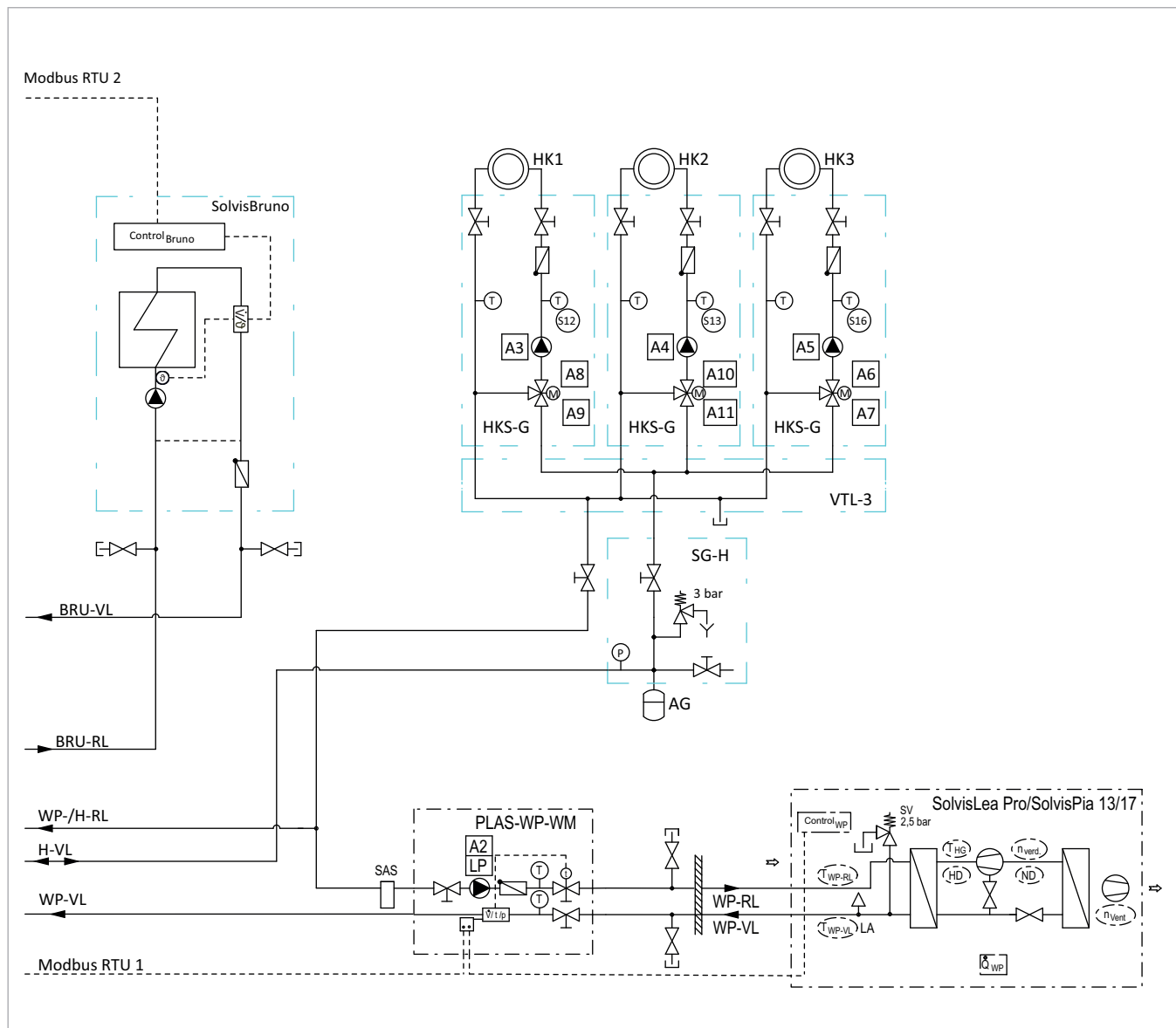
Abb. 37 Anlagenschema SolvisMax Solo mit SolvisBruno, drei Heizkreise und Wärmepumpe - Teil 2 von 2
