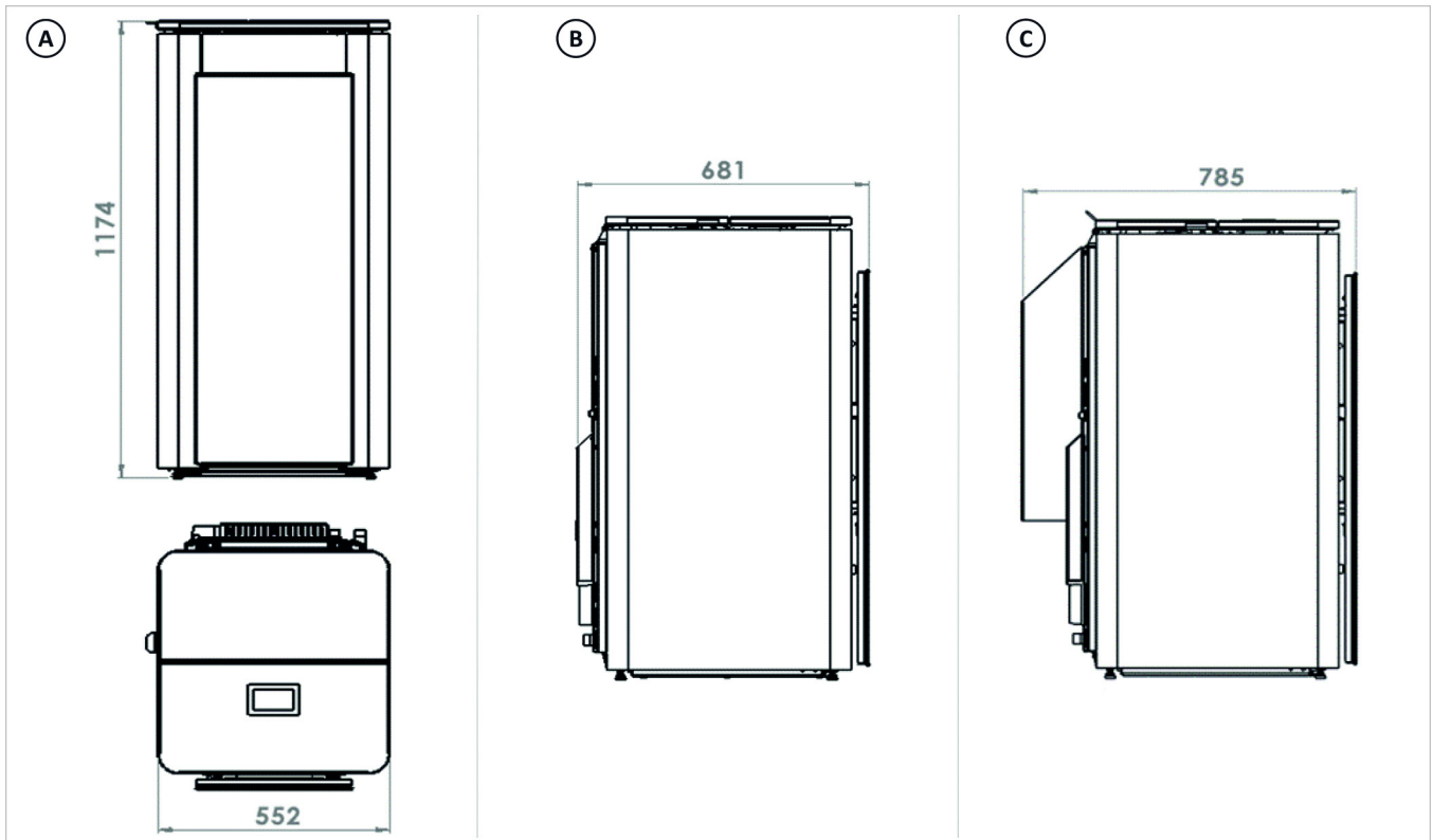
Abb. 30: Maße SolvisBruno (A) Höhe und Breite, (B) Tiefe ohne Saugfördersystem, (C) Tiefe mit Saugfördersystem
