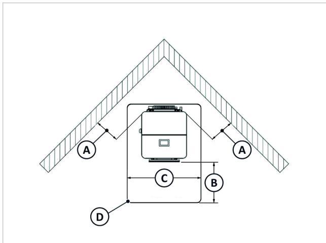
Abb. 4: Mindestabstände Bruno bei Aufstellung schräg in Wohnraumecke
