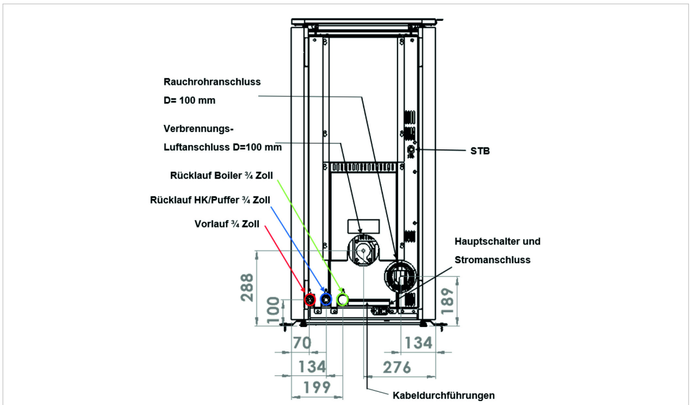
Abb. 31: Rückseite SolvisBruno mit Abmessungen Rohrleitungen und Stromanschluss
