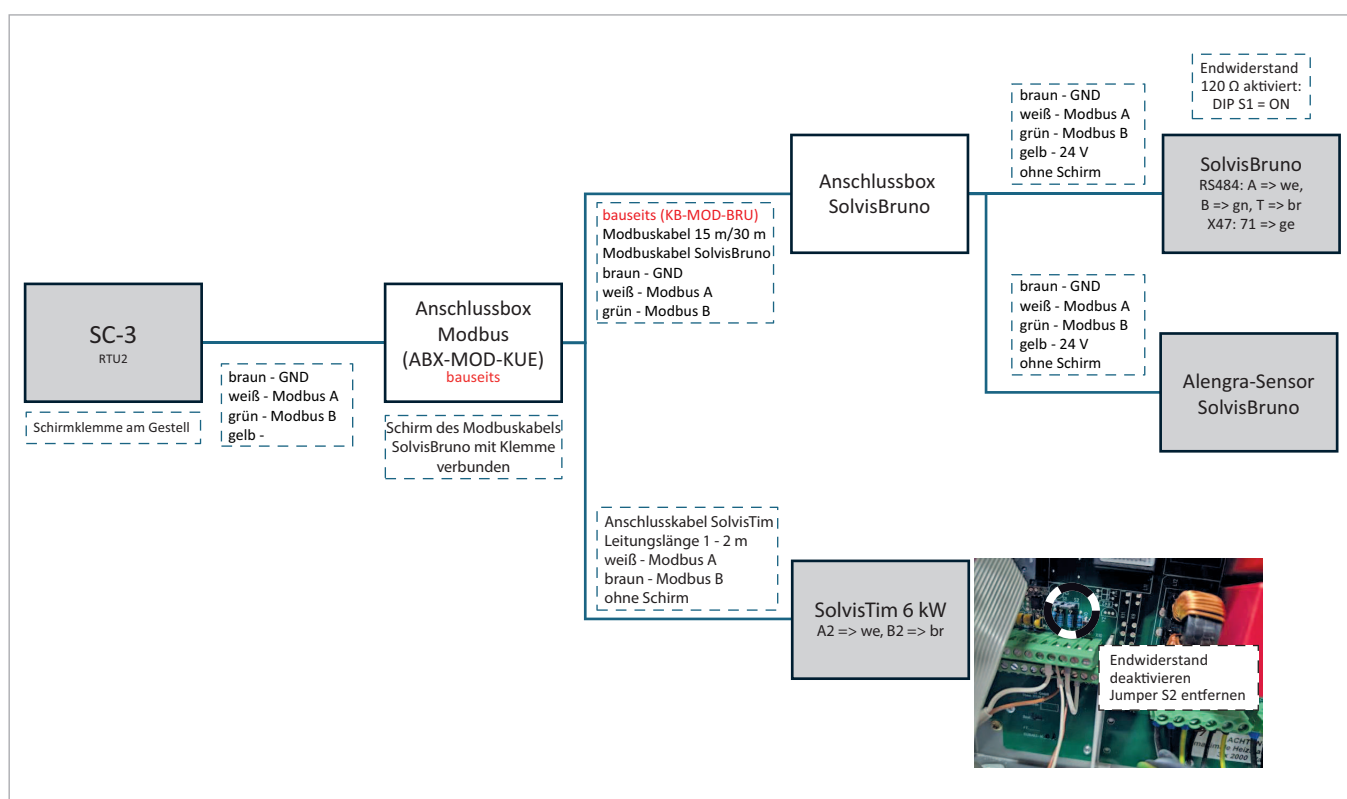
Abb. 45: Schematische Darstellung des Modbus-Anschlusses von SolvisBruno und SolvisTim 6 kW
