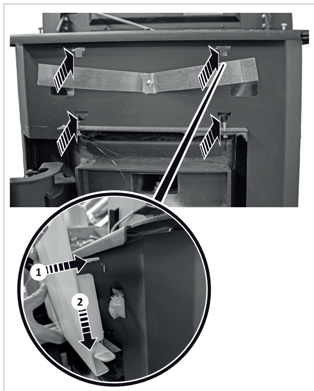
Abb. 7: Verkleidung oberhalb der Brennraumtür montieren
