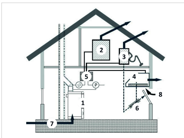
Abb. 14: Gemeinsamer Betrieb von Abluftanlagen und raumluftabhängiger Feuerstätte
