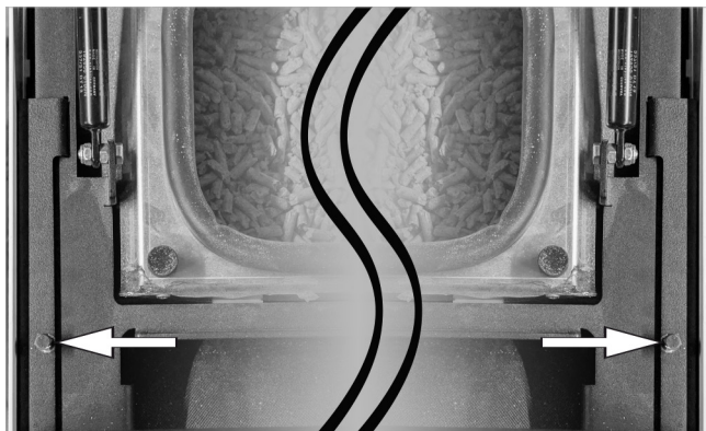
Abb. 10: Seitliche Verkleidungen festschrauben
