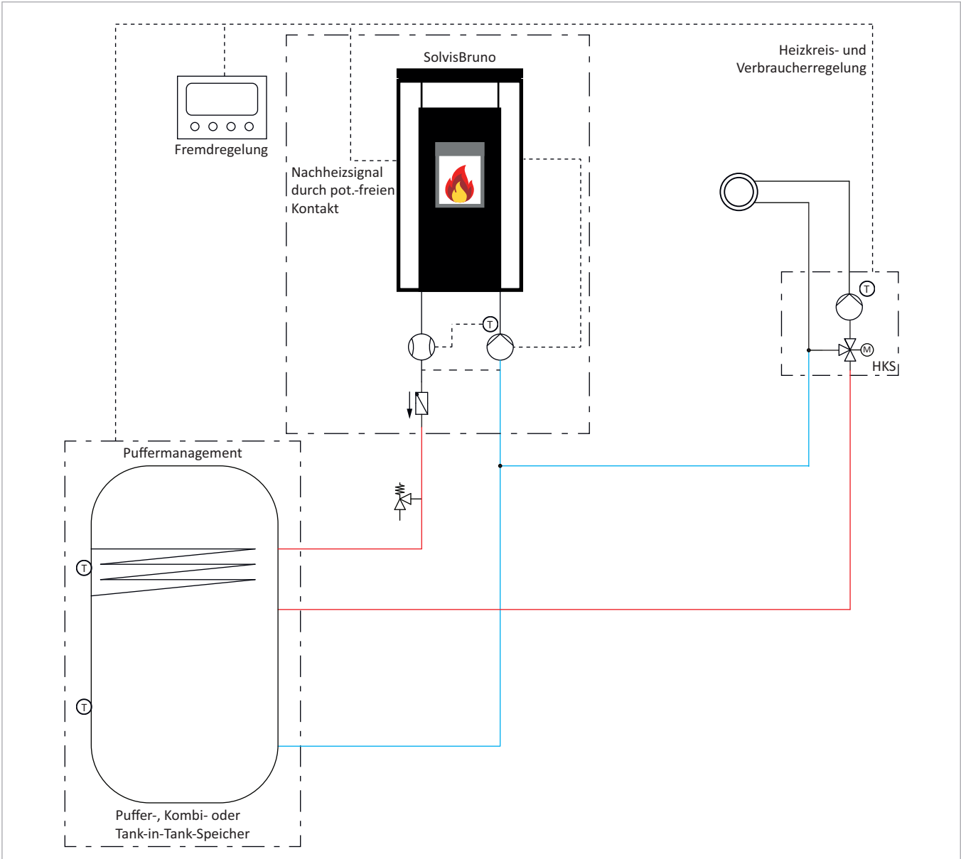
Abb. 48: Anlagen mit Pufferspeicher, Kombispeicher oder Tank-in-Tank-Speicher und Fremdregelung
