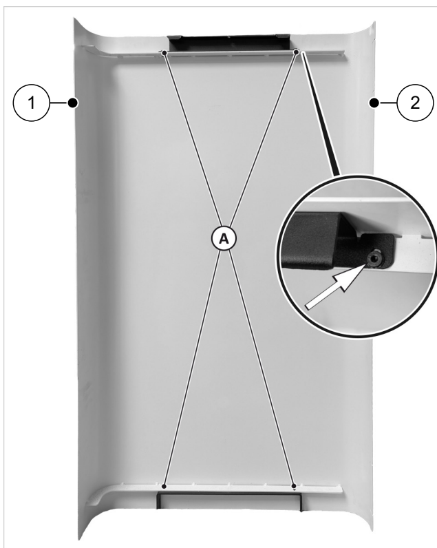
Abb. 11: Position der Schrauben/Langlöcher auf der Innenseite der Seitenverkleidungen
