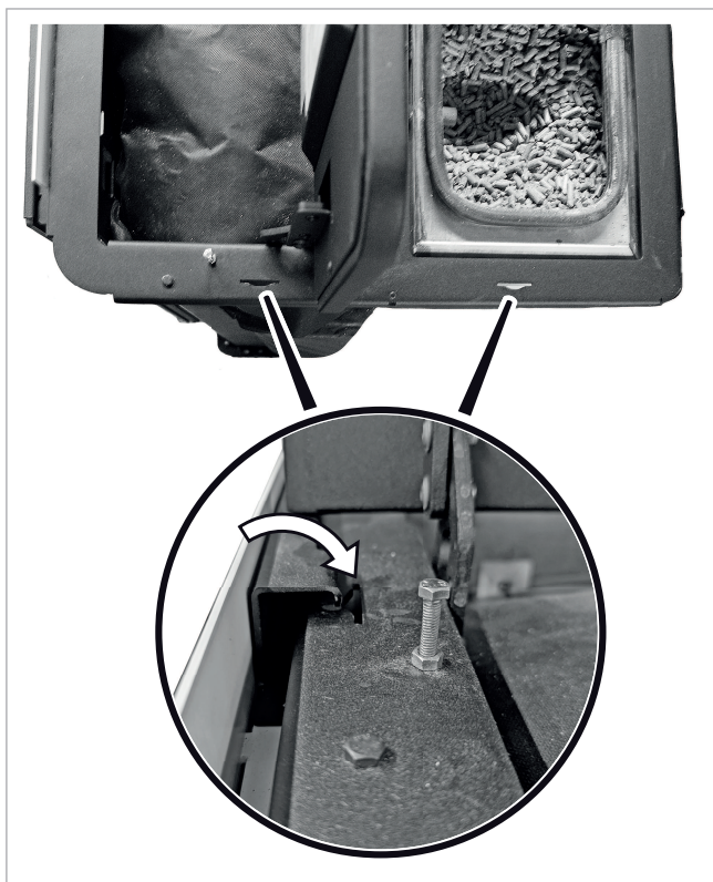
Abb. 9: Seitliche Verkleidungen montieren - oberer Rahmen
