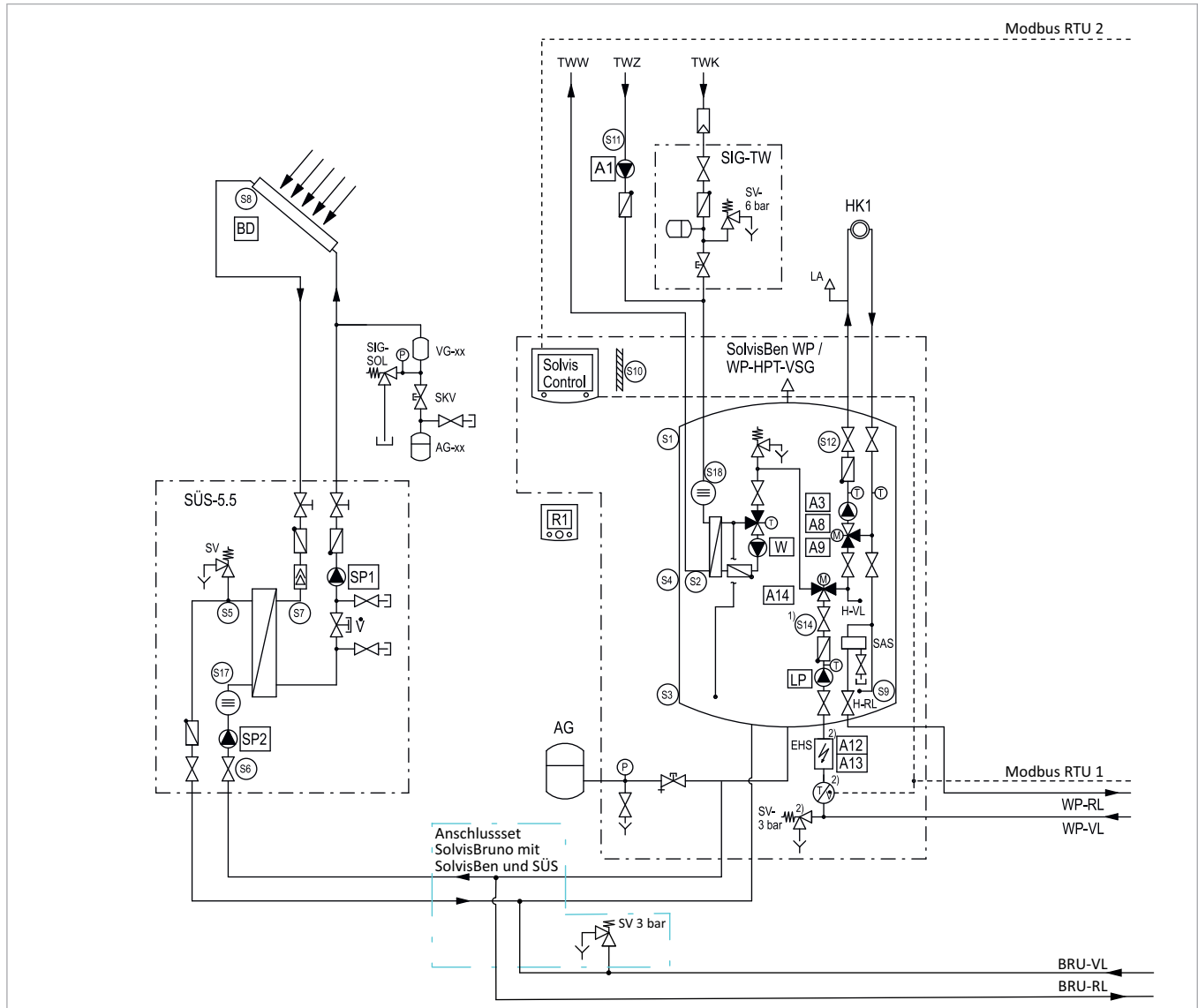
Abb. 34 Anlagenschema SolvisBen WP mit SolvisBruno, ein Heizkreis, Wärmepumpe und Solar - Teil 1 von 2
