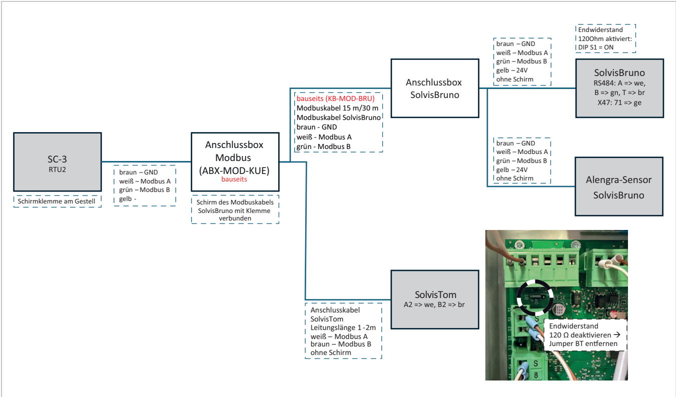
Abb. 46: Schematische Darstellung des Modbus-Anschlusses von SolvisBruno und SolvisTom 9 kW
