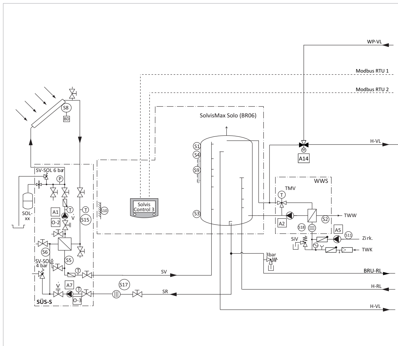
Abb. 40 Anlagenschema SolvisMax Solo der Baureihe 6 mit SolvisBruno, drei Heizkreise und Wärmepumpe - Teil 1 von 2
