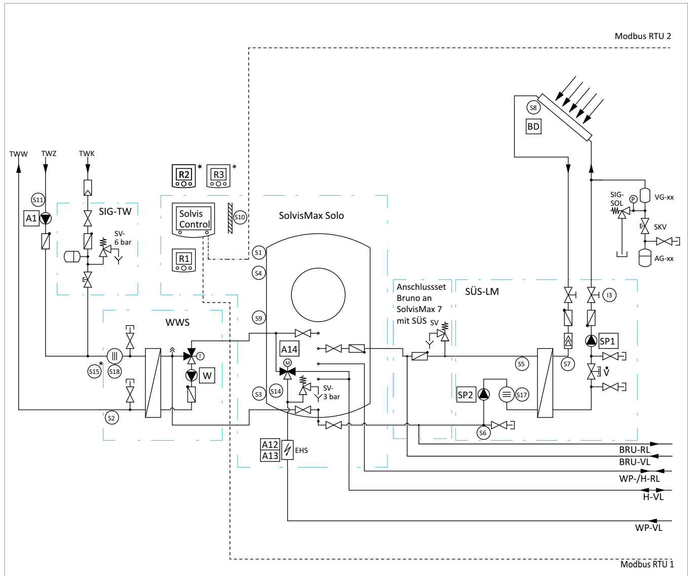
Abb. 38 Anlagenschema SolvisMax 7 mit SolvisBruno, drei gemischte Heizkreise, Wärmepumpe und Solar - Teil 1 von 2
