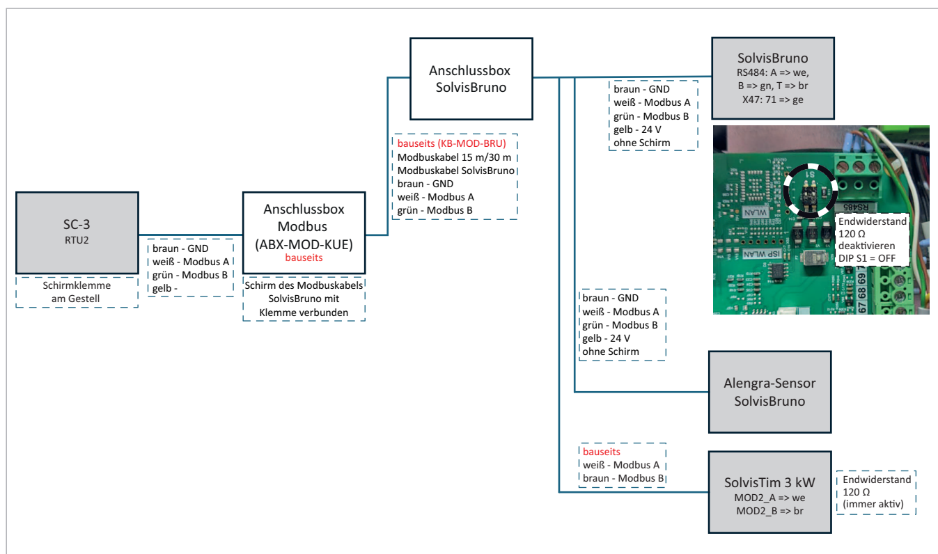
Abb. 44: Schematische Darstellung des Modbus-Anschlusses von SolvisBruno und SolvisTim 3 kW
