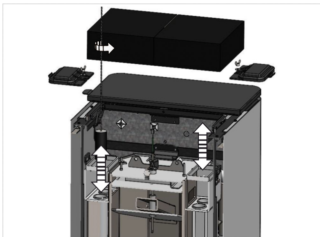
Abb. 23: Vier Wärmetauscher-Rohre reinigen
