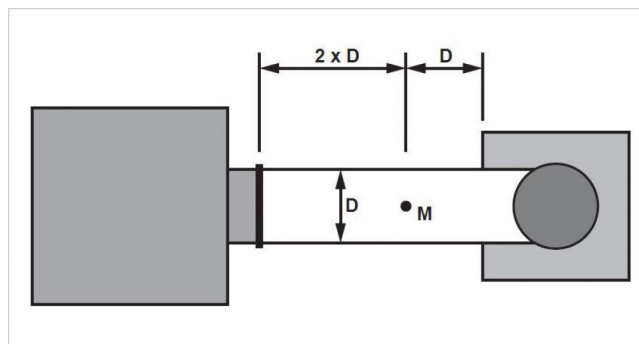
Abb. 15: Schematische Darstellung zur Ausführung/Platzierung der Messöffnung
