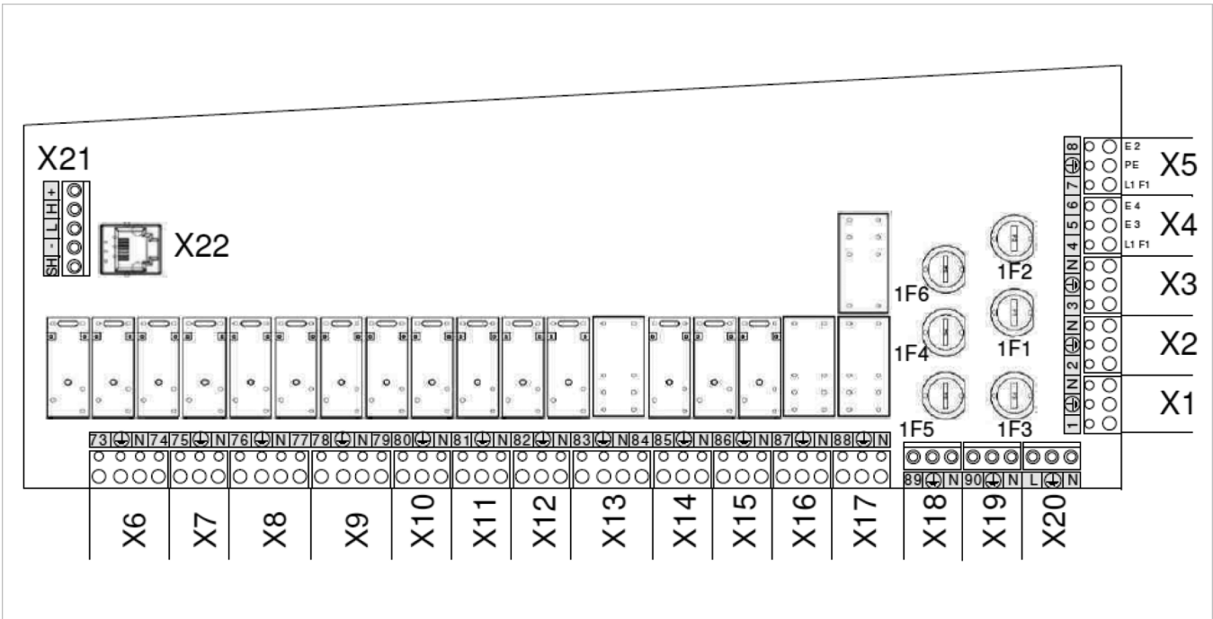
Abb. 42: Integrierte Regelungsplatine SolvisBruno - Aktoren
