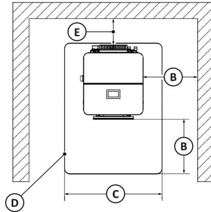
Abb. 5: Mindestabstände SolvisBruno bei Aufstellung dreiseitig von Wänden umgeben
