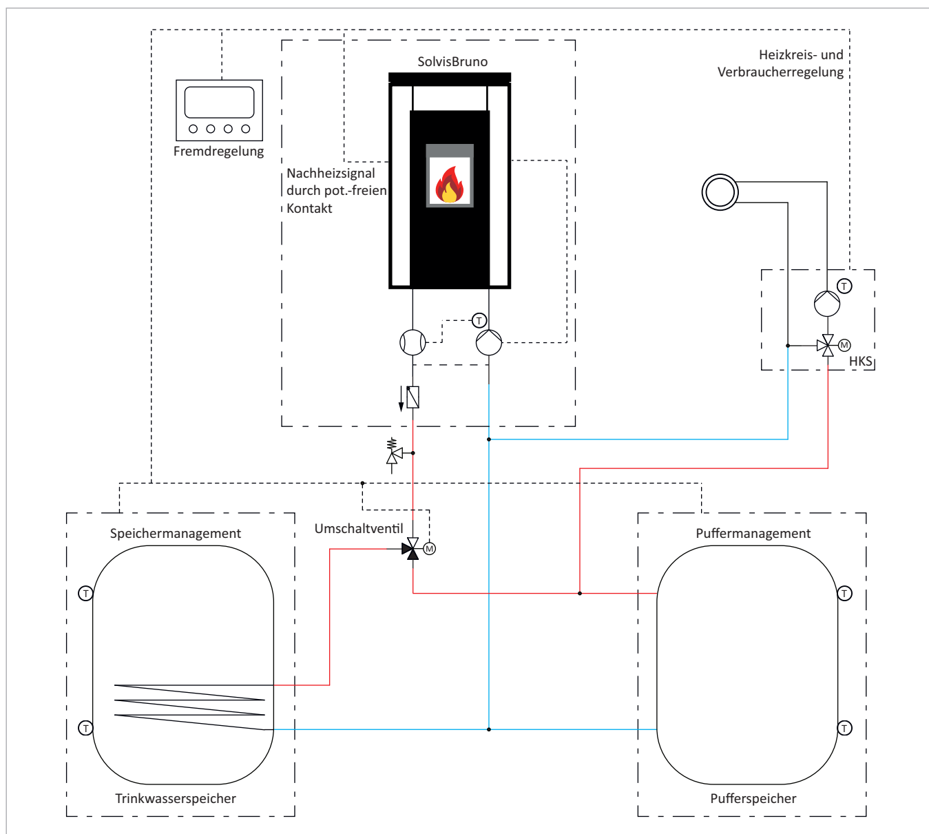
Abb. 49: Kombination aus Pufferspeicher und Warmwasserspeicher und Fremdregelung
