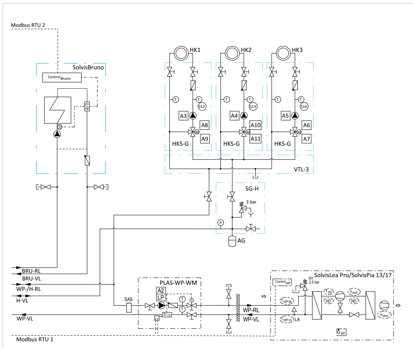
Abb. 39 Anlagenschema SolvisMax 7 mit SolvisBruno, drei gemischte Heizkreise, Wärmepumpe und Solar - Teil 2 von 2
