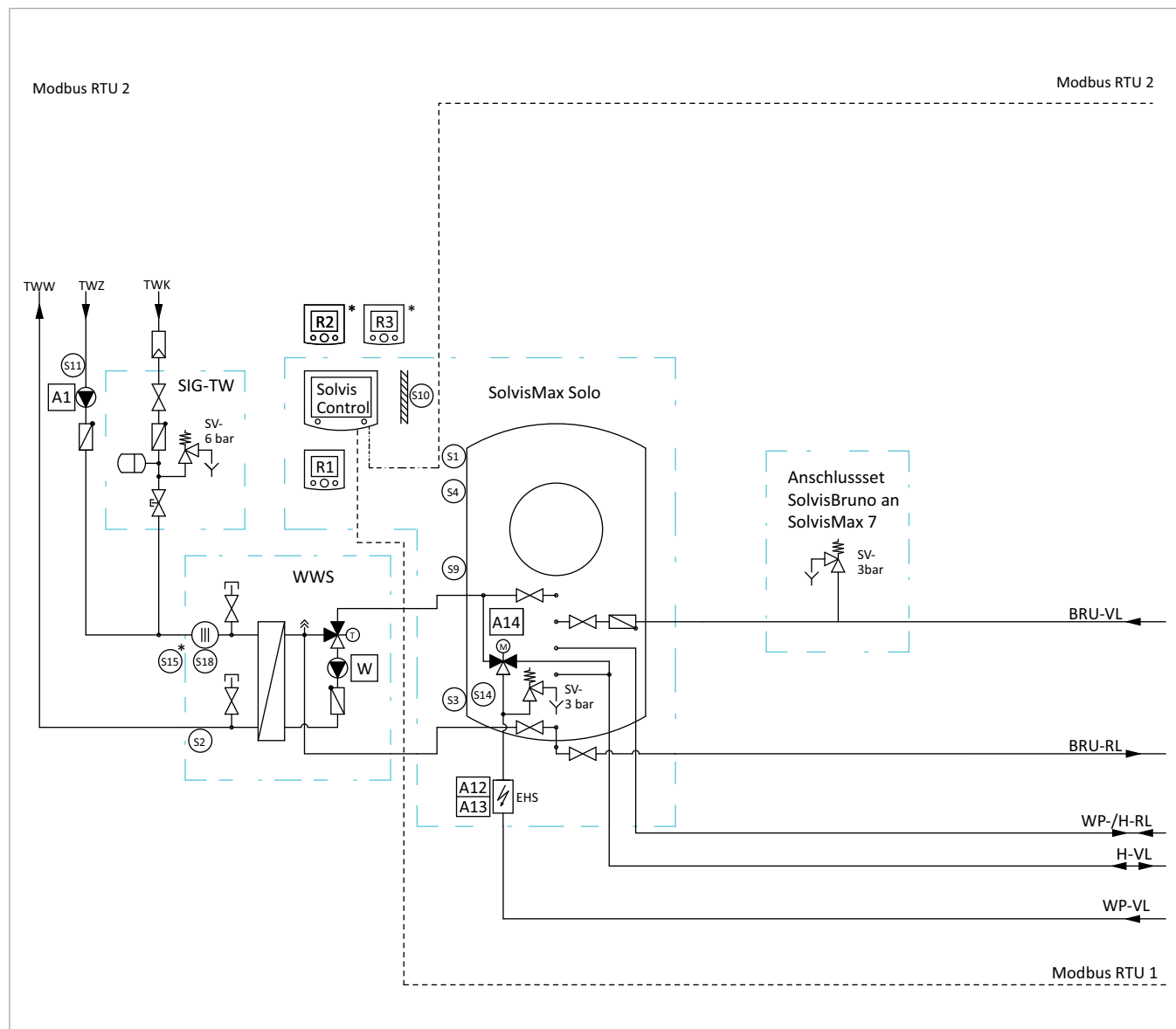
Abb. 36 Anlagenschema SolvisMax Solo mit SolvisBruno, drei Heizkreise und Wärmepumpe - Teil 1 von 2
