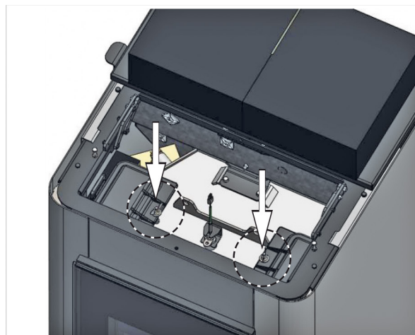
Abb. 22: Flügelmuttern der Wärmetauscher-Abdeckungen lösen
