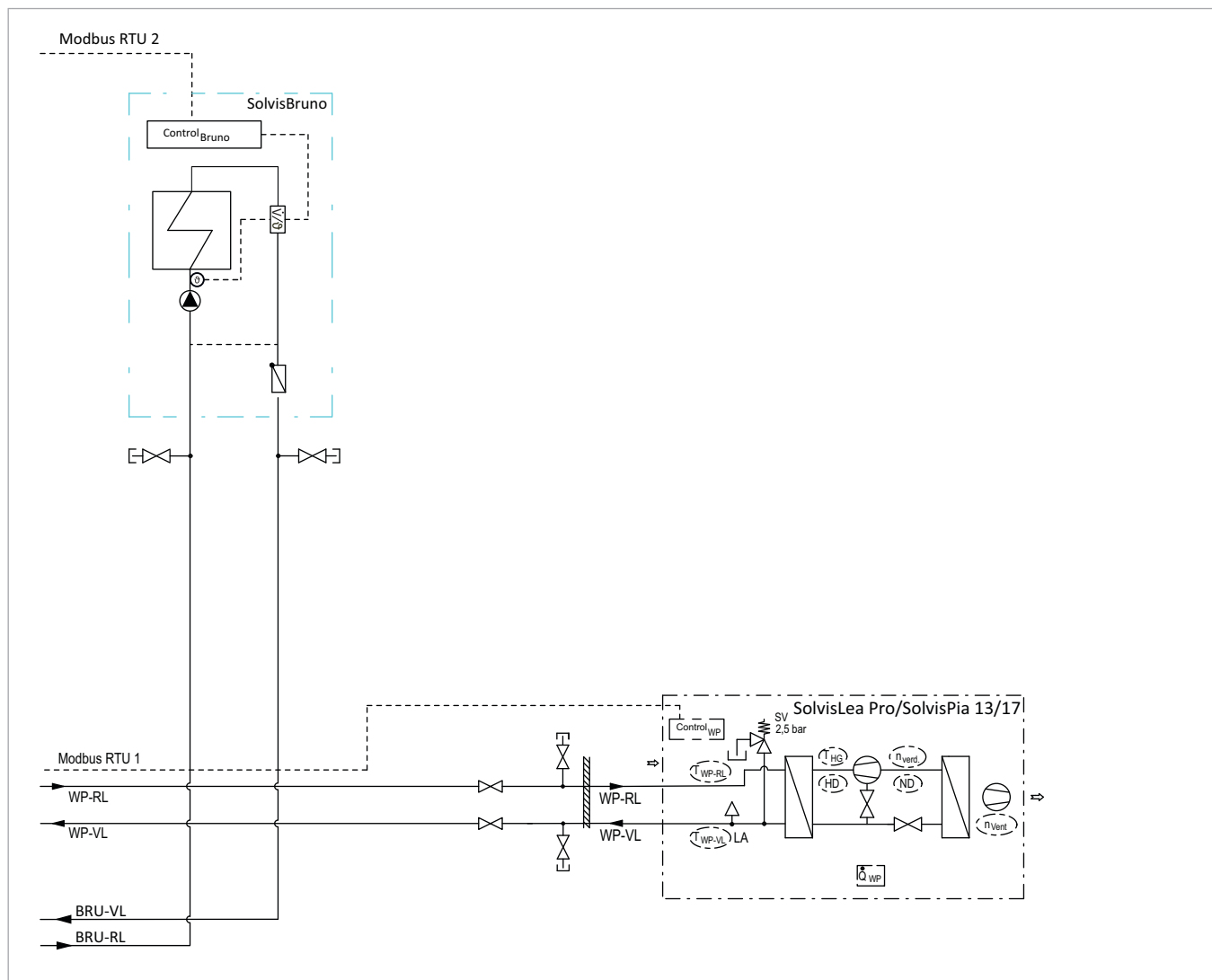
Abb. 33 Anlagenschema SolvisBen WP mit SolvisBruno, ein Heizkreis und Wärmepumpe - Teil 2 von 2
