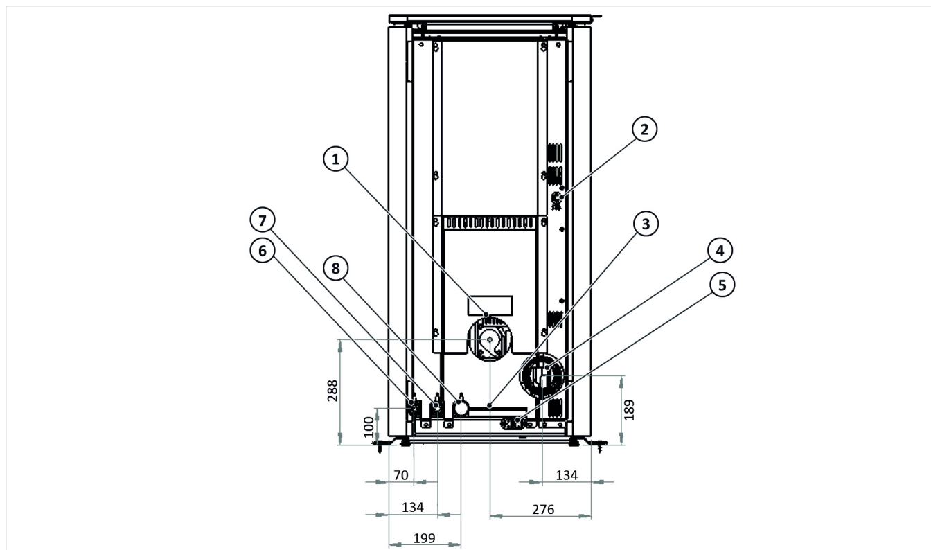
Abb. 13: Anschlusszuordnung SolvisBruno (Rückseite)
