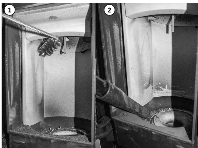
Abb. 26: Innenwände der Brennkammer mit Reinigungsbürste/Aschesauger reinigen
