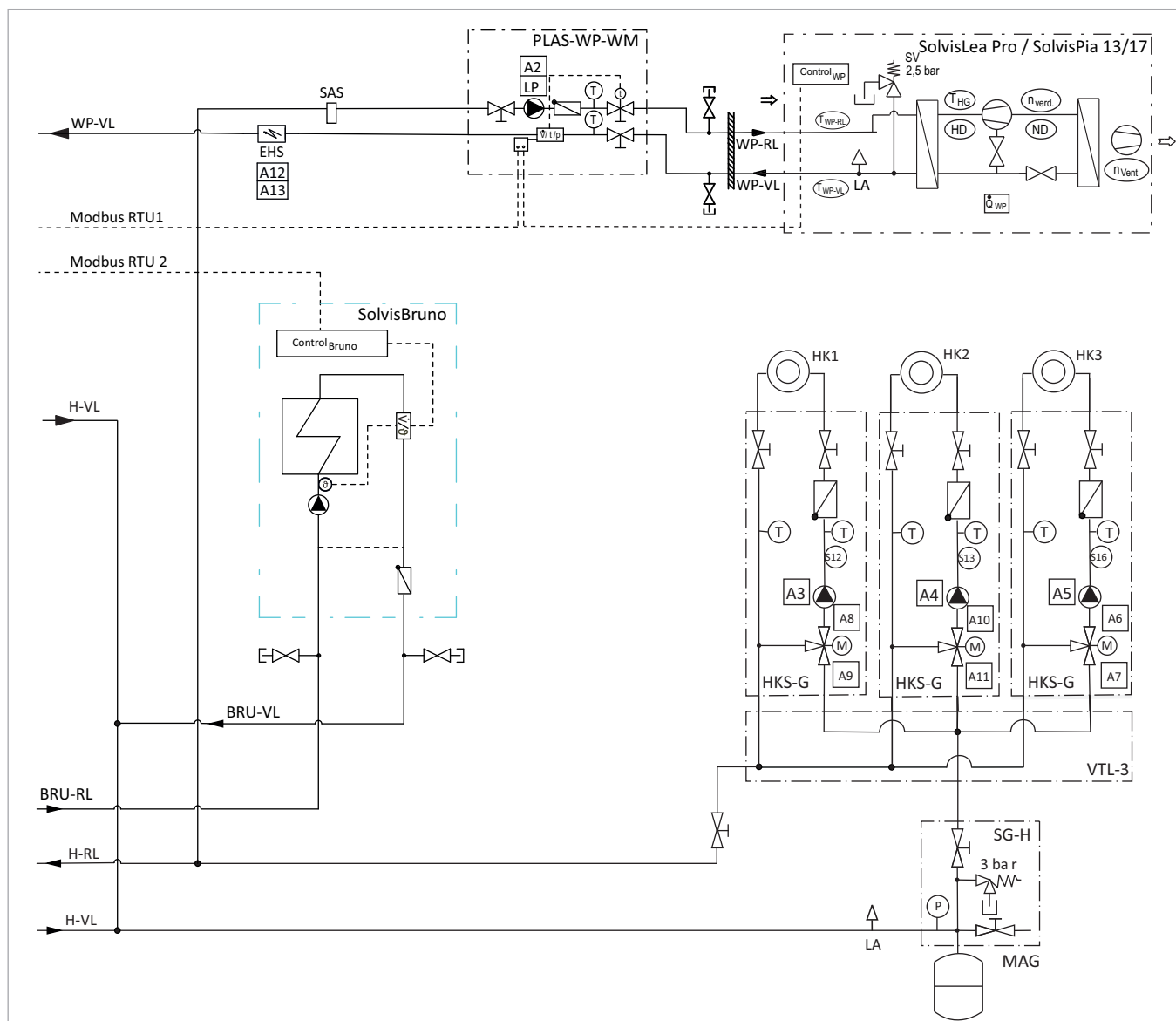
Abb. 41 Anlagenschema SolvisMax Solo der Baureihe 6 mit SolvisBruno, drei Heizkreise und Wärmepumpe - Teil 2 von 2
