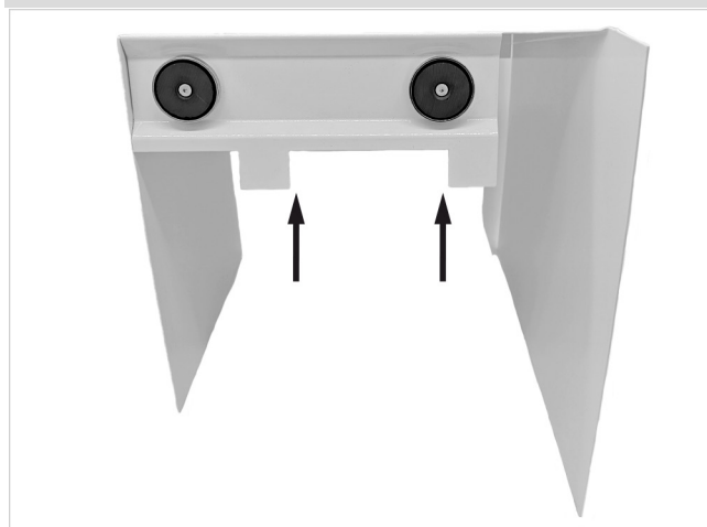
Abb. 2: Aussparung für elektrischen Anschlussstecker für korrekte Ausrichtung der Abdeckhaube
